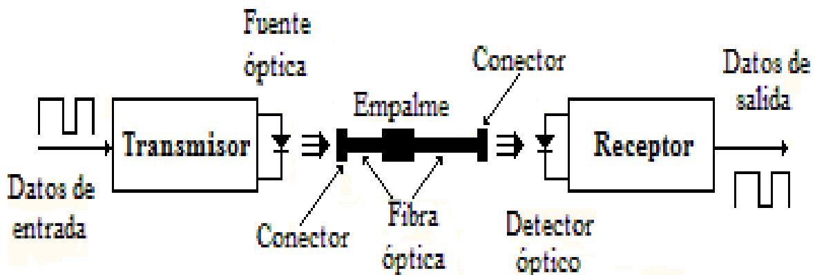
Figura 2.2.3 Enlace de comunicaciones punto a punto por fibras ópticas
