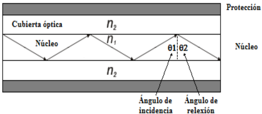
Figura 2.2.7 Estructura de una fibra óptica
