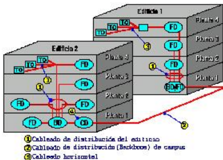
Figura 4.3.4 Varios edificios interconectados
