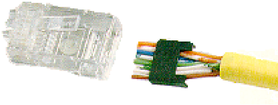
Figura 3.2.3 Conector RJ-45 sujetando al cable par trenzado
