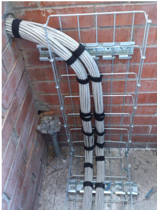
Figura 6.4.4 Instalación de escalerilla en Site de CTI
