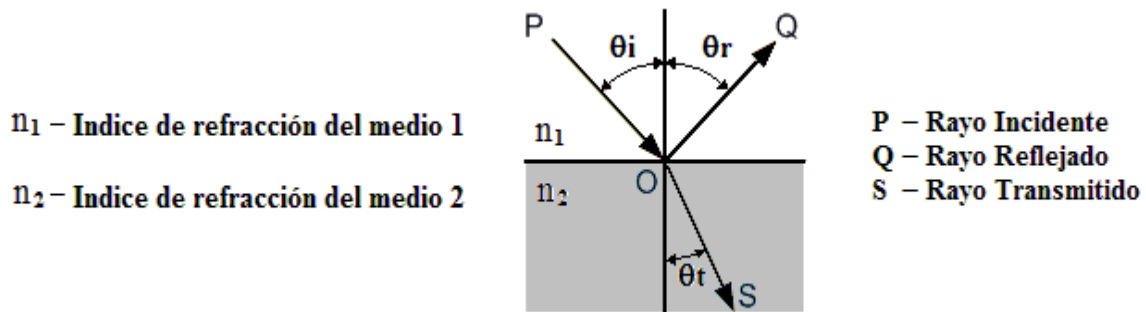
Figura 2.2.6 Representación de la reflexión y transmisión de una rayo al incidir en la frontera de dos medios
