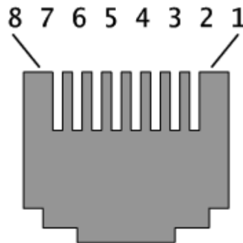
Figura 3.2.2 Vista frontal del conector RJ-45
