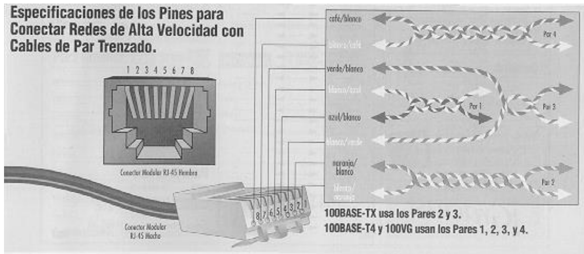
Figura 3.2.1 Conector RJ-45 con 8 contactos
