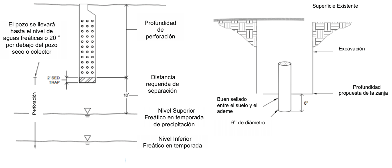
Figura 3.2.- Diagrama muestra para infiltración de agua pluvial según lo recomienda la Norma de Portland
