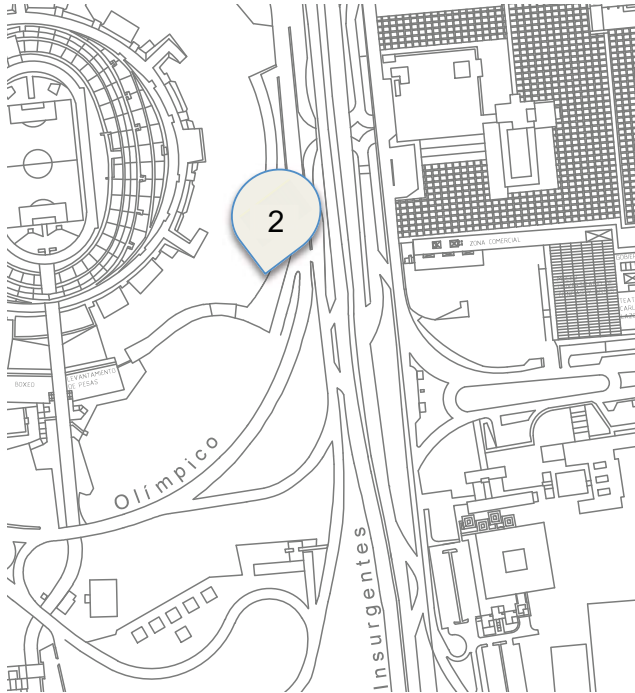
Figura B4.- El Pozo del Estadio Olímpico se encuentra debajo de la Av. de los insurgentes, lo que ocasiona la contaminación del agua de lluvia con grasas y aceites de los automóviles.
