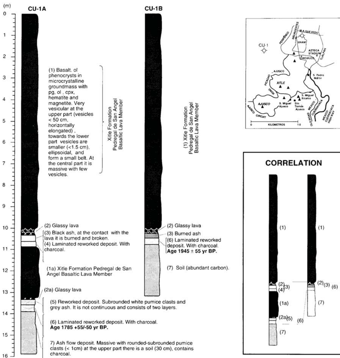
Figura A4.- Sondeo CU
