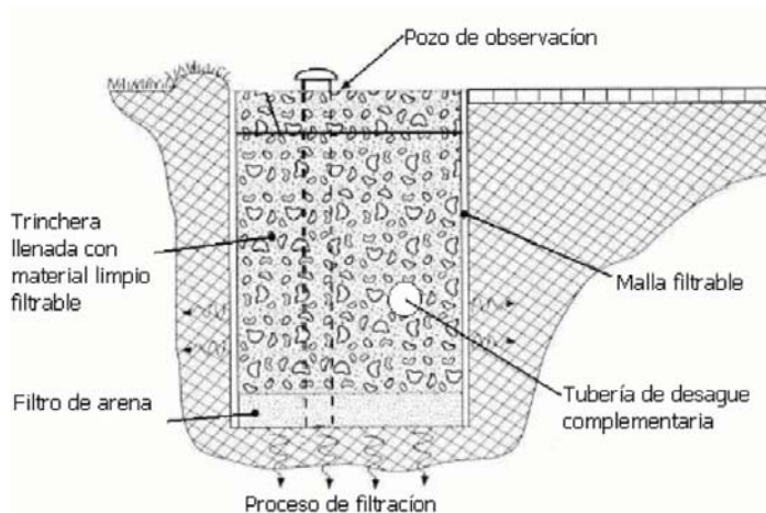
Figura 2.6.- Estructura de una trinchera de infiltración
