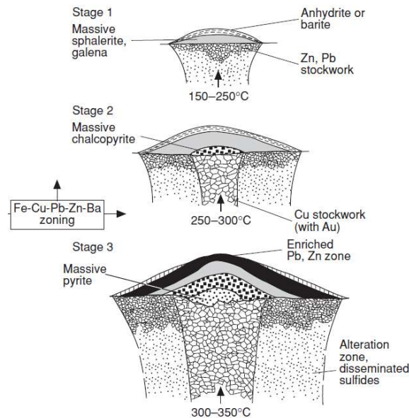
Figura 2.6 Modelo secular explicando la formación de fluidos en un yacimiento tipo VMS (Laurence, 2005).
