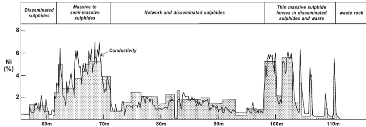
Figura 4.4. Gráfica de un yacimiento de Níquel de la mina Enonkoski, Finlandia, en la que se muestran los porcentajes de este a diferentes profundidades. La gráfica está superpuesta a un registro de conductividad (Fullagar, 1997).
