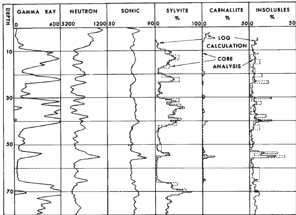
Figura 4.3. Comparación de un núcleo de barrenación con un registro geofísico de pozo en la formación de evaporita Prairie, Canada. Las unidades son convencionales para cada curva registrada (Tixier, 1970).
