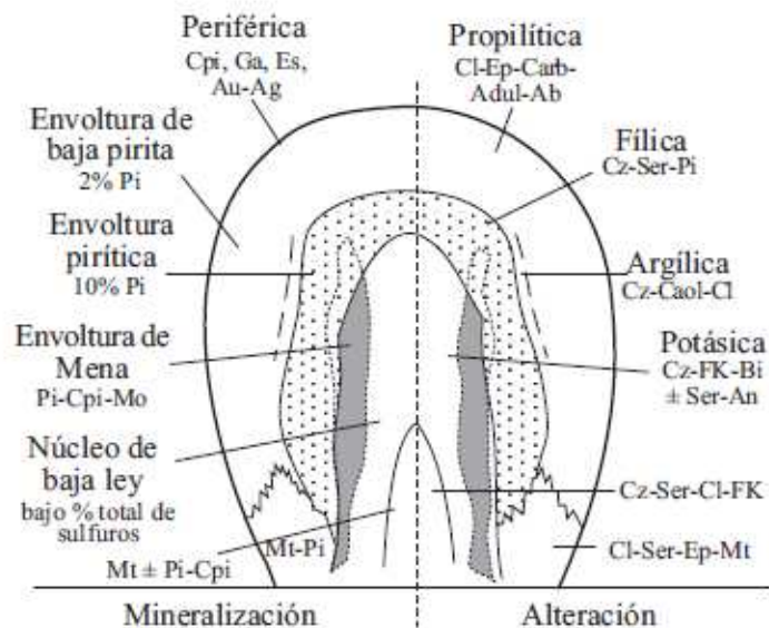
Fig. 2.2 Zonamiento vertical y lateral de la alteración y mineralización típico de los pórfidos de cobre (Valencia- Moreno et al, 2006).
