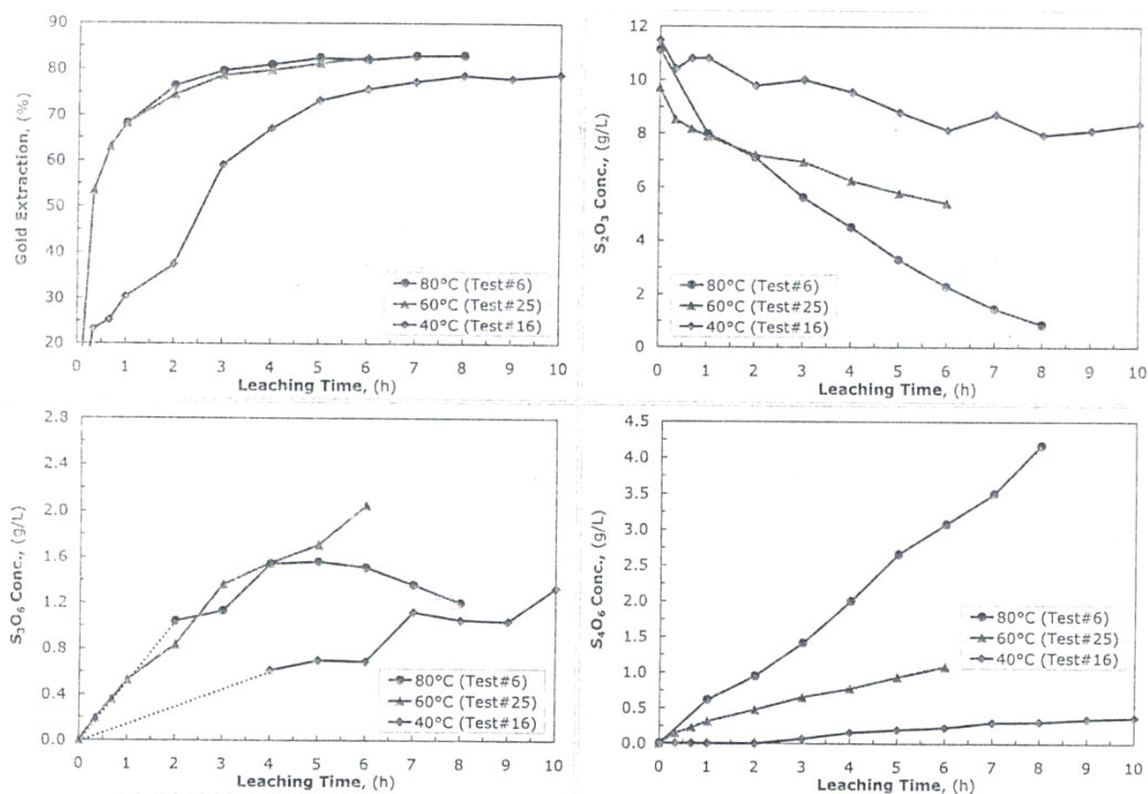
Fig. IV.II.III Efecto de la temperatura sobre la extracción de oro y la degradación del tiosulfato (Se utilizó agua destilada para la molienda, el mineral utilizado fue el 80% del acumulado con un tamaño de 75 \mu\text{m} , \text{Na}_2\text{S}_2\text{O}_3 0.1 M, 100 psig de \text{O}_2 , una autoclave SS de 2 l, 730 rpm de agitación, pulpa de 33% densidad y el pH inicial de la pulpa fue de 12 para la prueba No.6 y No.16 y de 11 para la prueba No.25).
