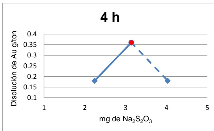
Gráfica 7.3.1. Disolución de Au para la mena a 2 h
