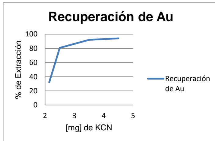
Gráfica. 7.2.5. Comportamiento de la recuperación de Au para la mena.
