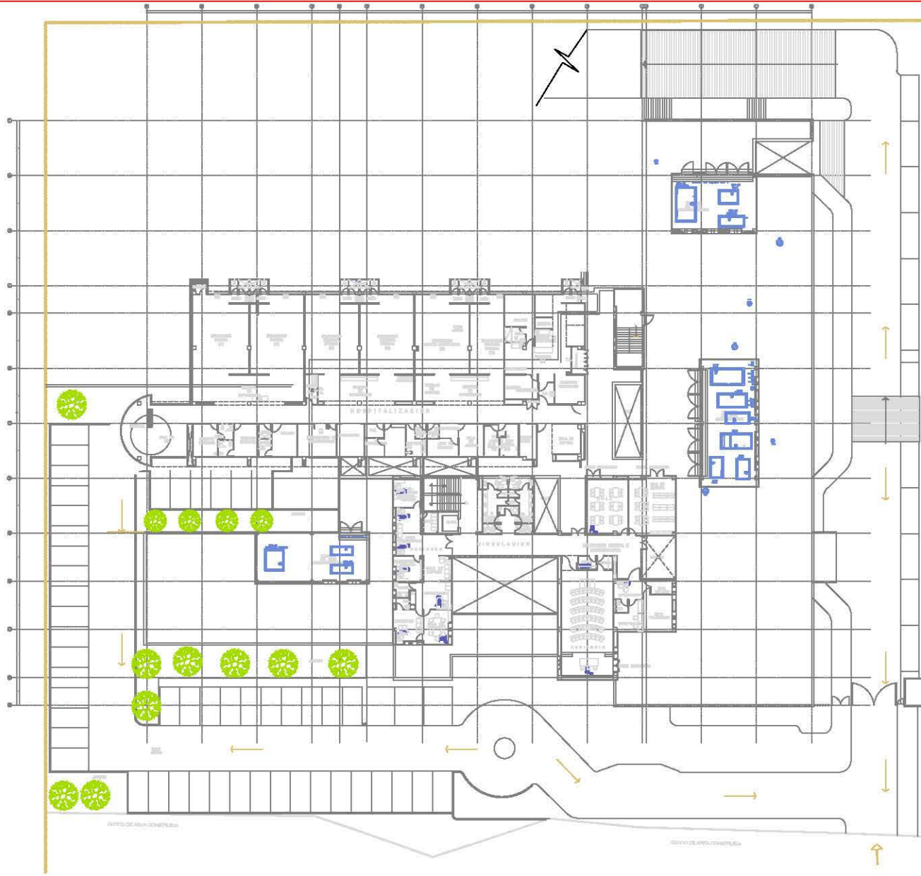
PLANTA ALTA ARQUITECTONICA N.P.T.+4.20
