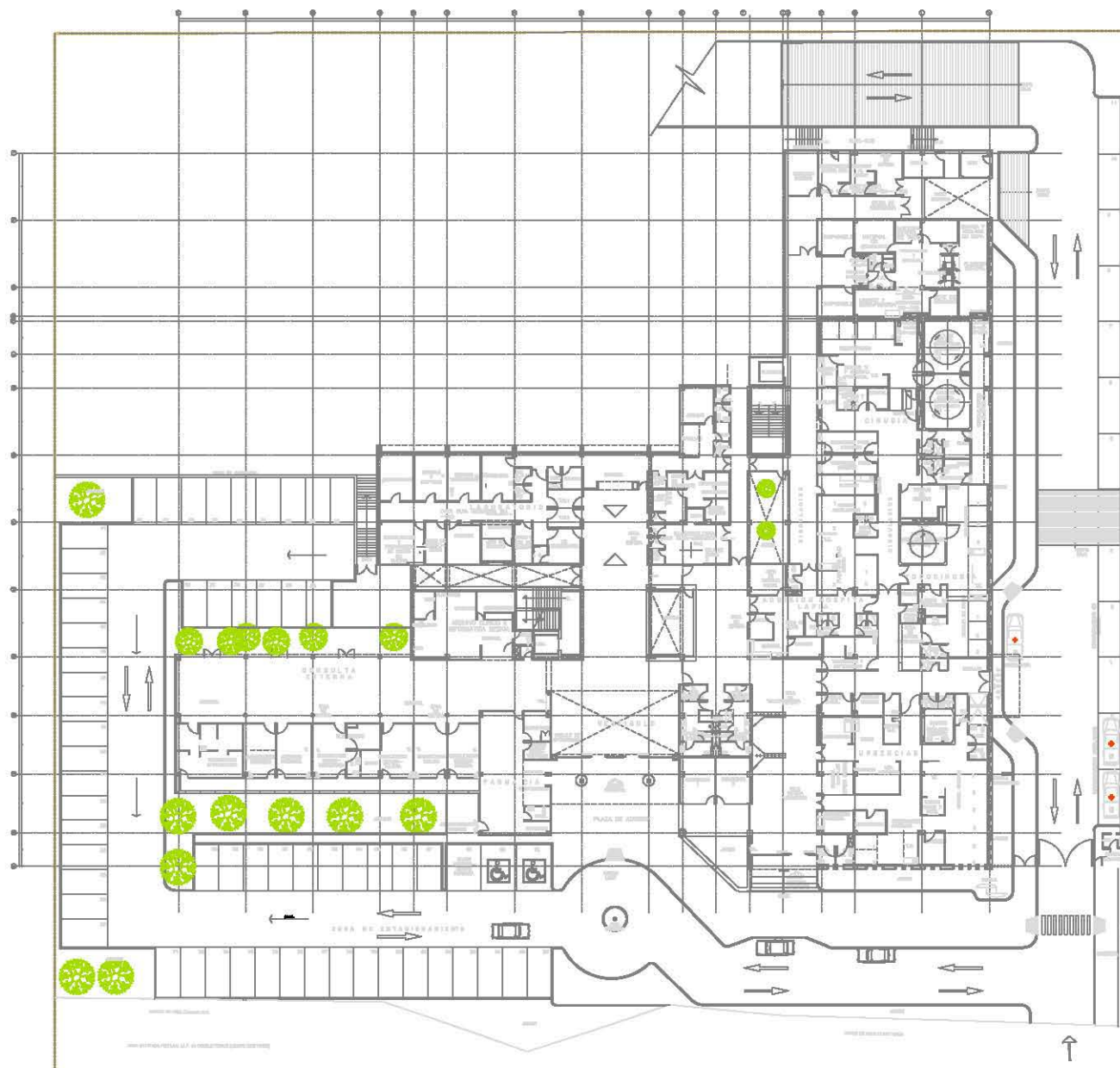
PLANTA BAJA ARQUITECTONICA N.P.T. ± 0.00
