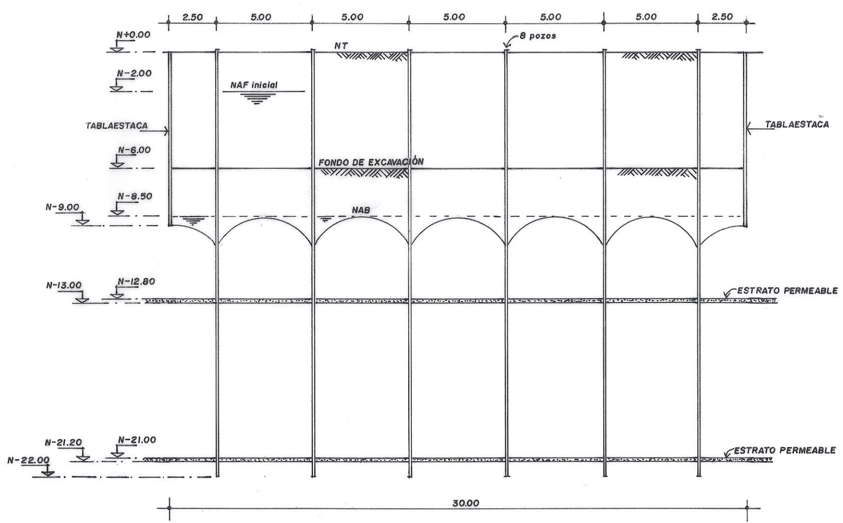
DISTRIBUCIÓN DE POZOS DE BOMBEO PROFUNDO
