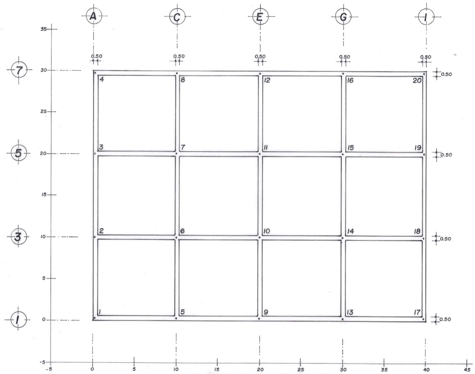
PLANTA DE CONTRATRABES
