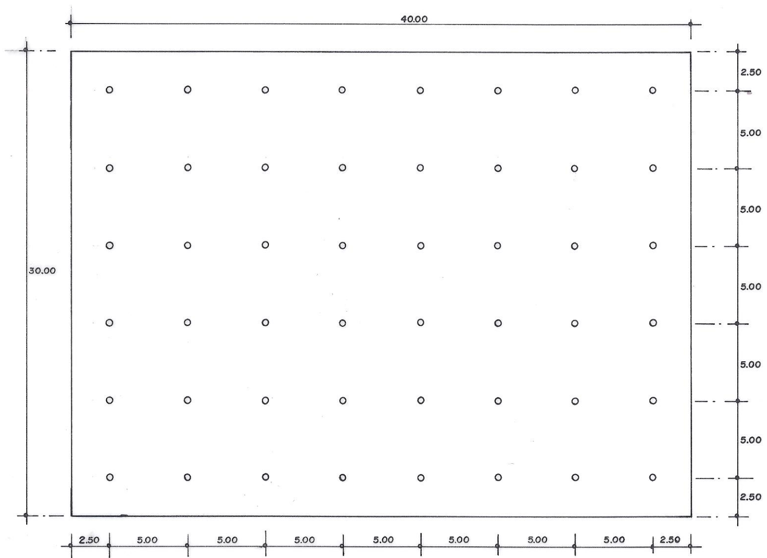
PLANTA DISTRIBUCIÓN DE POZOS DE BOMBEO PROFUNDO
