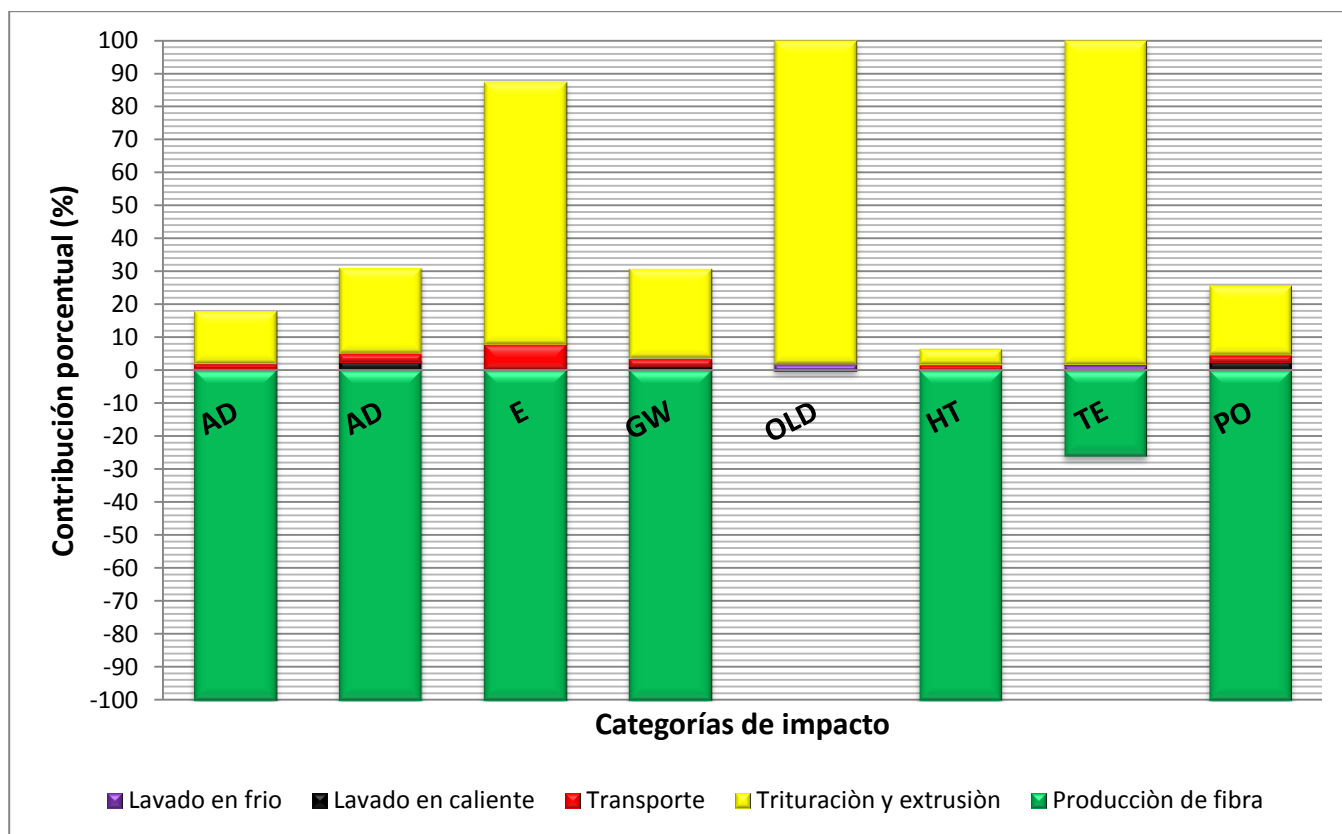
Figura 28. Contribución porcentual de cada operación proceso en el reciclaje de las botellas a fibra de poliéster.
