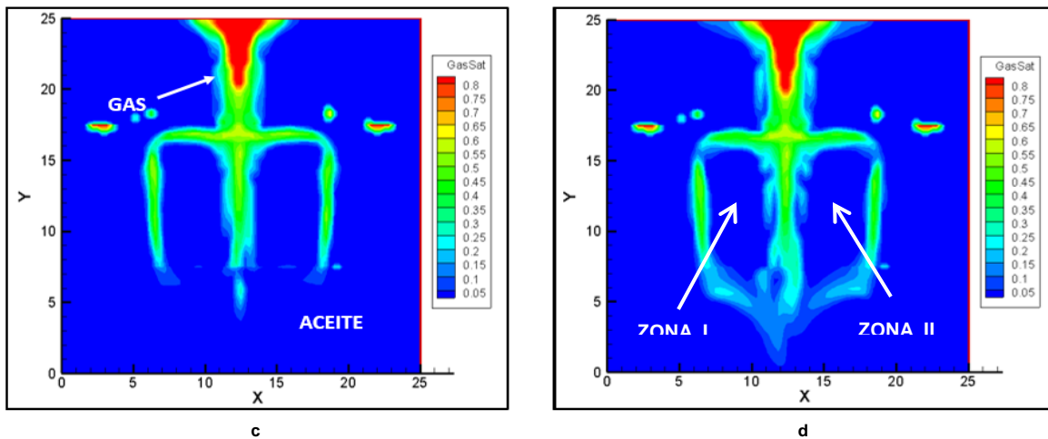
Figura 6.7. c y d. Inestabilidad en la canalización de \text{CO}_2 con un pseudo-gasto de 25 \text{ m}^2/\text{día} .
