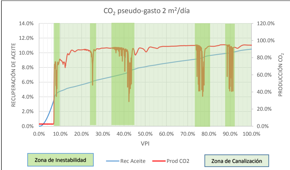
Figura 6.2. Recuperación de aceite y producción de CO 2 a un pseudo-gasto de 2 m 2 /día.
