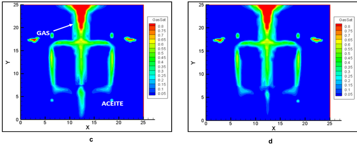
Figura 6.8. c y d. Inestabilidad en la canalización de CO 2 con un pseudo-gasto de 30 m 2 /día.
