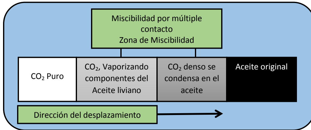
Figura 2.4 Zonas que se presentan en el proceso de miscibilidad. 19
