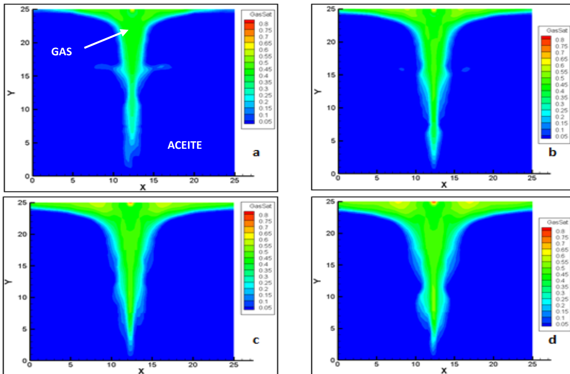
Figura 5.6. Saturación de gas arrojado por la simulación a diferentes volúmenes de inyección de poro.
