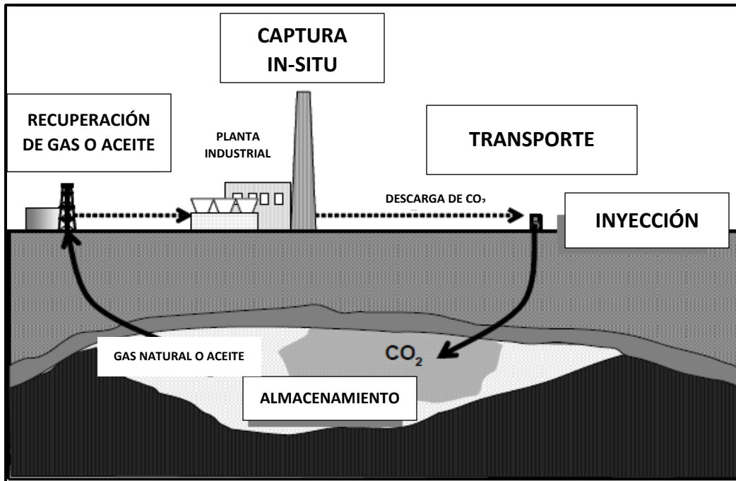
Figura 2.10 Proceso de captura, transporte e inyección de CO 2 . 23
