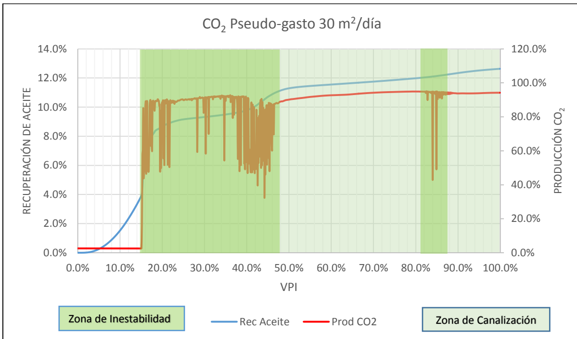
Figura 6.8. Recuperación de aceite y producción de CO 2 a un pseudo-gasto de 30 m 2 /día.
