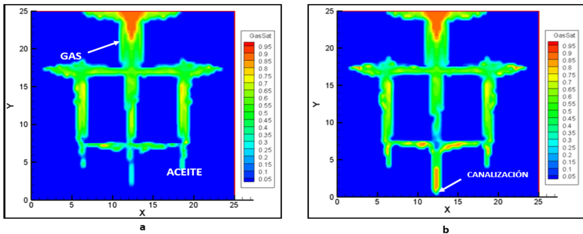
Figura 6.8. a y b. Imagen de VisIt para visualizar el comportamiento antes y durante la canalización de CO 2 con un pseudo-gasto de 30 m 2 /día.
