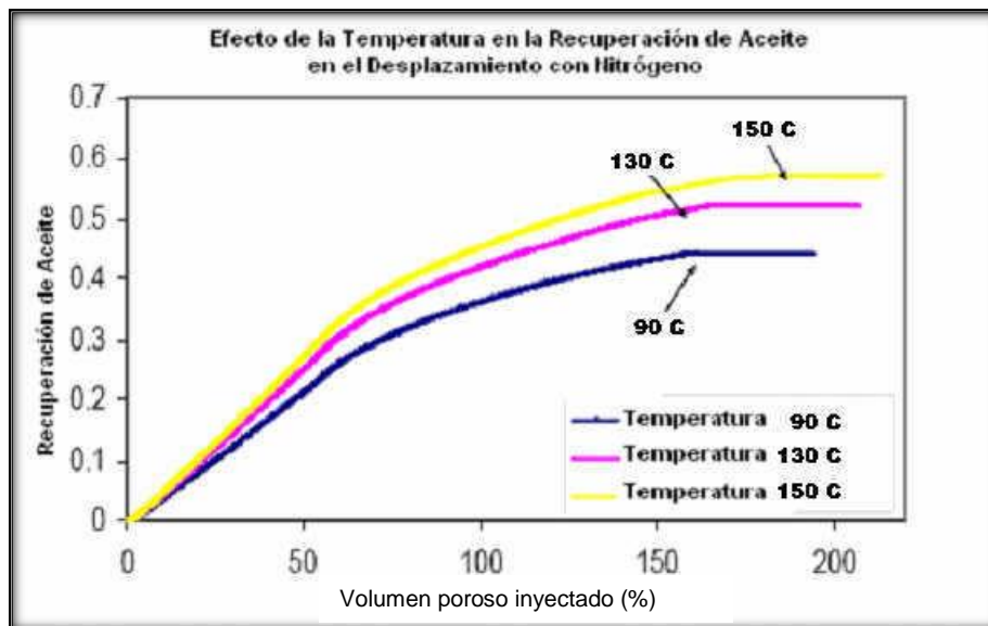
Figura 2.6 Recuperación de aceite por Inyección de N_2 variando la temperatura
