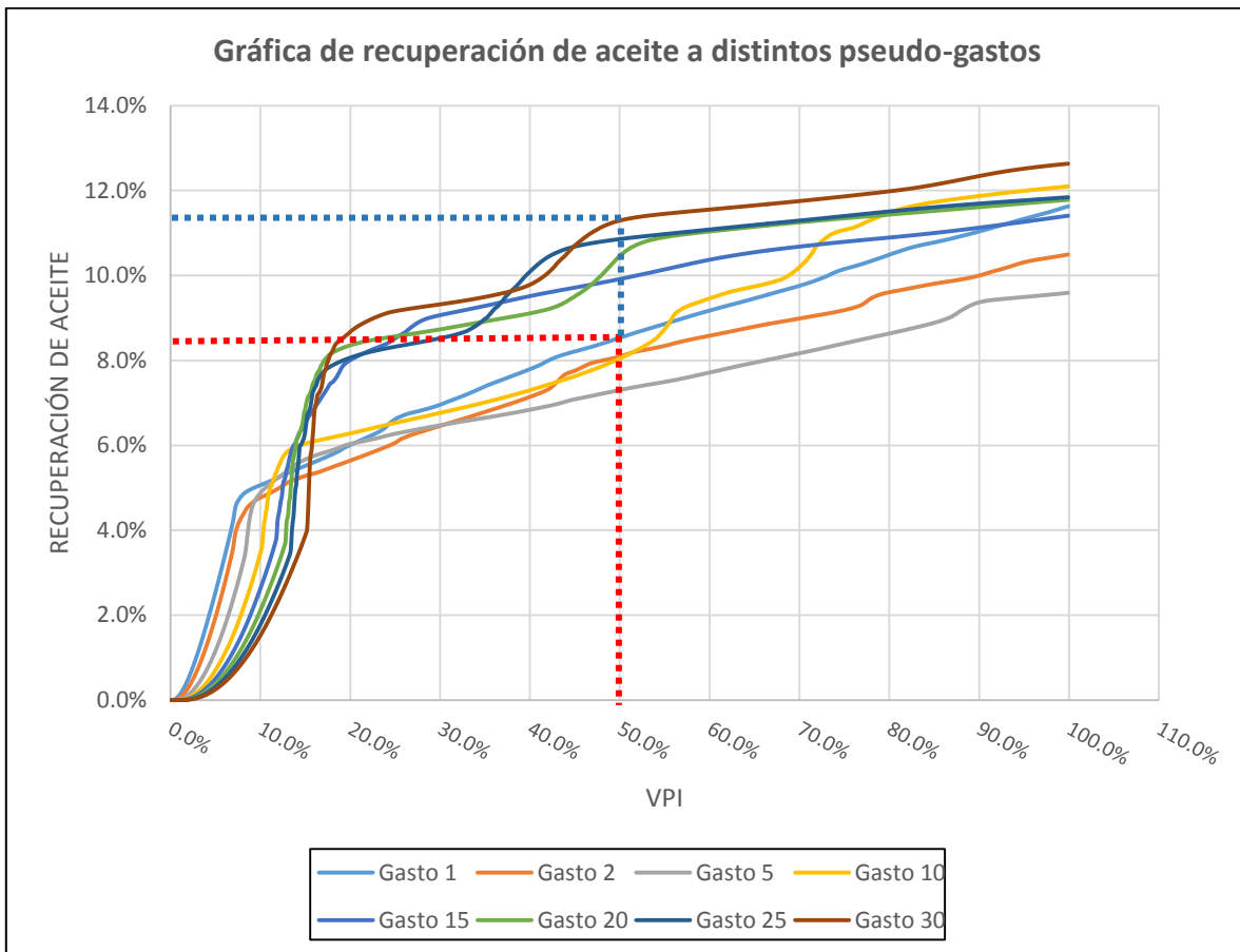
Figura 6.10. Comparativo de la recuperación de aceite con dos diferentes pseudo-gastos para un mismo volumen de poro inyectado.
