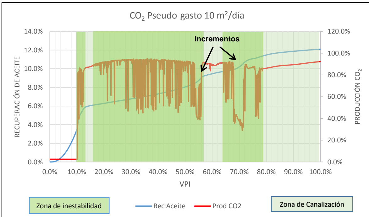
Figura 6.4. Recuperación de aceite y producción de CO 2 a un pseudo-gasto de 10 m 2 /día.
