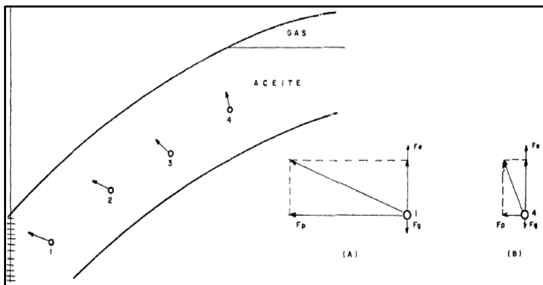
Figura 1.5. Representación de las fuerzas que actúan sobre una burbuja de gas en un yacimiento.
