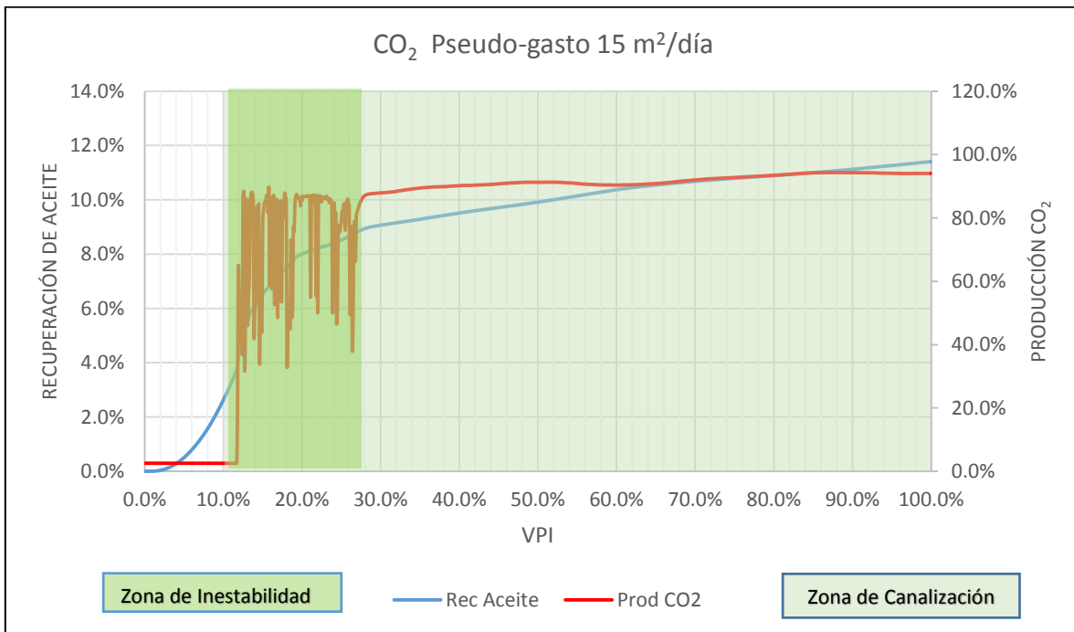
Figura 6.5. Recuperación de aceite y producción de CO 2 a un pseudo-gasto de 15 m 2 /día.
