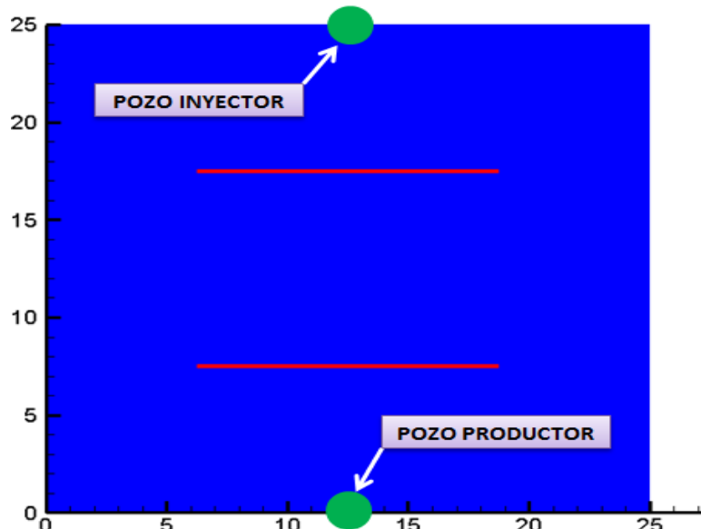
Figura 5.4. Malla de 25 x 25 m donde se localizan los pozos inyector y productor.
