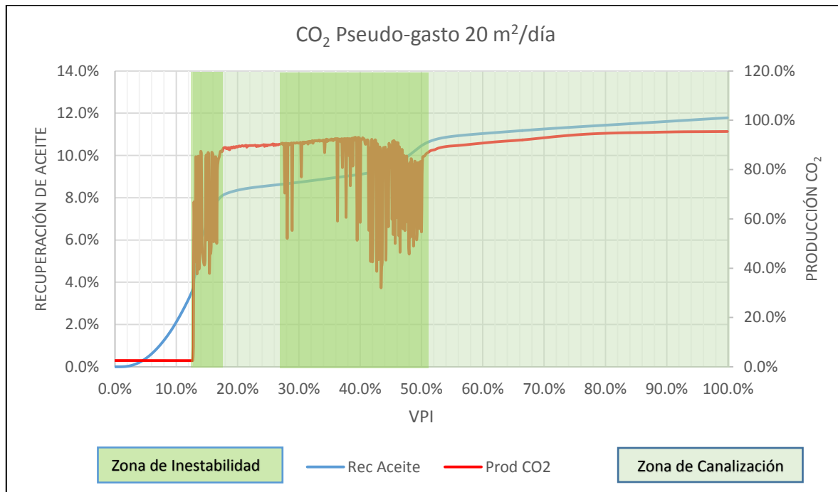
Figura 6.6. Recuperación de aceite y producción de CO 2 a un pseudo-gasto de 20 m 2 /día.
