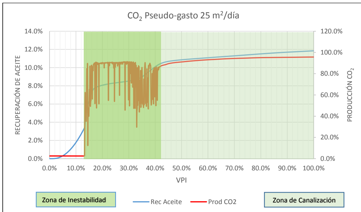
Figura 6.7. Recuperación de aceite y producción de CO 2 a un pseudo-gasto de 25 m 2 /día.
