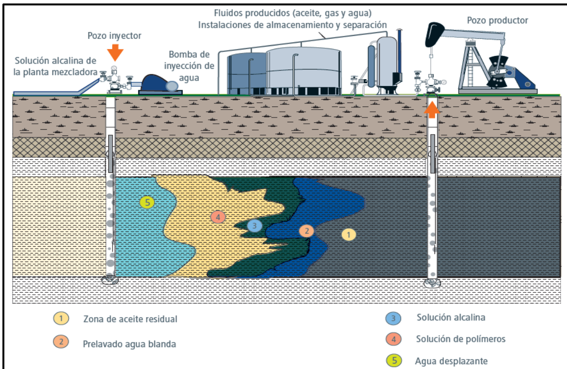
Figura 1.15. Proceso de inyección de alcalinos. 15
