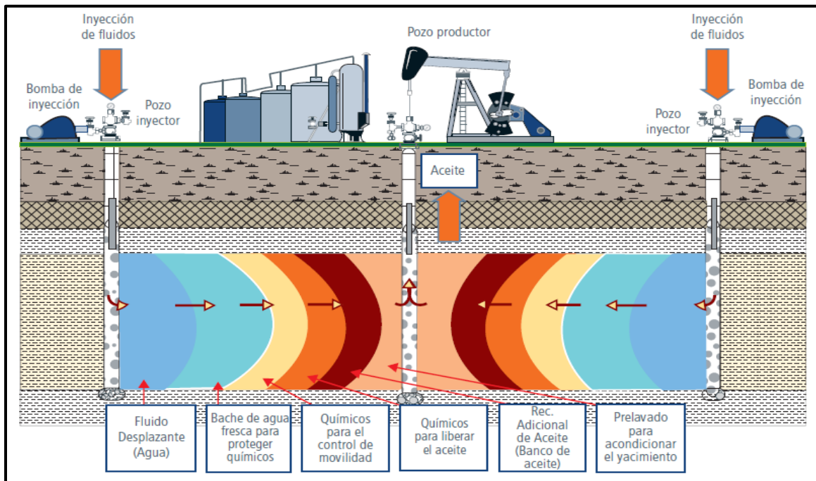
Figura. 1.13. Descripción del proceso de inyección de químicos. 14
