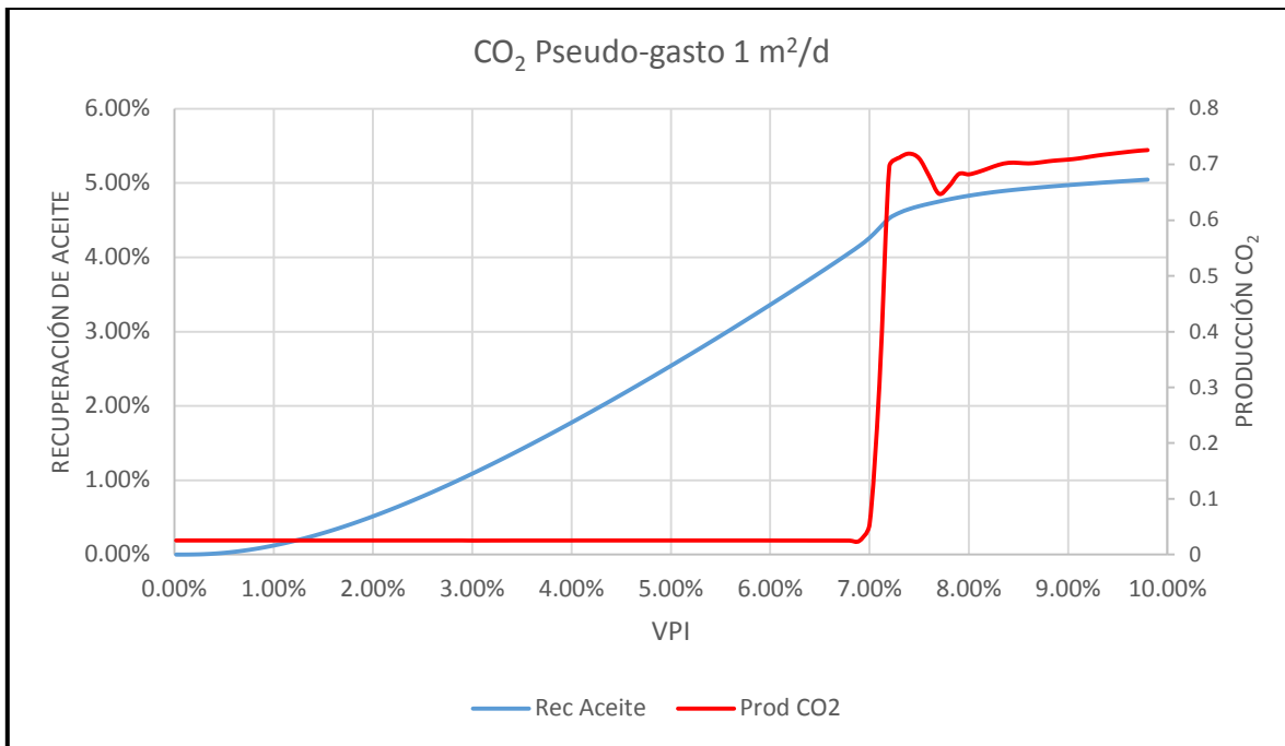
Figura 6.1.c. Recuperación de aceite y producción de CO 2 a un pseudo-gasto de 1 m 2 /día vista hasta el 10 % de volumen de poro.
