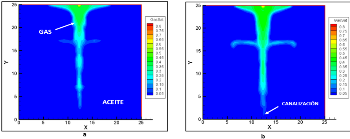
Figura 6.2. a y b. Imagen de VisIt para visualizar el comportamiento antes y durante la canalización de CO 2 con un gasto de 2 m 2 /día.
