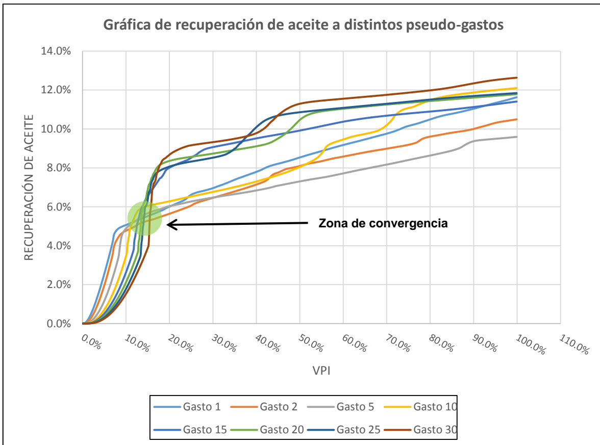
Figura 6.9. Comparativo de recuperación de aceite a diferentes pseudo-gastos.
