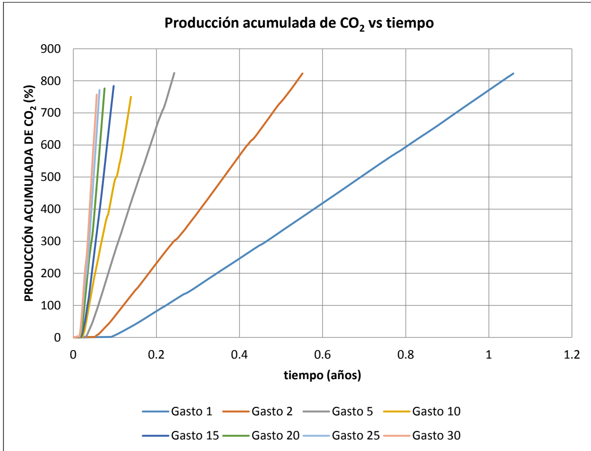
Figura 6.11. Acumulado de producción de CO 2 vs tiempo.
