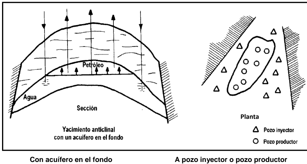
Figura1.7 a. Inyección de agua externa o periférica.
