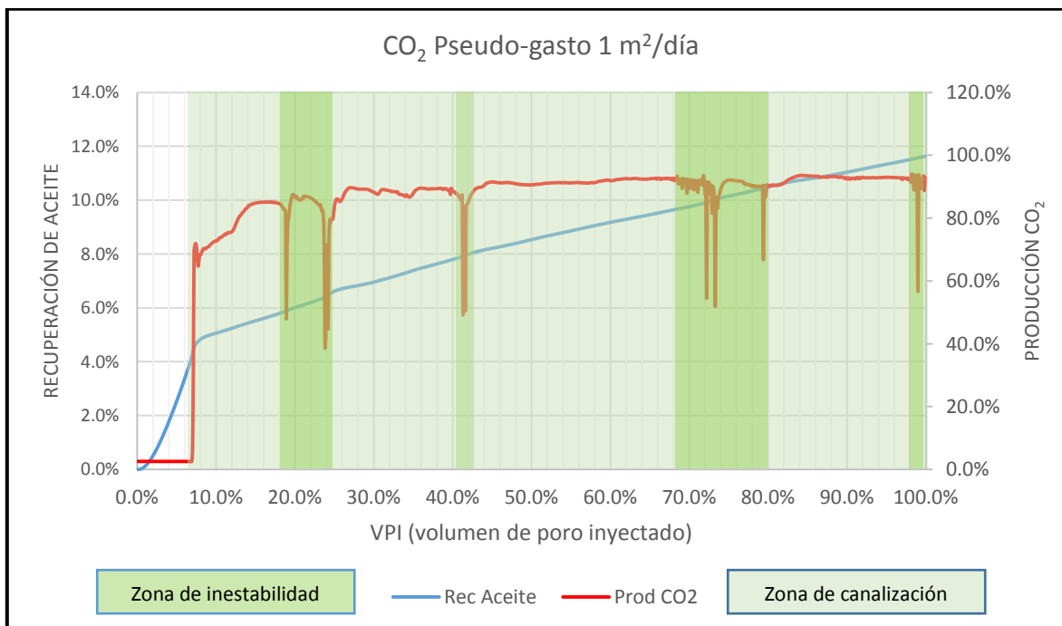
Figura 6.1. Recuperación de aceite y producción de \text{CO}_2 a un pseudo-gasto de 1 \text{ m}^2/\text{día} .
