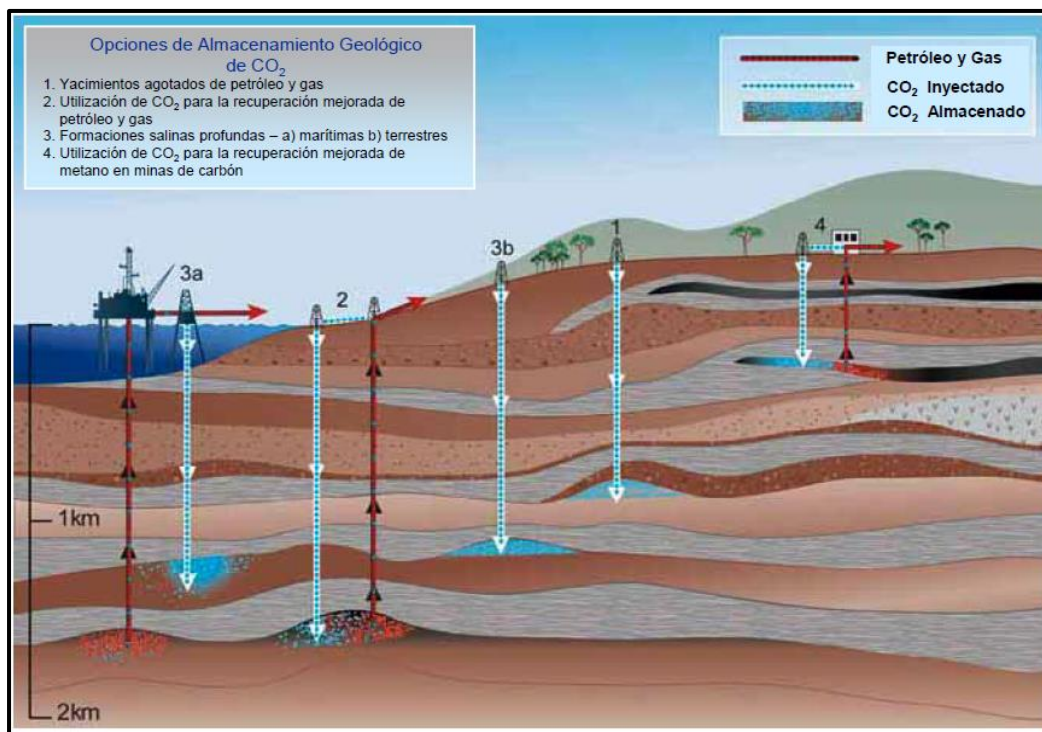
Figura 2.8 Opciones de almacenamiento geológico de CO 2 . 23
