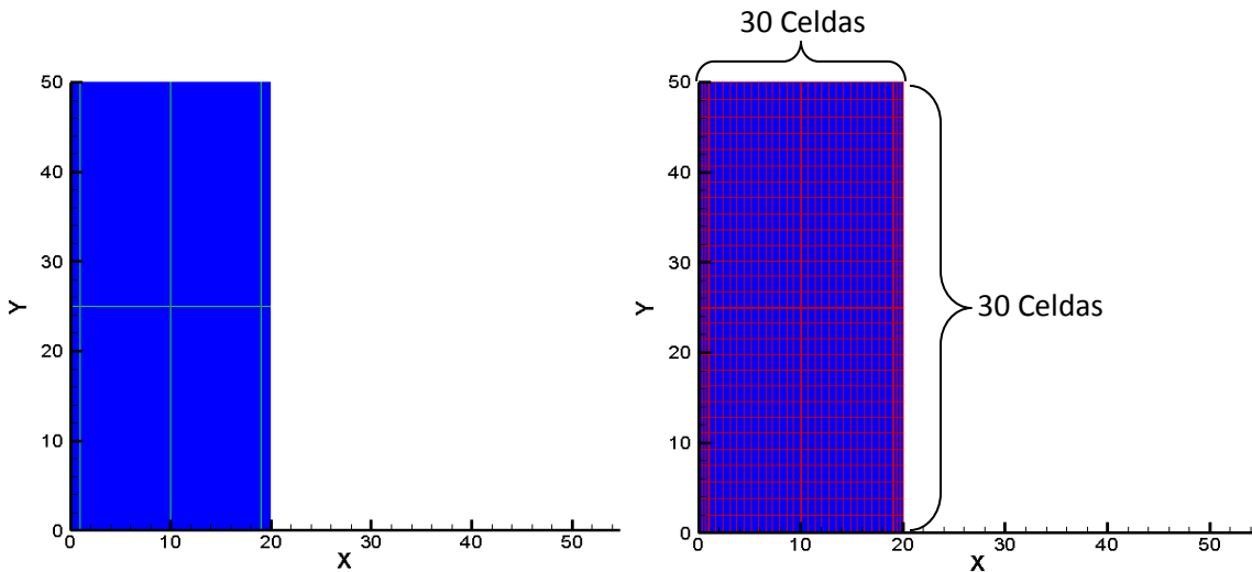
Figura 4.1. Ejemplo ilustrativo para la generación de mallas; con una fractura horizontal y tres fracturas verticales; sin suavizado de malla (figura de la izquierda) y con suavizado (figura de la derecha mx= mz= 0.05).
