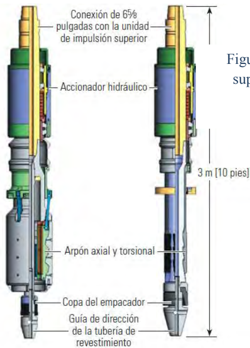
Figura 1.25 Operaciones de perforación y entubación simultáneas con tuberías de revestimiento cortas (liners) o sargas de revestimiento completas.
