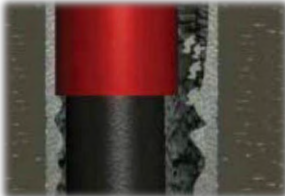
Figura 2.38 La tubería de revestimiento es forzada en la pared del pozo a medida que avanza dentro del agujero.
