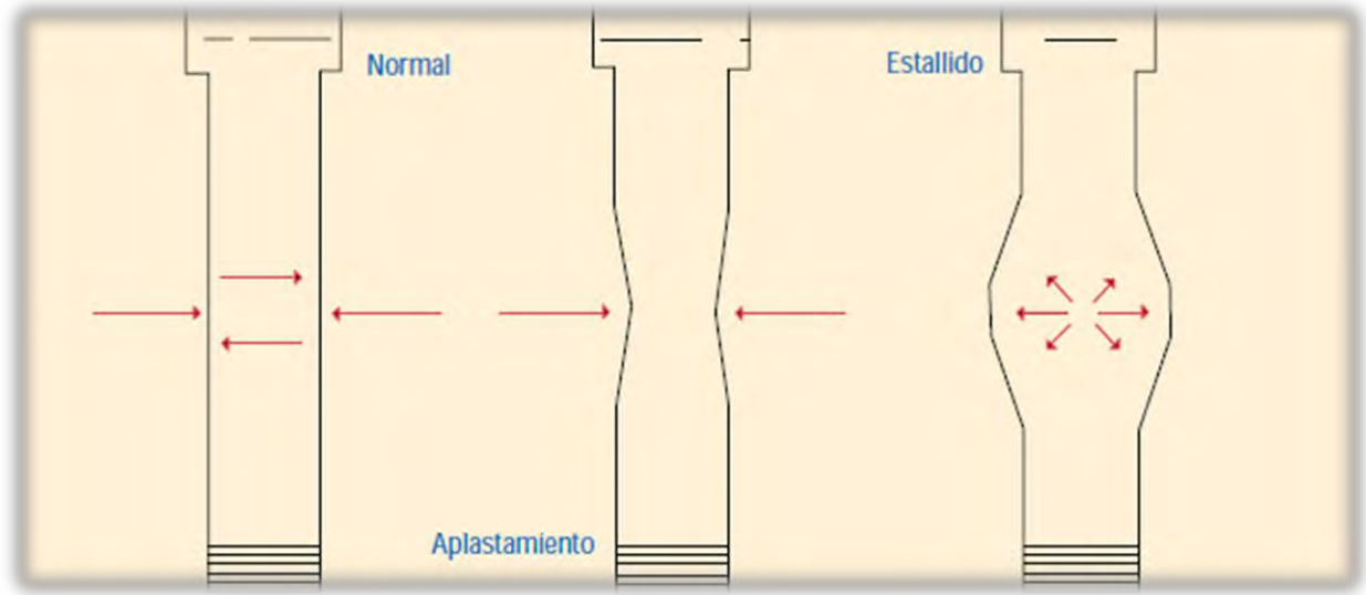
Figura 2.21 Efectos de presión en la TR
