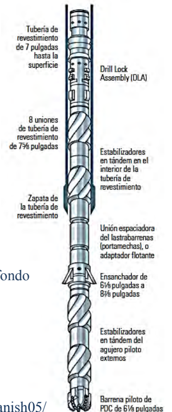
Figura 1.25 Operaciones de perforación y entubación simultáneas con tuberías de revestimiento cortas (liners) o sargas de revestimiento completas.
