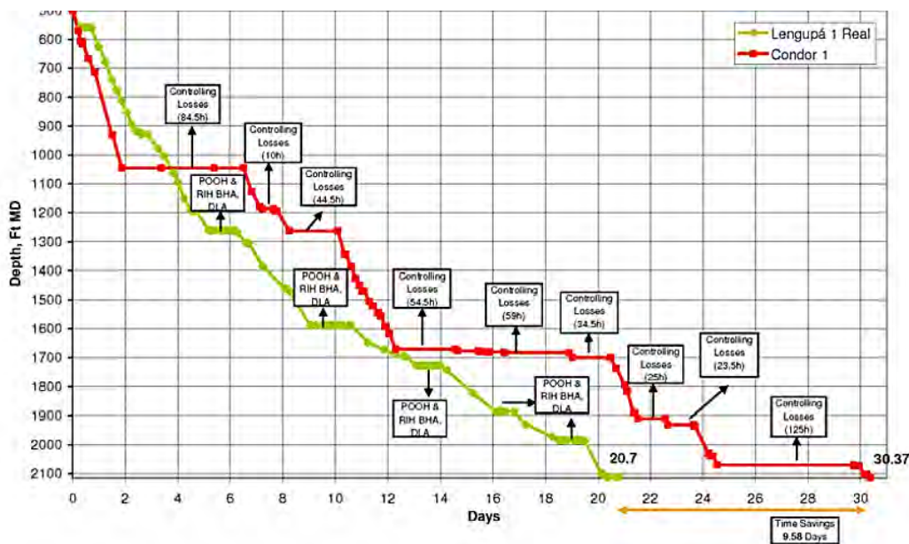
Figura 4.3 Comparación de tiempos entre el pozo Cóndor 1 y los pozos Lengupá 1 y Cóndor 2 para la sección de 17 1/2” .
