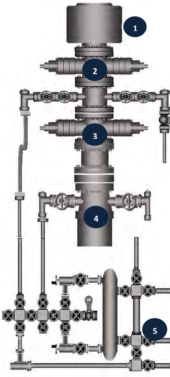
Figura 2.14 Arreglo de preventores
