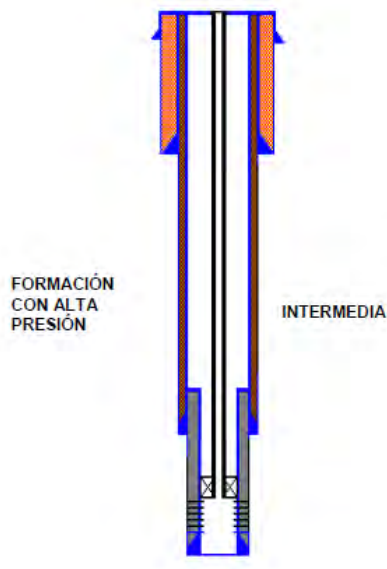
Figura 2.18 Tubería de revestimiento intermedia
