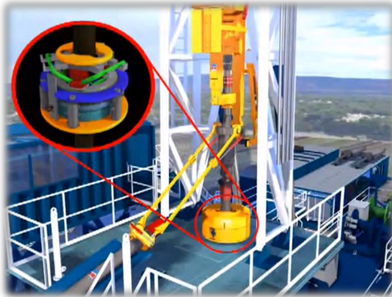
Figura 2.41 Procedimiento de perforación con TR
