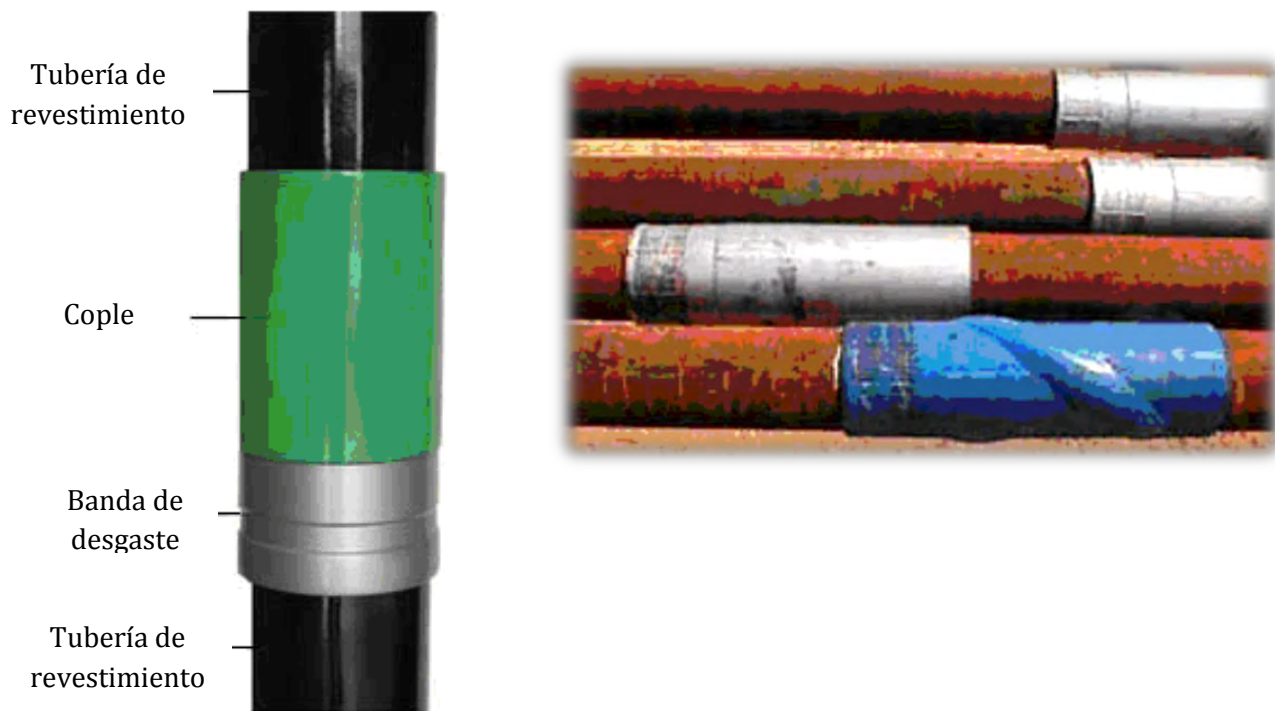
Figura 2.49 Banda de desgaste (izquierda) y Manga de desgaste (Derecha) Fuente: ABUBAKAR Mohammed, Current Trends and Future Development in Casing Drilling. 2012
