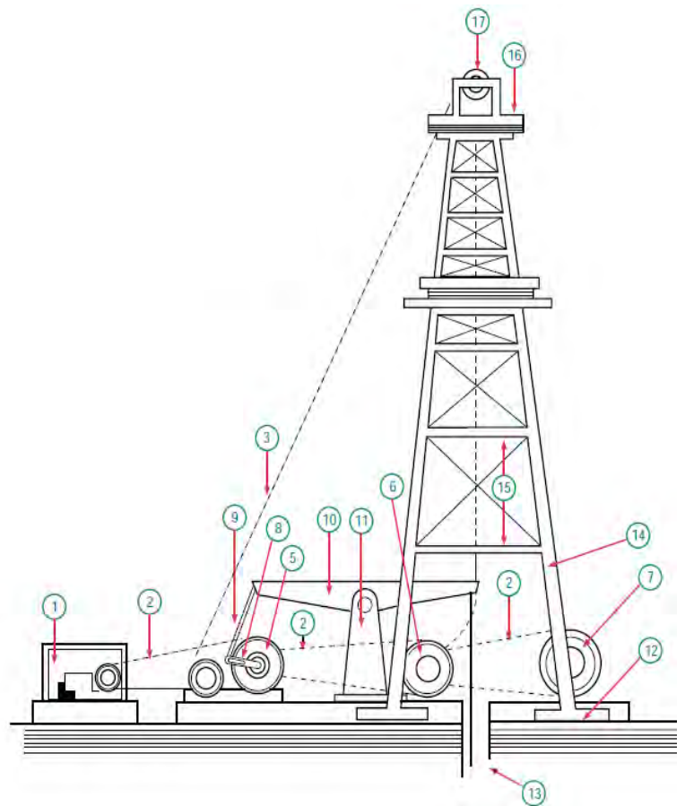
Figura 1.8 Componentes del equipo de perforación a percusión
