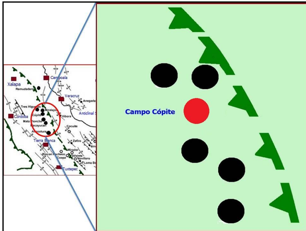
Figura 3.12. Localización del campo Cópite dentro de la Plataforma de Córdoba (Modificada de González, 1976).
