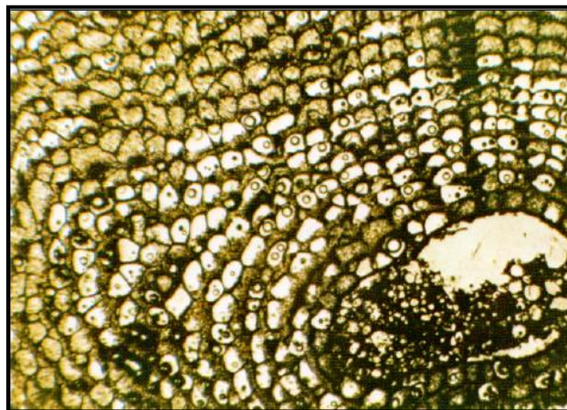
Figura 2.15. Sección de briozoarios Schizoporella floridana en la región de Florida (Tomado de Handford, 2004).
