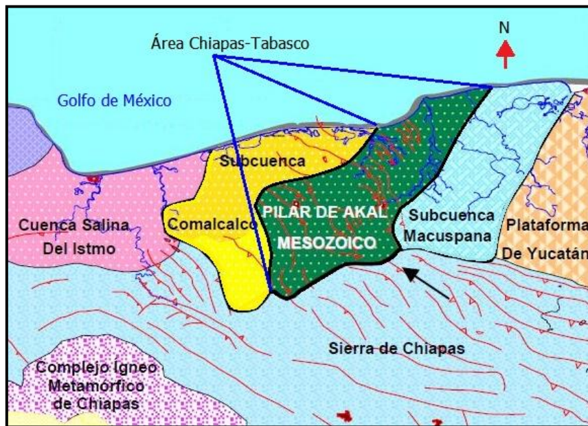
Figura 3.17. Ubicación geográfica del área Chiapas – Tabasco en la Cuenca del Sureste Mexicano (Modificado de Martínez, 2005).
