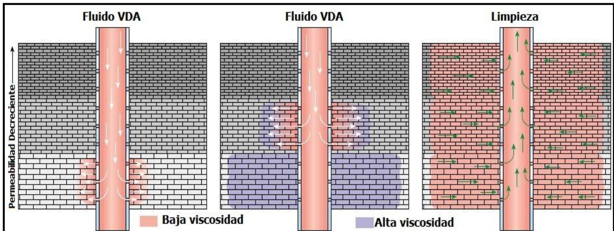
Figura 4.6. Estimulación con divergencia local en carbonatos (tomado de Al-Anzi y Al-Habib, 2004).
