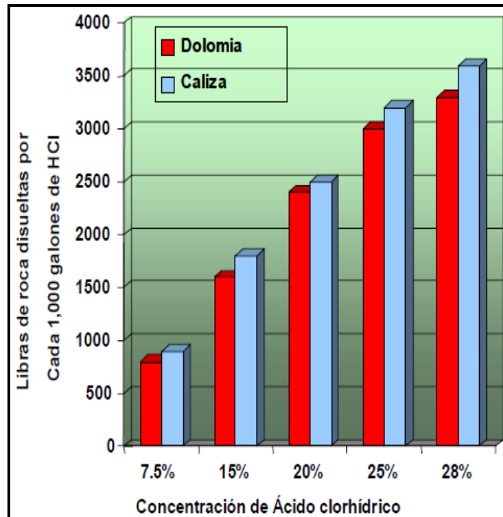
Figura 4.3. Gráfico que muestra la solubilidad del ácido clorhídrico en la caliza y dolomía (Pemex, 2008).
