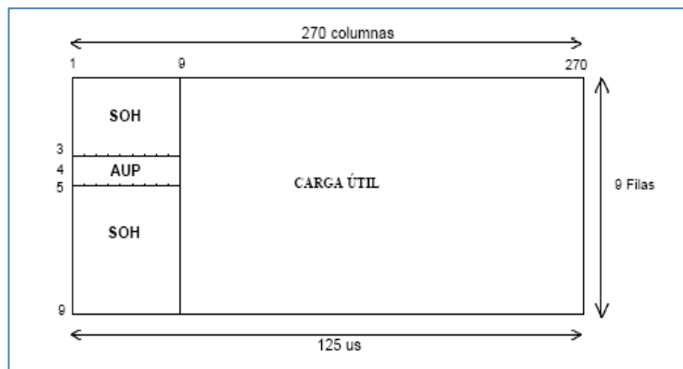
Figura 4.2 Estructura de la trama básica SDH
