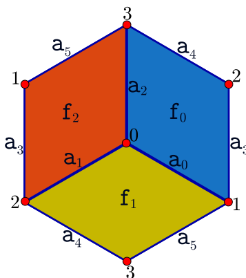
FIGURA 1. Hemicubo
