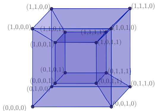
FIGURA 2. 4-cubo.
