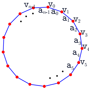
FIGURA 1. n -ágono.
