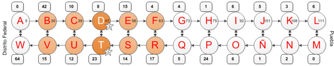
Figura 15. Esquema de red de la autopista México – Puebla, primera instalación seleccionada.
