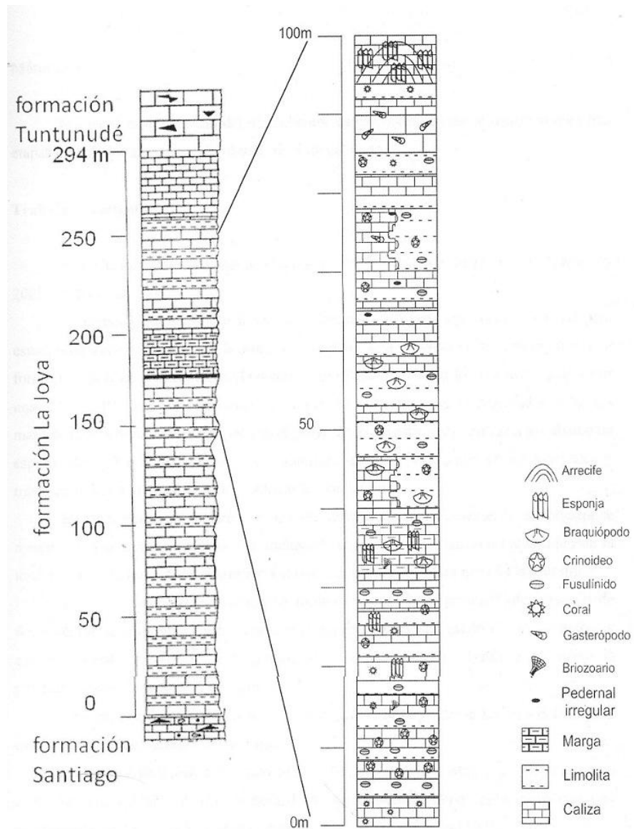
Figura 7. Columna estratigráfica en el arroyo La Joya de la Formación La Joya en la Sierra Agua Verde (Tomado de Ochoa y Sosa, 1993).
