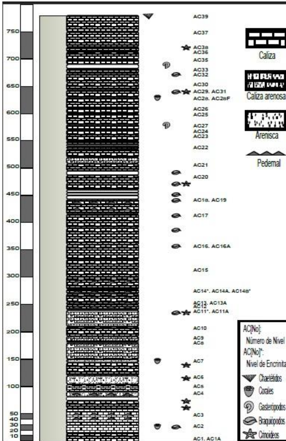
Figura 8. Columna estratigráfica de la localidad Agua Caliente. (Chacón, Garcés, Jiménez y Ortiz, 2012).
