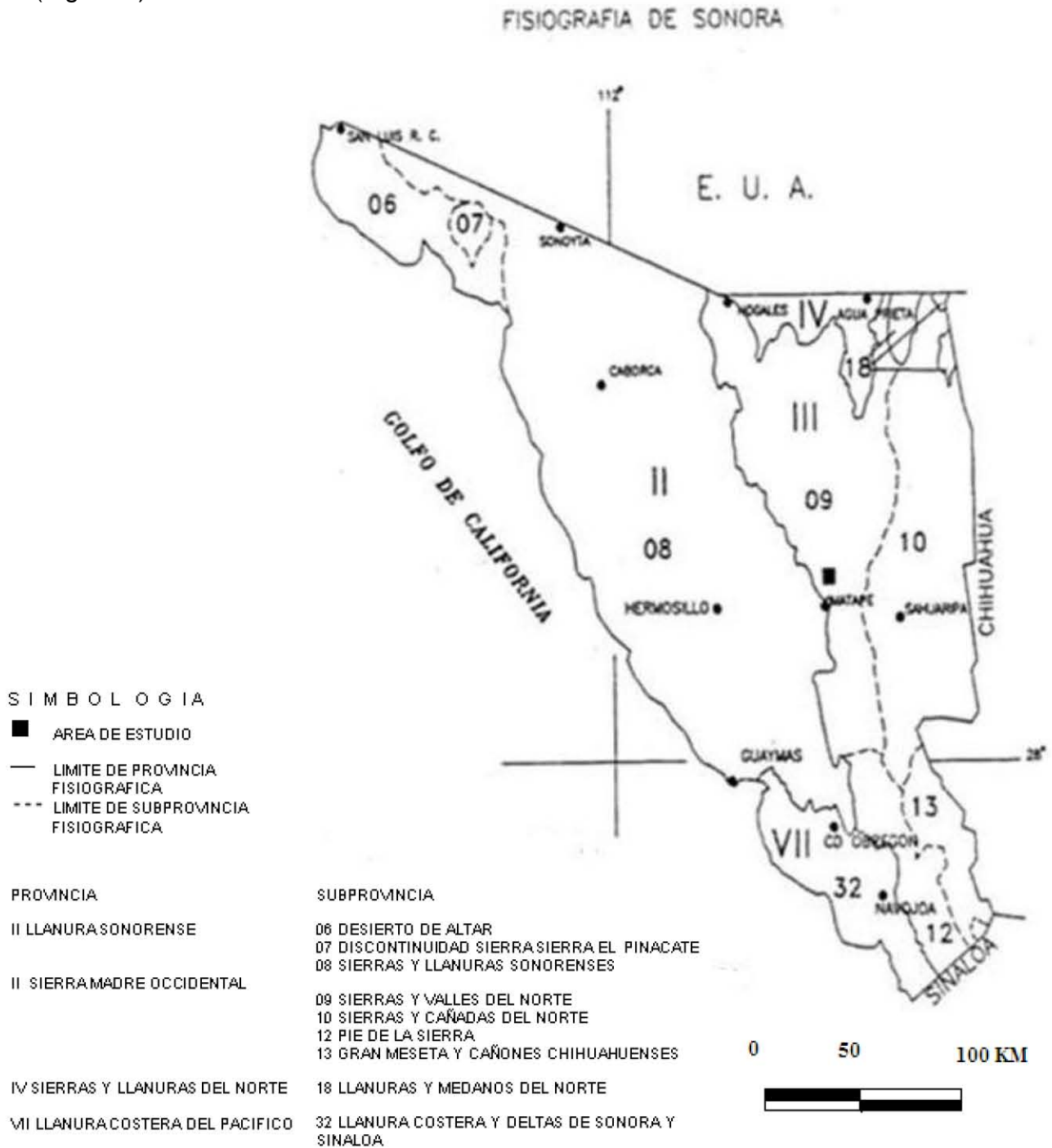
Figura 2. Mapa de las provincias Fisiográficas de Sonora (tomado de Ochoa y Sosa, 1993).
