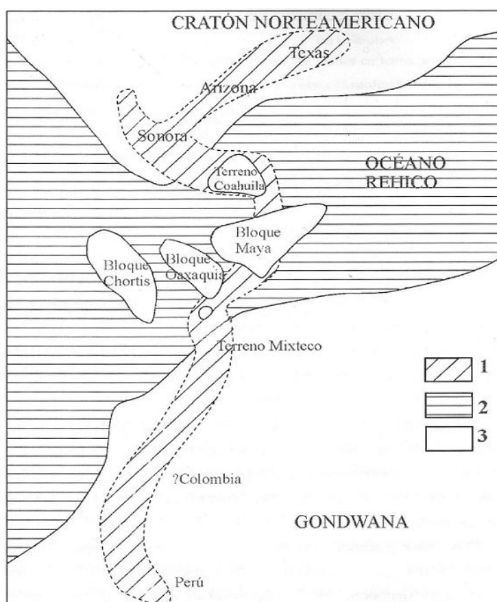
Figura 40. Reconstrucción paleogeográfica donde se muestra la conexión entre Sonora, el cratón norteamericano (Arizona, Texas) y el dominio sudamericano a través de diferentes terrenos mexicanos: Coahuila, Maya, Oaxaquia y Mixteco. 1 plataformas carbonatadas, 2 cuencas de flysch, 3 islas y continentes (Gómez et al. , 2008).
