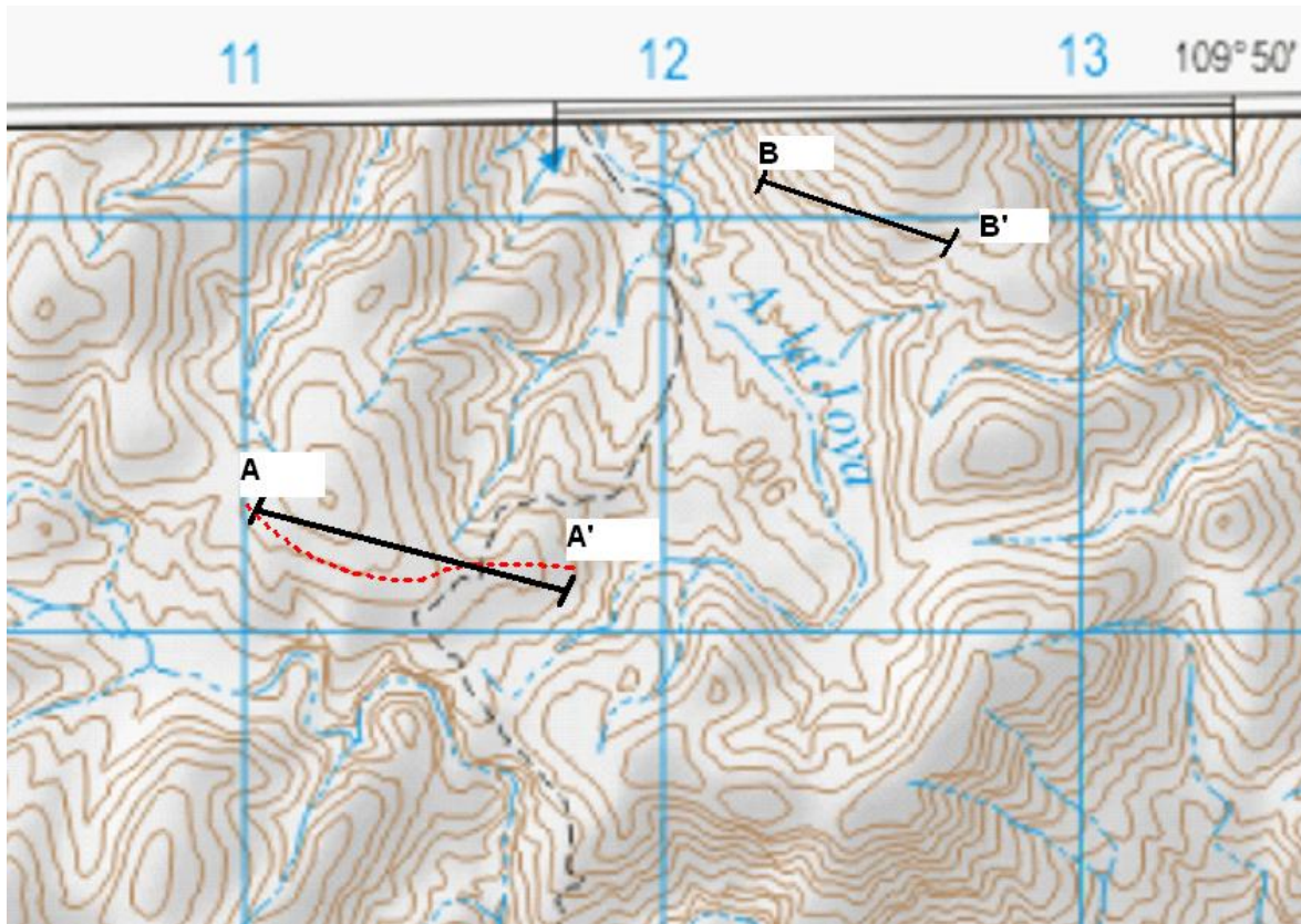
Figura 6. Mapa Topográfico que muestra los transectos estudiados (Carta San José Batúc H12D44).
