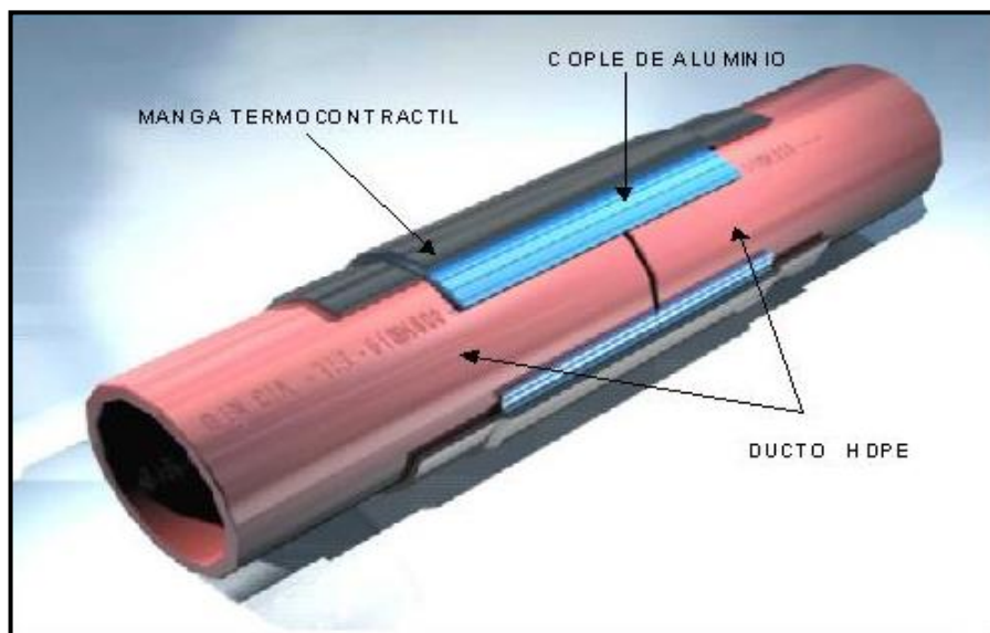
FOTOGRAFÍA 5 “ACOPLAMIENTO DE TUBOS HDPE”
