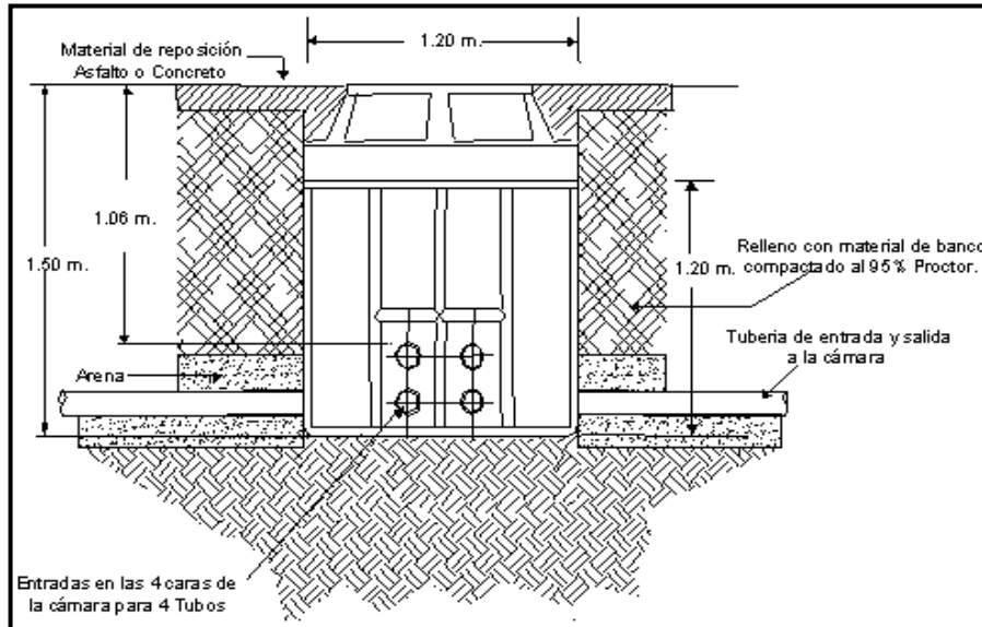
FIGURA 44 “CORTE Y DIMENSIONES DE CÁMARA MANHOLE”
