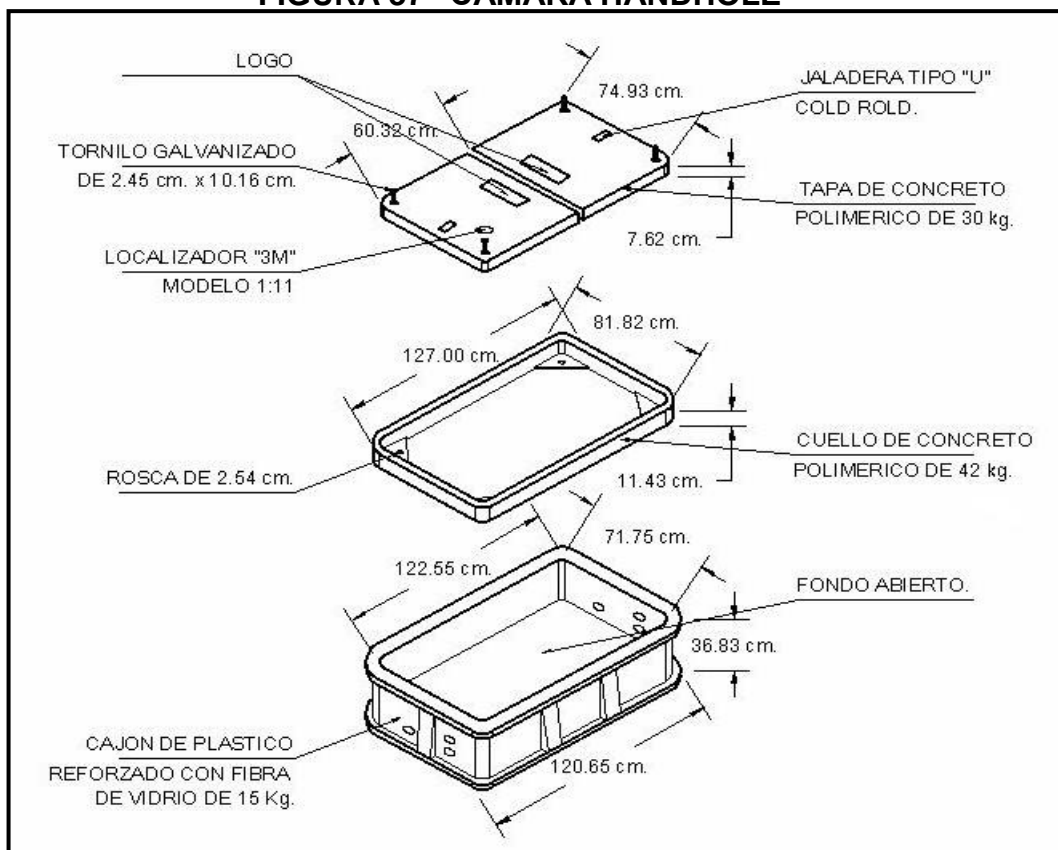
FIGURA 37 “CÁMARA HANDHOLE”
