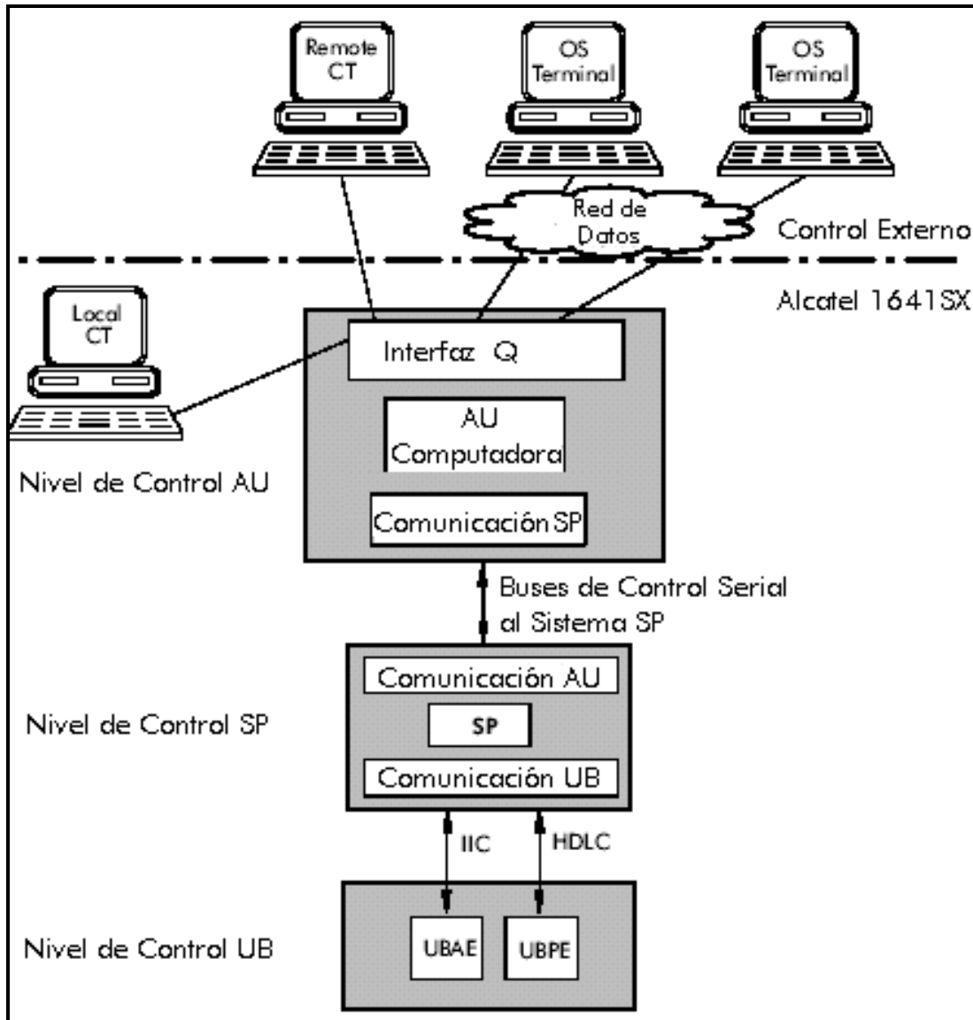
FIGURA 53 "DIAGRAMA DE INTERFACE"
