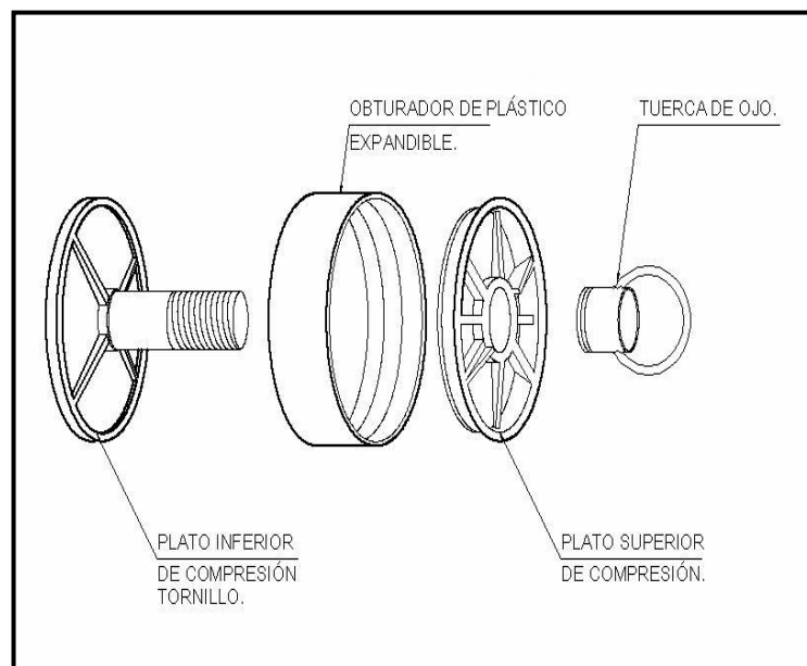
FIGURA 38 “TAPÓN HERMÉTICO DE EXPANSIÓN”
