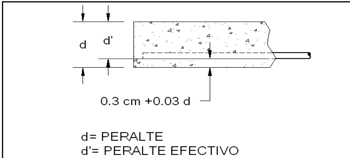
FIGURA 51 "POSICIÓN DE ACERO DE REFUERZO"
