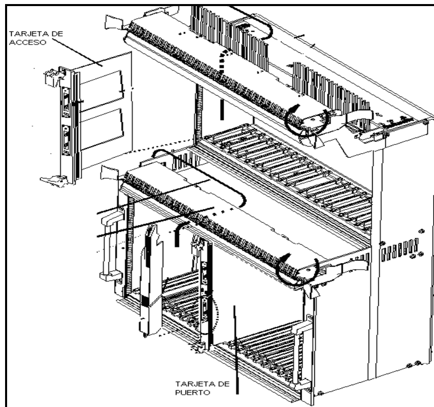
FIGURA 55 “BASTIDOR PARA TARJETAS DE PROGRAMACIÓN”
