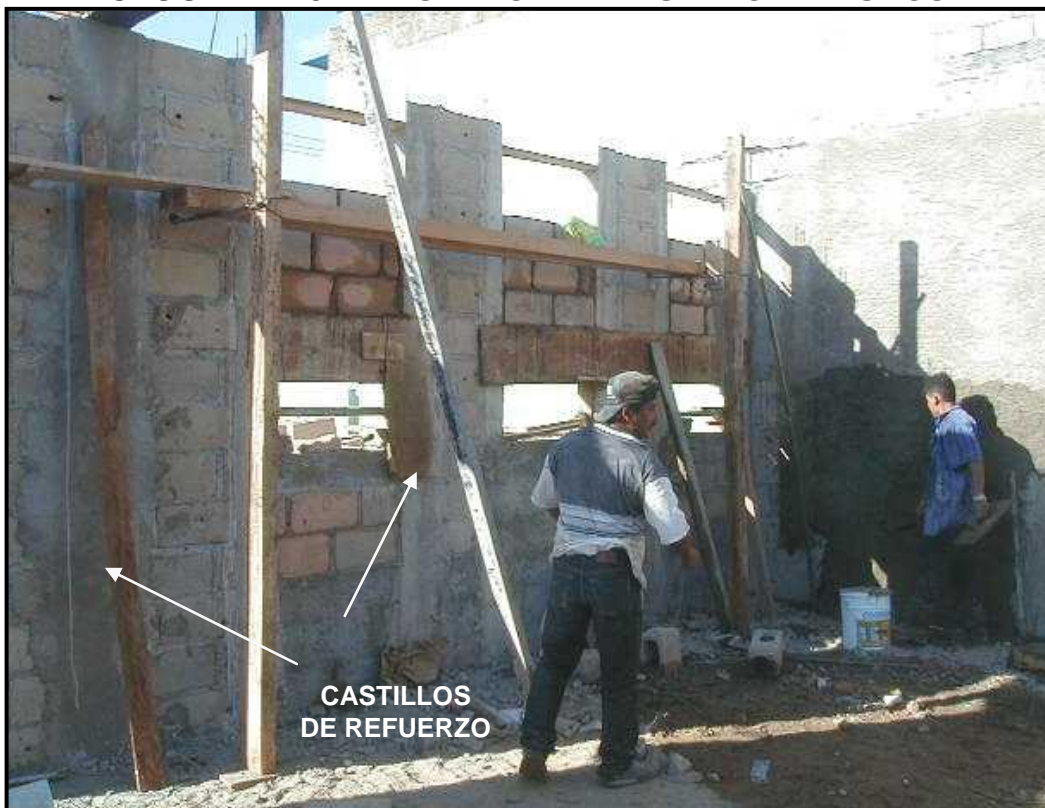
FOTOGRAFÍA 32 "CASTILLO DE REFUERZO EN MUROS"
