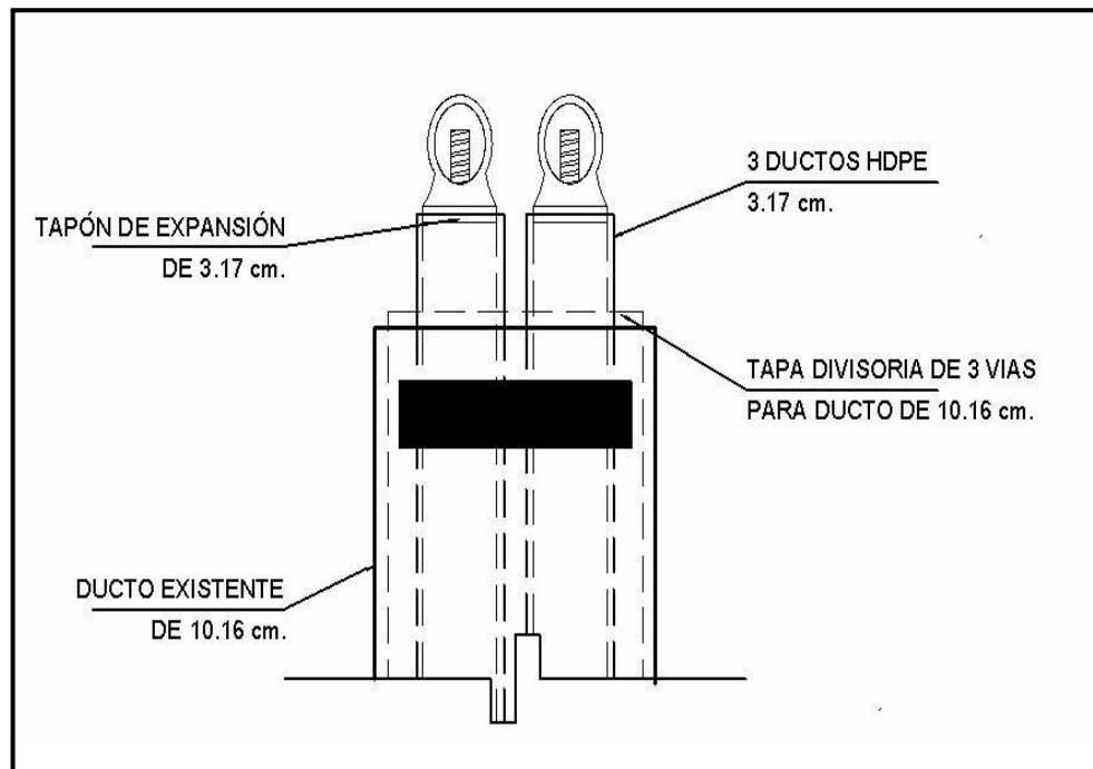
FIGURA 33 “CORTE VERTICAL DE TUBERÍA DE PVC EXISTENTE”
