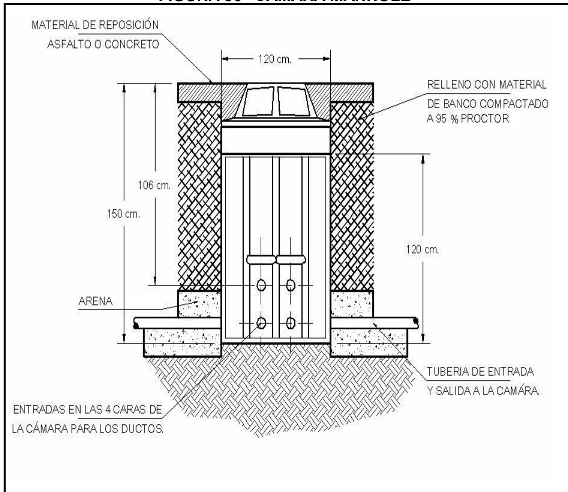
FIGURA 36 “CÁMARA MANHOLE”
