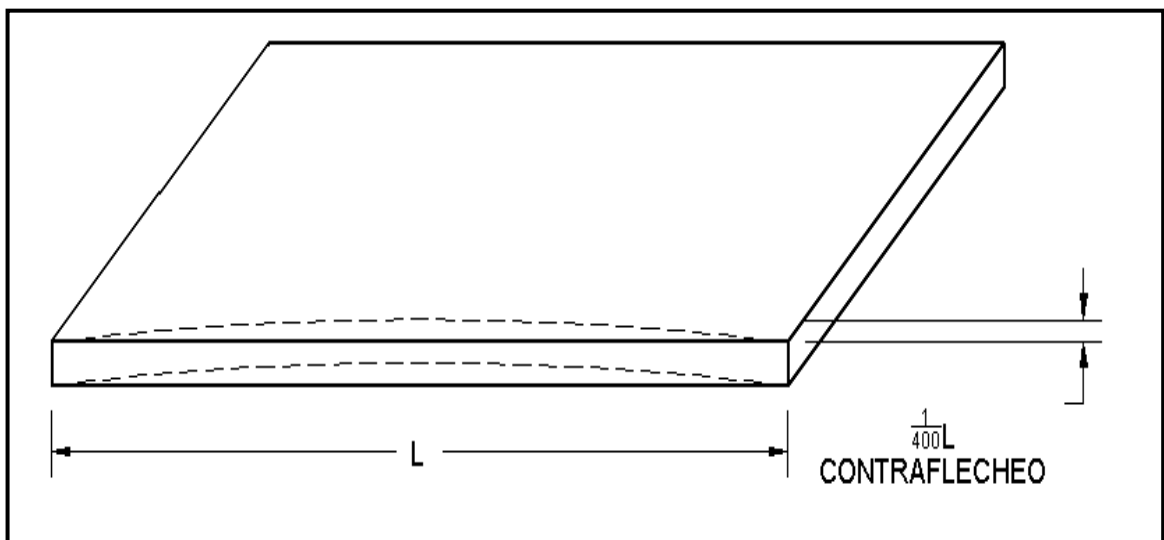
FIGURA 49 “CONTRAFLECHA PERMISIBLE”
