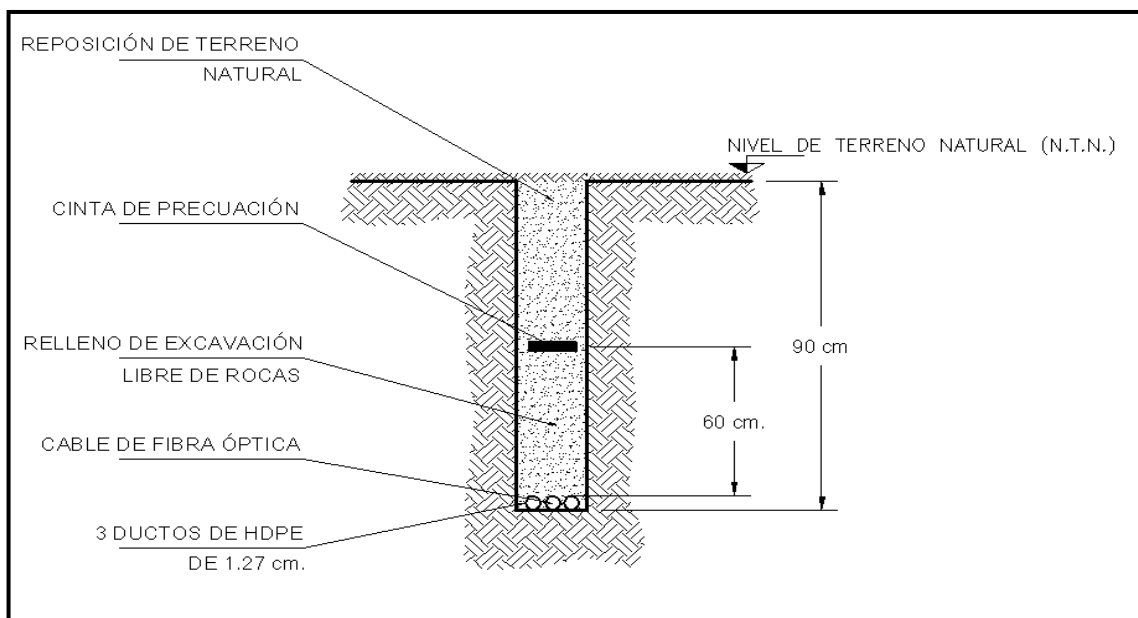
FIGURA 35 “CONSTRUCCIÓN DE ZANJA EN SUELOS TIPO B Y C”
