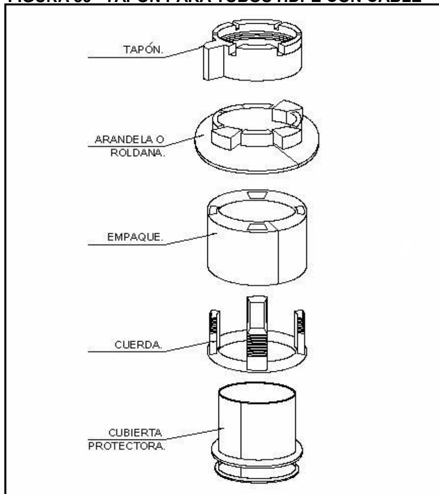
FIGURA 39 “TAPÓN PARA TUBOS HDPE CON CABLE”
