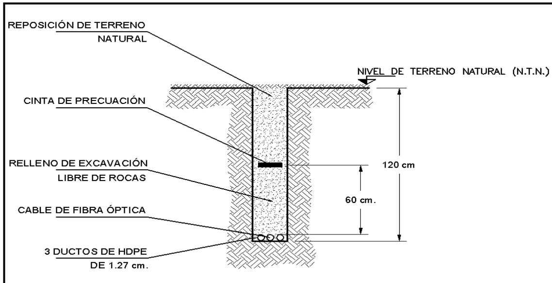
FIGURA 35 “CONSTRUCCIÓN DE ZANJA EN SUELOS TIPO B Y C”
