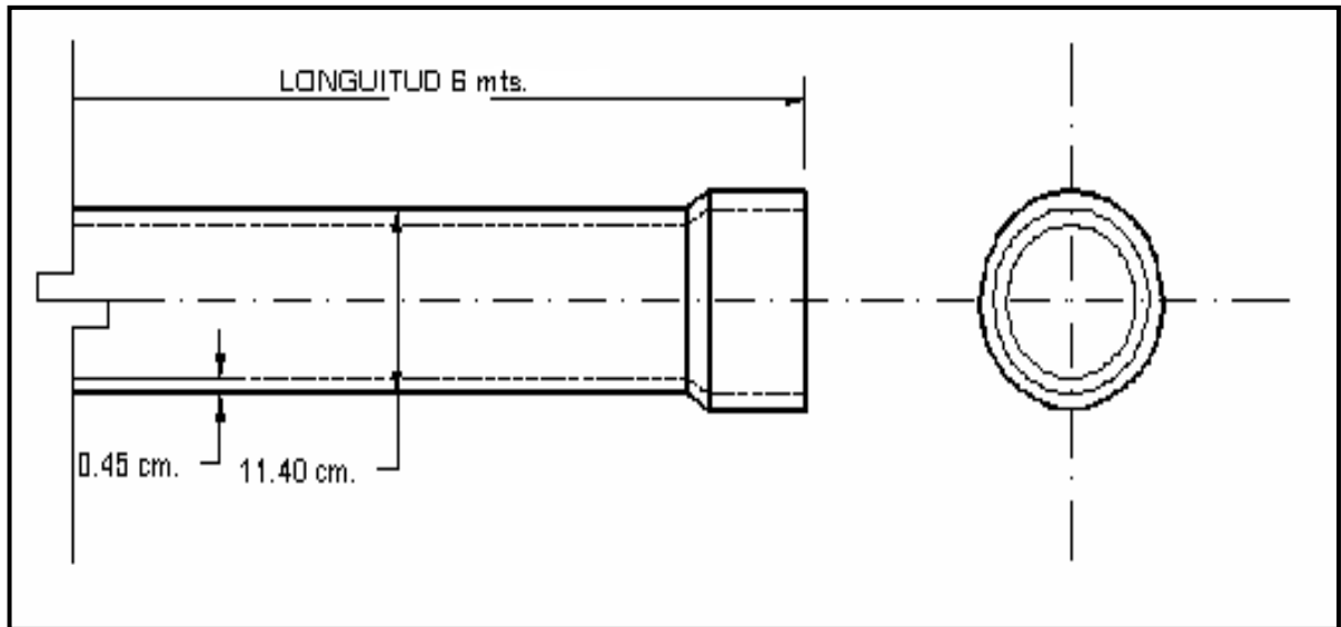
FIGURA 47“CORTE DE TUBO DE PVC”
