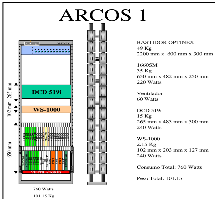
FIGURA 54 “BASTIDOR TIPO”
