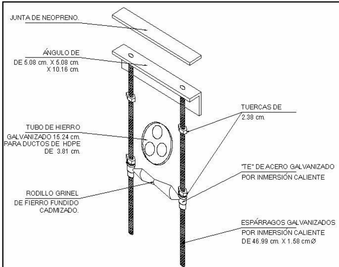
FIGURA 40 “PARTES DE HERRAJE DE COLUMPIO
