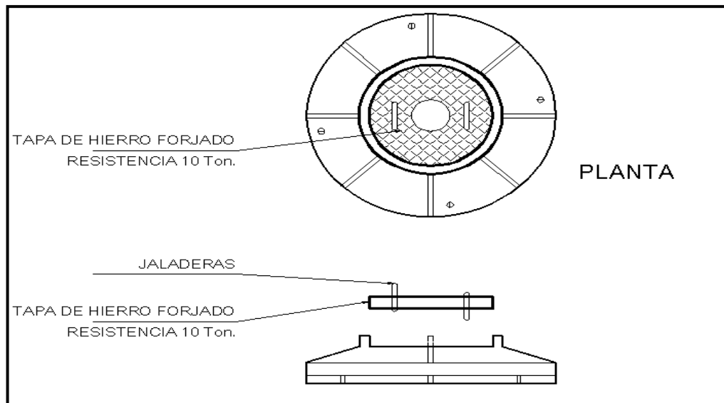
FIGURA 43 “TAPA DE HIERRO FUNDIDO”
