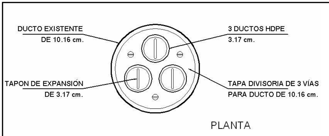
FIGURA 41 “TAPÓN PARA LA TRIPLICACIÓN DE TUBOS”
