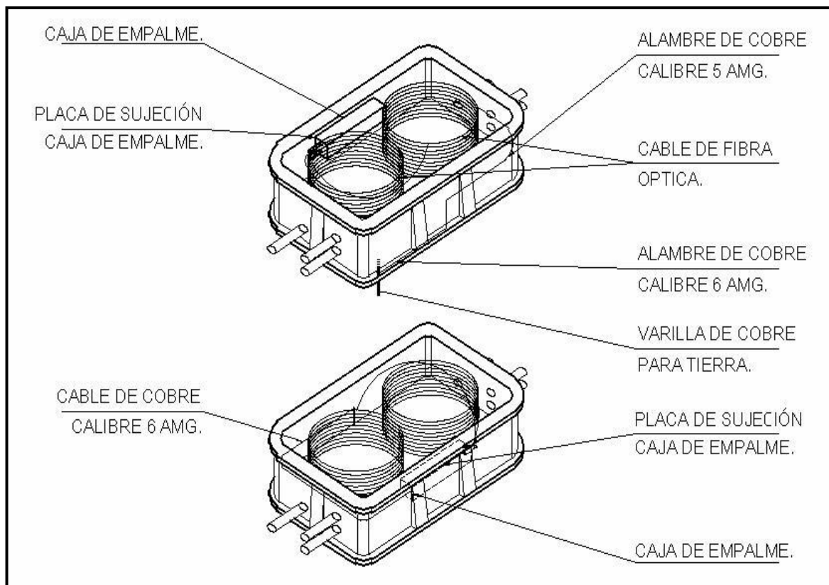
FIGURA 46 “SISTEMA DE TIERRAS EN CÁMARAS”
