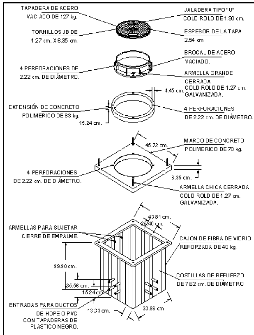
FIGURA 42 "CÁMARA MANHOLE"
