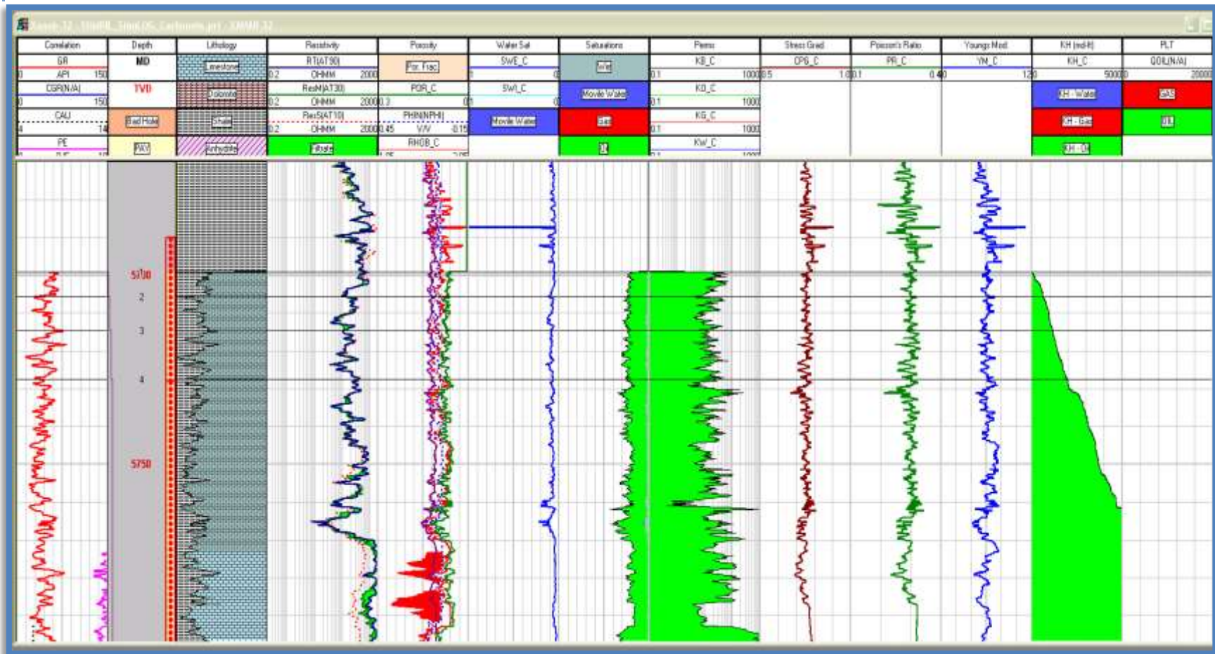
Figura 5.15. Interpretación (valores promedios): Caliza limpia, porosidad 7%, Shc= 93%, K=21.1 mD. Productor de aceite.
