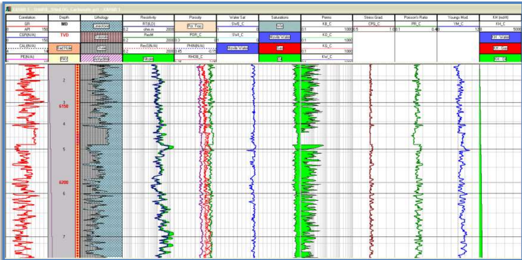
Figura 5.3. Interpretación (valores promedios): Caliza arcillosa, porosidad 4%, Shc= 89%, K=1.1 mD. No productor.
