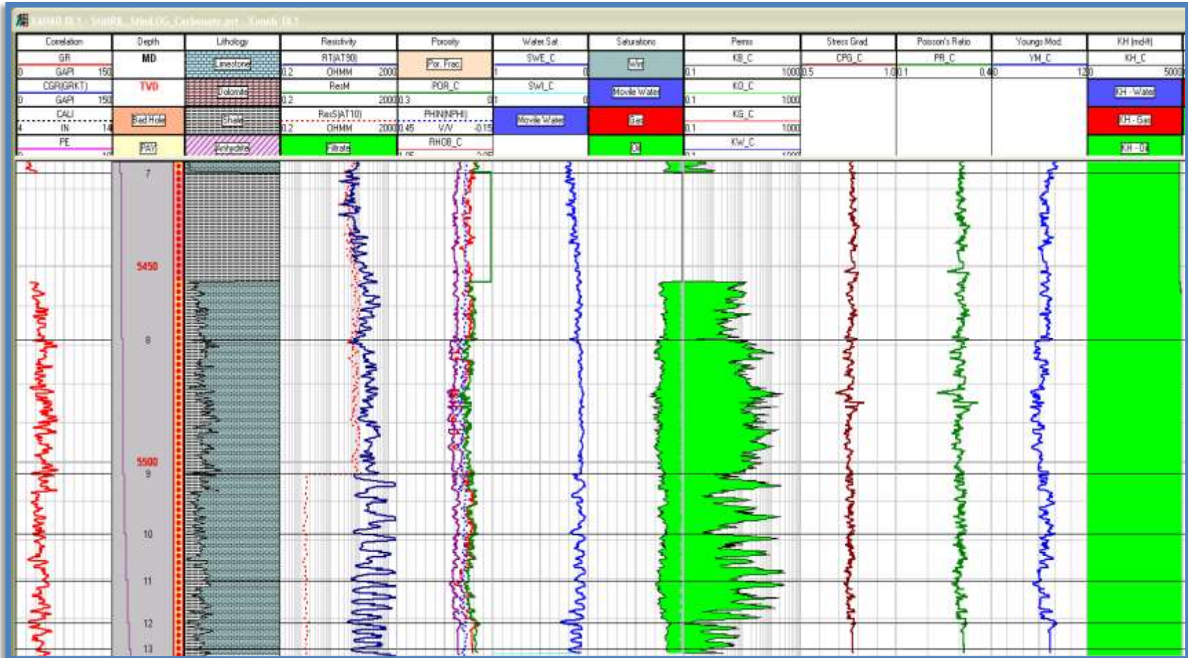
Figura 5.17. Interpretación (valores promedios): Caliza limpia, porosidad 7%, Shc= 88%, K=23.7 mD. Productor de aceite.
