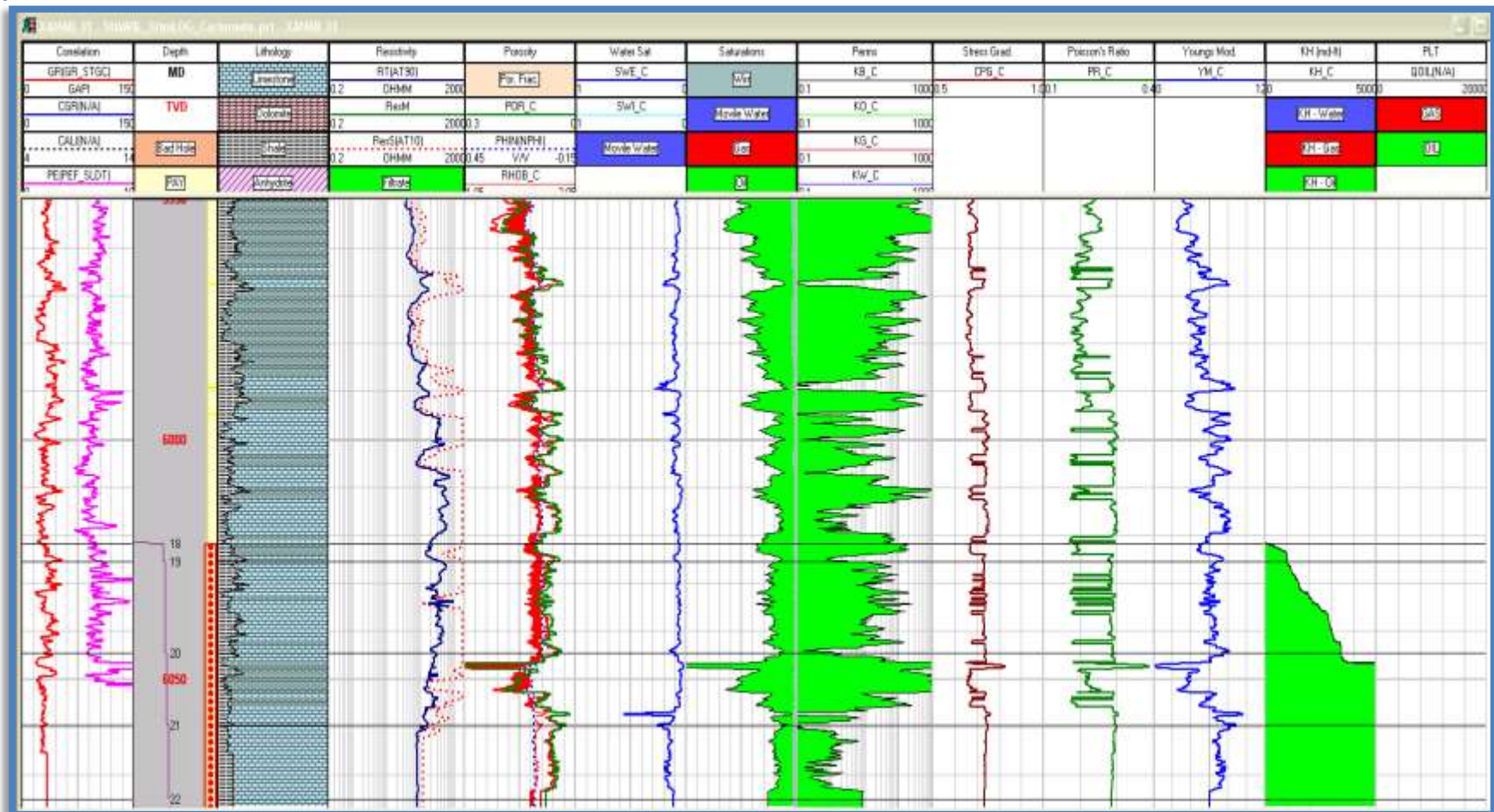
Figura 5.14. Interpretación (valores promedio): Caliza limpia, porosidad 8%, Shc= 92%, K=355.2 mD. Productor de aceite.
