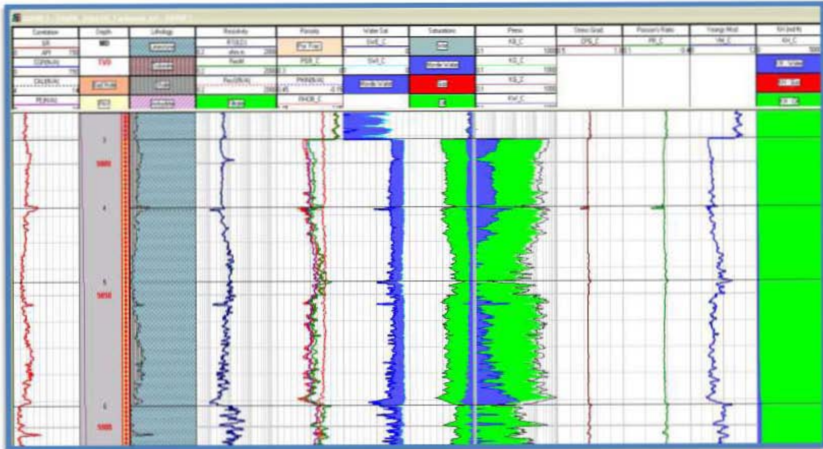
Figura 5.1 Interpretación (valores promedios): Caliza limpia, porosidad 11%, Shc= 74%, K=113.7 mD. Productor de aceite.
