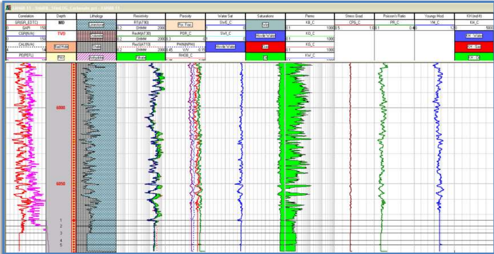
Figura 5.12. Interpretación (valores promedios): Caliza arcillosa, porosidad 4%, Shc= 90%, K=2.188mD. No productor .
