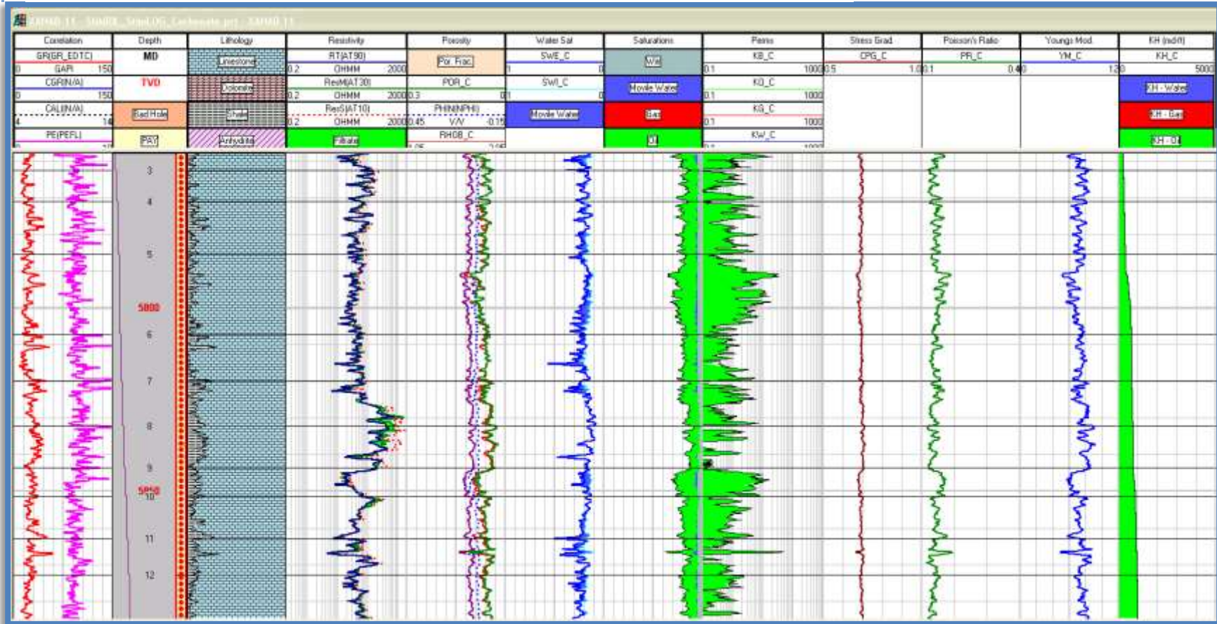
Figura 5.10. Interpretación (valores promedios): Caliza muy limpia, porosidad 6%, Shc= 81%, K=26.23 mD. Productor de aceite.
