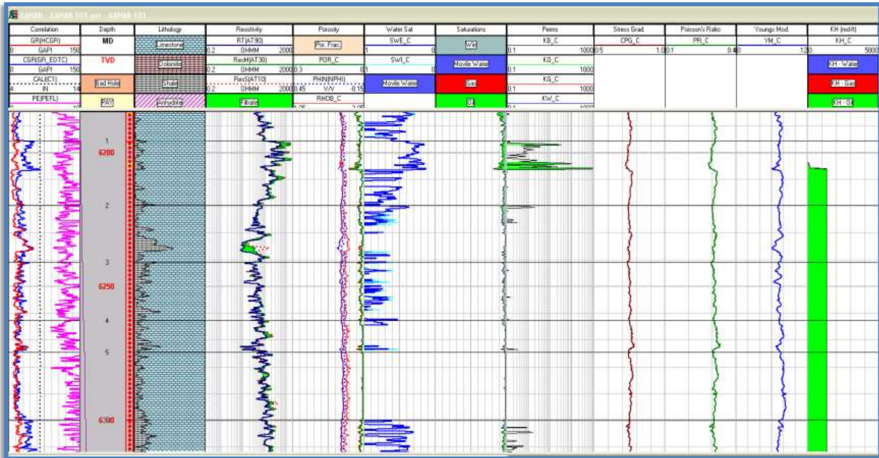
Figura 5.7. Interpretación (valores promedios): Caliza limpia, porosidad 5%, Shc= 83%, K=0.105 mD. Poco volumen de aceite.
