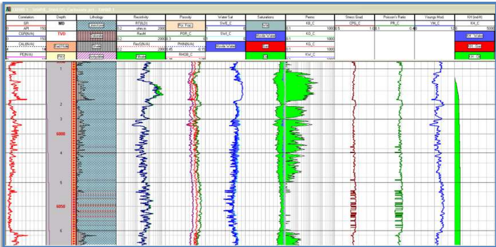
Figura 5.2 Interpretación (valores promedios): Caliza limpia, porosidad 6%, Shc= 79%, K=6.8 mD. Productor de aceite.
