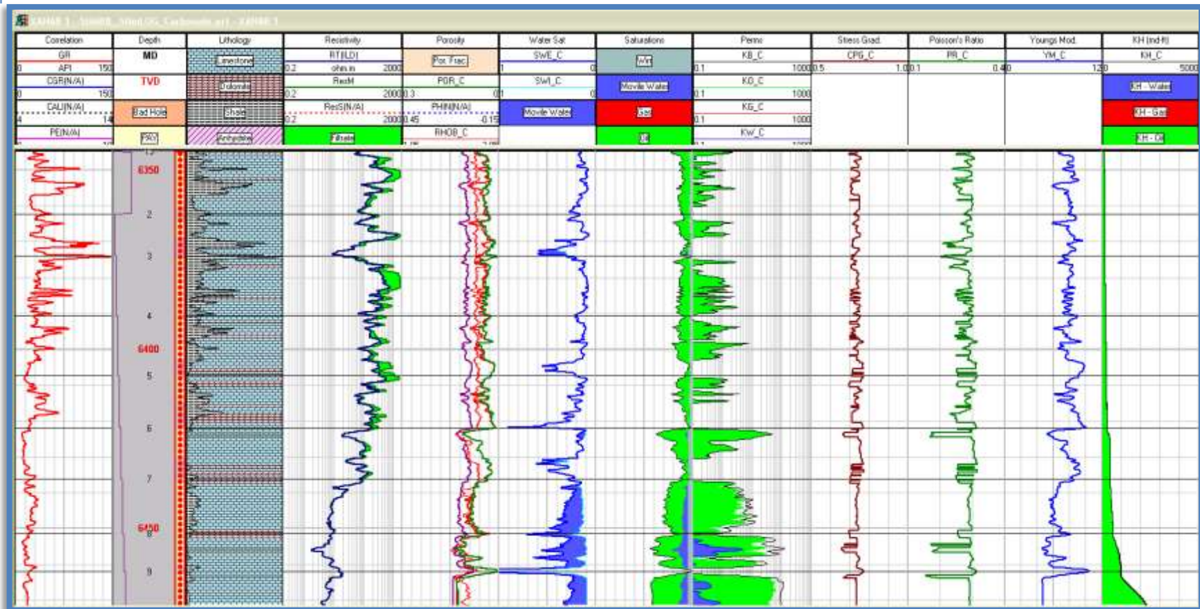
Figura 5.4. Interpretación (valores promedios): Caliza limpia y arcillosa, porosidad 6%, Shc= 81%, K=8.9 mD. Productor de aceite
