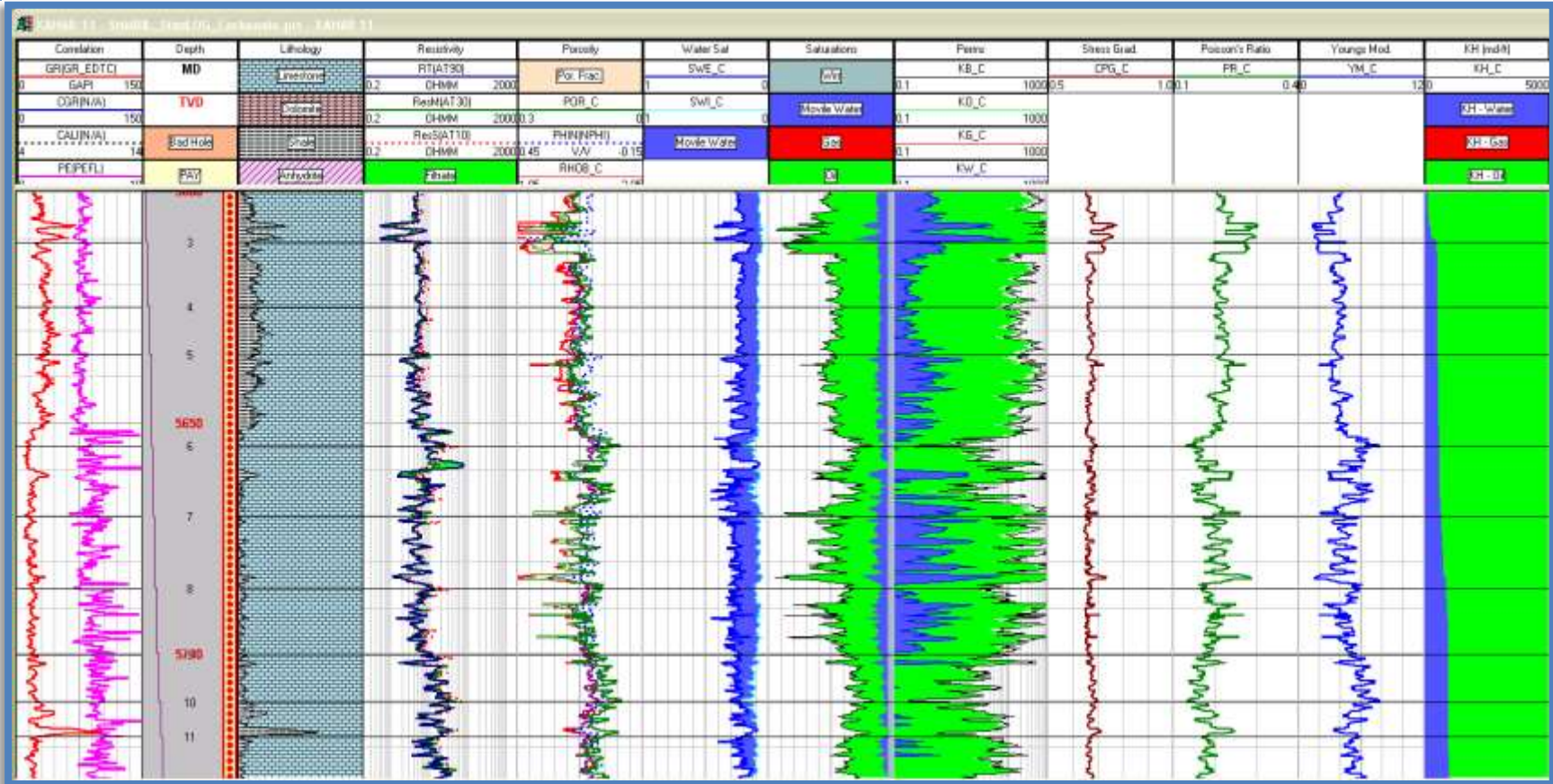
Figura 5.9. Interpretación (valores promedios): Caliza limpia, porosidad 14%, Shc= 77%, K=317.2 mD. Productor de aceite.
