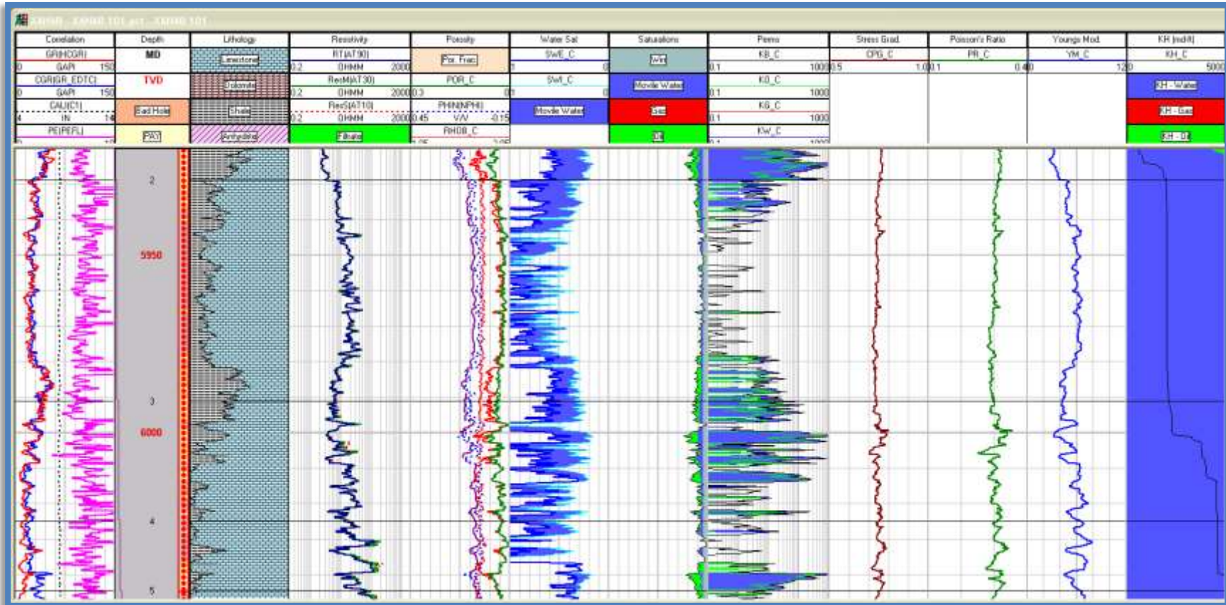
Figura 5.5. Interpretación (valores promedios): Caliza arcillosa y limpia, porosidad 5%, Shc= 44%, K=29.35 mD. Mayor permeabilidad al agua
