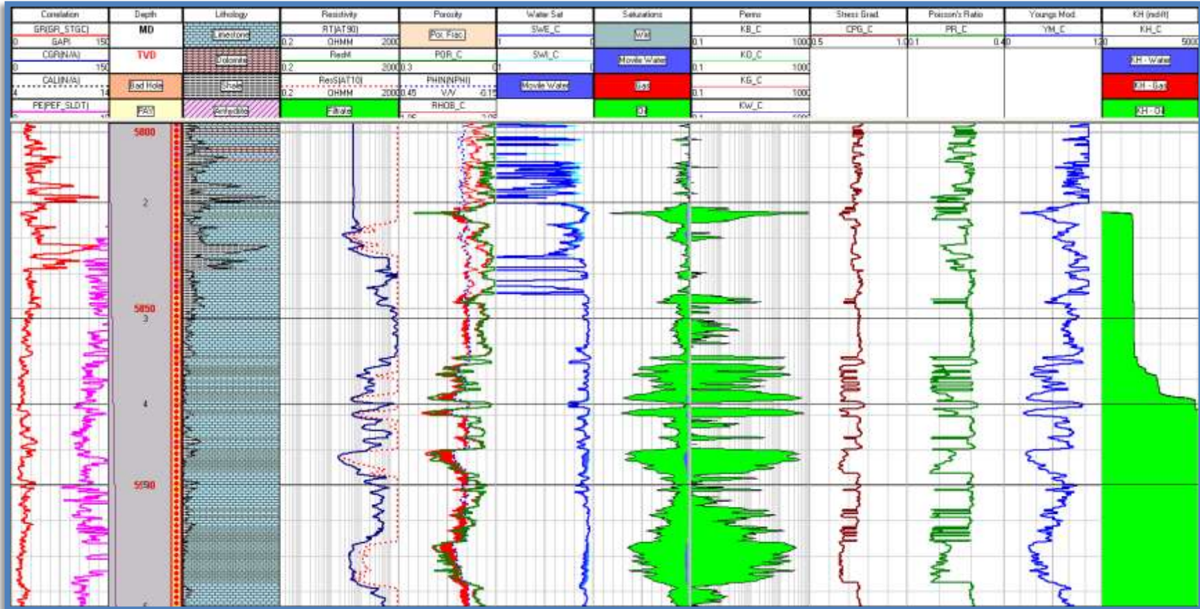
Figura 5.13. Interpretación (valores promedios): Caliza limpia y arcillosa, porosidad 10%, Shc= 92%, K=47.5 mD. No productor.
