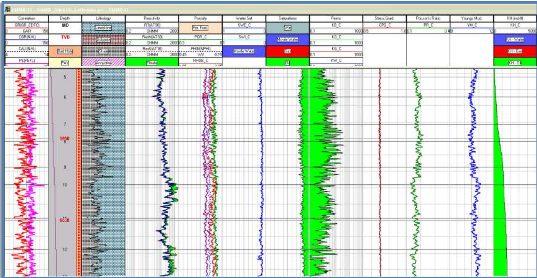
Figura 5.11. Interpretación (valores promedios): Caliza arcillosa, porosidad 5%, Shc= 90%, K=10.7 mD. Productor de aceite.
