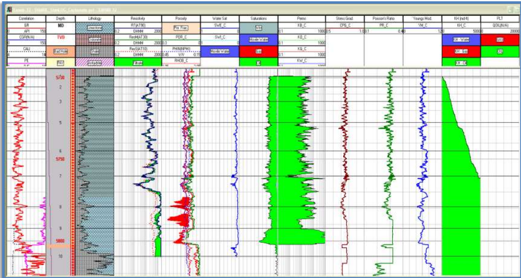
Figura 5.16. Interpretación (valores promedios): Caliza limpia Y arcillosa, porosidad 7%, Shc= 95%, K=333.8 mD. Productor de aceite
