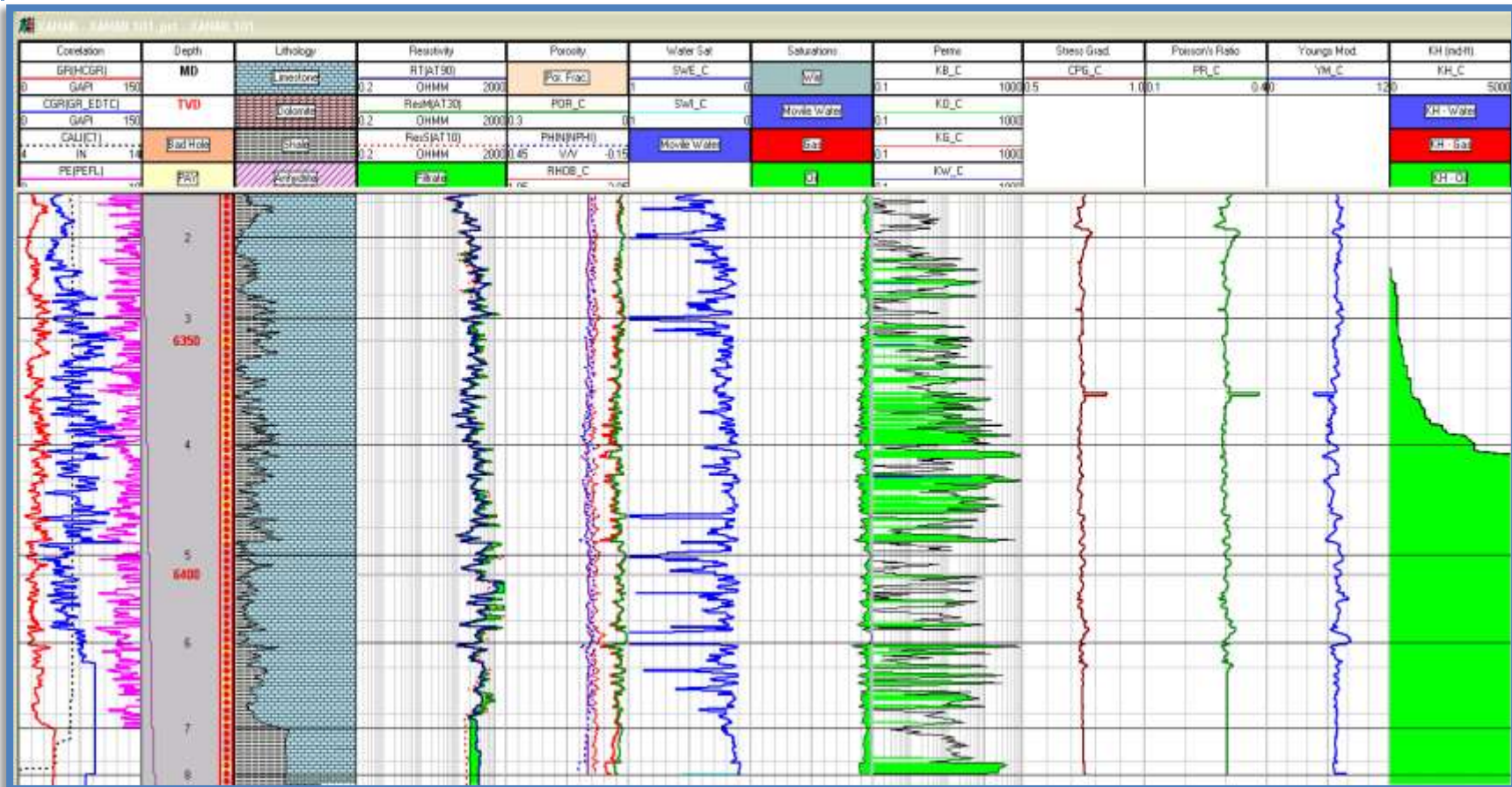
Figura 5.8. Interpretación (valores promedios): Caliza limpia, porosidad 4%, Shc= 87%, K=162.5 mD. No productor.
