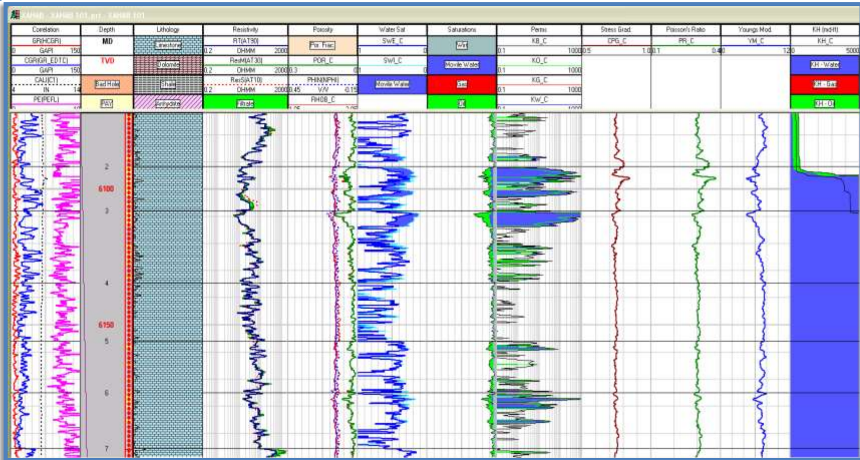
Figura 5.6. Interpretación (valores promedios): Caliza muy limpia, porosidad 5%, Shc= 58%, K=160.88 mD. Mayor permeabilidad al agua
