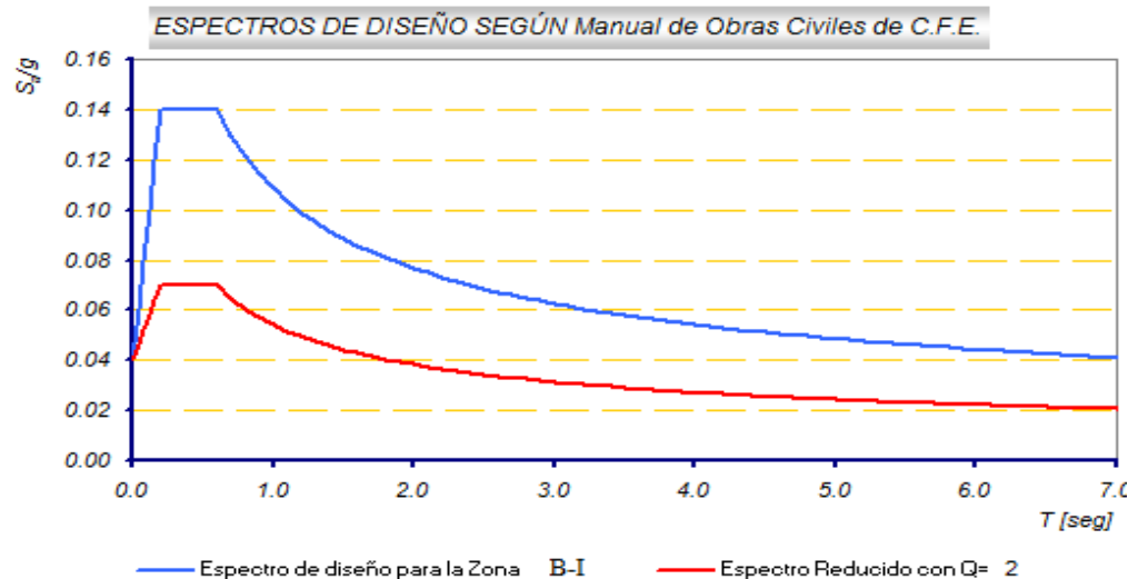
Figura #3.2 Definición del espectro sísmico.
