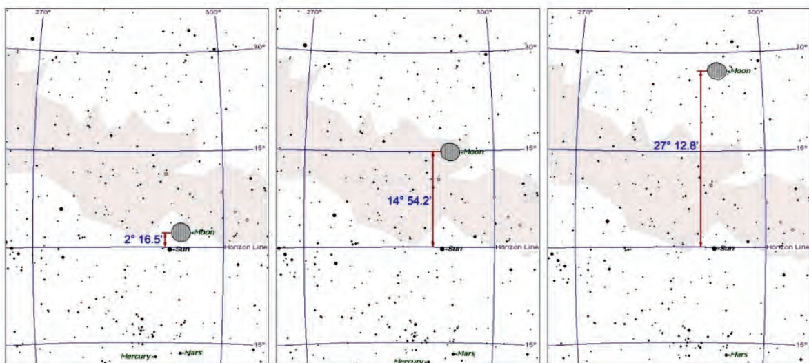
Figura 1.6: Primera visibilidad del creciente lunar para la Estela 26 de Piedras Negras del 22 al 24 de Mayo del 608 (gráficas realizadas con Starry Night Pro , 2000).
