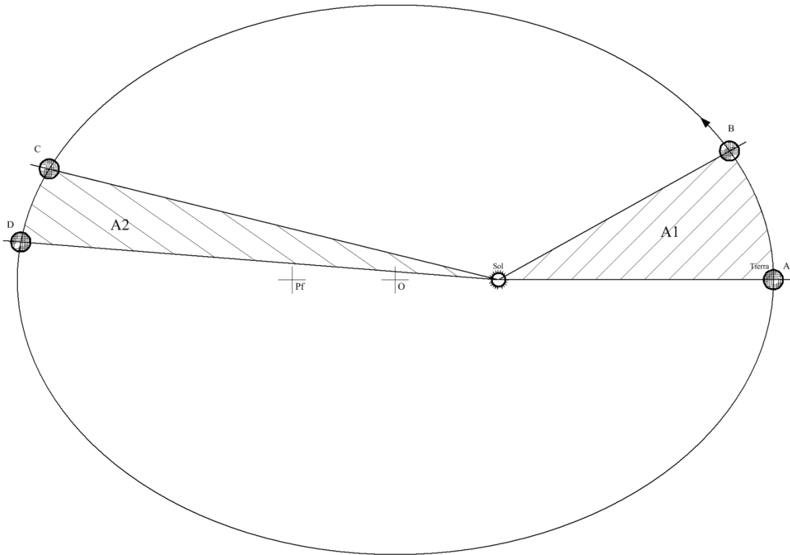
Figura 1.2 Segunda Ley de Kepler.
