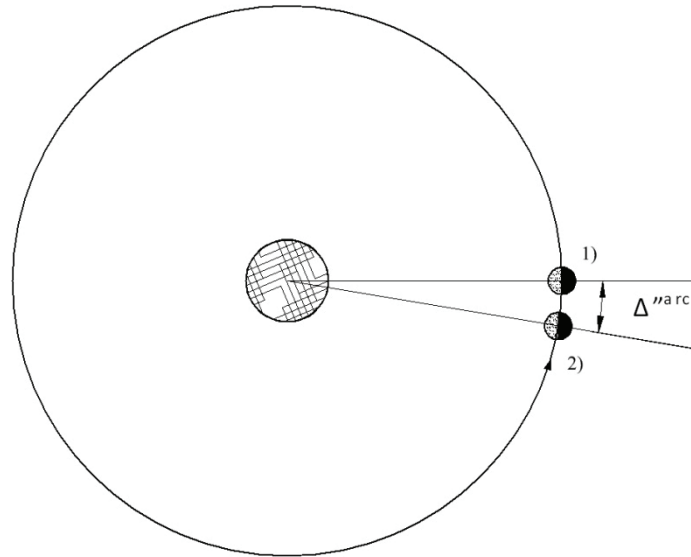
Figura 1.7: Esquema de desaceleración de la Luna.
