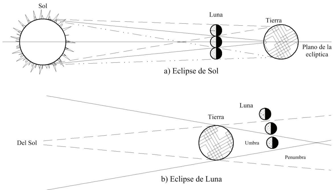
Figura 1.4: Proyecciones de eclipses; a) eclipse de Sol, b) eclipse de Luna.
