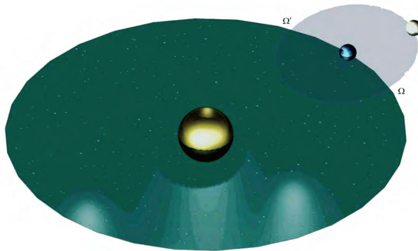
Figura I.1: Plano de la eclíptica, órbita terrestre e inclinación de la órbita lunar.
