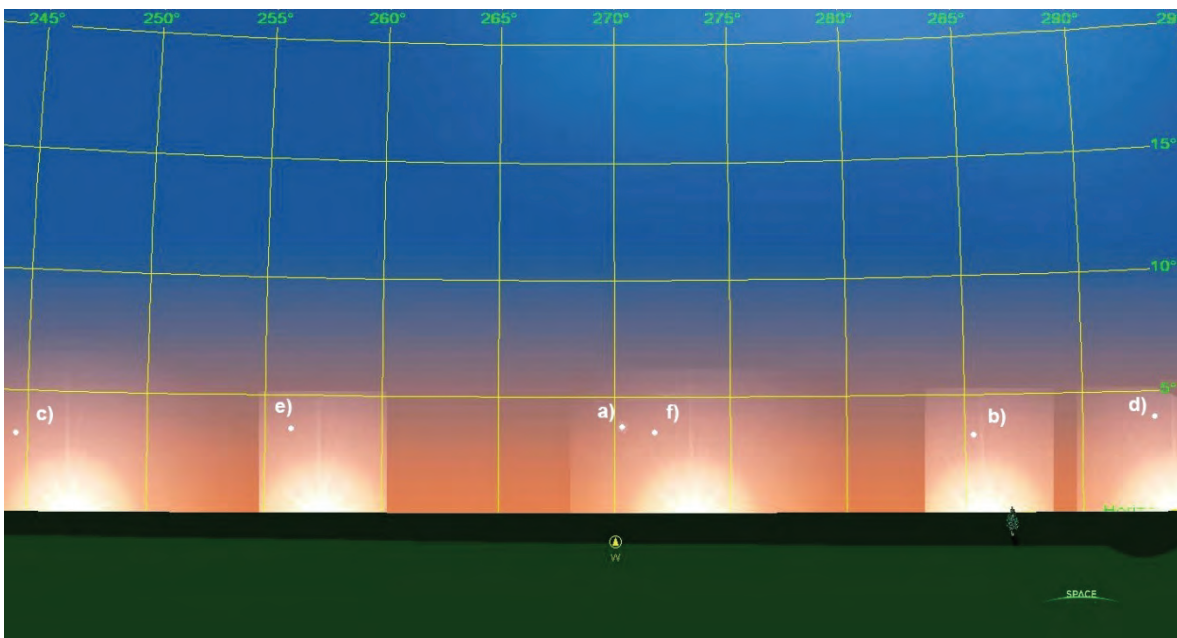
Figura 1.11: “Gran Ciclo” de Venus; a) 17/Sep/692; b) 30/Abr/694; c) 2/Dic/695; d) 8/Jul/697; e) 16/Feb/699; f) 15/Sep/700 (gráficas realizadas con Starry Night Pro , 2000).
