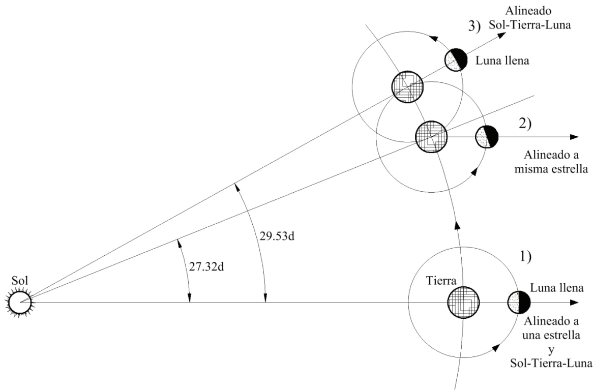
Figura 1.1: Revolución sidérea y sinódica de la Luna.
