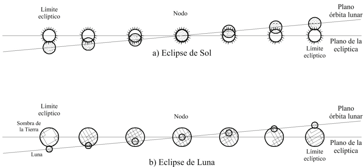
Figura 1.5: Límites eclípticos; a) eclipses de Sol, b) eclipses de Luna.
