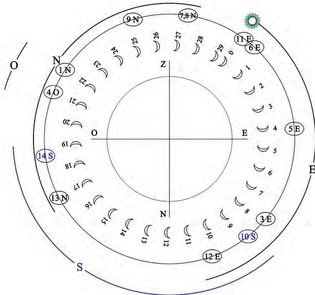
Figura 9.2: Gráfica de las posiciones del K'awiil en el ciclo de 819 días.
