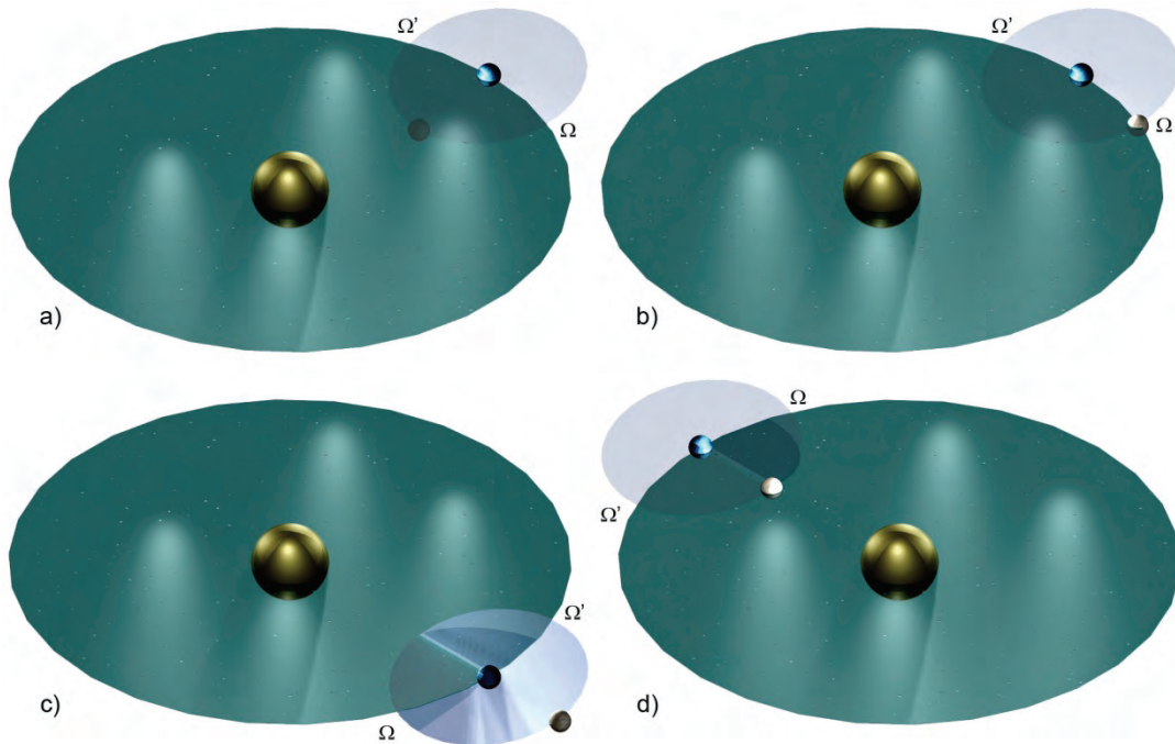
Figura 1.3: Plano de la eclíptica, órbita terrestre e inclinación de la órbita lunar, y la configuración de eclipses.
