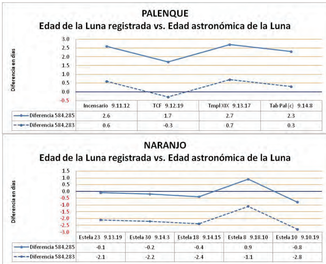
Gráfica 9.1: Gráficas de la diferencia entre la edad astronómica de la Luna menos la edad registrada en los monumentos mayas. Las diferencias se calculan con respecto de la edad astronómica según las correlaciones GMT y GMT+2.
