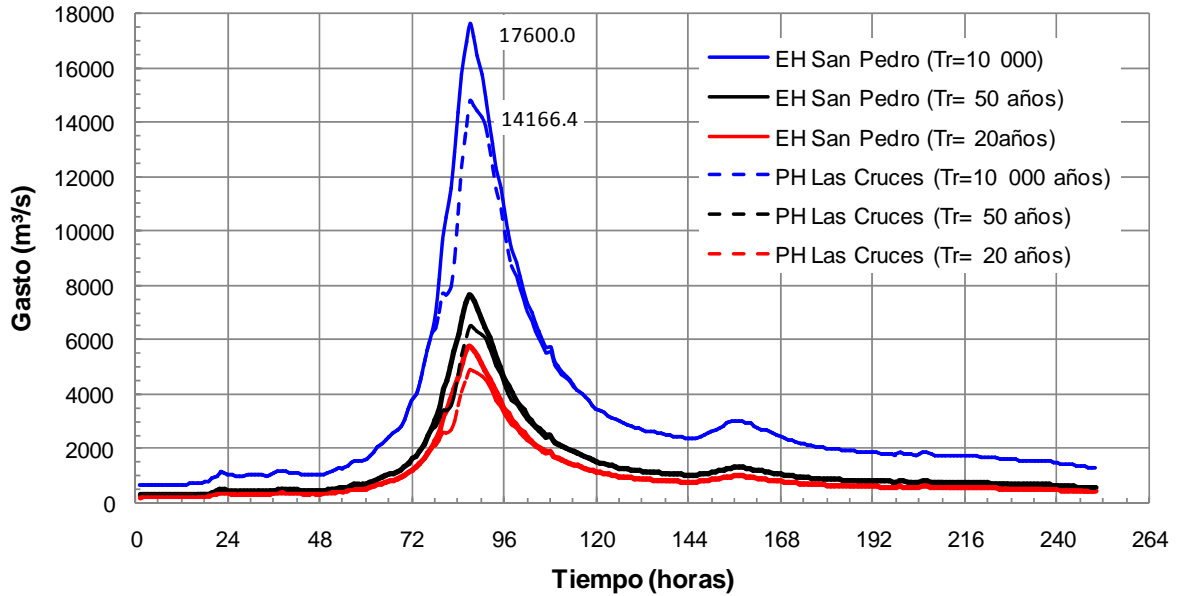
Figura 5-7 Avenidas de diseño para la EH San Pedro y el PH Las Cruces para diferentes periodos de retorno
