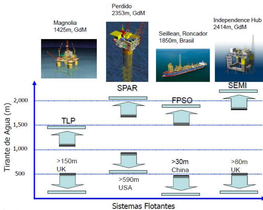
Figura 2.2 Equipos de perforación, utilizados en aguas profundas actualmente, a diversas profundidades y campos. 22
