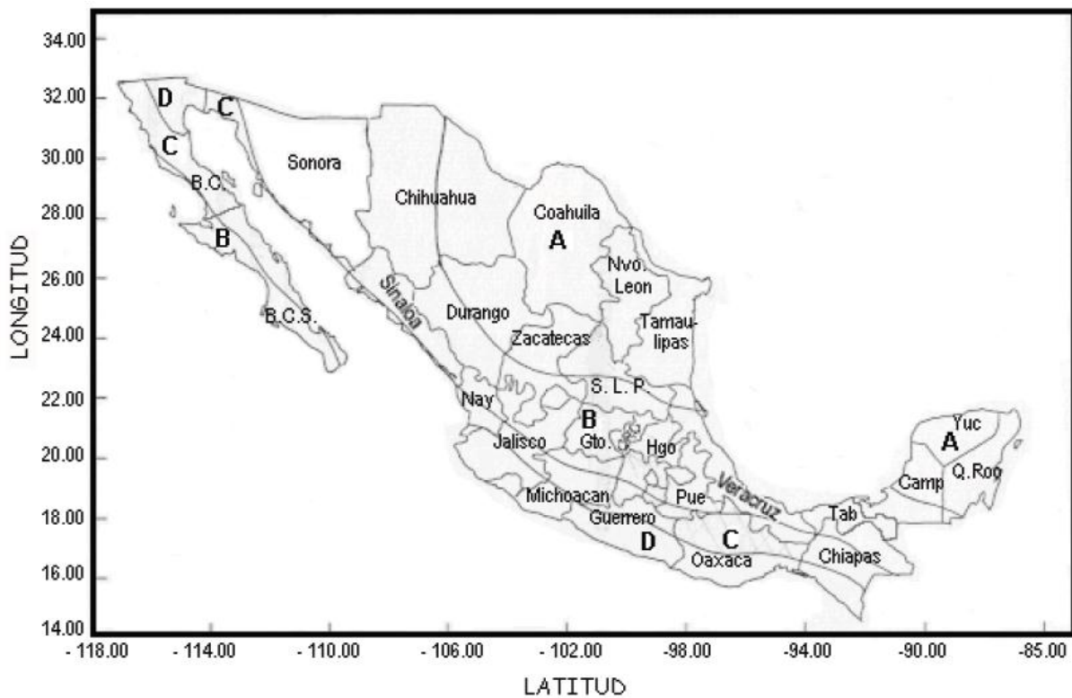
Fig. 4.3 Zonificación sísmica de la República Mexicana. Tomado del Manual de diseño de Obras Civiles (Diseño por Sismo) de Comisión Federal de Electricidad
