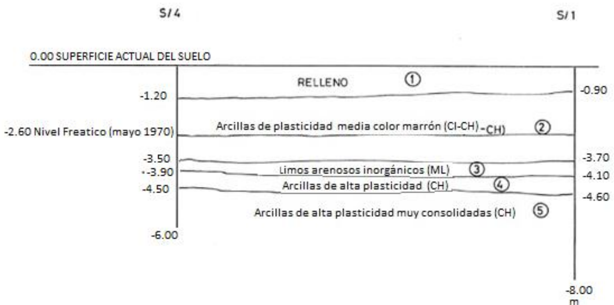
Fig. 6.15 Perfil Estratigráfico X-X'. Tomado de Ref.5 "SILOS"
