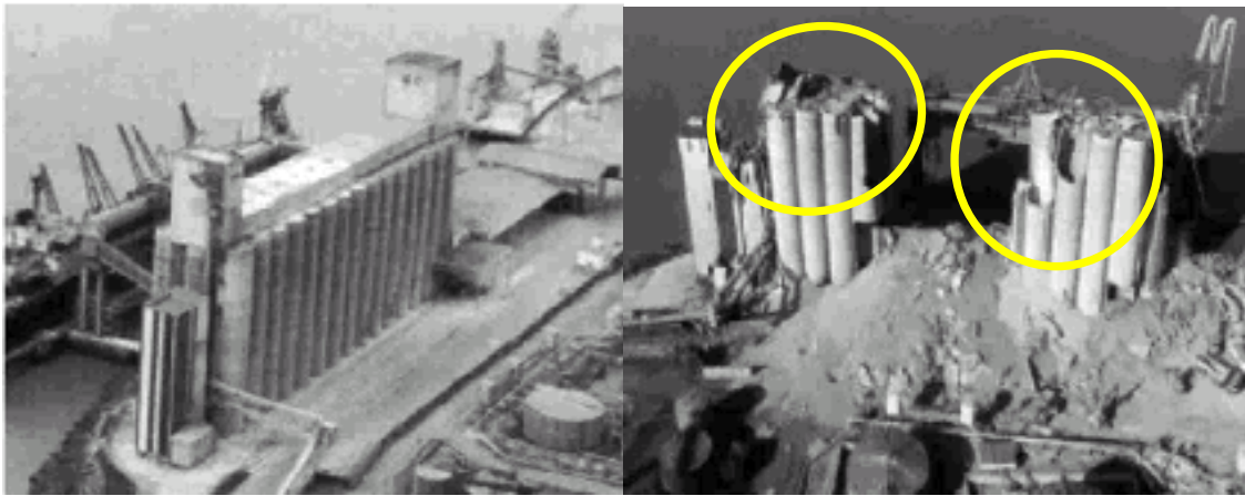
Fig. 3.5 Antes y después de explosión en un silo de concreto en Canadá. Tomado de Ref. 2 “Cause of damage and failures in silo structures”
