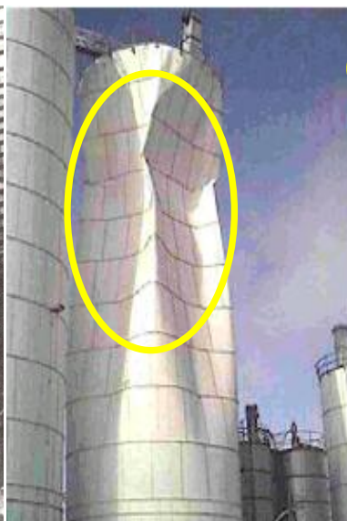
Fig. 3.2 Falla de silo metálico por problemas de flujo en carga y descarga. Tomado de Ref.2 “Causas de Daños y fallas en silos”
