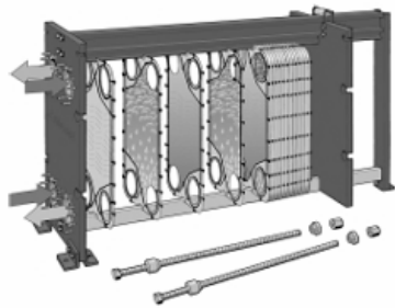
Intercambiador tipo "placas"
