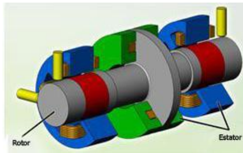
Figura 4.8 Cojinetes magnéticos. [18]
