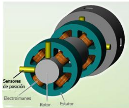
Figura 4.13 Sistema de control de los cojinetes magnéticos 2. [18]
