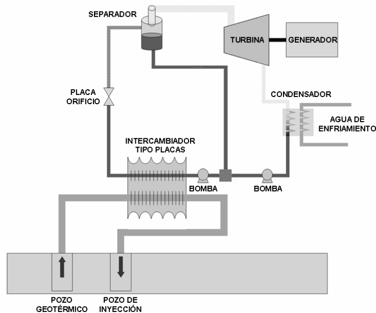
Figura 3.2 Planta de ciclo PWG. [13]
