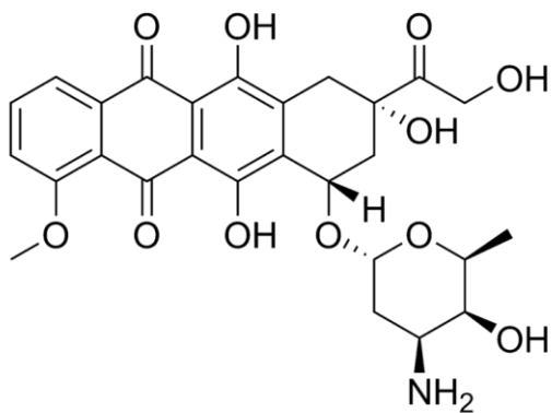
Doxorubicina 7 (natural)
