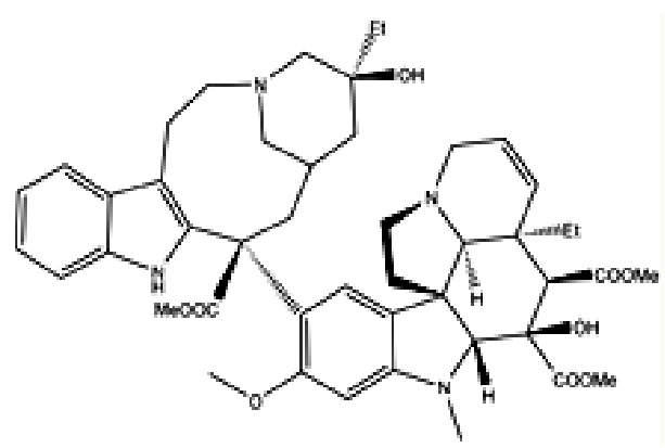
Vinblastina 3 (natural)
