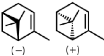
\alpha -Pineno 19
