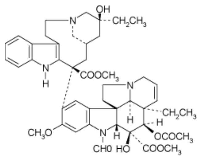
Vincristina 2 (natural)
