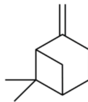
\beta -Pineno 20
