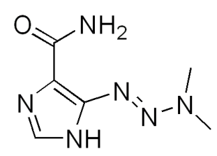
Dacarbazina 4 (sintético)
