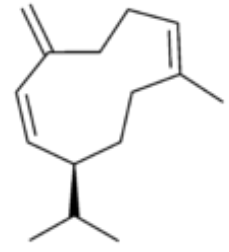
Germacreno D 35
