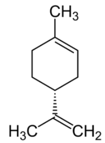
Limoneno 15
