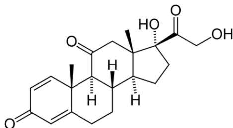
Prednisona 10 (sintético)
