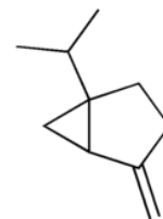
Sabineno 21
