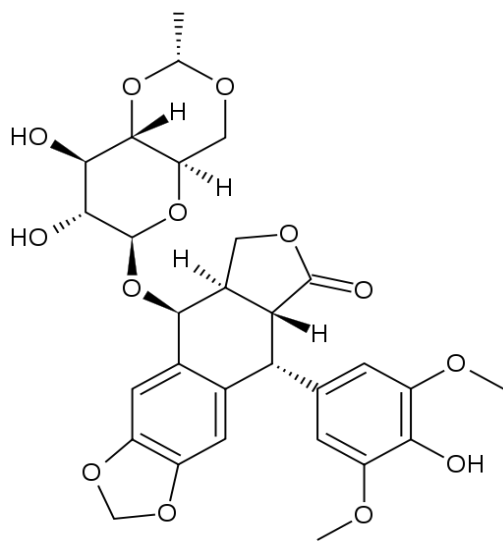
Etoposido 1 (semisintético)
