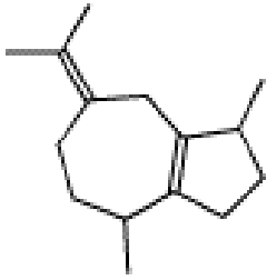
\beta -Guaieno 36
