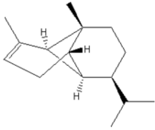
\alpha -Copaeno 33
