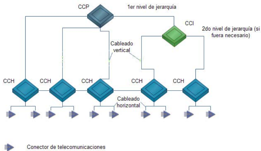
Figura 2.2 Conexiones cruzadas
