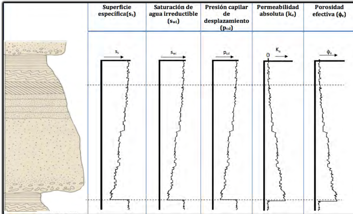
Figura 4.4 Propiedades petrofísicas en una secuencia turbidítica (Zaldívar, 2008).
