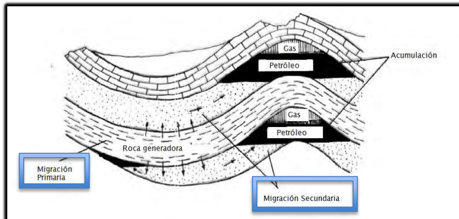
Figura 4.10 Tipos de migración (Martell, 2010).
