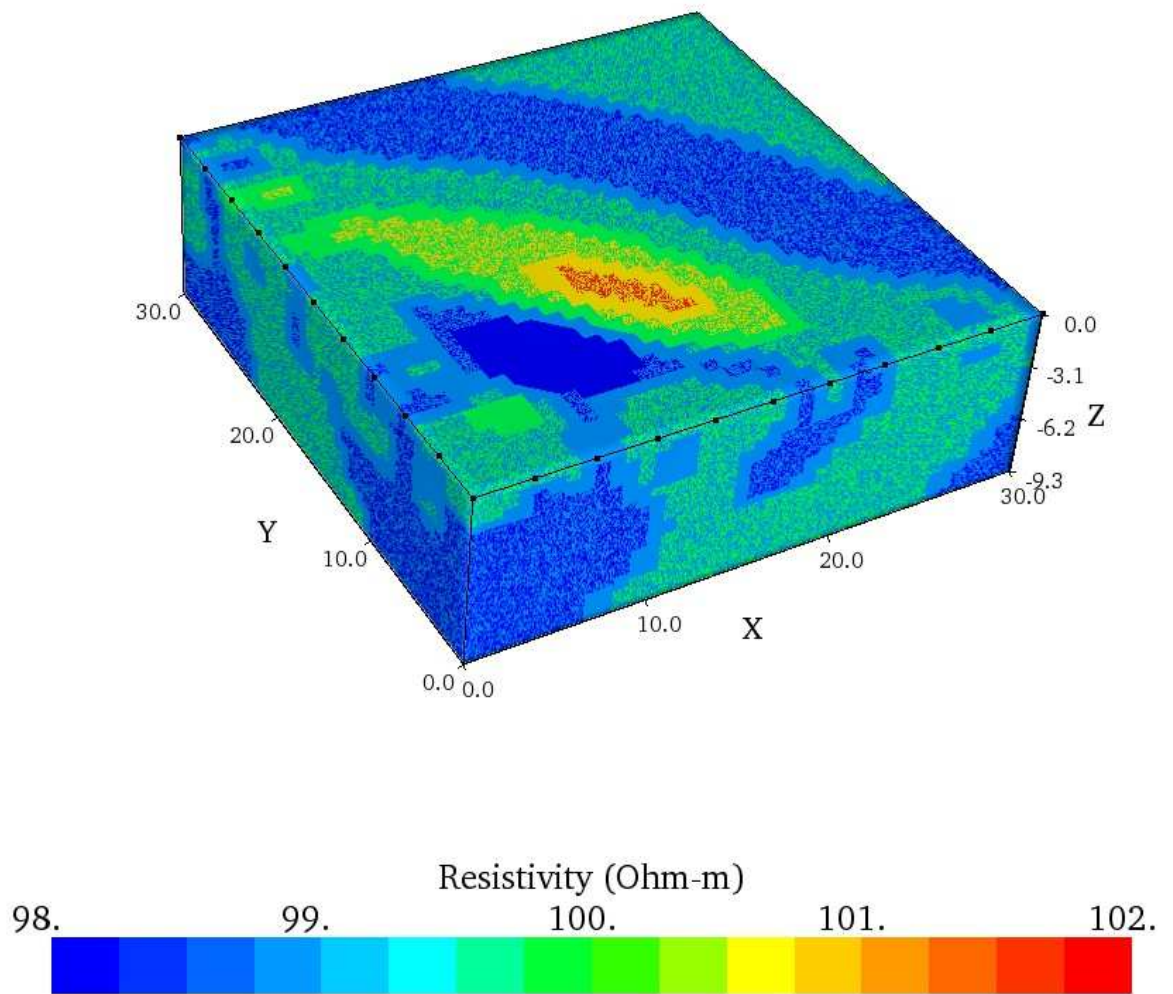
Figura3.09 Inversión de los datos con el Arreglo en “L” para Modelado sintético de un cuerpo de dimensiones (5, 5, 3) unidades de rejilla. Ubicación (15, 15, 3)
