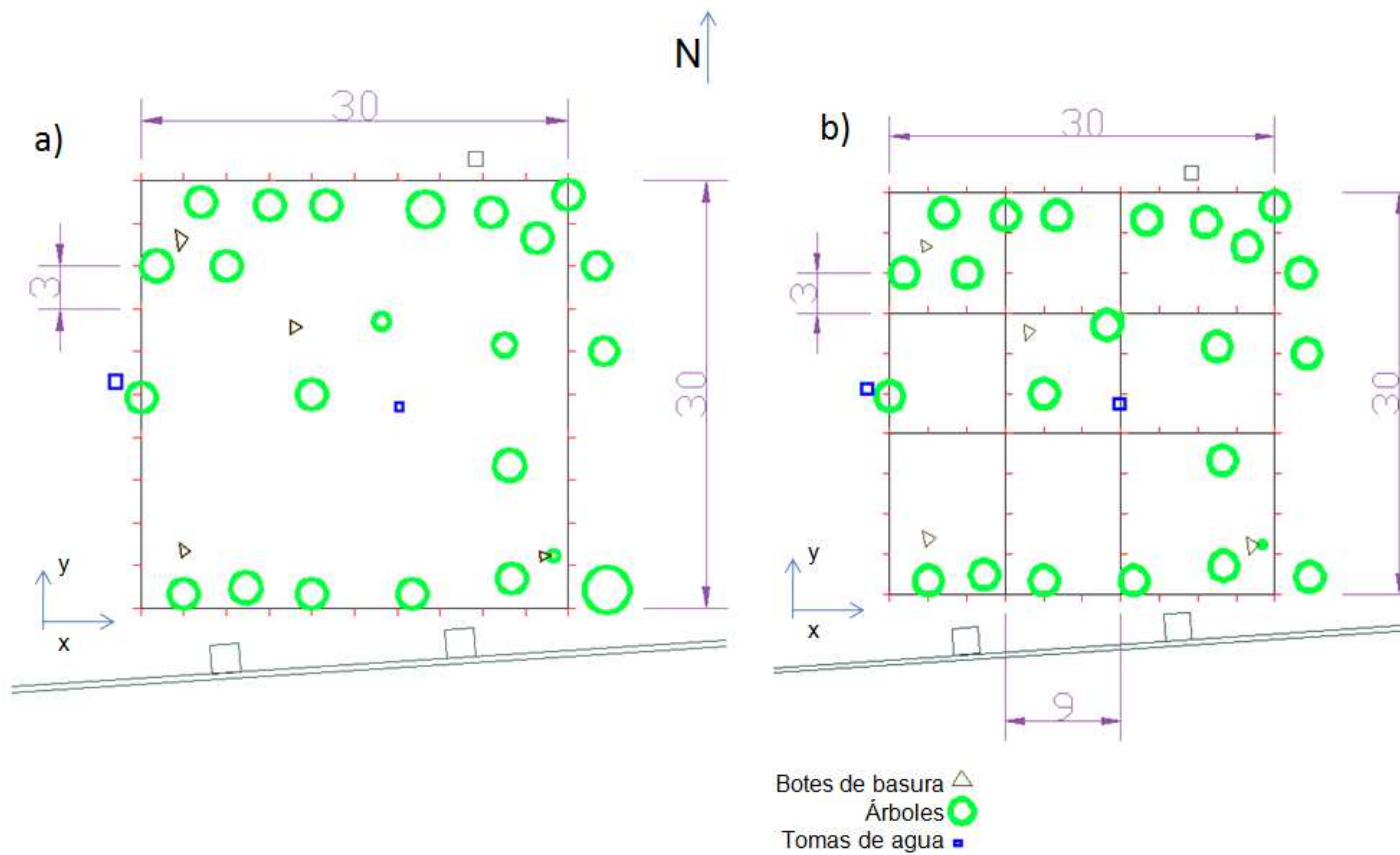
Figura 3.19 a) Croquis de ubicación de los electrodos para un cubo de 30x30 m con arreglo en “L.” b) Croquis de ubicación de los electrodos con líneas paralelas. En ambos croquis la separación electródica es de 3 m. Los círculos verdes representan los árboles, los puntos azules las tomas de agua y los puntos marrón los botes de basura. En la parte de abajo se representa con dos líneas grises una barda construida con basalto, tomado de la zona.
