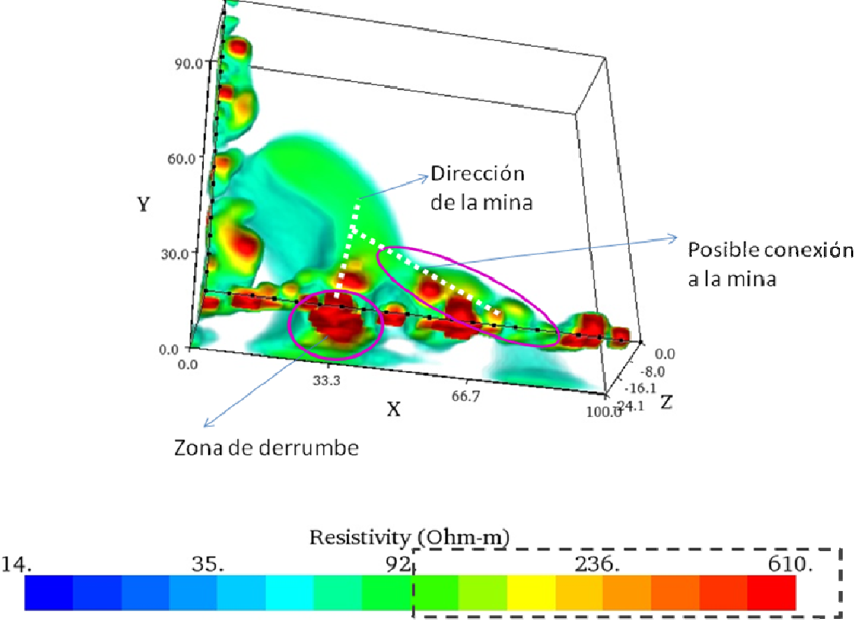
Figura 4.06 Vista con opacidad de los datos del arreglo en L. El recuadro marca las resistividades utilizadas.
