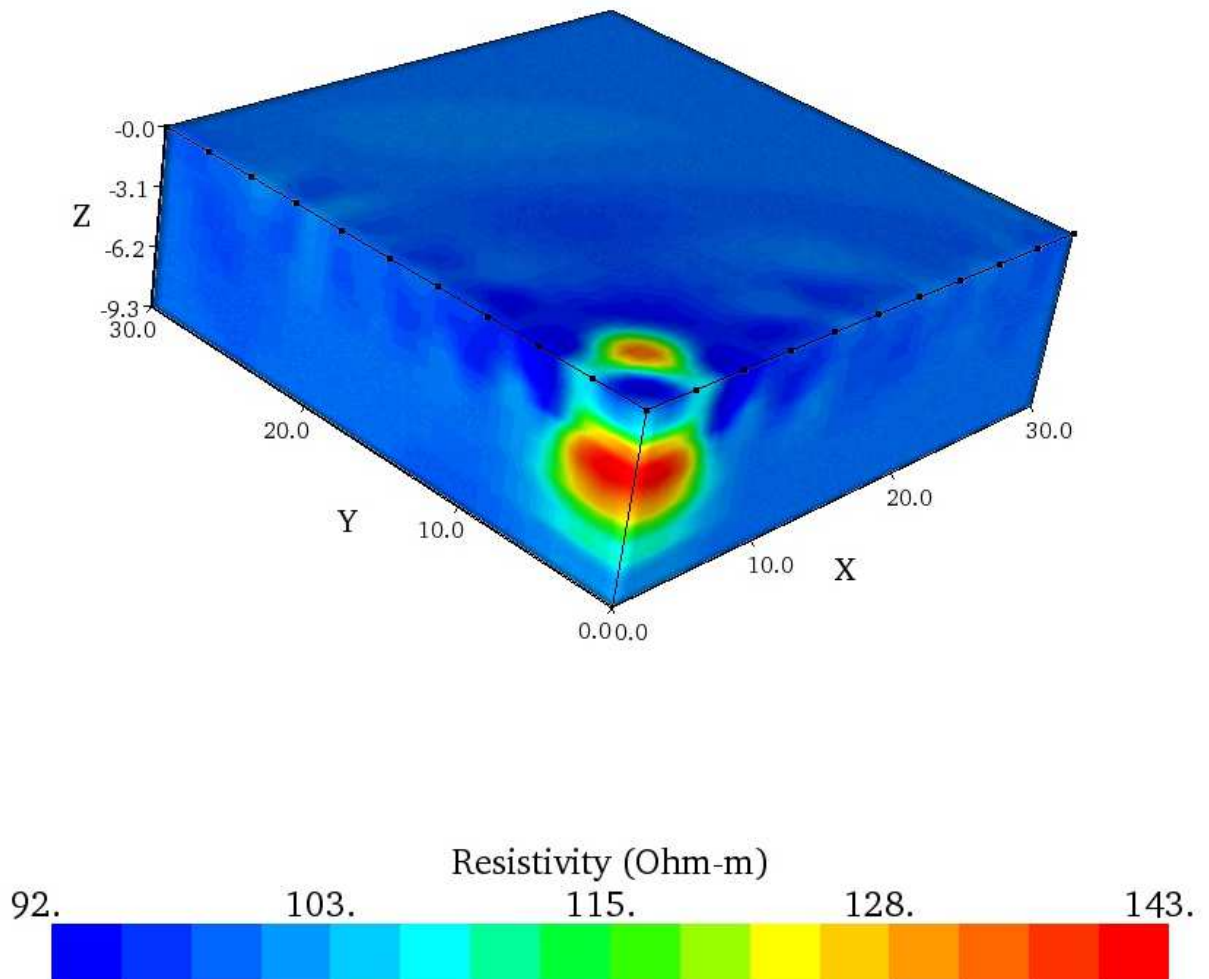
Figura 3.16 Inversión de los datos con el Arreglo “L” junto con el arreglo en “Esquina” para Modelado sintético de un cuerpo de dimensiones (5, 5, 3) unidades de rejilla. a) ubicación (1, 1, 3) unidades de rejilla.
