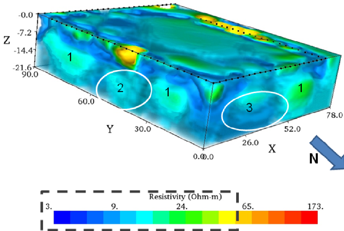
Figura 29. Cubo de resistividad en 3D de la catedral de Morelia, con opacidad, resistividades menores a 50 ohm-m en recuadro.
