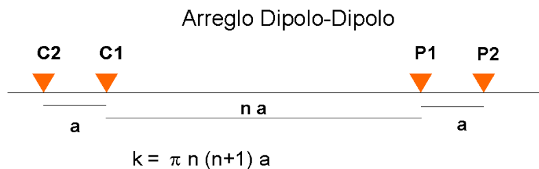
Figura 2.03 Representación del arreglo dipolo-dipolo Loke (1996-2010).
