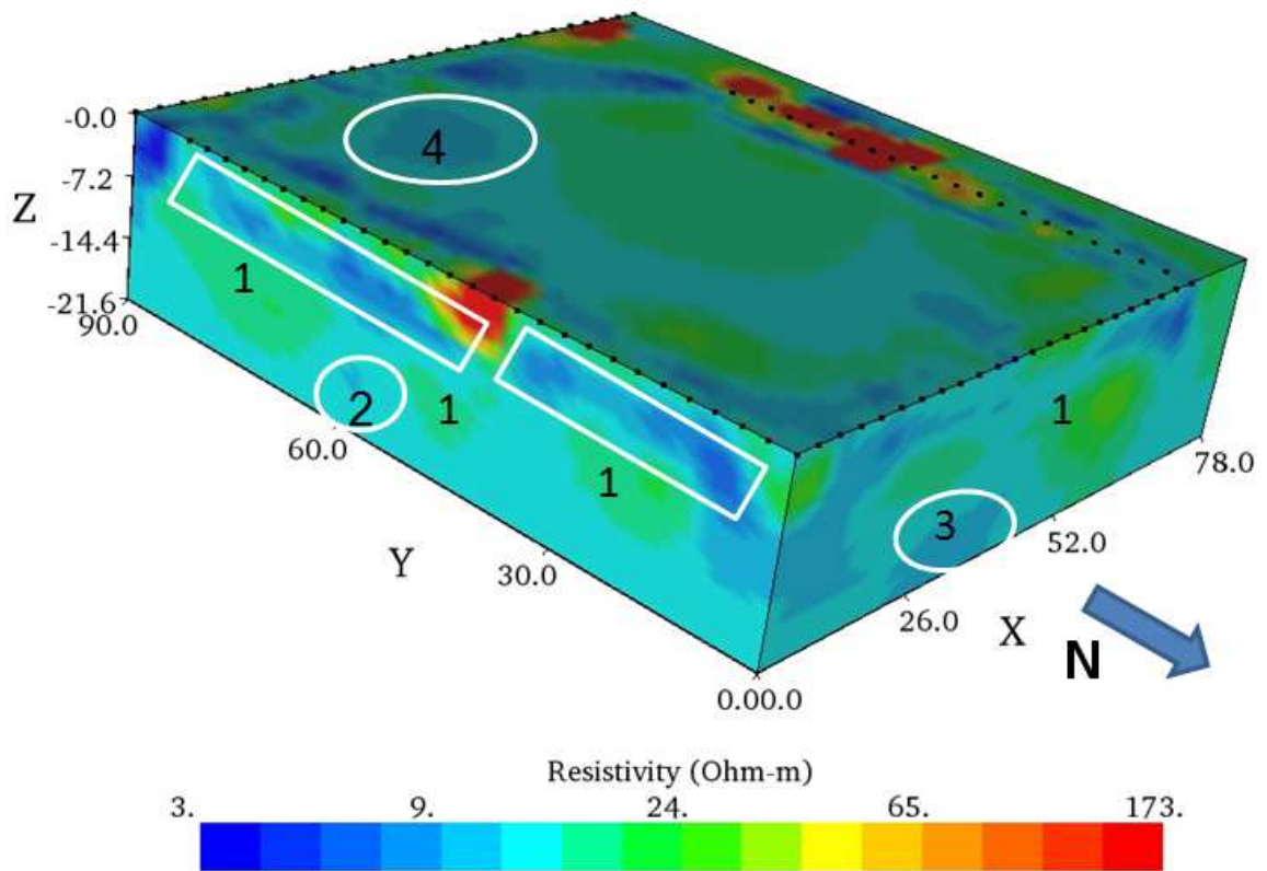
Figura 4.08. Cubo en 3D de la catedral de Morelia. El detalle de los números de encuentra en el texto.
