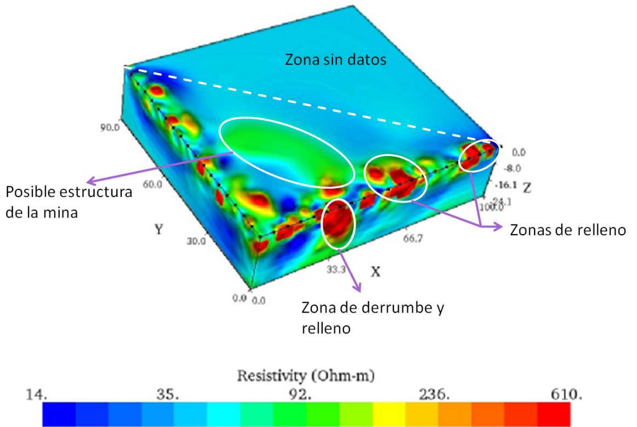
Figura 4.03 inversión de los datos del arreglo en L en la delegación Álvaro Obregón
