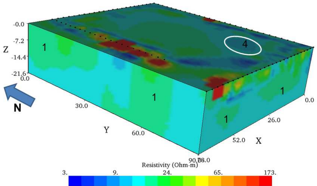
Figura 4.10. cubo en 3D de la catedral de Morelia Vista SW. Se observa el material insitu (1) y la estructura que coincide con la cripta de los obispos (4)
