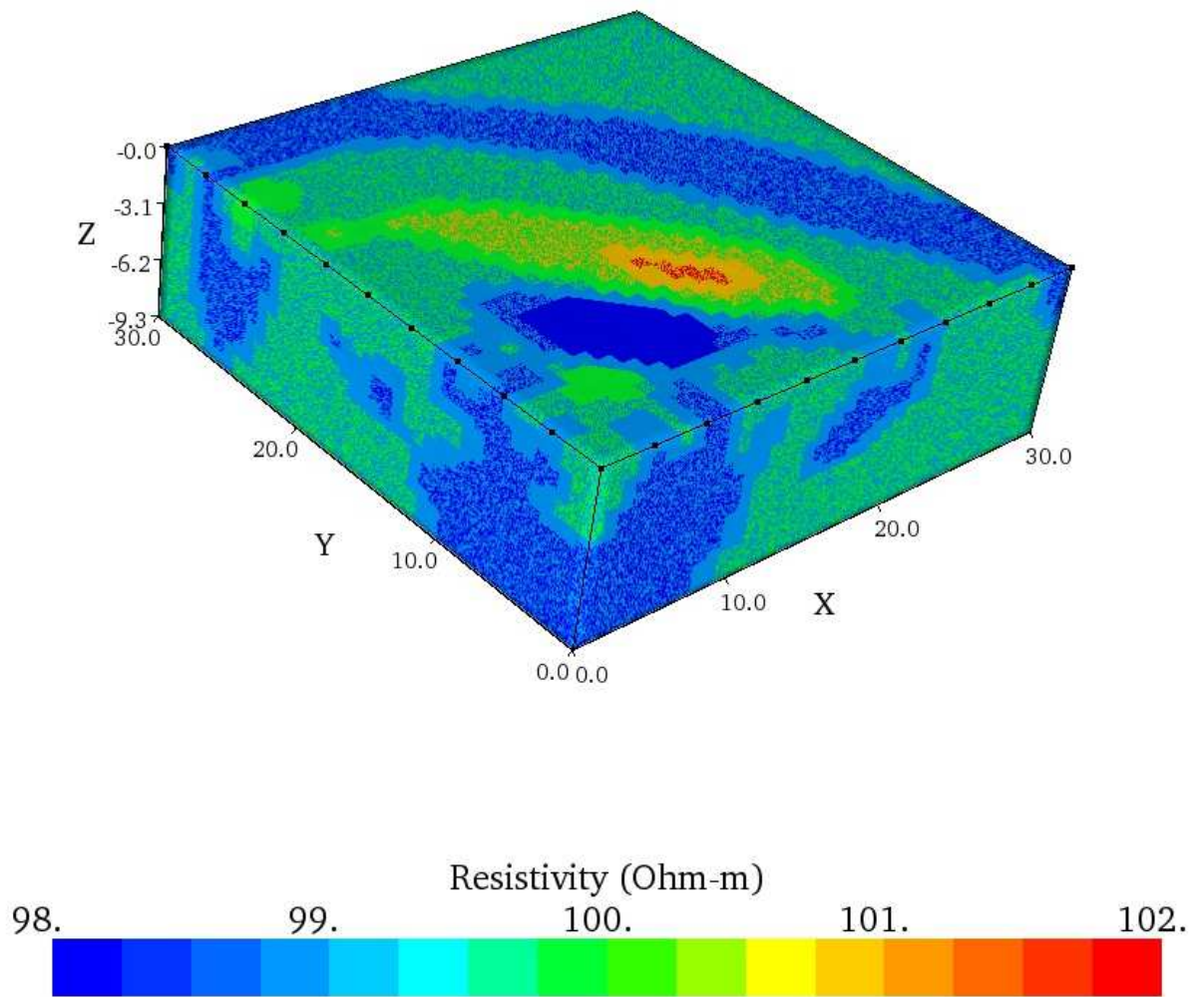
Figura 3.08) Inversión de los datos del Arreglo en “L” junto con el arreglo en “Esquina” para Modelado sintético de un cuerpo de dimensiones (5, 5, 3) unidades de rejilla.
