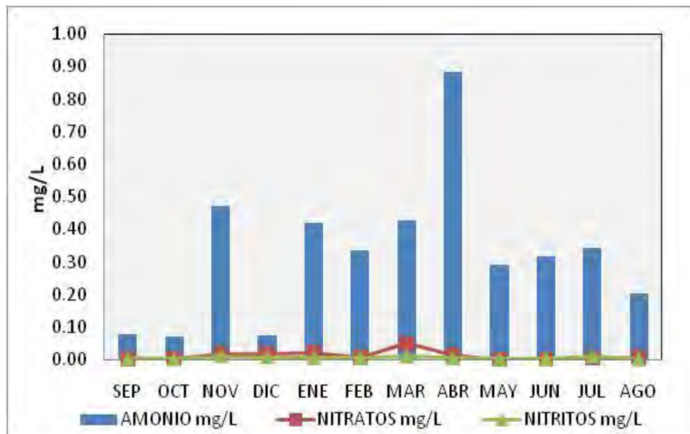
Fig. 8. Relación entre el amonio, nitratos y nitritos.
