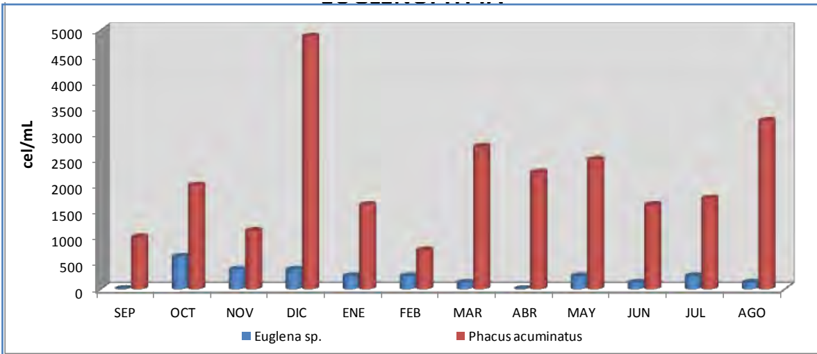
Fig. 17. Variación temporal de las principales especies de Euglenophyta en “Huitchila”, Morelos
