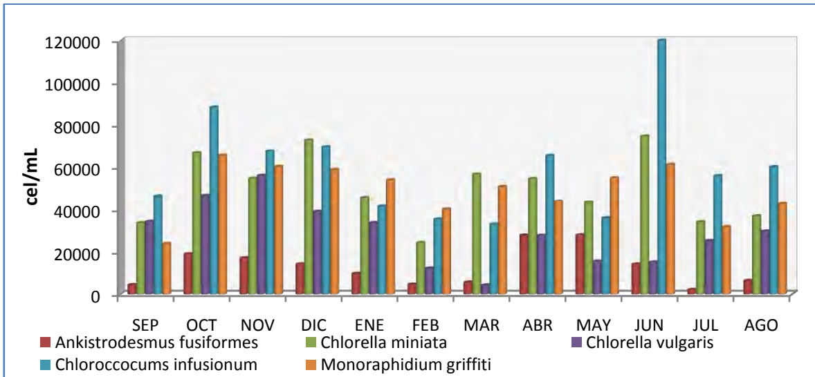
Fig. 15. Variación temporal de las principales especies de Chlorophyta en “Huitchila”, Morelos
