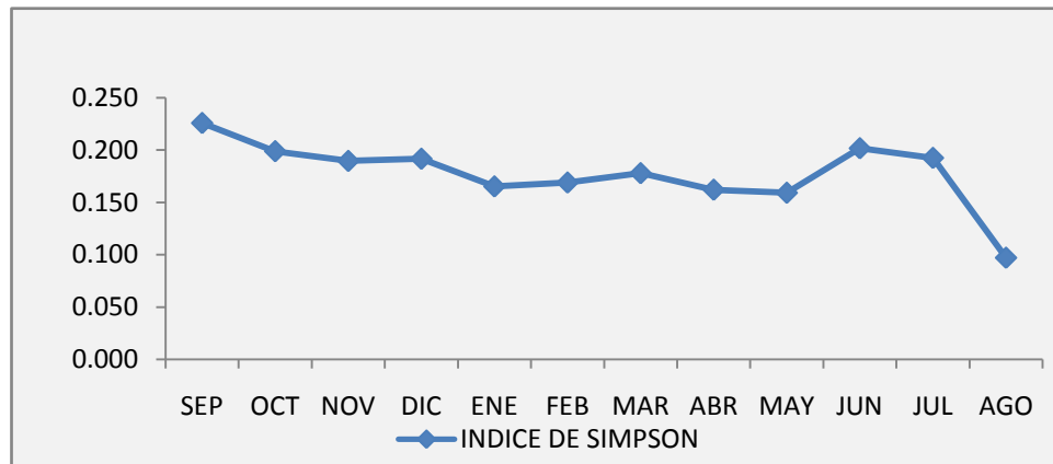
Fig. 19. Comportamiento temporal del índice de Simpson en Huitchila
