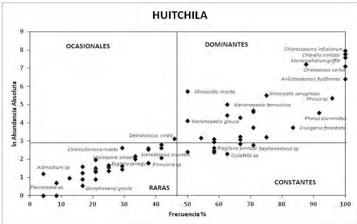
Fig. 20. Diagrama de asociación de Olmstead-Tuckey para el sistema “Huitchila”
