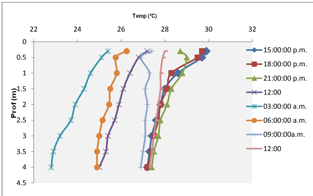
Fig. 23. Ciclo nictemeral de la temperatura en el sistema Huitchila, 26 de agosto de 2011.
