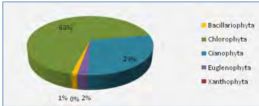
Fig. 11. Proporción de las principales divisiones fitoplanctónicas registradas en el sistema "Huitchila"
