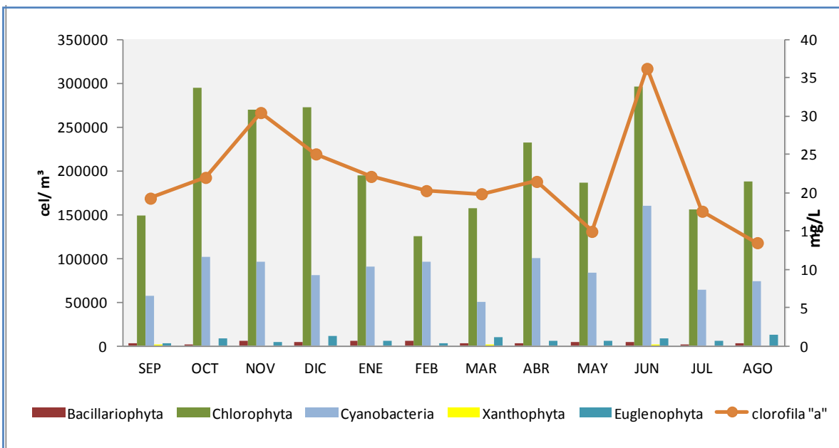
Fig. 12. Variación temporal de cada uno de los grupos fitoplanctónicos
