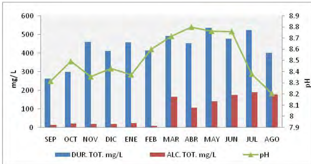
Fig. 6. Variación temporal de la alcalinidad total, dureza total y pH
