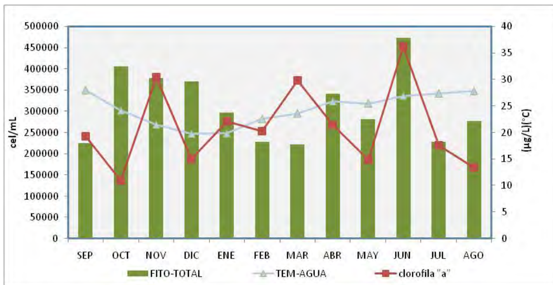
Fig. 10. Relacion entre la clorofila "a" y la abundancia del fitoplancton.
