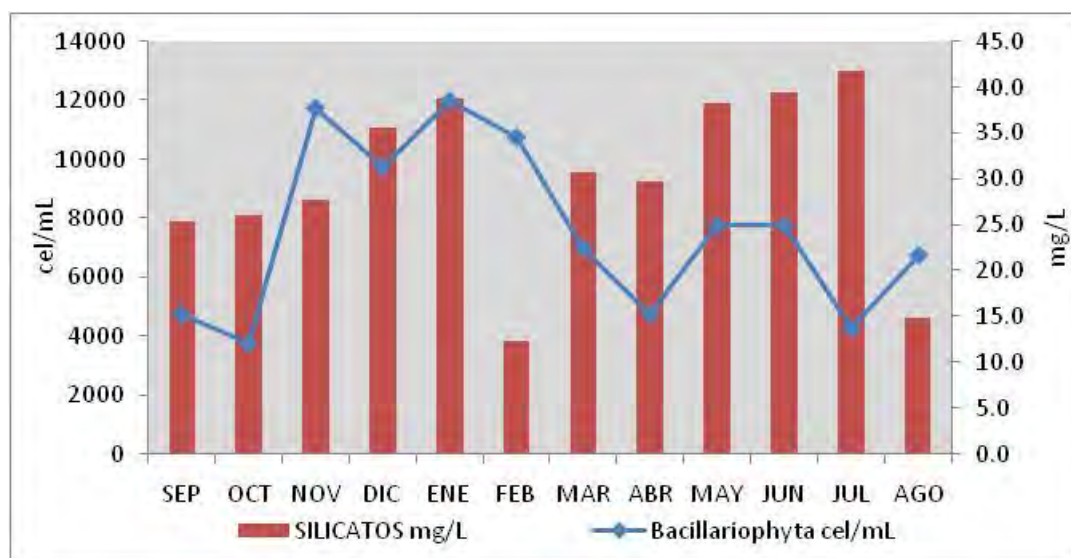
Fig. 9 Relación entre silicatos y Bacillariophyta.
