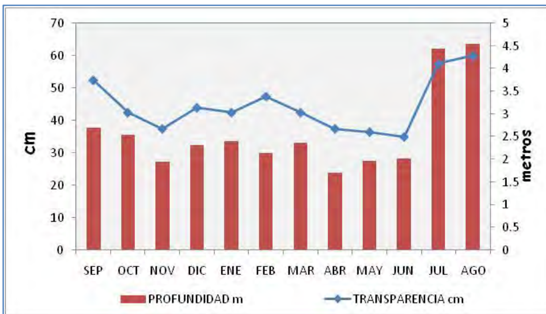
Fig. 4. Relación entre transparencia y la profundidad del agua
