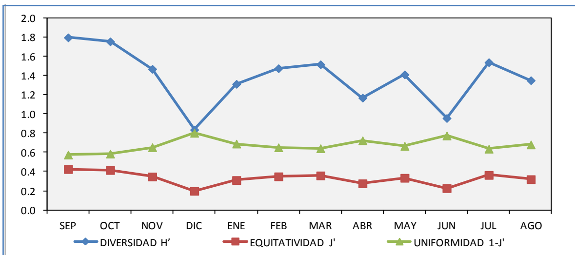
Fig. 18. Comportamiento temporal de los índices de Shannon-Wiener (Diversidad), Pielou (Equitatividad) y uniformidad del fitoplancton en el sistema Huitchila.
