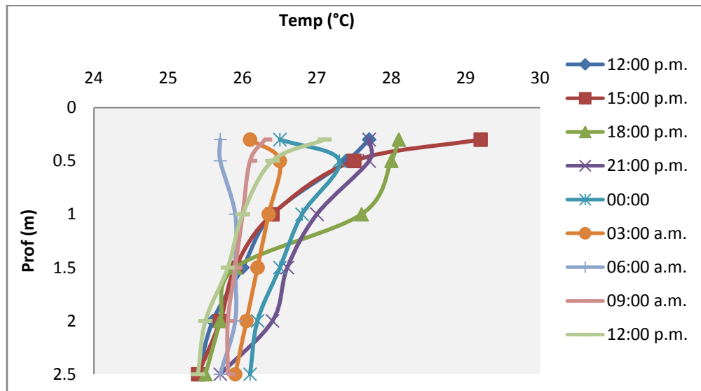
Fig. 21. Ciclo nictemeral de la temperatura del agua en el sistema Huitchila el 9 de abril de 2011
