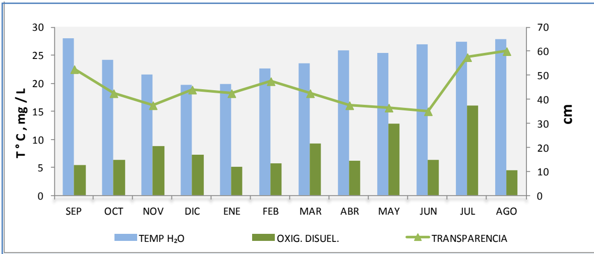
Fig. 5. Relación entre el oxígeno disuelto, transparencia y la temperatura del agua
