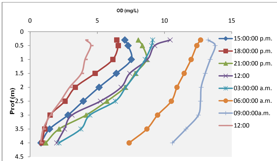
Fig. 24. Ciclo nictemeral del oxígeno disuelto el sistema Huitchila, 26 de agosto de 2011.
