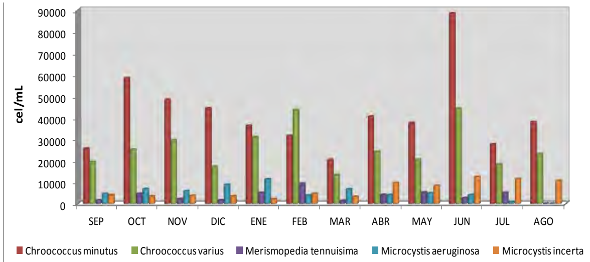
Fig. 16. Variación temporal de las principales especies de Cyanophycota en “Huitchila”, Morelos
