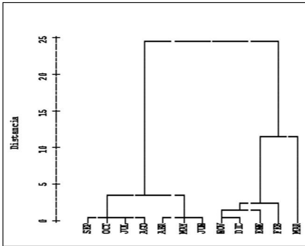
Fig. 26. Dendograma que muestra la asociación de los meses de muestreo para el sistema Huitchila
