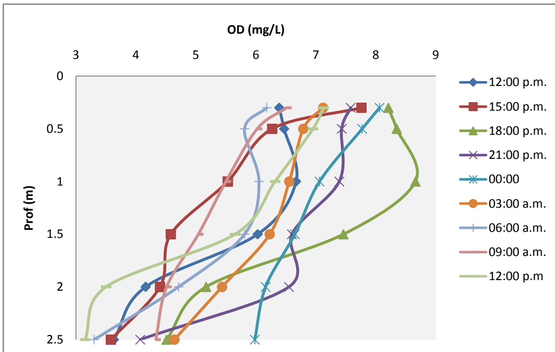
Fig. 22. Ciclo nictemeral del oxígeno disuelto en el sistema Huitchila, 9 de abril de 2011.
