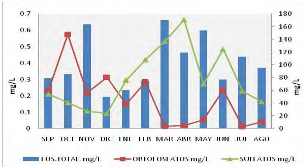
Fig. 7. Relación de los ortofosfatos, fósforo total y sulfatos, para el bordo Huitchila
