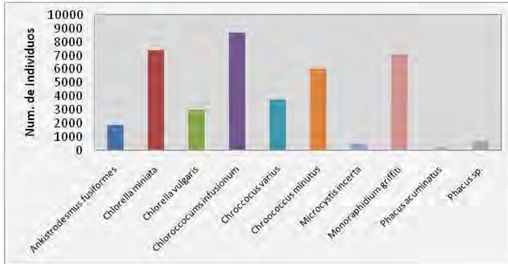
Fig.13. Especies que presentaron mayor abundancia durante el estudio
