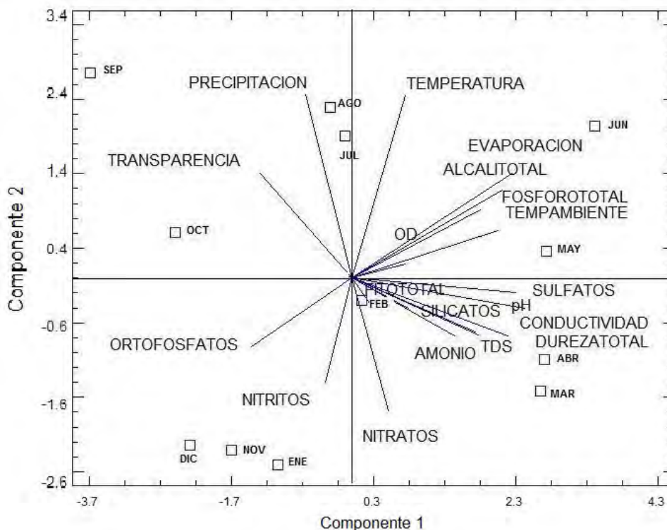
Fig. 25. Representación grafica de los pesos de los componentes.
