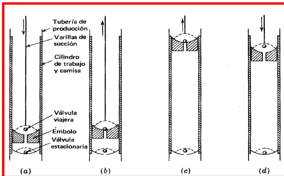
Fig. 1.15.- Ciclo de bombeo del BM: a) el émbolo se mueve hacia abajo cerca del fondo de la carrera, b) el émbolo sube, cerca del fondo de la carrera, c) el émbolo sube cerca de la parte superior de la carrera, d) el émbolo se mueve hacia abajo cerca del tope de la carrera. Fuente: Fundamentos de producción y mantenimiento de pozos petroleros
