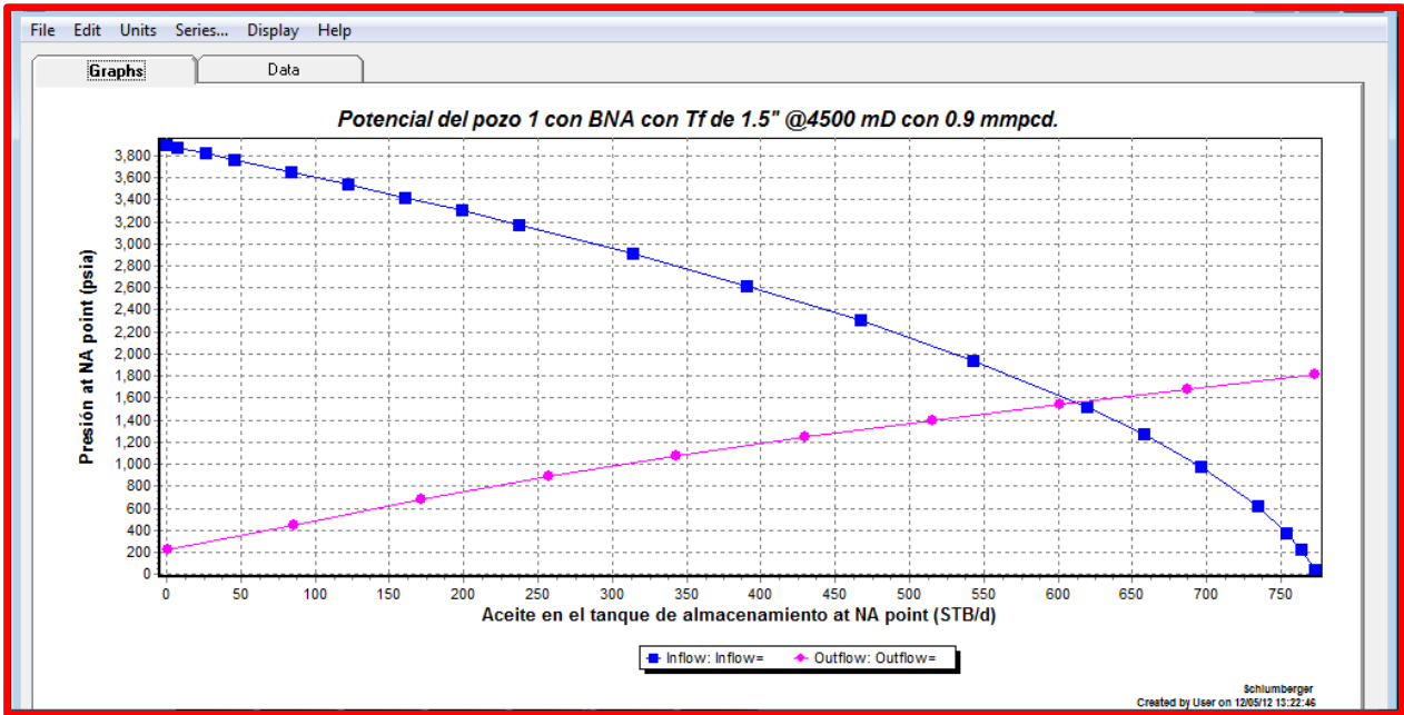
Fig. 4.33.- Curvas de comportamiento de afluencia y capacidad de transporte para el aceite con BNA.
