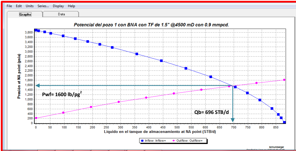
Fig.5.6.-Comportamiento de afluencia y capacidad de transporte del Pozo 1 con BNA.
