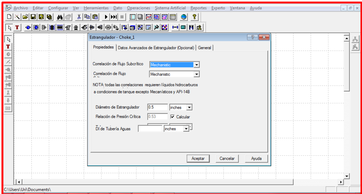
Fig. 4.11.- Configuración de la apertura del estrangulador ½ “
