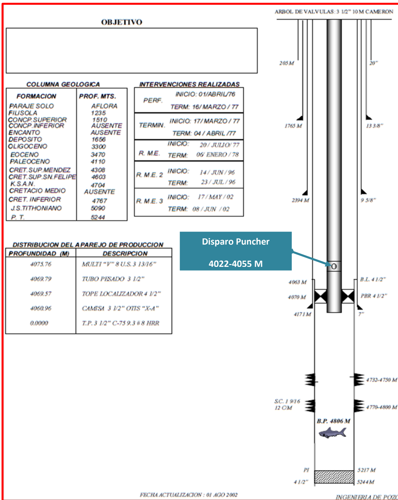
Fig. 4.46.- Estado mecánico del pozo 2 con un disparo puncher
