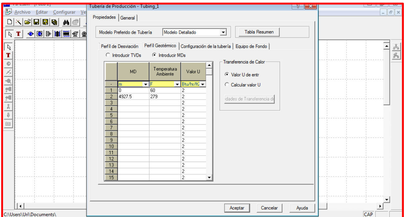
Fig. 4.9.- Configuración del perfil geotérmico de TP
