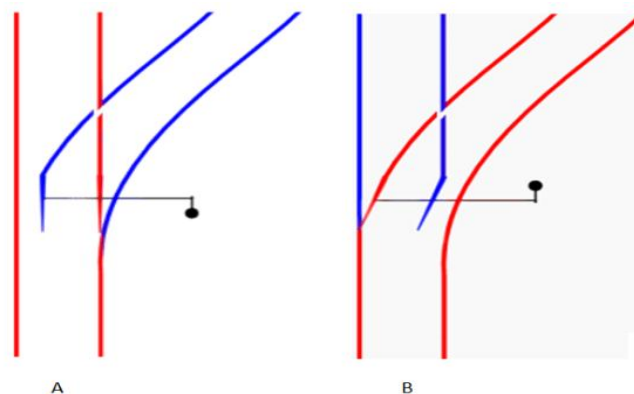
Figura 2.22. Representación de un cambio de vía sencillo.
