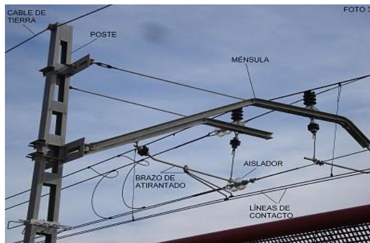
Figura 2.62. Esquema general de los elementos que componen una catenaria.
