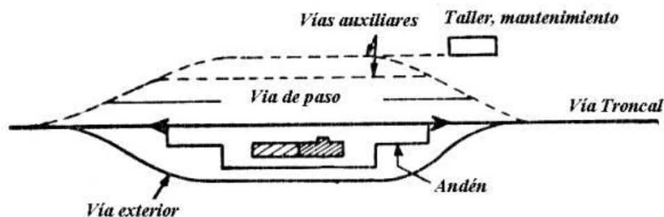
Figura 2.4. Configuración típica de una estación de paso para pasajeros.
