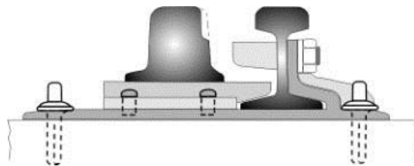
Figura 2.28. Cojinetes de resbalamiento fijados sobre los durmientes.
