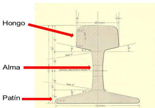
Figura 2.7. Partes que conforman el riel.
