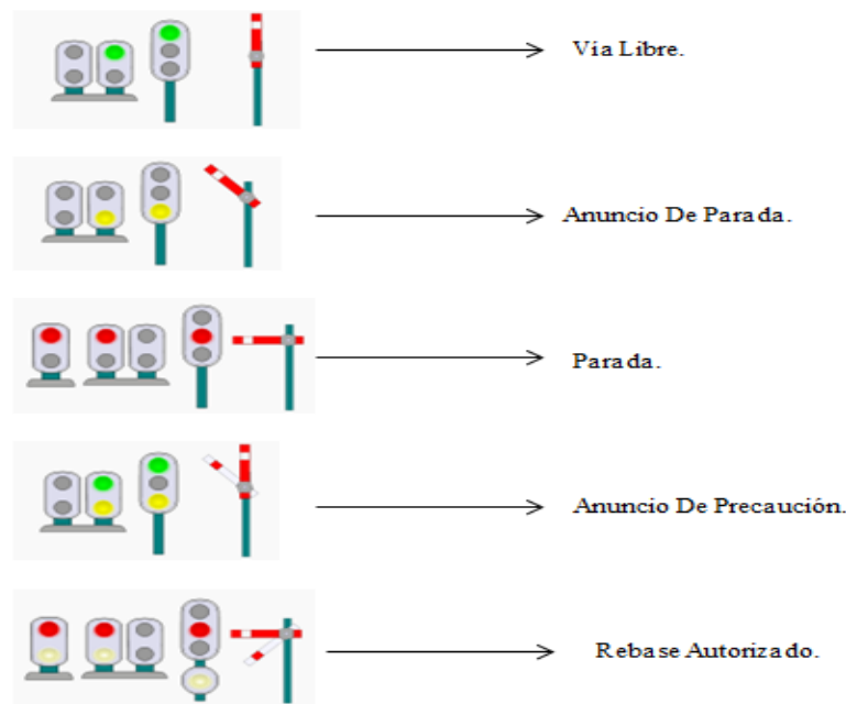
Figura 2.56. Señalización de semáforos en vías férreas.
