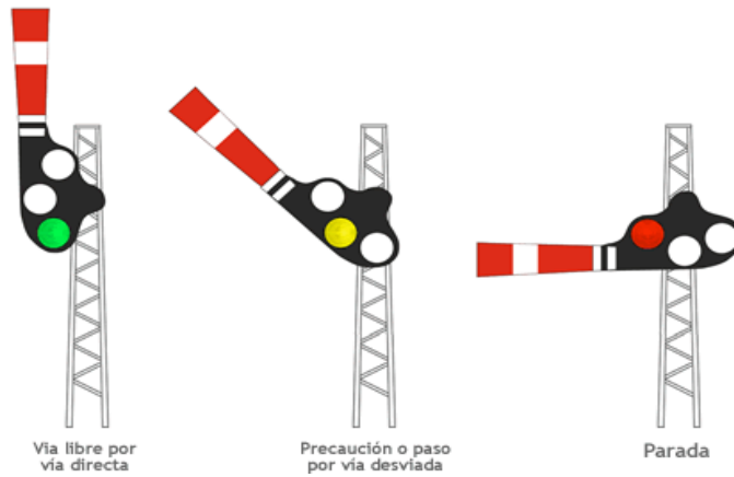
Figura 2.53. Señales mecánicas.
