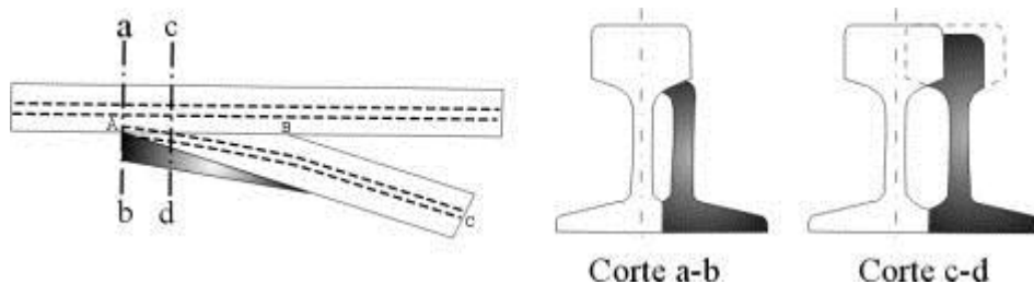
Figura 2.25. Encuentro de las cabezas de los rieles y sección transversal de aguja y contra aguja.
