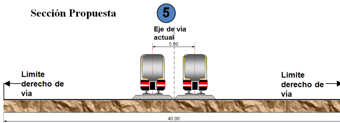
Figura 4.45. Sección propuesta de la vía férrea mostrando el derecho de vía que quedara disponible.
