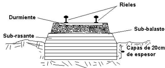
Perfil de la vía ferroviaria
