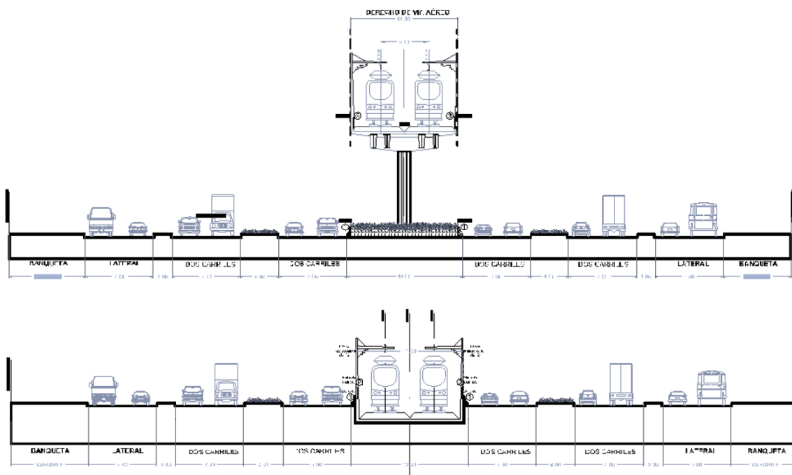
Figura 4. 24. Secciones de tramos sobre la autopista México – Puebla.
