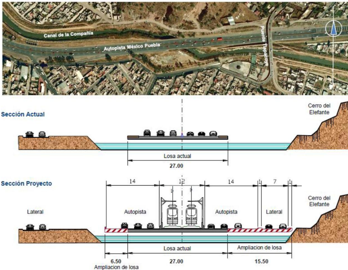
Figura 4.29. Esquema de cruce en el canal de la compañía.
