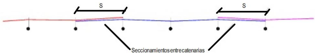
Figura 2.64. Seccionamiento de catenarias.
