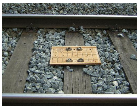
Figura 2.57. Baliza EBICAB instalada en el corredor Mediterráneo.
