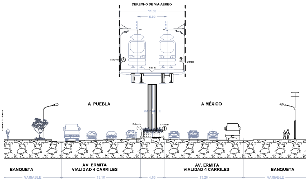
Figura 4.28. Sección tipo de estructura elevada sobre Ermita – Iztapalapa.
