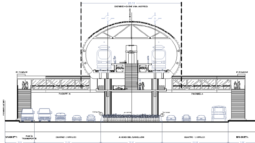
Figura 4. 27. Sección de estación tipo elevada sobre el tramo Ermita – Iztapalapa.
