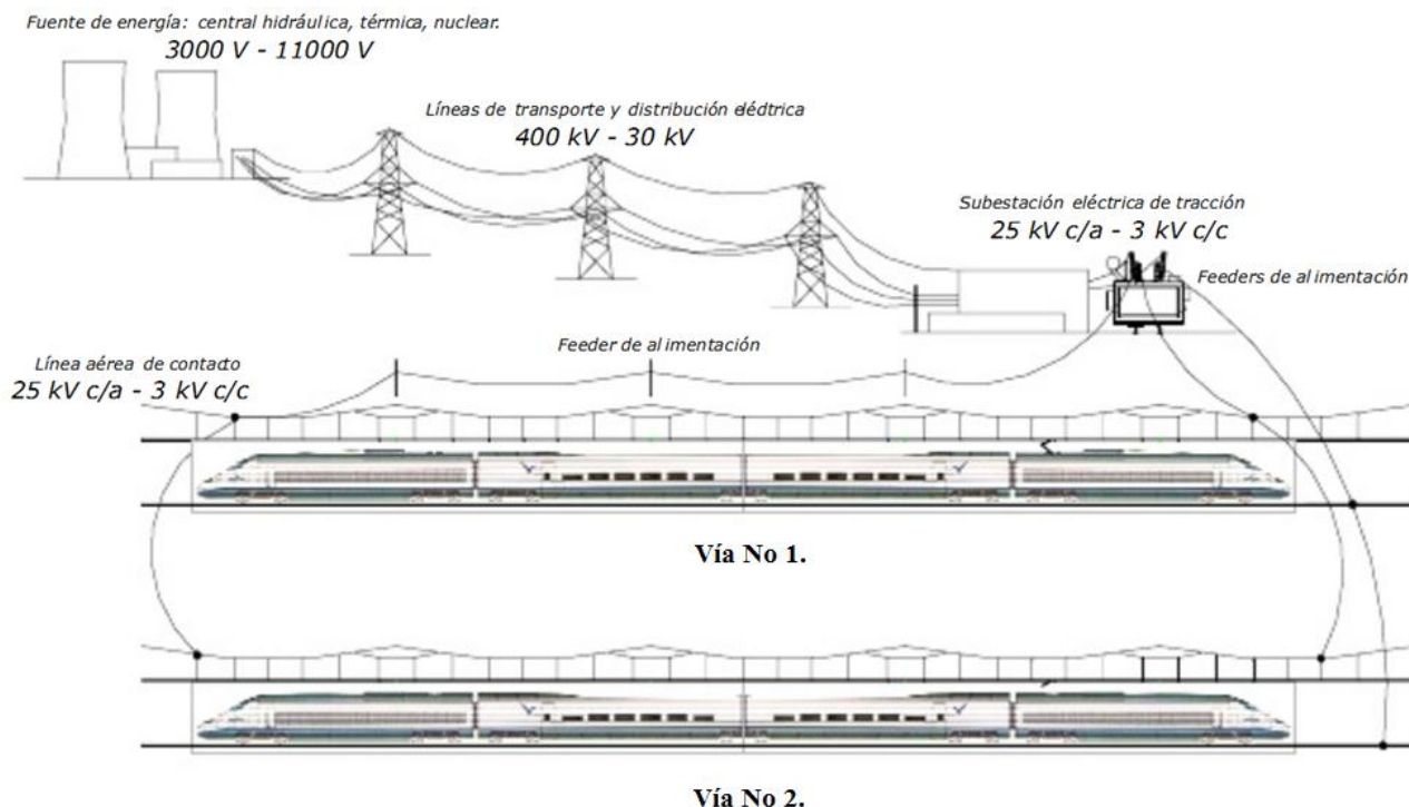
Figura 2.65. Esquema representativo de los elementos que componen un sistema eléctrico ferroviario.
