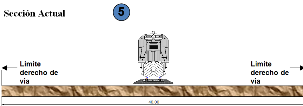
Figura 4.44. Sección actual de la vía férrea mostrando el derecho de vía disponible.
