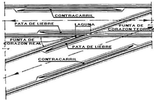
Figura 2.30. Partes que constituyen un cruce de vías.
