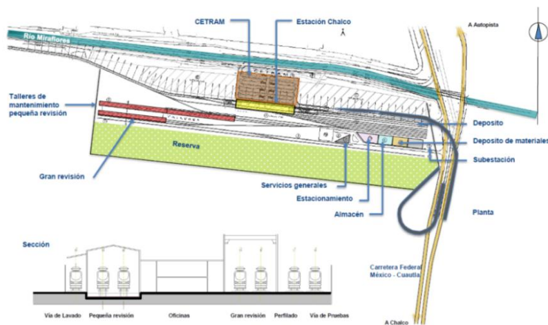
Figura 4.22. Talleres de mantenimiento en la zona de Chalco.
