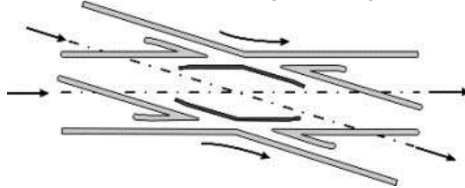
Figura 2.20. Entre vía oblicua.
