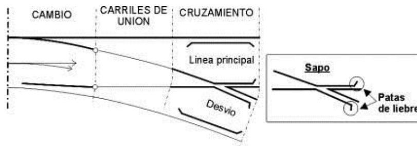
Figura 2.18. Desvíos y cruzamientos.
