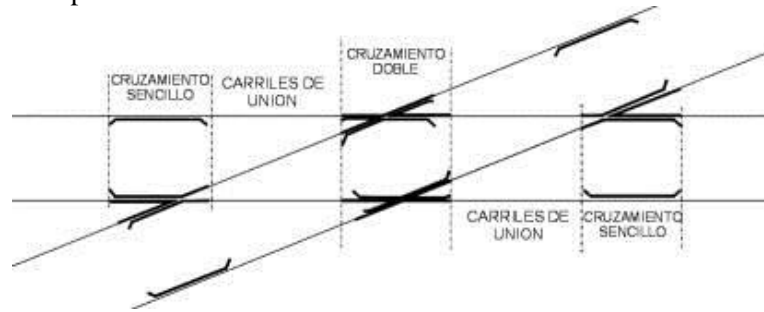
Figura 2.19. Entre vía rectangular.
