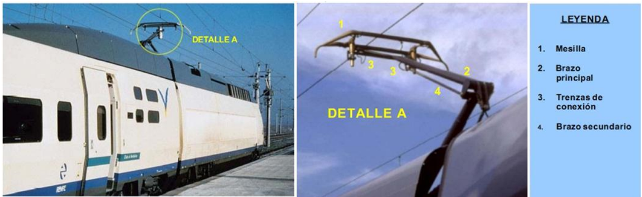
Figura 2.63. Pantógrafo de un tren de la serie 100 de Renfe (trenes Ave).
