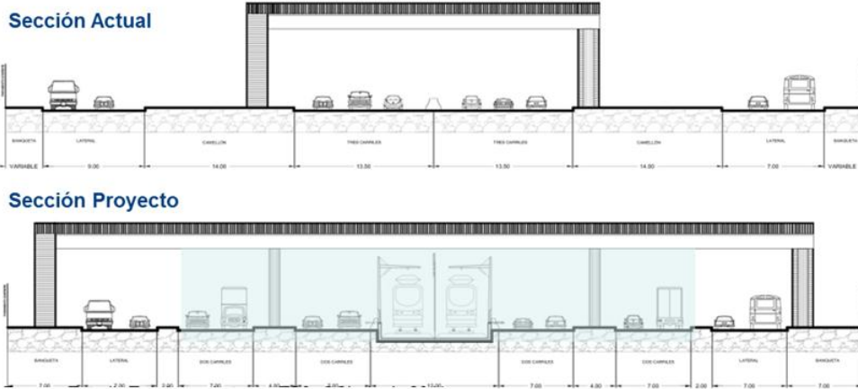
Figura 4.25. Secciones de tramos sobre la autopista México – Puebla.
