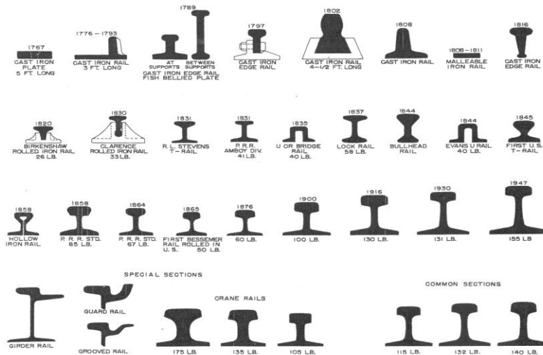
Figura 2.8. Perfiles de los tipos de rieles más utilizados.
