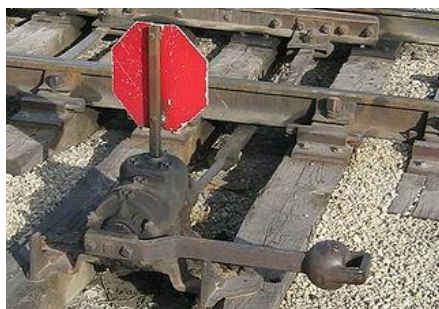
Figura 2.23. Palanca para cambios de vía de forma manual.
