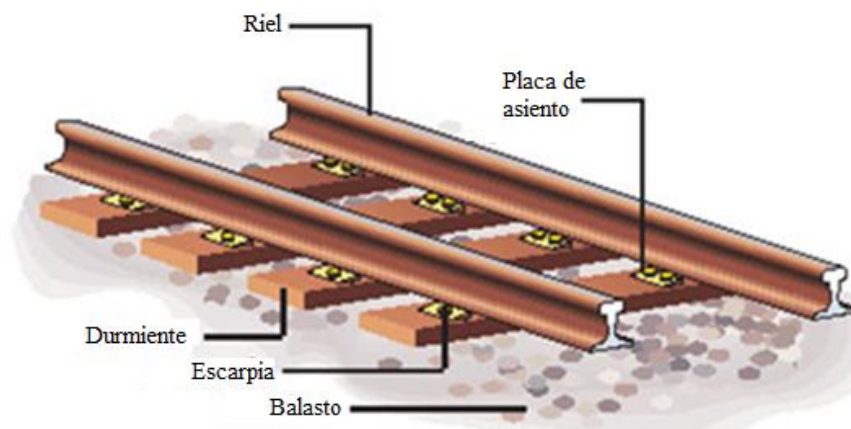
Figura 2.5. Componentes de una vía férrea.
