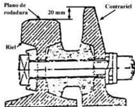
Figura 2.29. Elevación del contrarriel sobre el plano de rodadura.
