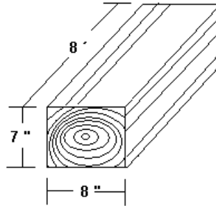
Figura 2.12. Dimensiones del durmiente de madera.
