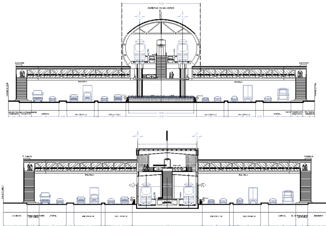
Figura 4. 26. Secciones de estaciones sobre la autopista México – Puebla.
