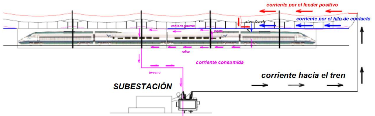
Figura 2.67. Esquema del circuito eléctrico de tracción ferroviaria.
