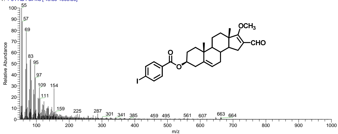
Espectro 25.4
