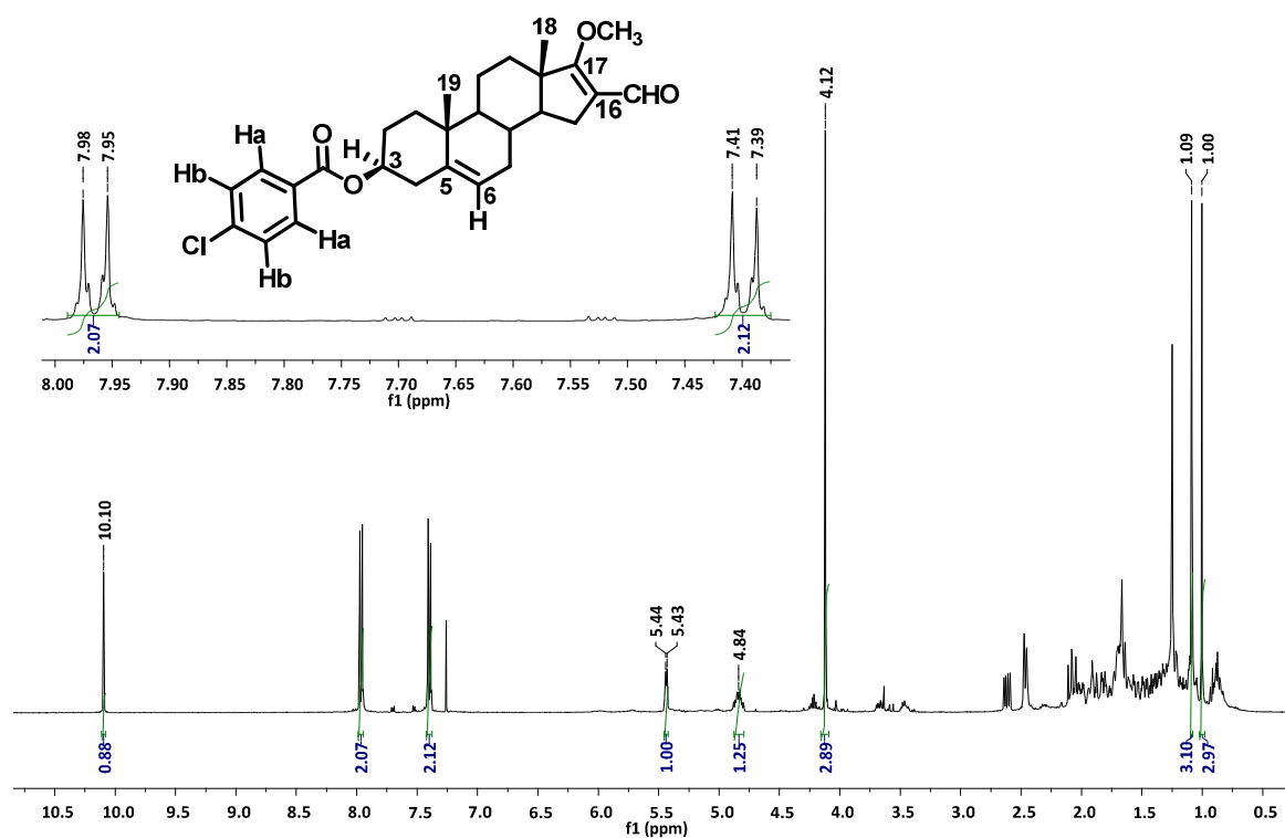
Espectro 23.2
