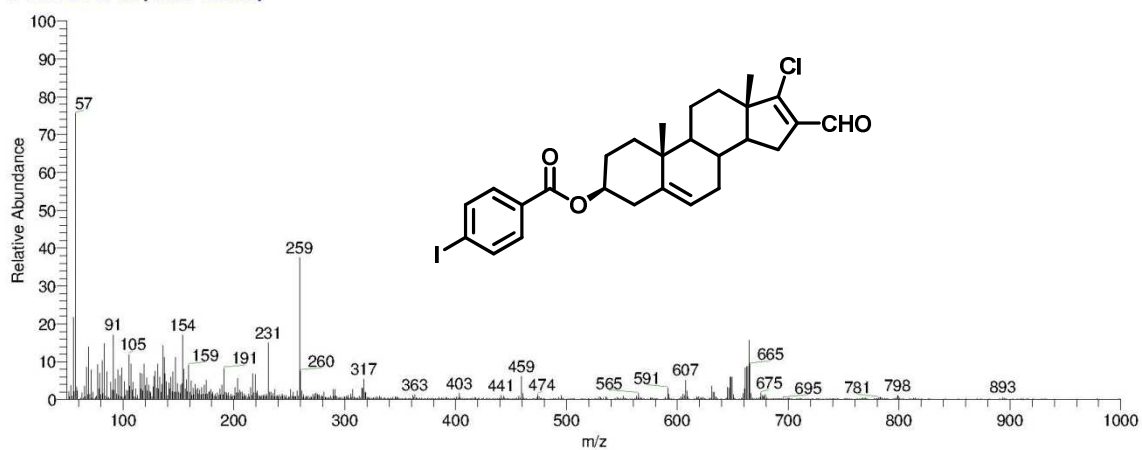
Espectro 11.4
