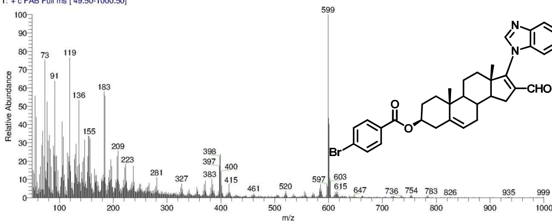
Espectro 16.4
