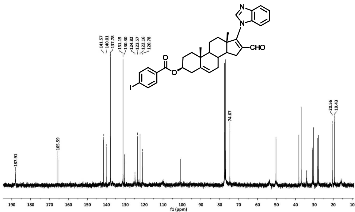
Espectro 17.3
