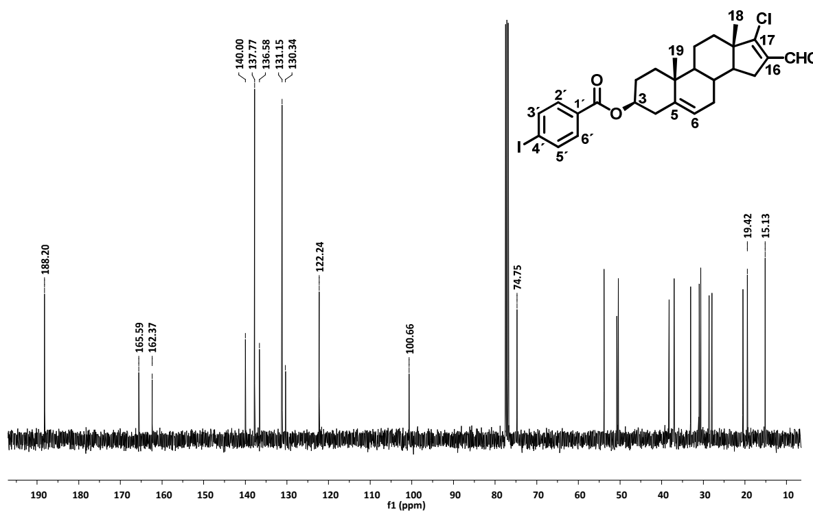
Espectro 11.3
