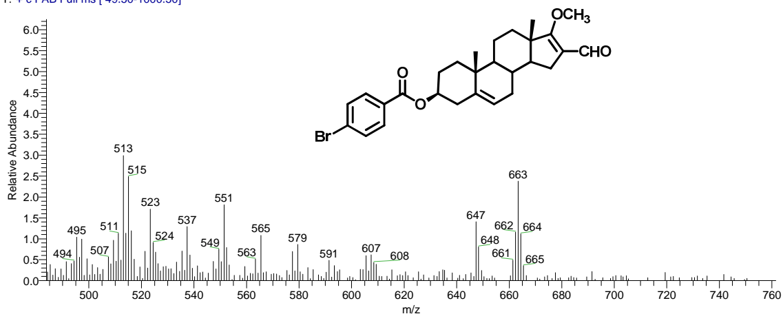
Espectro 24.4.1
