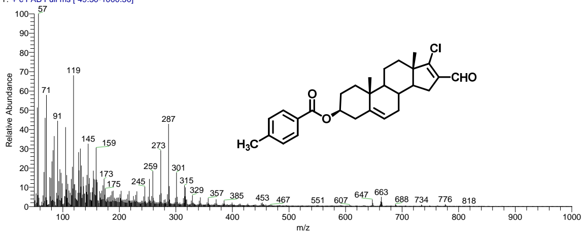
Espectro 12.4
