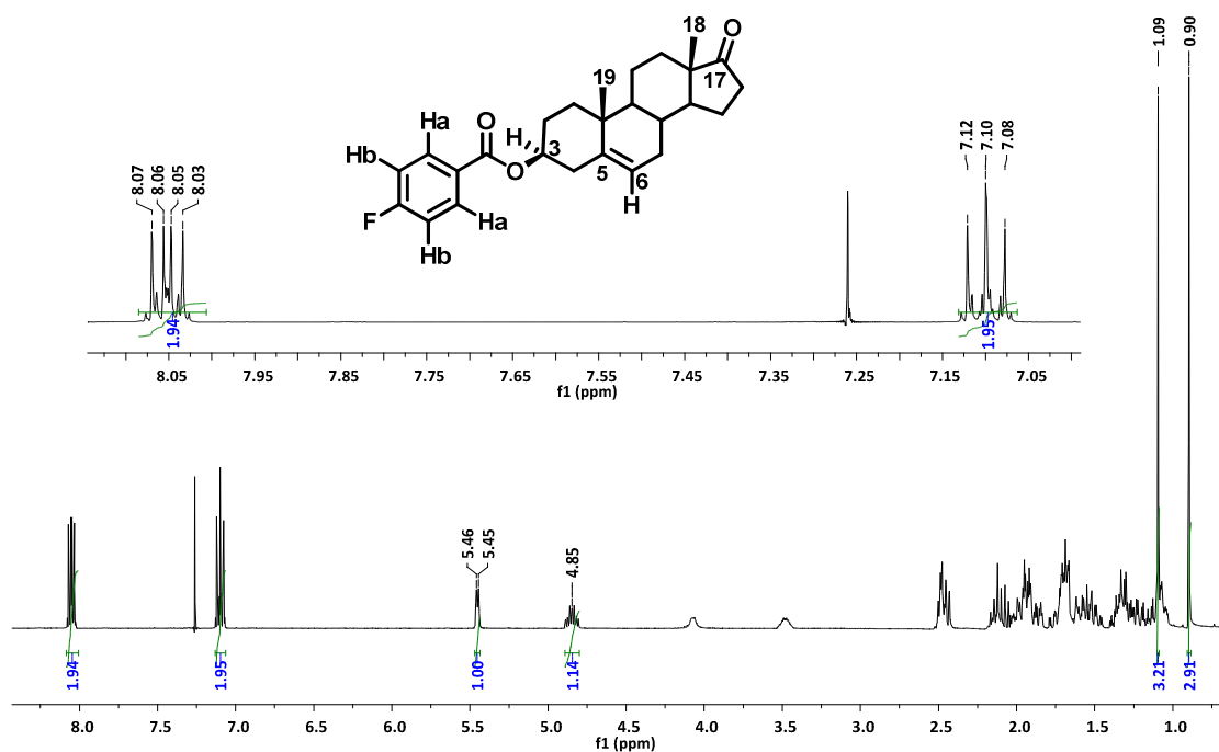
Espectro 2.2
