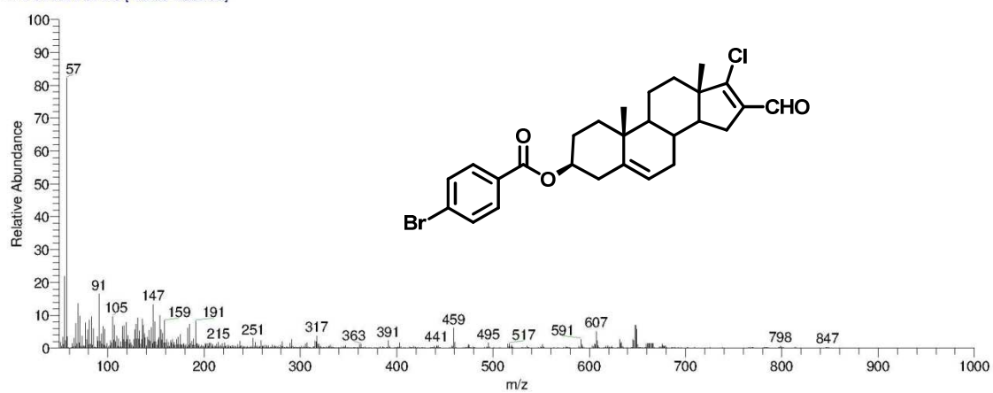
Espectro 10.4
