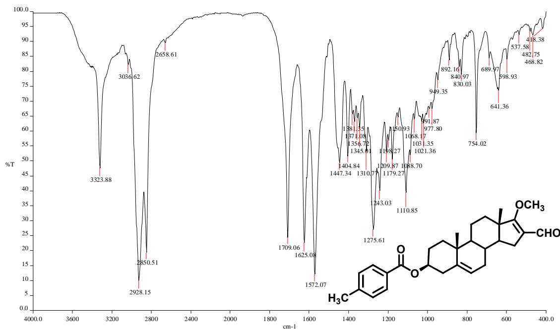
Espectro 26.1
