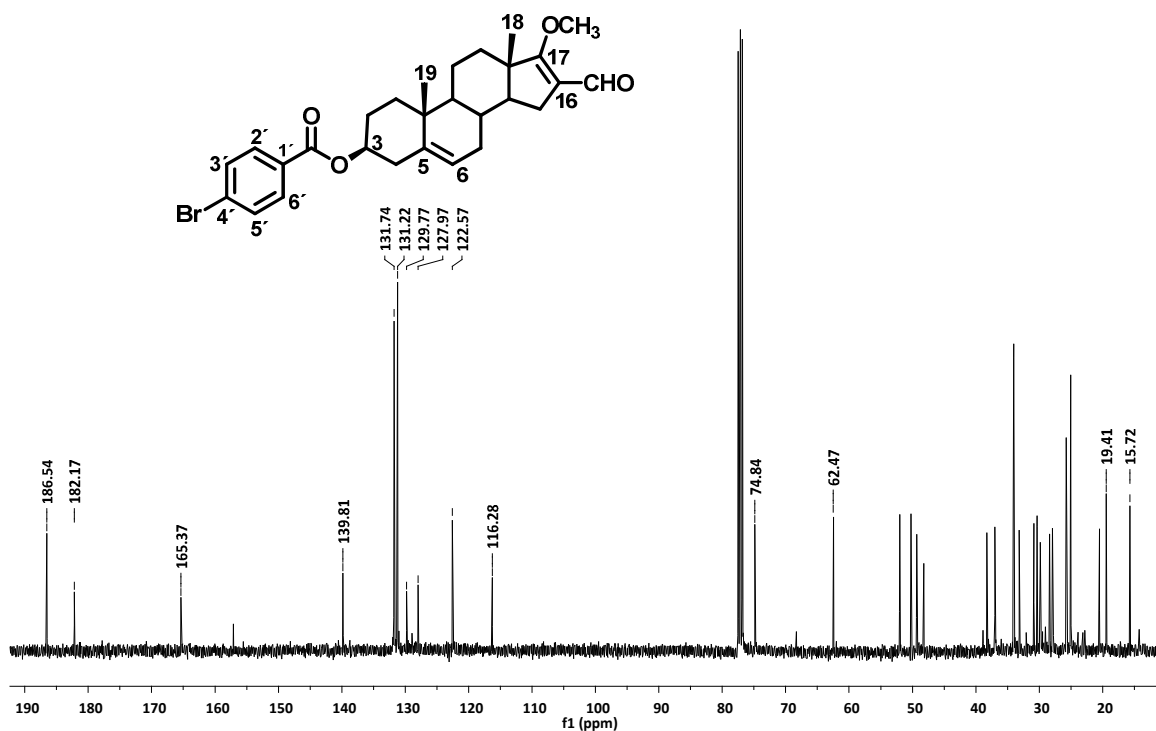
Espectro 24.3
