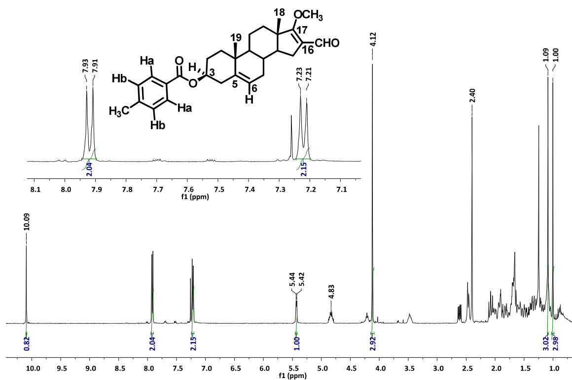
Espectro 26.2
