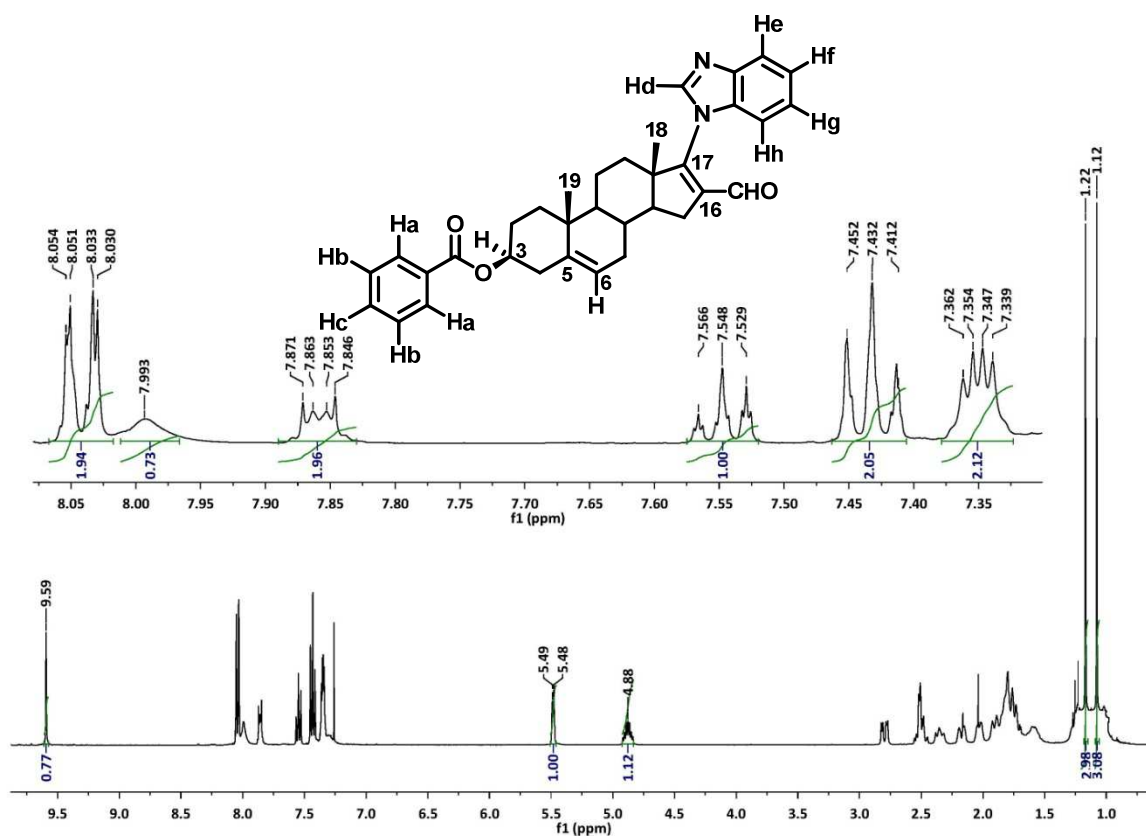
Espectro 13.2
