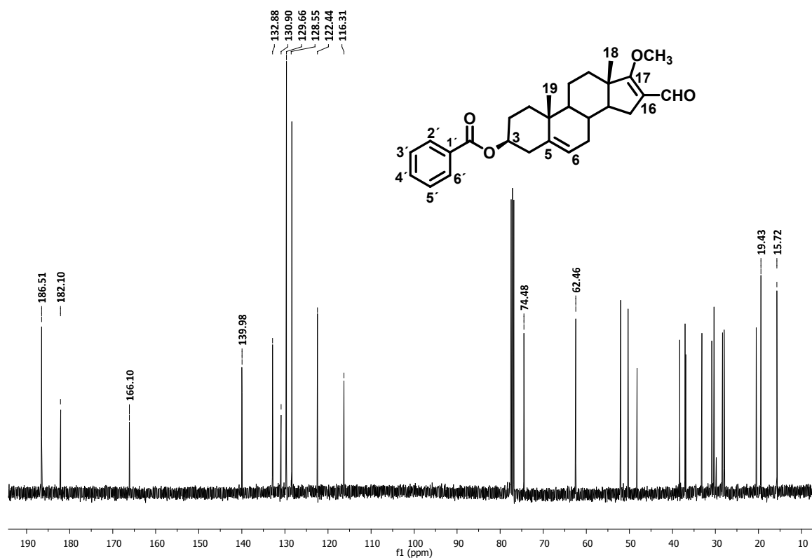
Espectro 21.3
