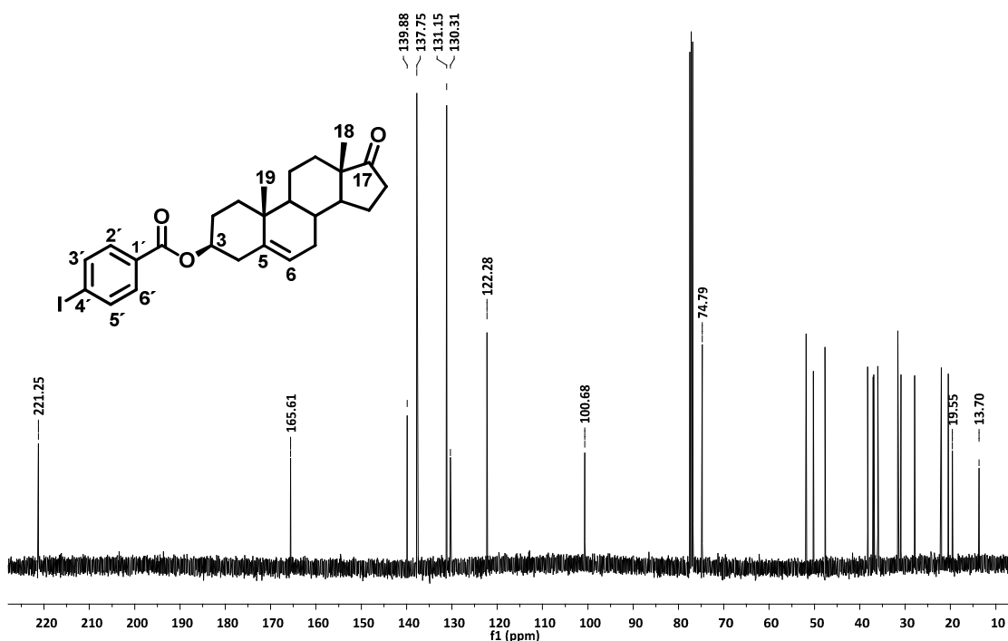
Espectro 5.3
