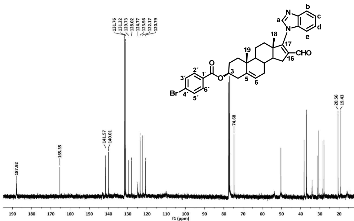
Espectro 16.3
