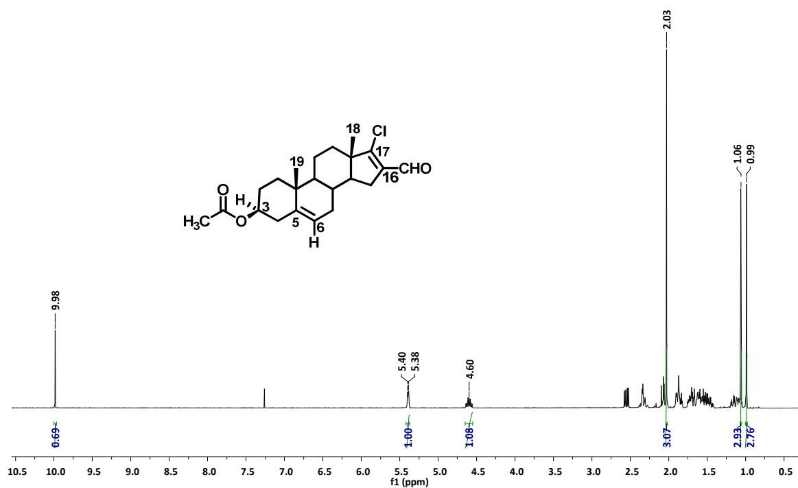
Espectro 19.2
