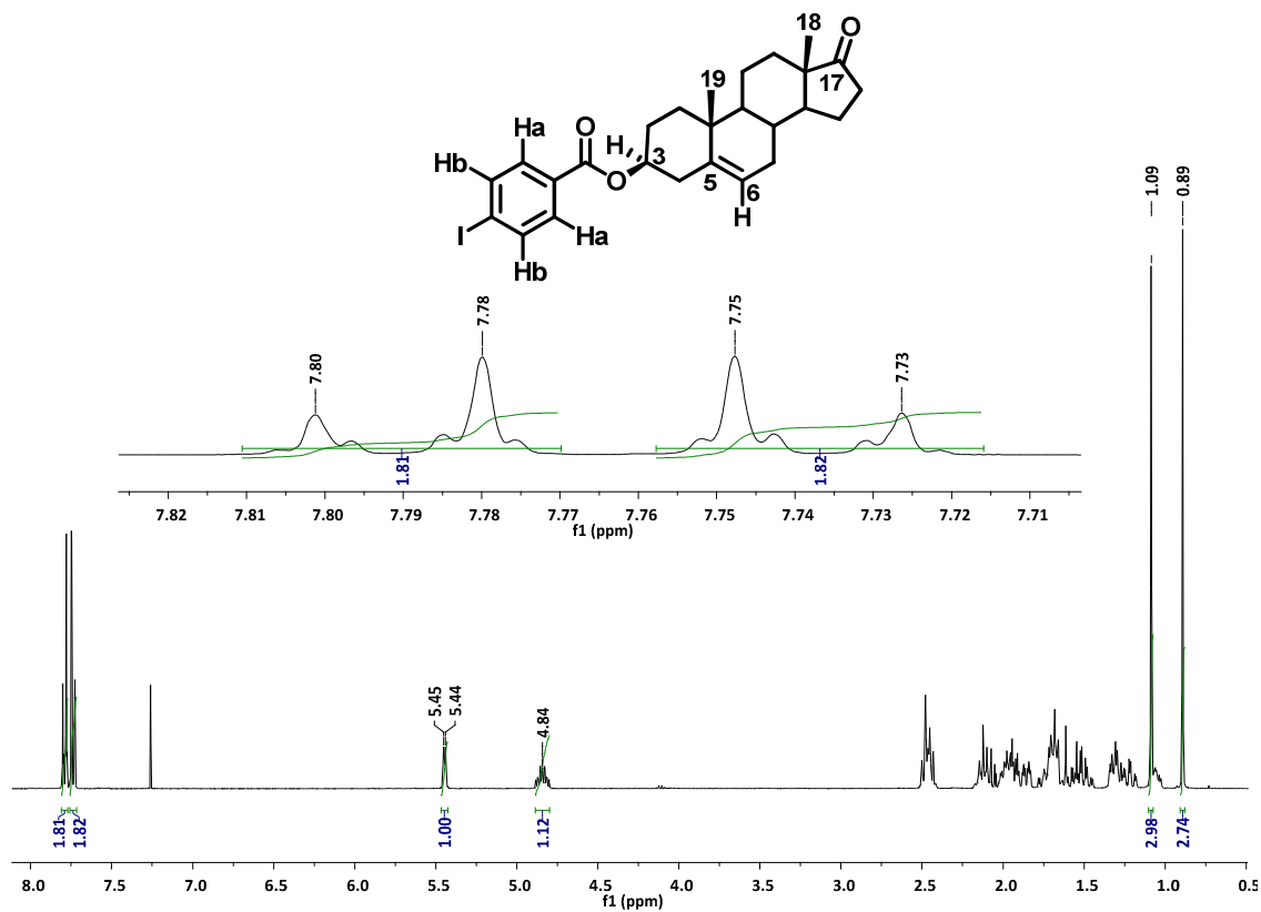
Espectro 5.2
