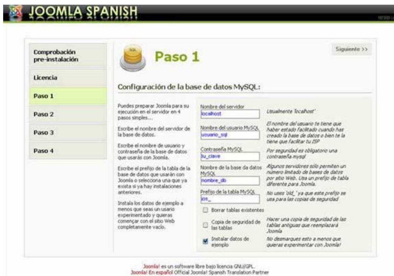
Figura 5.33. Ventana de configuraci3n de la base de datos MySQL.
