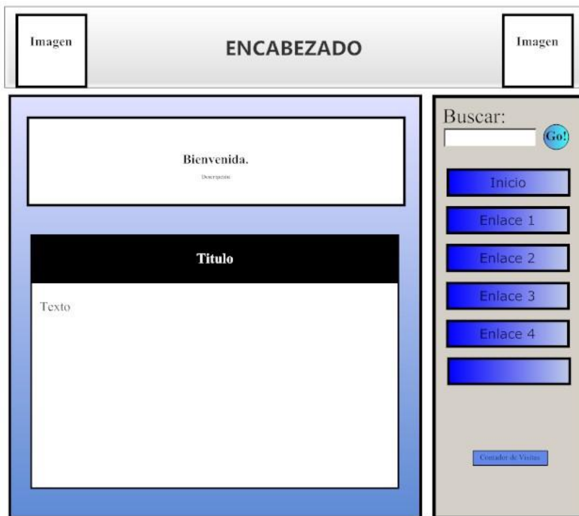
Figura 5.14. Boceto de la p3gina de inicio.
