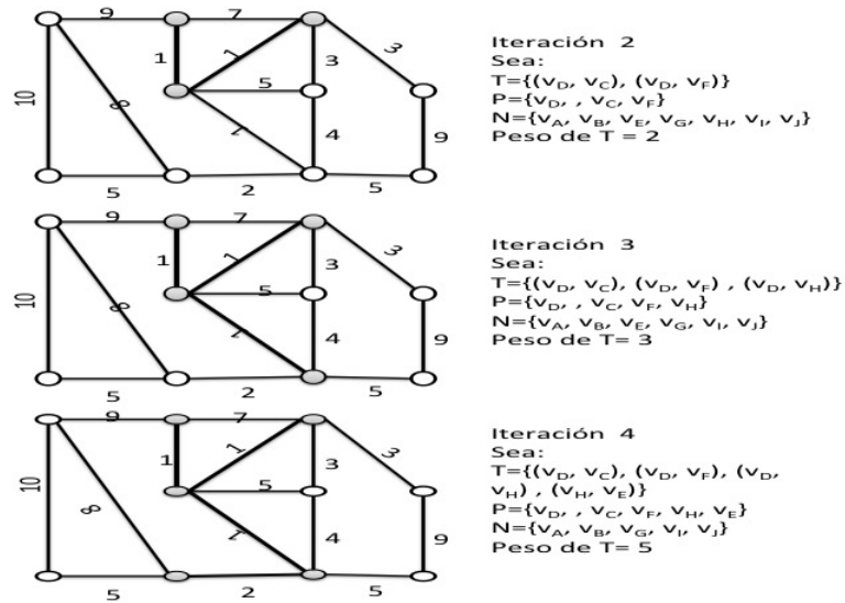
Figura 1.27: Aplicación el algoritmo de Prim (continuación).
