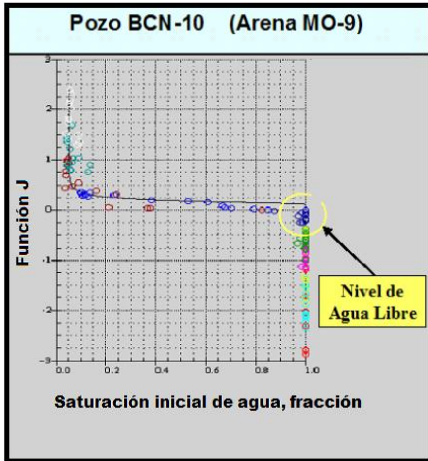
Gráfica 4.13. Nivel de agua libre según la función J en el pozo BCN-10
