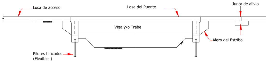
Fig. 1. Características típicas de un puente integral
