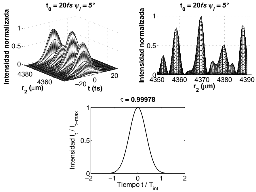
Figura 3.24: \tau_0 = 20 fs, \psi_i = 5^\circ , Iluminación Gaussiana, k = k_0, S_{III} + S_{IV}
