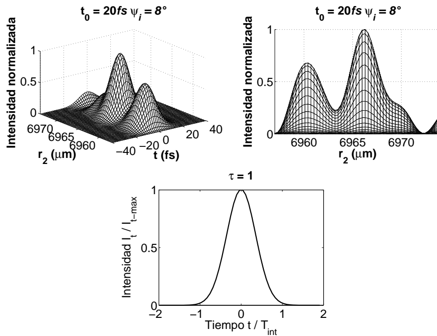
Figura 3.16: \tau_0 = 20\text{fs} , \psi_i = 8^\circ , Iluminación Gaussiana, k = k_0 , coma
