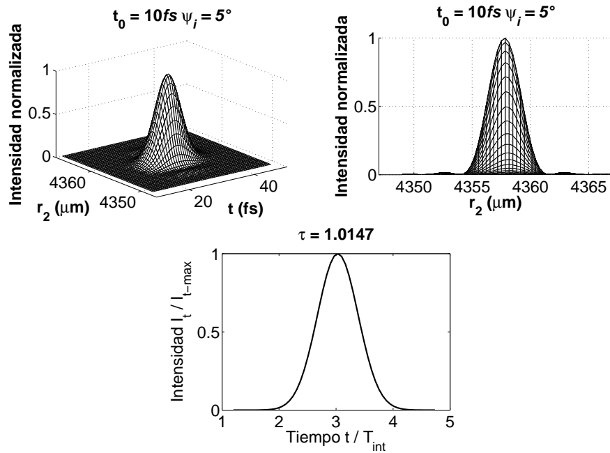
Figura 2.50: Duración inicial \tau_0 = 10 fs , \psi_i = 5^\circ , iluminación uniforme.
