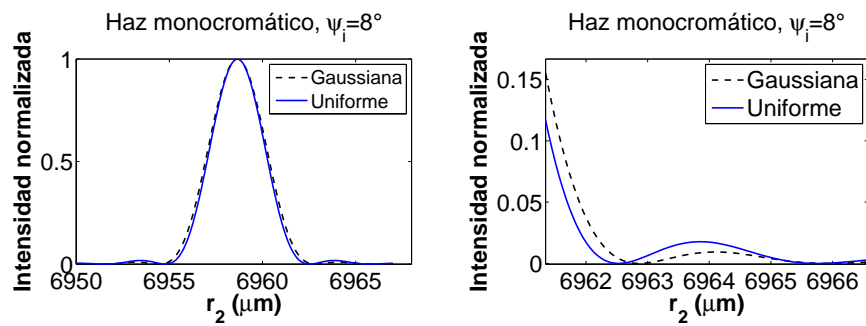
Figura 1.25: Incidencia \psi_i = 8^\circ .
