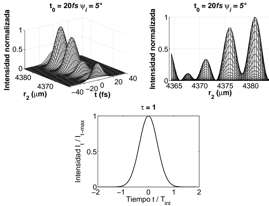
Figura 3.15: \tau_0 = 20\text{fs} , \psi_i = 5^\circ , Iluminación Gaussiana, k = k_0 , coma
