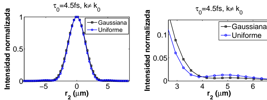
Figura 2.64: Pulso de 4.5 fs sin la aproximación k = k_0 con iluminación Gaussiana y Uniforme.
