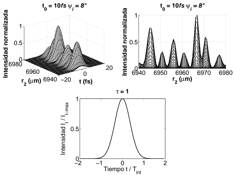
Figura 3.67: \tau_0 = 10\text{fs} , \psi_i = 8^\circ , Iluminación uniforme, k = k_0 , todas las aberraciones
