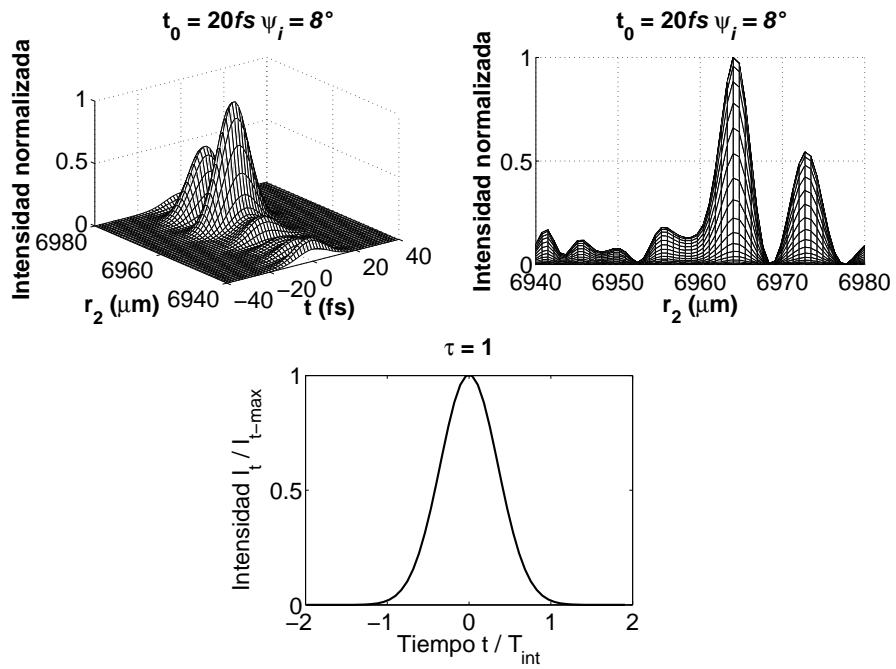
Figura 3.7: \tau_0 = 20 fs , \psi_i = 8^\circ , Iluminación Gaussiana k = k_0 , aberración esférica
