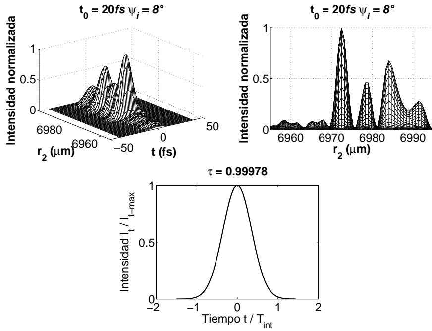
Figura 3.25: \tau_0 = 20 fs, \psi_i = 8^\circ , Iluminación Gaussiana, k = k_0, S_{III} + S_{IV}
