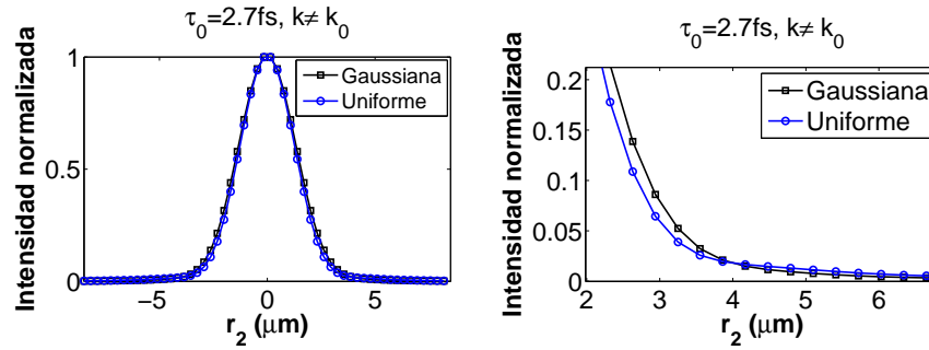
Figura 2.63: Pulso de 2.7 fs sin la aproximación k = k_0 con iluminación Gaussiana y Uniforme.
