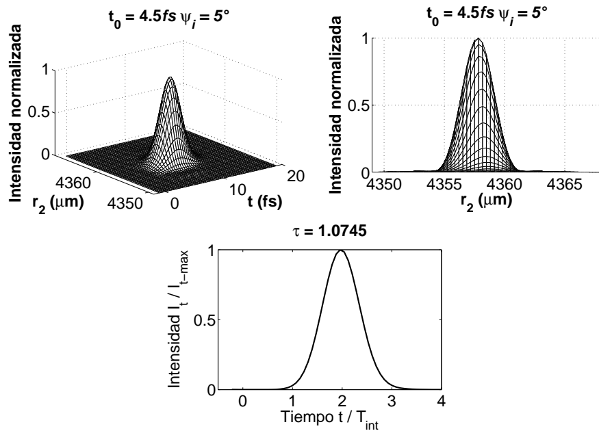
Figura 2.47: Duración inicial \tau_0 = 4.5\text{fs} , \psi_i = 5^\circ , iluminación uniforme.
