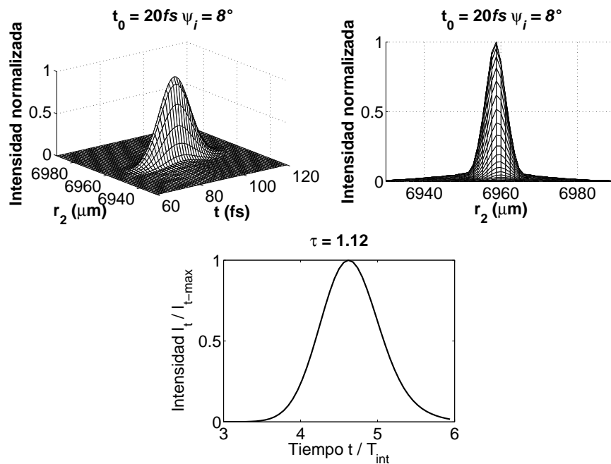
Figura 3.79: \tau_0 = 20\text{fs} , \psi_i = 8^\circ , Iluminación Gaussiana, k = k_0 , aberración esférica
