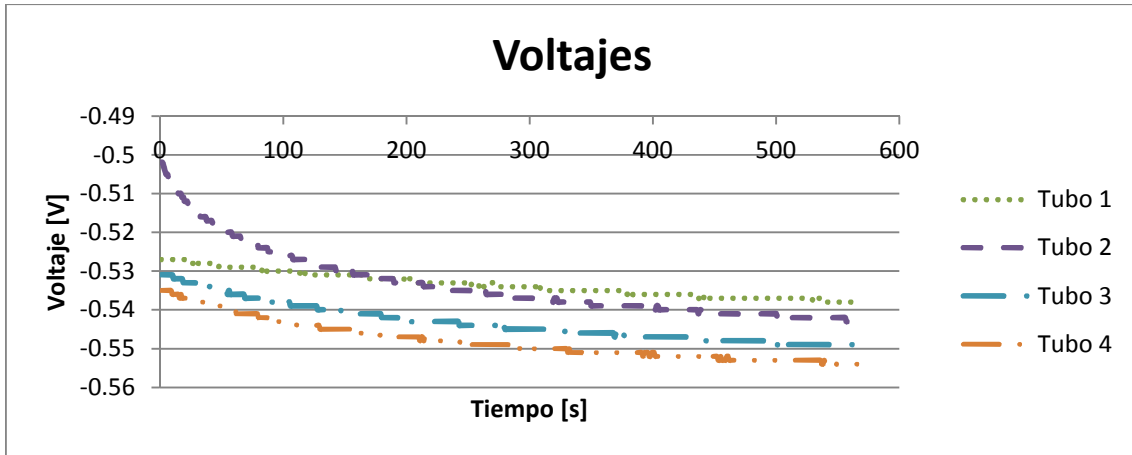
Gráfica 3.2 Potencial vs tiempo. Primer día de prueba.
