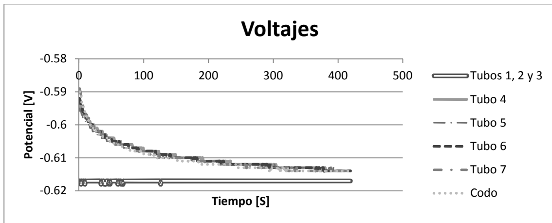
Gráfica 3.10 Potencial vs tiempo. Disolución en tubos 1, 2 y 3 durante 24 horas.
