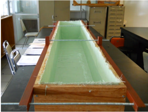
Fig. 2.3 vista final de la celda en picada.
