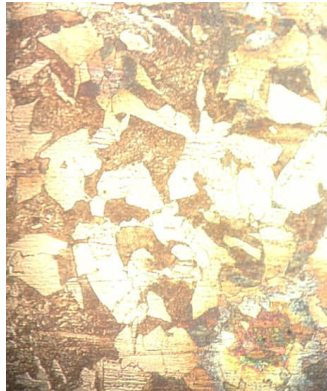
Fig. 3.1 Micrografía de la microestructura de la muestra testigo a 1000x.
