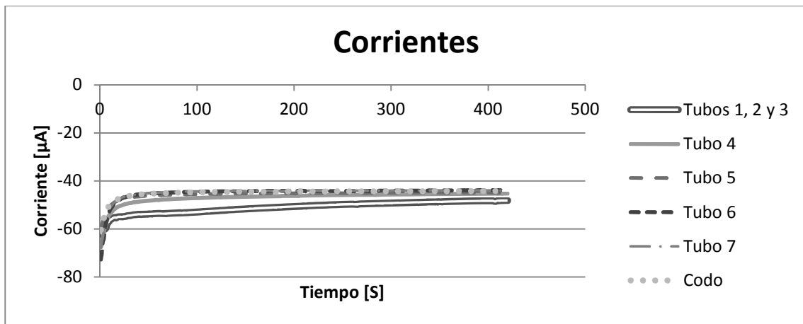
Gráfica 3.9 Corriente vs tiempo. Disolución en tubos 1, 2 y 3 durante 24 horas.
