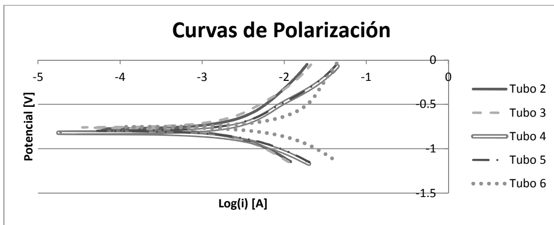
Figura 1.3 Representación de diferentes curvas de polarización anódicas y catódicas.
