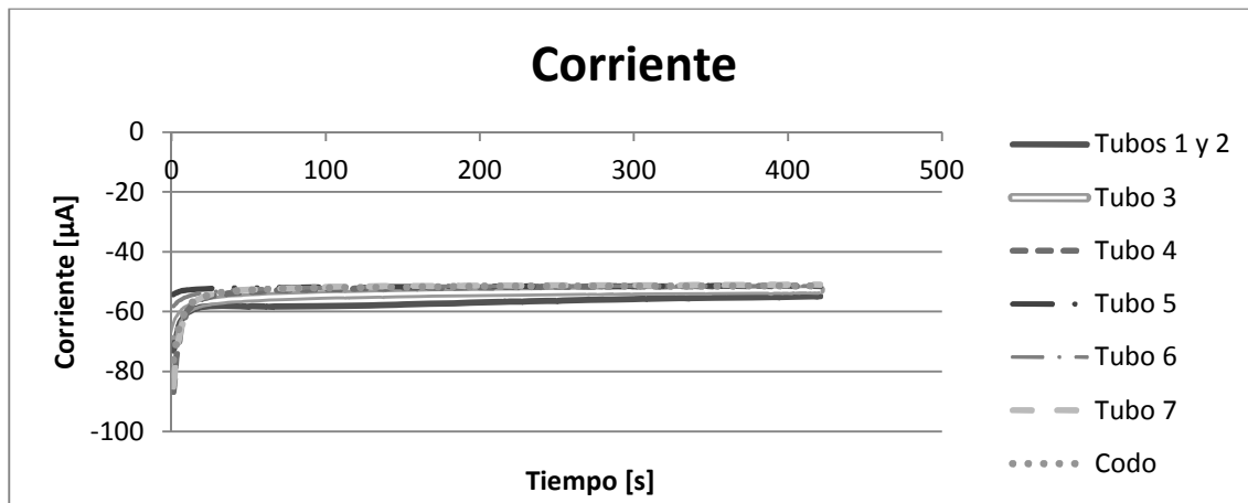
Gráfica 3.7 Corriente vs tiempo. Disolución en tubos 1 y 2 durante 48 horas.
