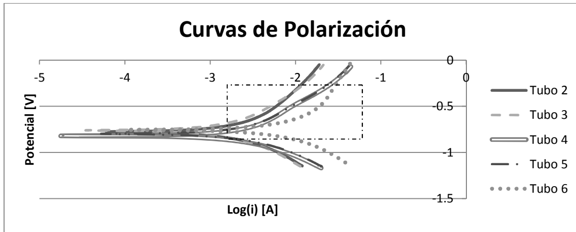
Gráfica 3.33 Curvas de polarización en el medio húmedo.
