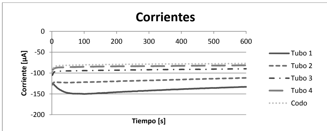
Gráfica 3.5 Corriente vs tiempo. Solución en Tubo 1 durante 48 horas.
