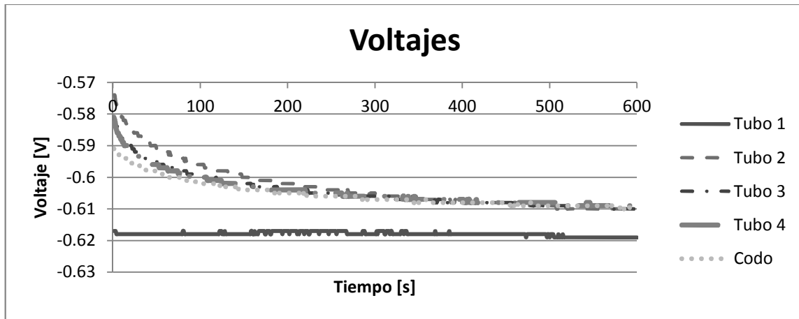
Gráfica 3.6 Potencial vs tiempo. Solución en Tubo 1 durante 48 horas.
