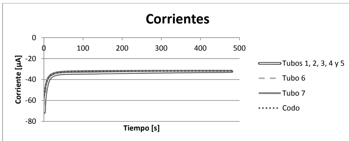
Gráfica 3.13 Corriente vs tiempo. Disolución en tubos 1, 2, 3, 4 y 5 durante 24 horas.
