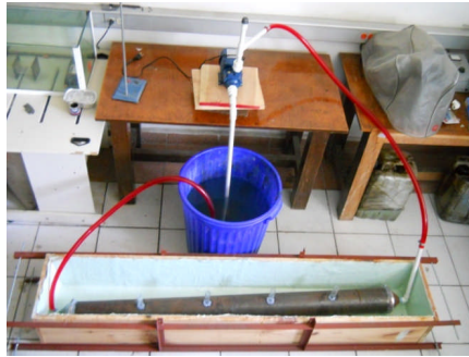
Fig. 2.9 Vista final del sistema de bombeo de flujo constante.
