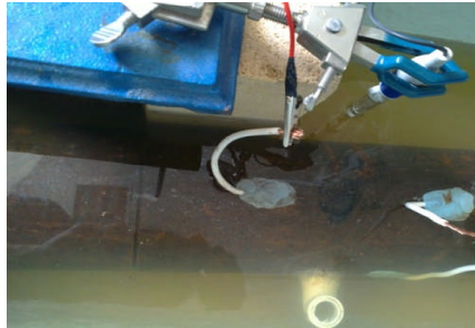
Fig. 2.13 Medición de ruido electroquímico en el primer punto.
