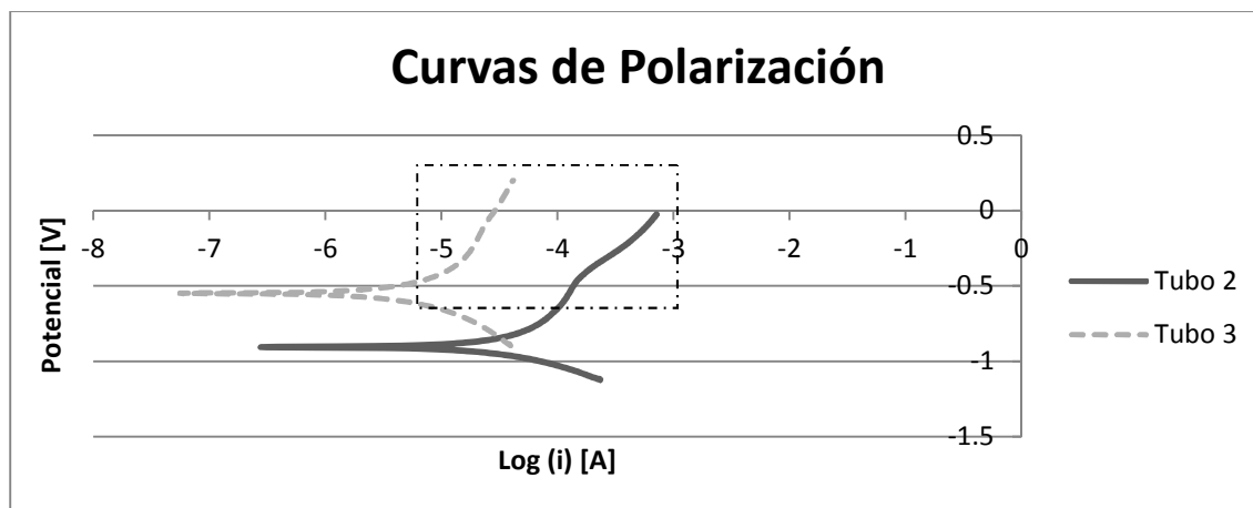
Gráfica 3.32 Curvas de polarización en el medio seco.
