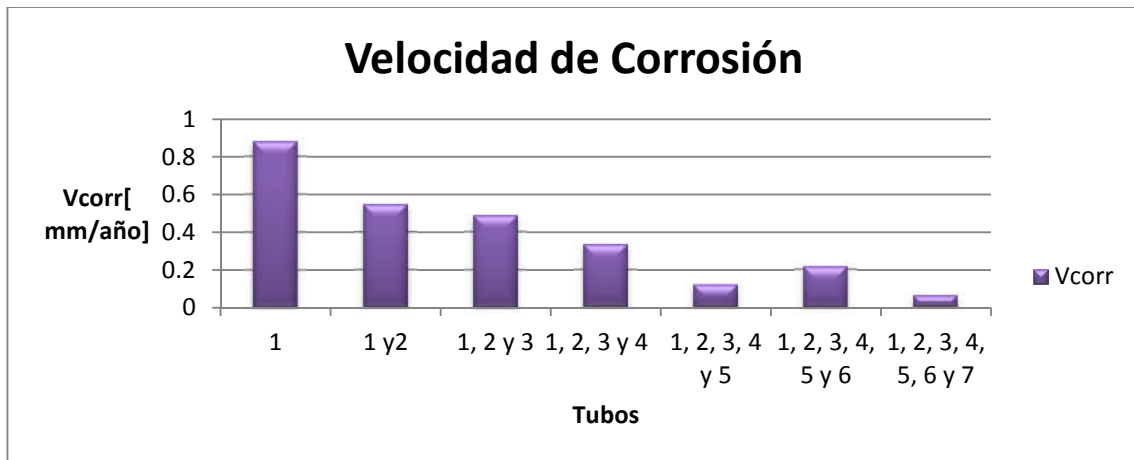
Gráfica 3.19 Velocidad de corrosión perteneciente a los tubos en donde se dejó reposar la solución de cloruro de sodio.
