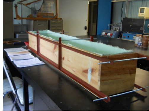
Fig. 2.4 Vista final lateral de la celda.
