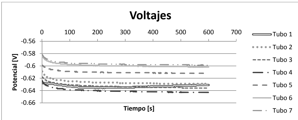
Gráfica 3.23 Potencial vs tiempo. 5 días de inmersión.
