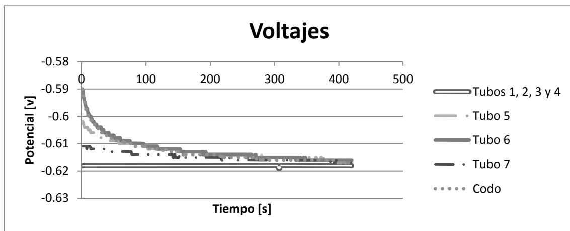
Gráfica 3.12 Potencial vs tiempo. Disolución en tubos 1, 2, 3 y 4 durante 120 horas.
