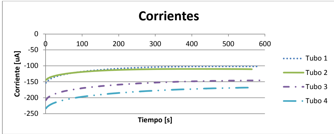
Gráfica 3.3 Corriente vs tiempo. Segundo día de experimentación.
