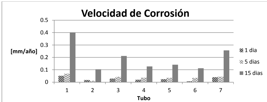
Gráfica 3.26 Velocidad de corrosión en el primer día, quinto día y después de 15 días de la inmersión del tubo.
