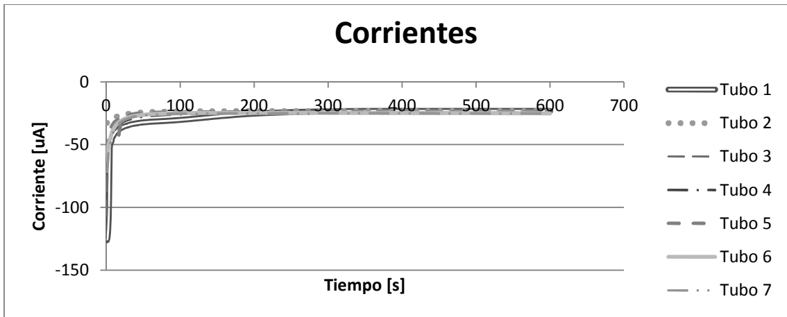
Gráfica 3.22 Corriente vs tiempo. 5 días de inmersión.
