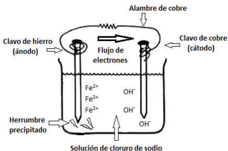
Figura 1.1 Celda galvánica compuesta por un clavo de hierro (ánodo), un clavo de cobre (cátodo) y cloruro de sodio como electrolito.
