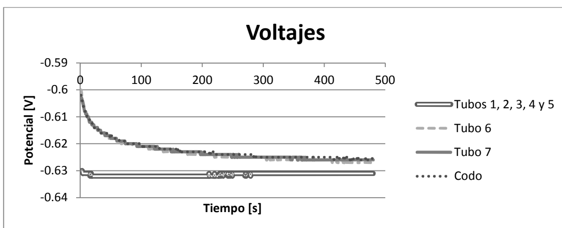
Gráfica 3.14 Potencial vs tiempo. Disolución en tubos 1, 2, 3, 4 y 5 durante 24 horas.
