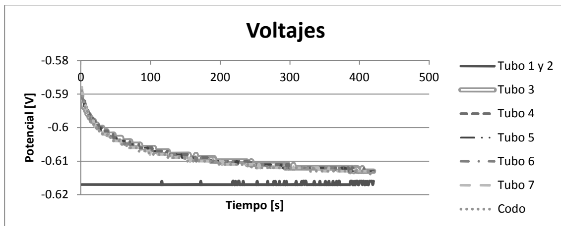
Gráfica 3.8 Potencial vs tiempo. Disolución en tubos 1 y 2 durante 48 horas.
