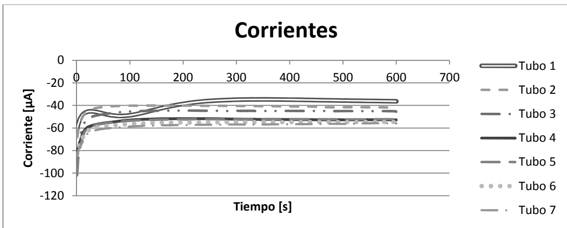
Gráfica 3.24 Corriente vs tiempo. 15 días de inmersión.
