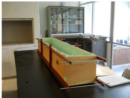
Fig. 2.2 Cajón reforzado por medio de una estructura metálica.
