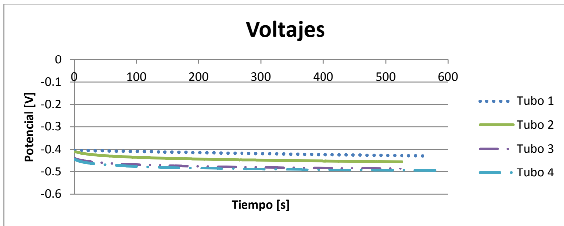
Gráfica 3.4 Potencial vs tiempo. Segundo día de experimentación.
