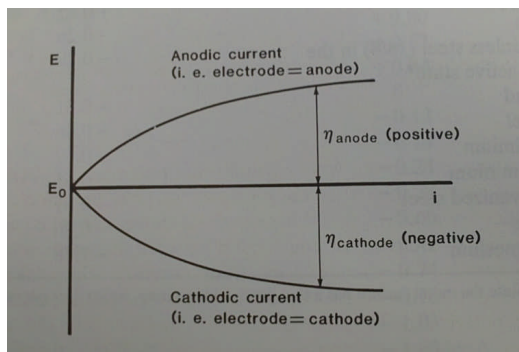
Figura 1.2 Curva de polarización anódicas y catódicas; E = potencial de electrodo, i = densidad de corriente y \eta = polarización. 43
