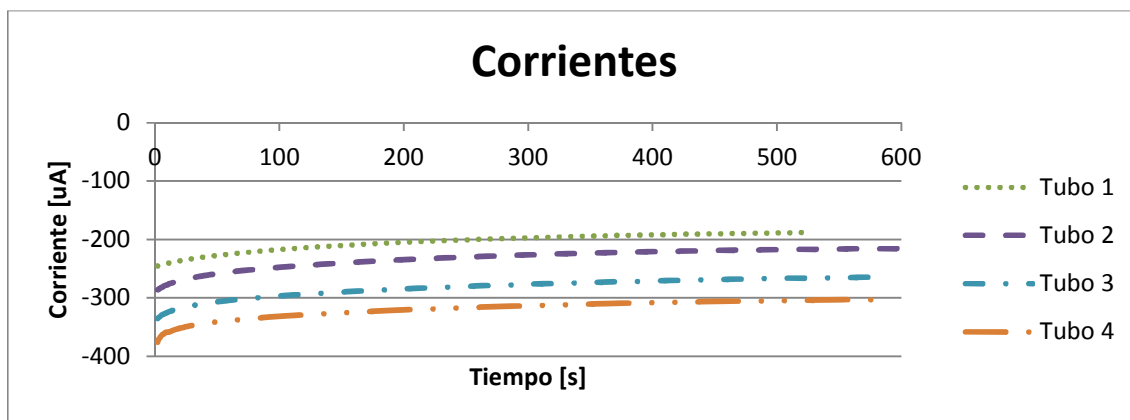
Gráfica 3.1 Corriente vs tiempo. Primer día de prueba.
