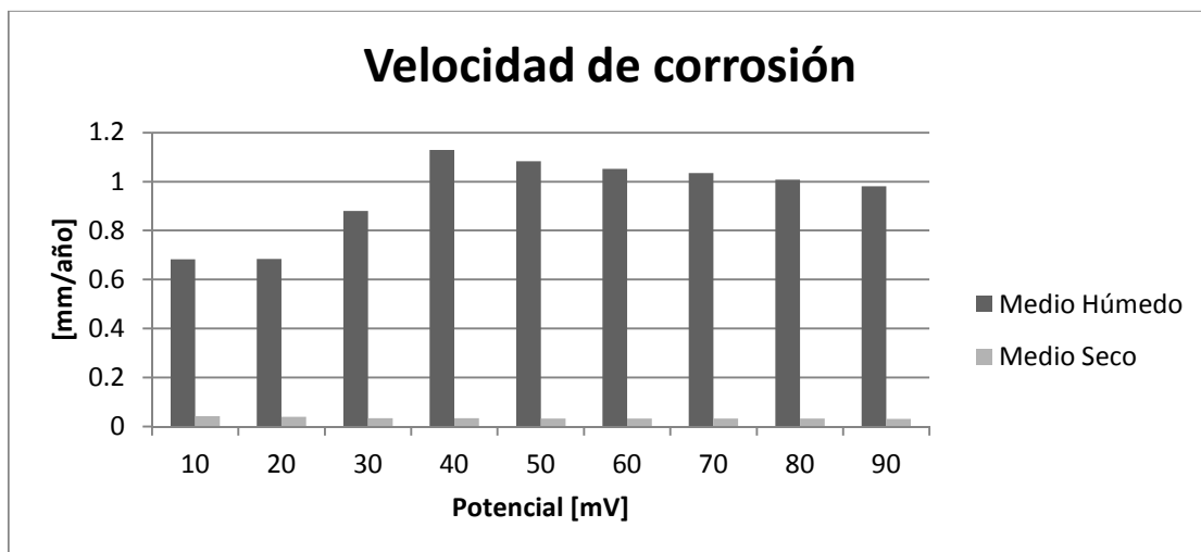
Gráfica 3.31 Velocidades de corrosión para los medio húmedo y seco, por medio de la técnica R_p .
