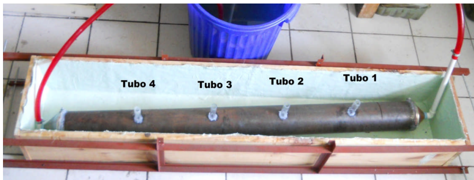
Fig. 3.3 Posición de los 4 tubos de acrílico.
