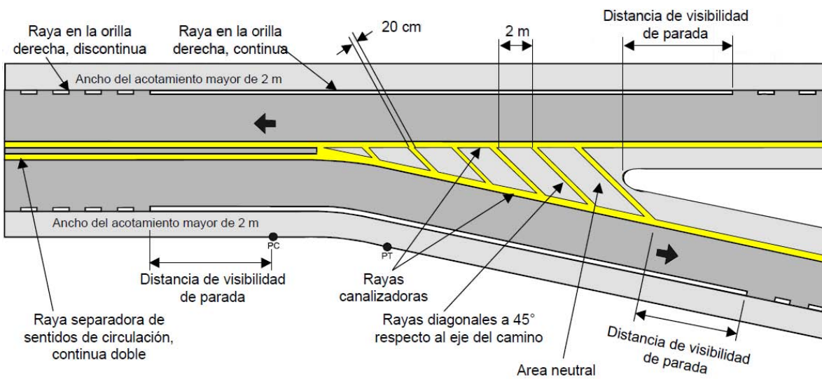
Figura 2.8 Rayas M-1, M-3, y M-5 en caminos con calzada mayor a 6.5 m.
