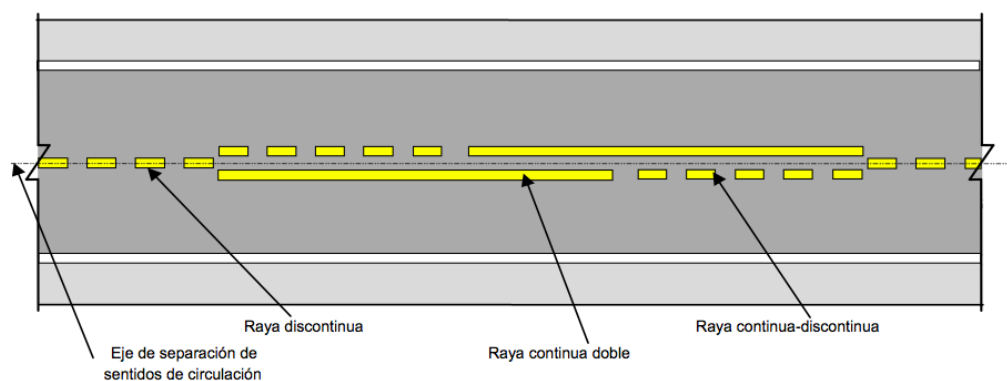
Figura 2.2 Rayas M-1 para caminos con calzada mayor a 6.5 m.
