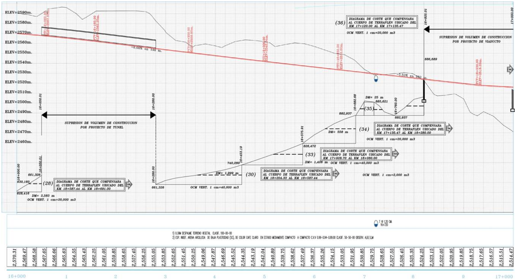
Figura 6.36 Alineamiento vertical del sub-tramo del km 16+000 al km 17+000.
