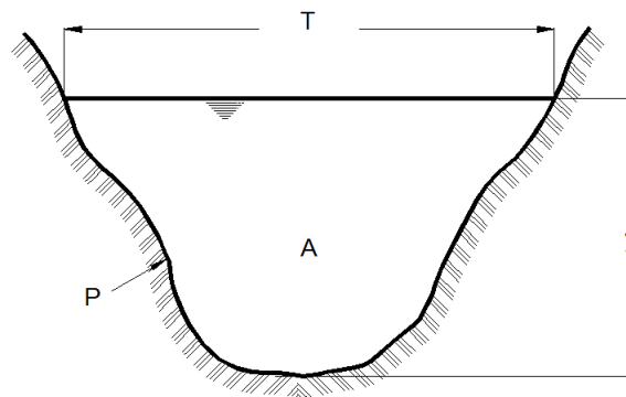
Figura 1.2 Elementos geométricos de un canal
