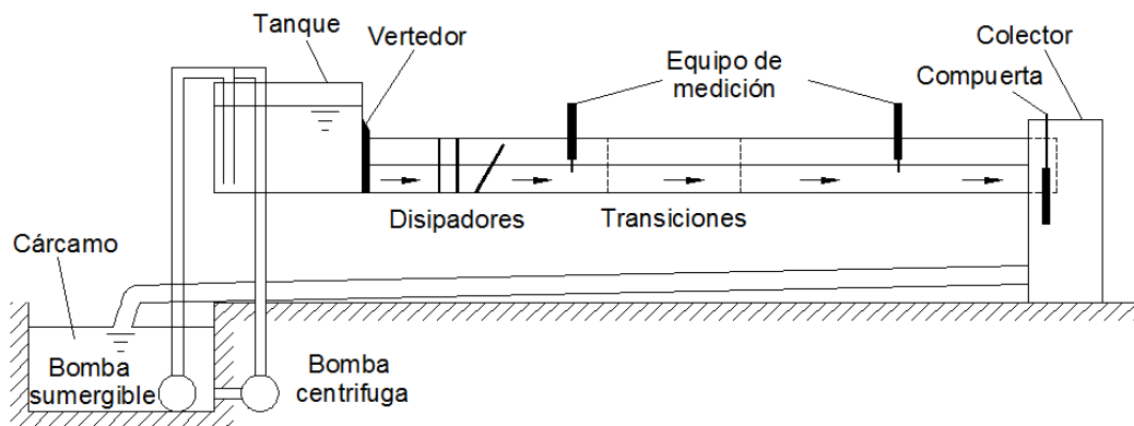
Figura 3.1 Canal de recirculación: a) dispositivo experimental, b) vista longitudinal del canal
