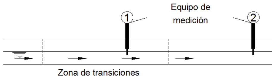
Figura 3.4 Posición de los equipos de medición para la expansión del canal
