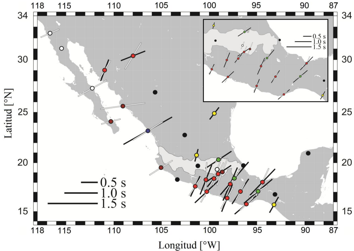
Figura 21. En la figura se muestran los resultados obtenidos para el sismo del 11/12/14 para todas las estaciones del SSN que se contaba con datos del evento. Las barras de color blanco indican las mediciones hechas con la fase SKS y las barras de color negro muestran los resultados medidos con la fase SKKS . La longitud de las barras es proporcional con el valor medido para \delta t . Con un círculo negro se presentan las estaciones donde se obtuvieron mediciones nulas con ambas fases. Con un círculo blanco se representan las estaciones en donde no se pudo obtener una medición con SKKS debido al ruido o a la cercanía de la estación al epicentro. Con un círculo café se muestran las estaciones donde se obtuvo una medición nula con la fase SKKS . Con un círculo rojo se indican las estaciones donde los valores medidos con SKS concuerdan con los de SKKS . En las estaciones con un círculo verde se midió un \delta t mas grande con la fase SKKS sin embargo no son los suficientemente diferentes que con los medidos con SKS . Con un círculo amarillo se muestran las estaciones que tuvieron el mismo comportamiento observado por Long [2008], con la diferencia de que los valores de \delta t medidos con SKKS no son tan grandes. Finalmente con un círculo azul se muestra la estación donde se obtuvieron resultados concordantes con Long [2008]. En el recuadro se muestra un acercamiento de la zona centro para su mejor apreciación
