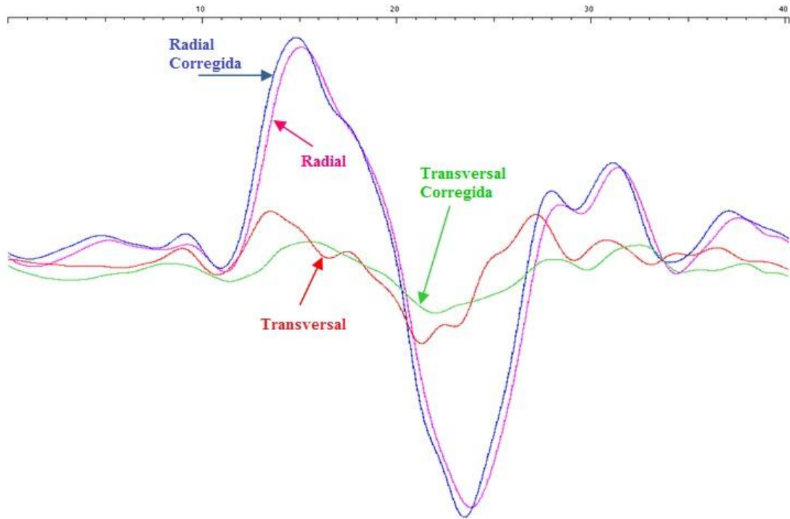
Figura 14. Formas de onda para la estación de Tlapa para el sismo del 25 de diciembre del 2010 de Vanuatu, se observan las componentes radial (rosa), radial corregida (azul), transversal (rojo) y transversal corregida (verde). Se puede apreciar como la amplitud de la onda radial corregida es mayor a la radial, la cual a su vez es mayor a la transversal y esta última a su vez es superior a la transversal corregida. Se puede ver que las cuatro componentes tienen formas de onda similares entre sí.
