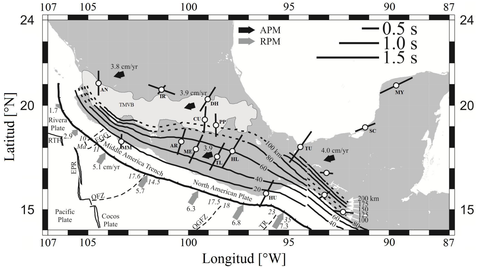
Figura 16. Mediciones apiladas de \phi y \delta t para las estaciones del SSN ubicadas en la zona centro del país y en la península de Yucatán. El tamaño de las barras es proporcional con el valor obtenido para el \delta t , según la escala mostrada y la inclinación de las barras representan el valor medido para \phi . El área sombreada en un tono más claro indica la región del Eje Volcánico Trans-Mexicano (TMVB por sus siglas en inglés). Las flechas negras indican la dirección del movimiento absoluto de la placa Norteamericana y las flechas grises demuestran la dirección del movimiento relativo entre las placas de Cocos y Norteamericana, cada una de las flechas cuenta con su respectiva velocidad 2 en cm por año. La línea con triángulos representa la trinchera mesoamericana y las líneas subparalelas a la trinchera ubicadas hacia el oeste de los 94° de longitud son las cotas de isopropundidad de la placa subducida tomadas de Pardo y Suárez, 1995 , las cotas situadas al este de los 94° se tomaron de Rodríguez-Pérez, 2007 .
