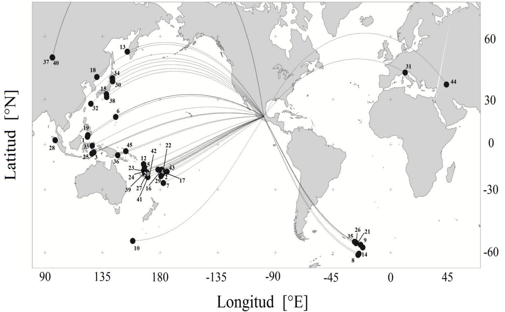
Figura 11. Mapa con las ubicaciones de los epicentros de los sismos empleados para la medición de los parámetros de anisotropía. Se muestran las trayectorias seguidas por las ondas sísmicas desde el epicentro hacia la estación CUIG, con lo cual podemos estimar visualmente el back azimuth de los eventos. El numero mostrado esta referenciado a la tabla 1 de los parámetros de fuente de los eventos usados.
