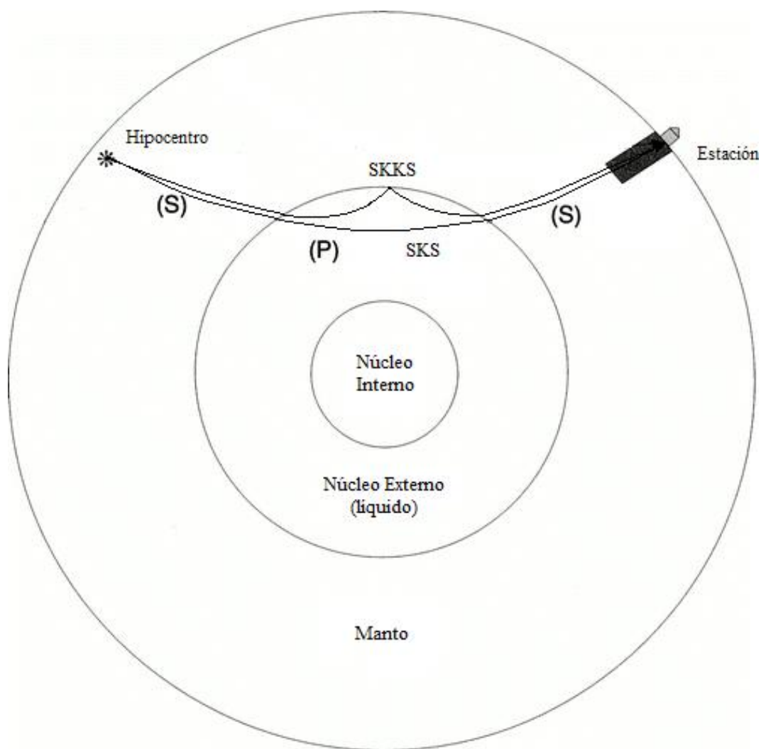
Figura 8. Esquema de las fases teleísticas SKS (se origina y viaja como S en el manto, se refracta en el CMB, sigue a través del núcleo externo como P vuelve a refractarse en el CMB y continúa su recorrido como S por el manto y la corteza hasta llegar a la estación) y SKKS (su trayectoria es muy similar a la de SKS , solo que una vez que ingresa al núcleo externo sufre una reflexión en el CMB). Figura modificada de Silver [1996].
