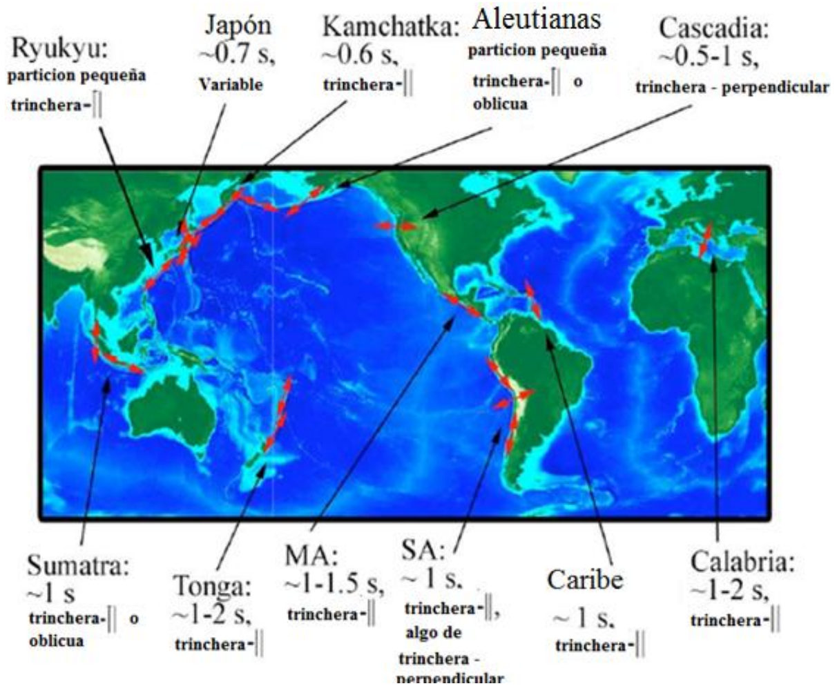
Figura 1. Muestra una recopilación de las mediciones de partición de onda de corte, realizadas en diversas zonas de subducción del mundo, las flechas en rojo indican el promedio de la dirección de polarización rápida. Del mismo modo se muestra el valor promedio de \delta t para cada una de las regiones que se ejemplifican. Figura modificada de Long y Silver , [2008].
