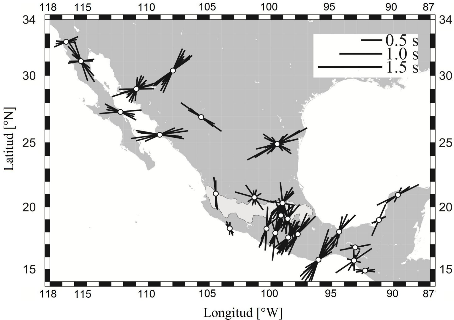
Figura A2.1. Mediciones individuales de \phi y \delta t para varias de las estaciones del SSN. El tamaño de las barras es proporcional con el valor obtenido para el \delta t , según la escala mostrada y la inclinación de las barras representa el valor medido para \phi . El área sombreada en un tono más claro indica la región del Eje Volcánico Trans-Mexicano (TMVB por sus siglas en inglés)
