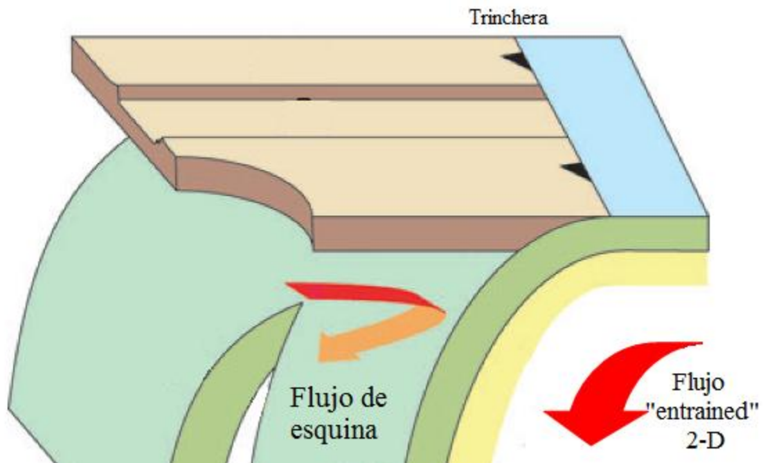
Figura 3. Muestra como es la dirección del flujo de esquina y del flujo "entrained" 2-D para un sistema de subducción. Figura modificada de León Soto et al. [2009].
