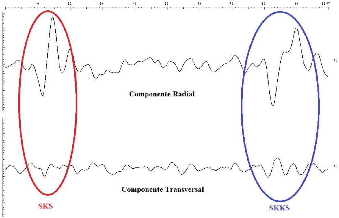
Figura 22. Formas de onda del sismo 11/12/14 de las componentes radial y transversal para la estación de LNIG. En color rojo se resalta la fase SKS y en azul la fase SKKS . Se observa que la fase SKKS sobresale del nivel de ruido, mientras que la fase SKS se pierde dentro del ruido.
