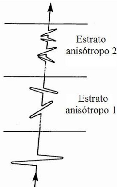
Figura 31. Esquema de la partición de onda para el caso de dos estratos anisótropos. La onda de corte entrante se divide dos veces dando como resultado cuatro ondas individuales. Figura modificada de Özalaybey y Savage , 1993.
