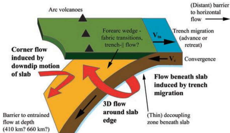
Figura 25. Modelo que ejemplifica los dos tipos de flujo que pueden existir en una zona de subducción. El flujo de esquina está dominado por la velocidad de subducción de la placa mientras que el flujo 3D está controlado principalmente por la velocidad de la migración de la trinchera. Figura tomada de Long [2009]
