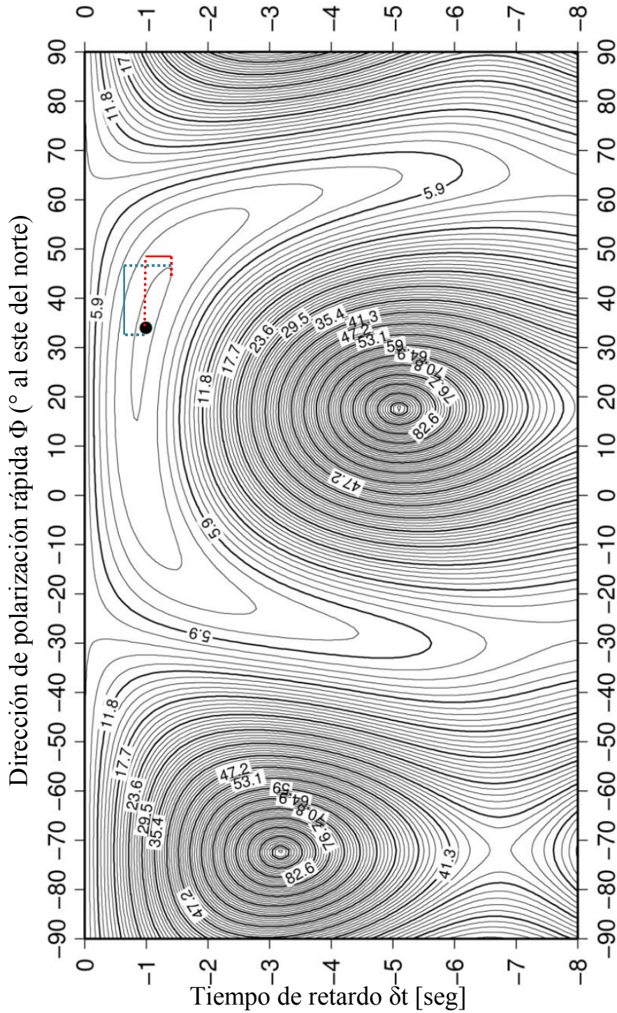
Figura 12. La gráfica muestra el valor mínimo característico en el espacio de (\varphi, \delta t) , el área que encierra la primer curva alrededor de la solución obtenida (punto negro) es el intervalo de confianza al 95%. El segmento continuo de línea en color rojo representa el valor medido de \sigma_{\delta t} , así como el segmento continuo de línea azul equivale al valor medido de \sigma_{\varphi} . EL valor encontrado para (\varphi, \delta t) = (34^\circ, 0.99 \text{ s}) es para la estación de Tlapa para el sismo del 25 de diciembre del 2010 de Vanuatu.
