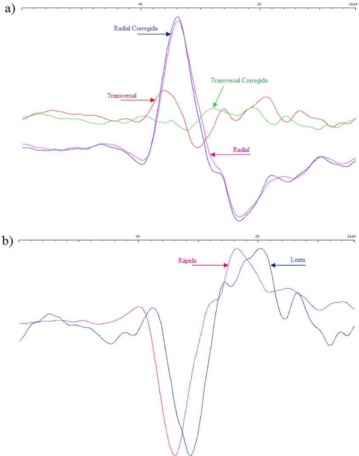
Figura 27. Formas de onda para la estación de LNIG para el sismo del 18 de febrero del 2010 con un back azimut de 325^\circ . Se puede apreciar que las correcciones con los valores de \phi = -54 y \delta t = 1.09 segundos son buenas ya que: a) Se observan las componentes radial (rosa), radial corregida (azul), transversal (rojo) y transversal corregida (verde) donde la amplitud de radial corregida es mayor que radial, mientras que la amplitud de transversal corregida disminuye con respecto de transversal. b) Podemos ver que la onda rápida (rosa) llega primero que la onda lenta (azul) y que ambas tienen forma de onda similar.
