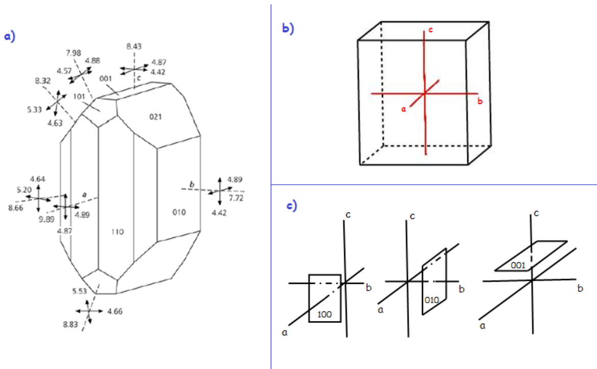
Figura 5. a) Se muestran las velocidades de las ondas P (líneas discontinuas) y S (pares perpendiculares en líneas solidas) en km/s para diferentes direcciones relativas a la estructura cristalina del olivino. El eje a , que es perpendicular al plano [100], es la dirección de velocidad más rápida a través del cristal, así como también es la dirección de deslizamiento dominante. La figura fue tomada del libro de Stein y Wysession [2003]. b) Se expone una de las posibles representaciones de los ejes cristalográficos de un cristal perteneciente al sistema ortorrómbico. Las longitudes de los ejes son todas diferentes y los ángulos formados entre si son iguales a 90°. c) Presenta los tres planos de simetría que posee un cristal del sistema ortorrómbico. El plano [100] es perpendicular al eje a , el plano [010] es perpendicular al eje b y el plano [001] es perpendicular al eje c .
