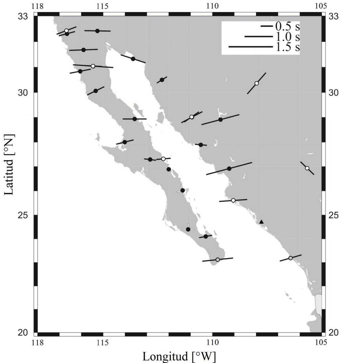
Figura 20. Recopilación de las mediciones realizadas en las estaciones del SSN y del arreglo NARS-Baja California. Con un círculo blanco se muestran las estaciones utilizadas para el presente trabajo con su respectiva medición. En círculo gris se presentan las estaciones del SSN en las que ya se contaba con mediciones 7 previamente. Con un círculo negro se enseñan las estaciones del arreglo NARS-Baja California con sus respectivas mediciones 8 . El tamaño de las barras es proporcional con el valor obtenido para el \delta t , según la escala mostrada y la inclinación de las barras representan el valor medido para \phi . Las mediciones nulas se muestran con dos barras blancas cruzadas a 90°. La estación NE83 se muestra con un triángulo negro, en esta estación no fue posible realizar mediciones. El área sombreada en un tono más claro indica la región del Eje Volcánico Trans-Mexicano (TMVB por sus siglas en inglés).
