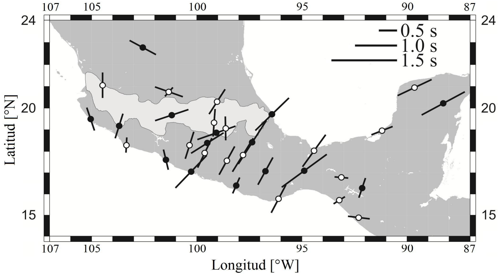
Figura 19. Recopilación de las mediciones realizadas en las estaciones del SSN. Con un círculo blanco se muestran las estaciones utilizadas para el presente trabajo con su respectiva medición. En círculo negro se presentan las estaciones del SSN en las que ya se contaba con mediciones 6 previamente. El tamaño de las barras es proporcional con el valor obtenido para el \delta t , según la escala mostrada y la inclinación de las barras representan el valor medido para \varphi . El área sombreada en un tono más claro indica la región del Eje Volcánico Trans-Mexicano (TMVB por sus siglas en inglés).
