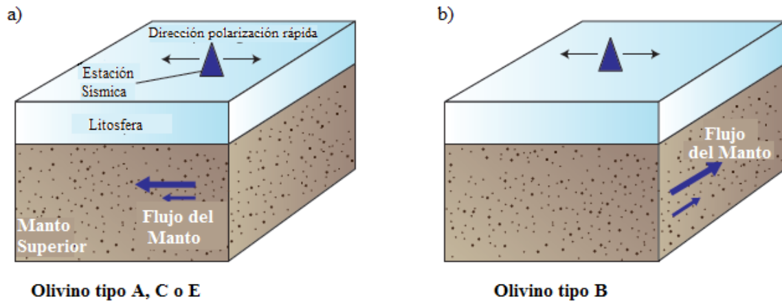
Figura 6. a) Se muestra que la relación entre la dirección del flujo del manto y la dirección de polarización rápida es subparalela entre sí para olivinos de tipo A, C y E. b) Se observa que la relación entre el flujo del manto y la dirección de polarización rápida es sub perpendicular entre sí para olivino tipo B. Figura modificada de Long , [2009]
