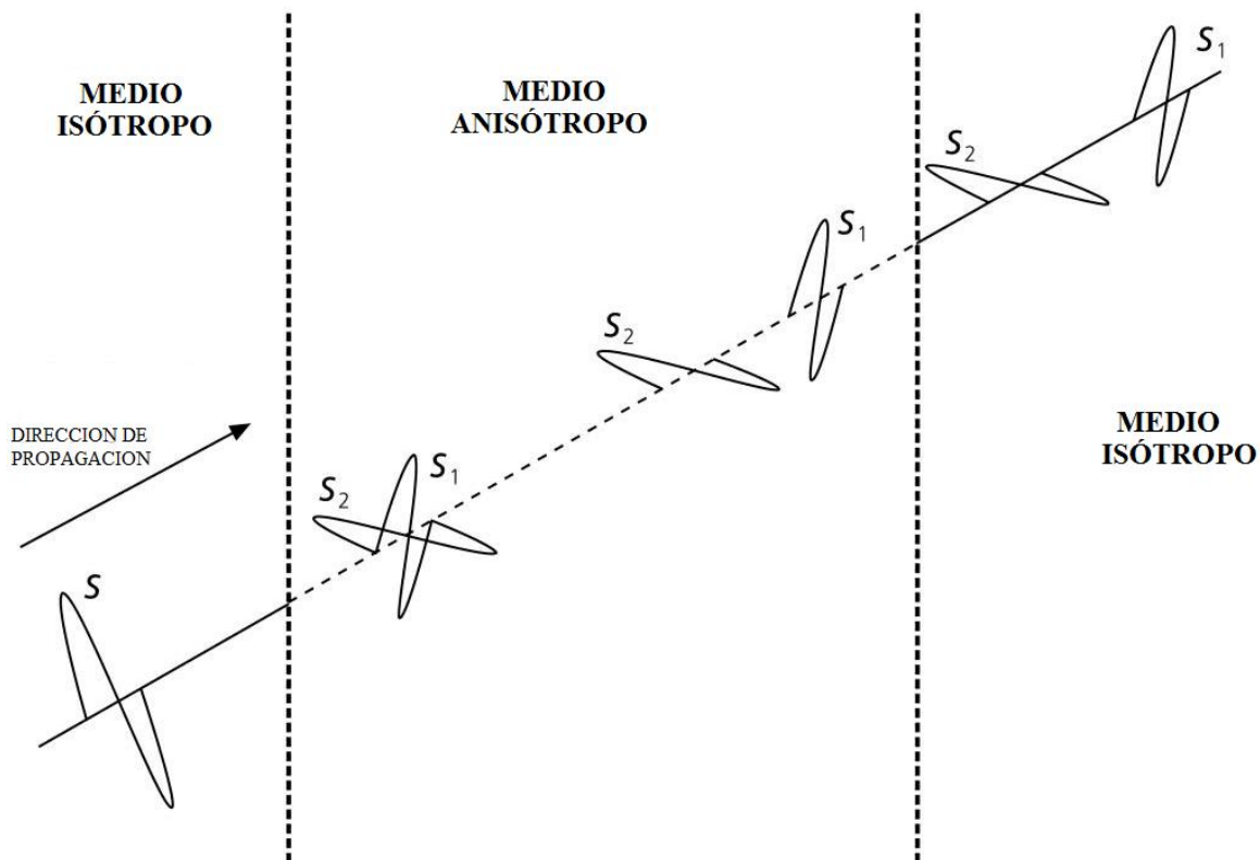
Figura 4. Esquema de una onda de corte con polarización radial. Al ingresar a un medio anisótropo es particionada a lo largo de las direcciones anisótropas rápida y lenta, originando una separación en tiempo. Al abandonar el medio anisótropo las ondas rápida y lenta no podrán reconstruir la onda original aun cuando vuelvan a ingresar a un medio isótropo. Figura modificada del libro de Stein y Wysession [2003].
