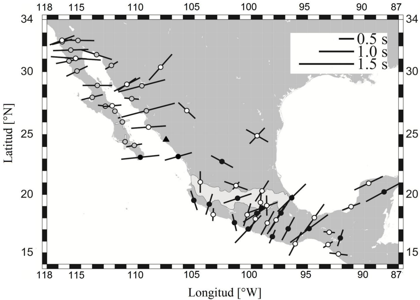
Figura 18. Recopilación de las mediciones realizadas en las estaciones del SSN y del arreglo NARS-Baja California. Con un círculo blanco se muestran las estaciones utilizadas para el presente trabajo con su respectiva medición. En círculo negro se presentan las estaciones del SSN en las que ya se contaba con mediciones 4 previamente. Con un círculo gris se enseñan las estaciones del arreglo NARS-Baja California con sus respectivas mediciones 5 . El tamaño de las barras es proporcional con el valor obtenido para el \delta t , según la escala mostrada y la inclinación de las barras representan el valor medido para \phi . Las mediciones nulas se muestran con dos barras blancas cruzadas a 90^\circ . La estación NE83 se muestra con un triángulo negro, en esta estación no fue posible realizar mediciones. El área sombreada en un tono más claro indica la región del Eje Volcánico Trans-Mexicano (TMVB por sus siglas en inglés).
