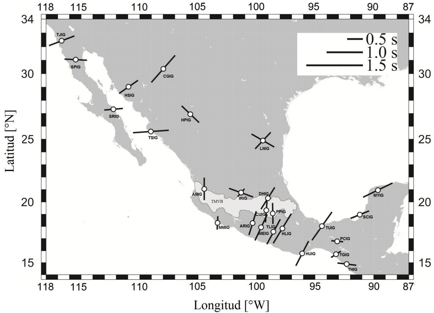
Figura 15. Mediciones apiladas de \phi y \delta t para varias de las estaciones del SSN. El tamaño de las barras es proporcional con el valor obtenido para el \delta t , según la escala mostrada y la inclinación de las barras representan el valor medido para \phi . El área sombreada en un tono más claro indica la región del Eje Volcánico Trans-Mexicano (TMVB por sus siglas en inglés).
