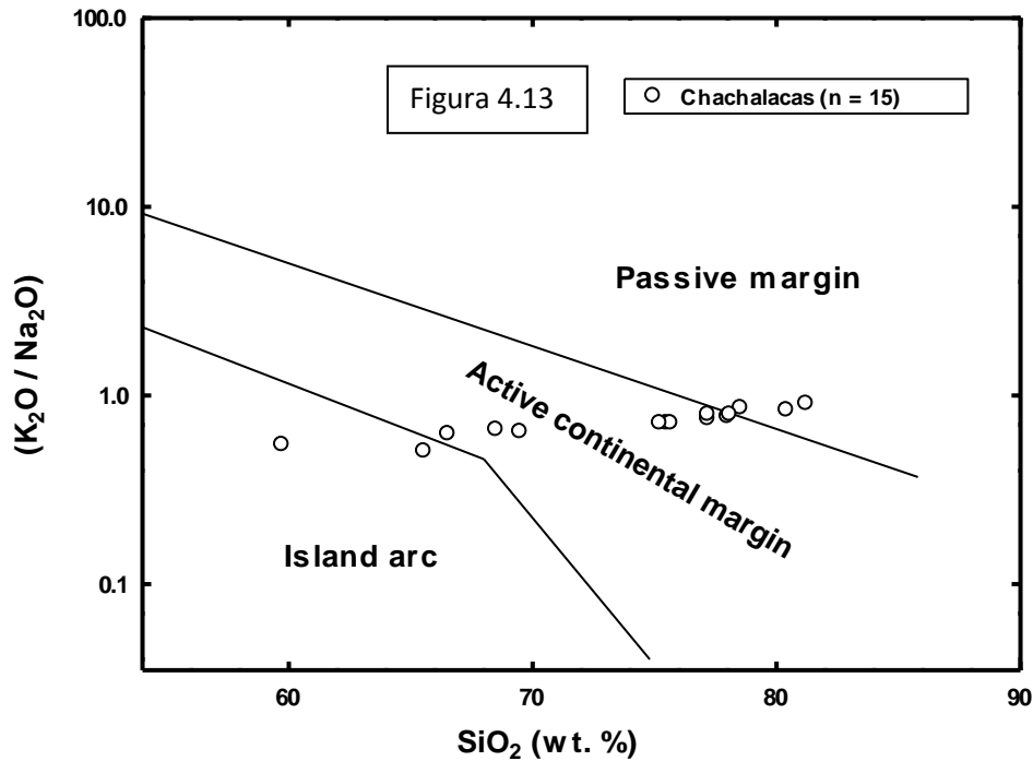
Figura 4.13. Diagrama de discriminación tectónica según (Roser and Korsch, 1986).
