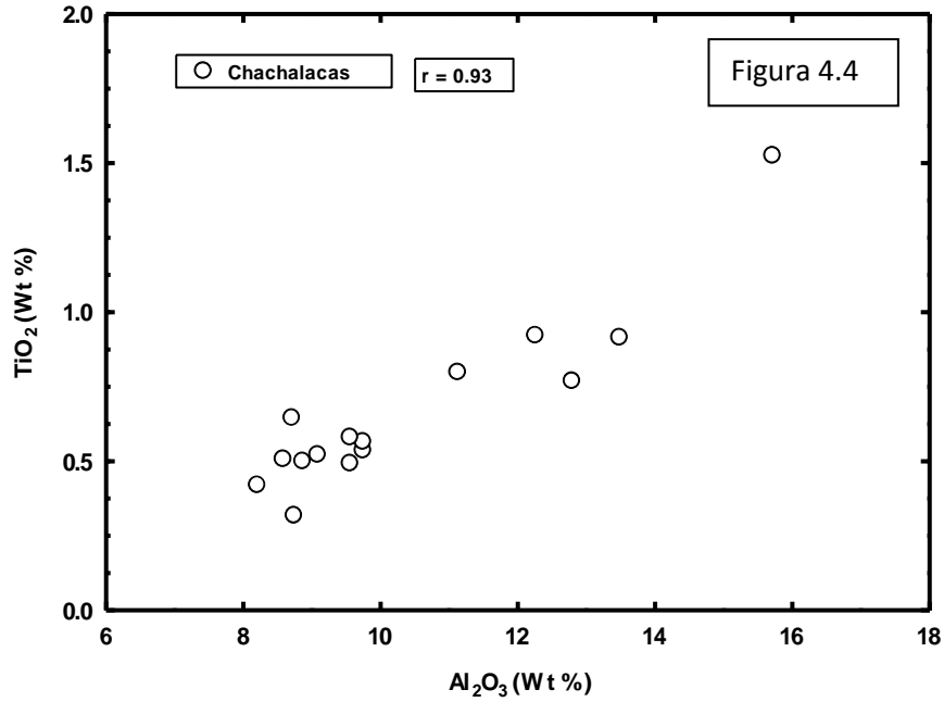
Figura 4.4. Diagrama de \text{Al}_2\text{O}_3 contra \text{TiO}_2 , donde se muestra el enriquecimiento de \text{TiO}_2 en algunas muestras.
