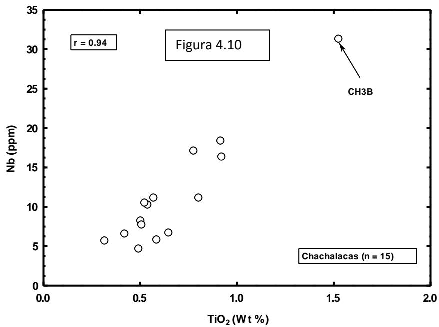
Figura 4.10. Diagrama de Nb contra \text{TiO}_2 , donde se muestra la buena correlación positiva ( r = 0.95 ).
