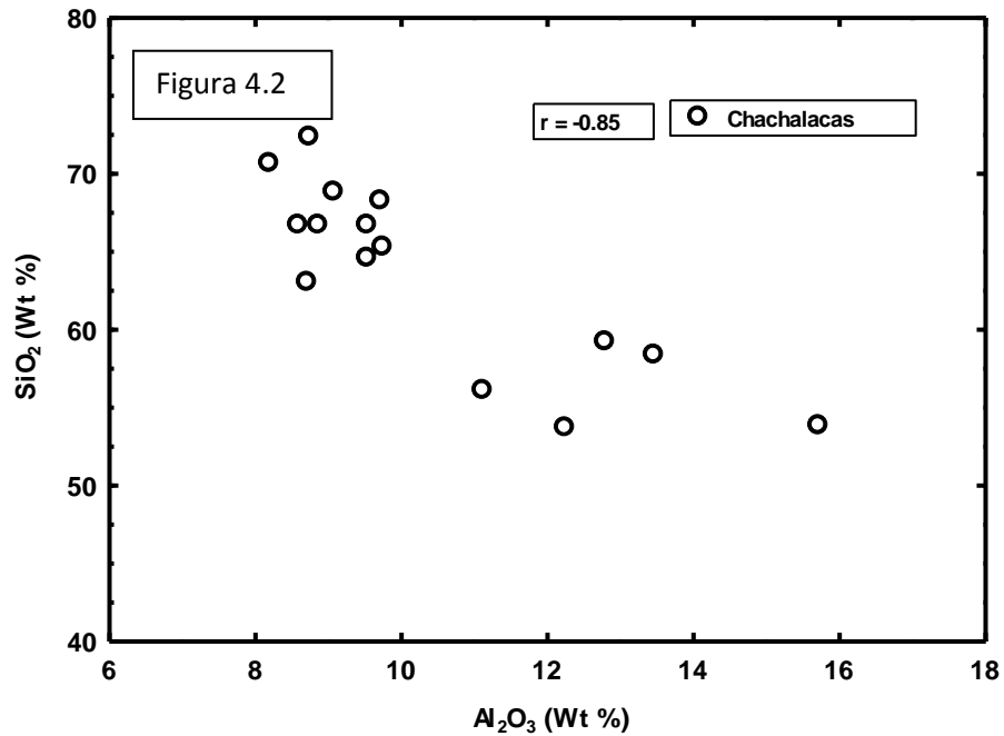
Figura 4.2. Diagrama bivalente de \text{SiO}_2 contra \text{Al}_2\text{O}_3 para las arenas de playa.
