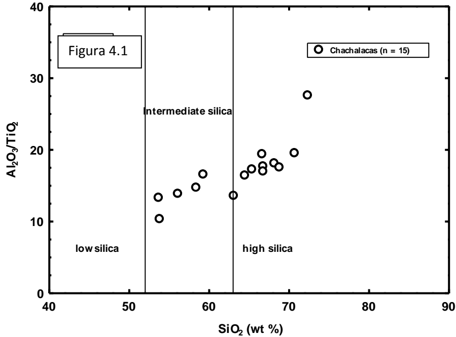
Figura 4.1. La relación Al_2O_3/TiO_2 vs SiO_2 , para las arenas de playa (Le Bas et al., 1986).
