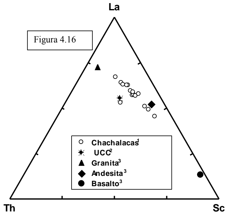
Figura 4.16. Diagrama triangular La-Th-Sc para muestras de arena estudiadas (McLennan, 2001), y Condie (1993).
