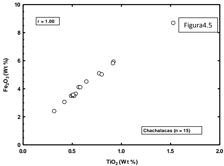
Figura 4.5. Diagrama de \text{TiO}_2 - \text{Fe}_2\text{O}_3 donde se muestra la excelente correlación positiva ( r = 1.00 ) para las arenas de Chachalacas.
