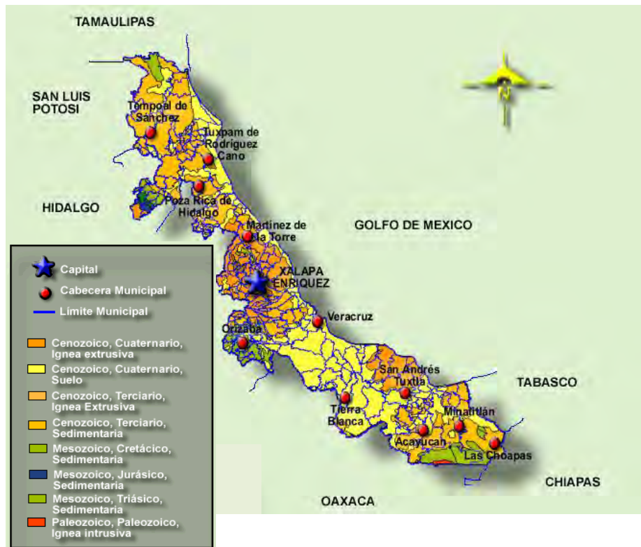
Figura 2.2 Geología del estado de Veracruz
