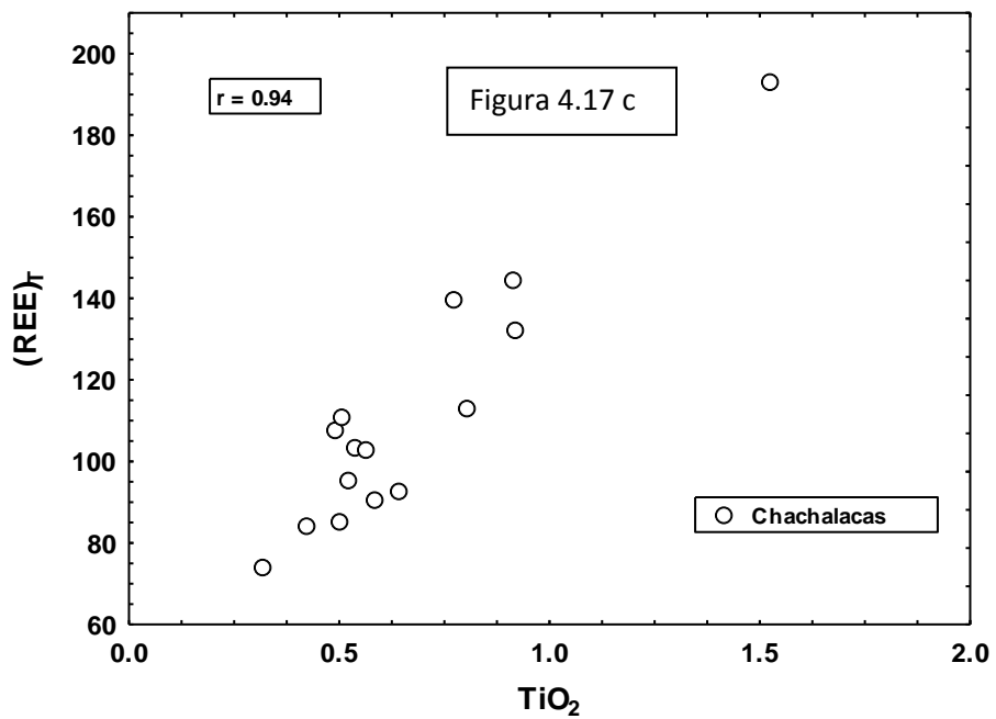
Figura 4.17a, 4.17b y 4.17c. Diagrama bivariantes de las arenas estudiadas. a) Fe 2 O 3 contra ΣREE b) Zr contra ΣREE c) TiO 2 contra ΣREE.
