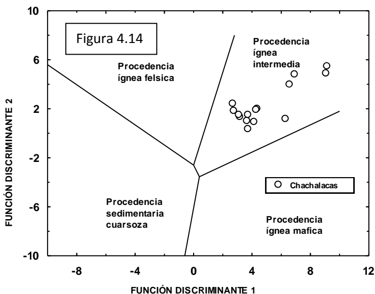
Figura 4.14. Diagrama de función discriminante para procedencia de sedimentos usando elementos mayores (Roser and Korsch, 1988).
