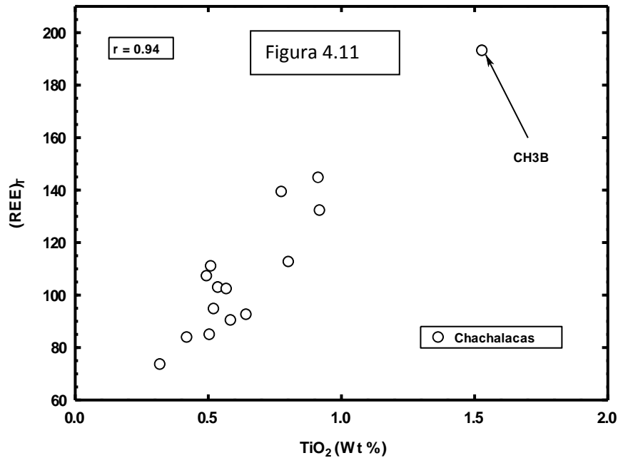
Figura 4.11. Diagrama de \text{TiO}_2 contra \Sigma\text{REE} de las arenas de playa estudiadas. La correlación positiva ( r = 0.94 ) indica que la distribución de las tierras raras esta controlada por minerales con contenido de \text{TiO}_2 .
