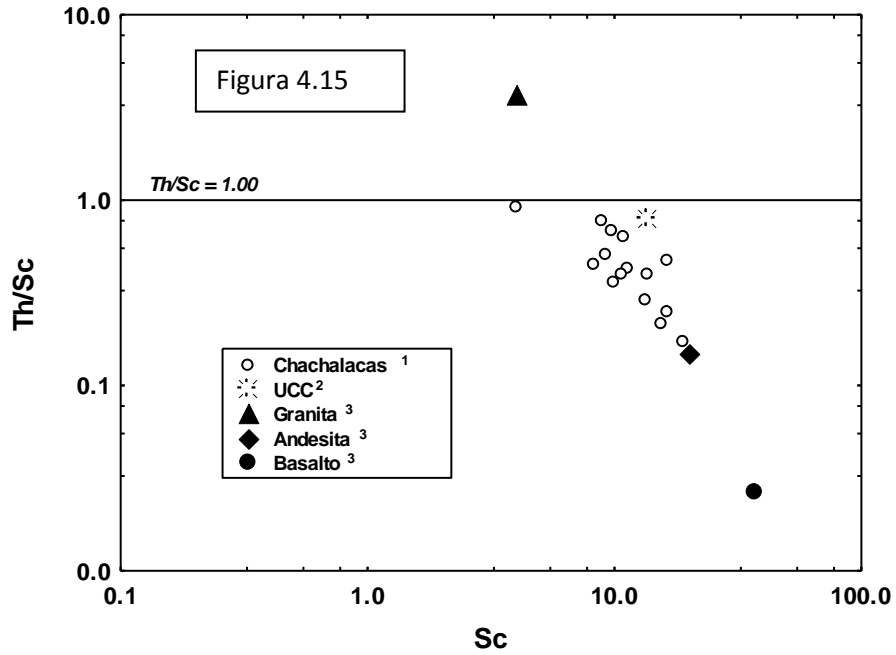
Figura 4.15. Diagrama bivalente Th/Sc contra Sc para muestras de arena (UCC; McLennan, 2001), y Condie (1993).
