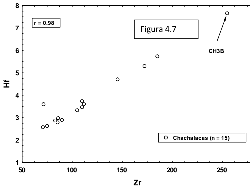
Figura 4.7. Diagrama bivalente que muestra la relación entre Zr y Hf.
