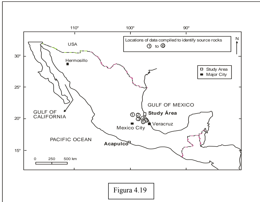
Figura 4.19. Áreas de fuente de donde fueron compilados los datos geoquímicos en este estudio para identificar la probable roca generadora.
