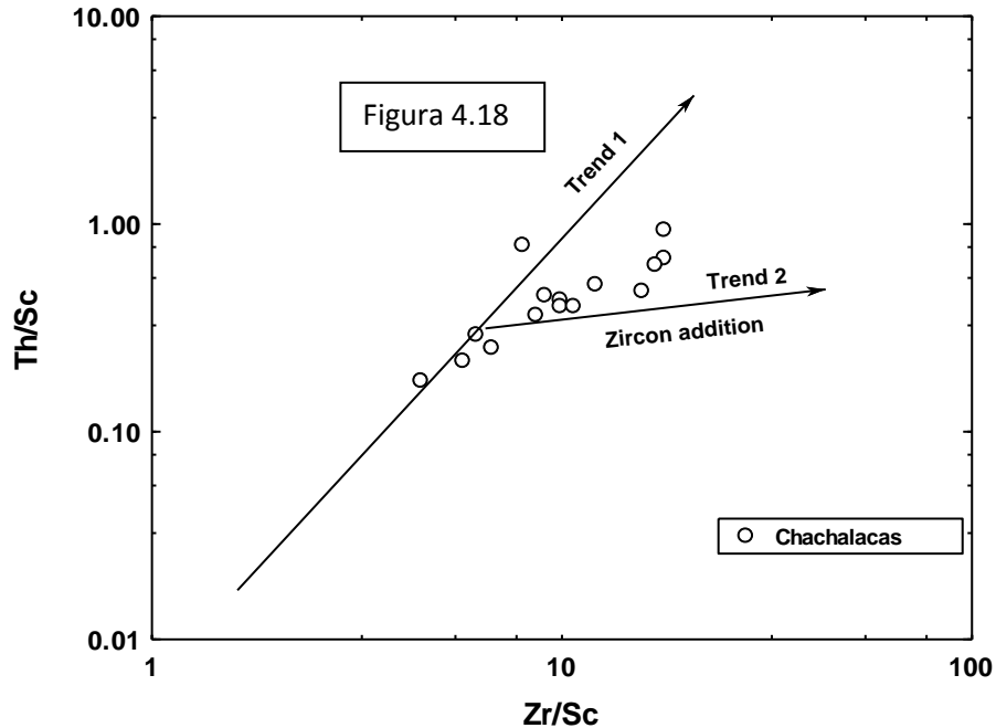
Figura 4.18. Diagrama bivariante de Th/Sc contra Zr/Sc m (McLennan et al., 1993). La adición de zircon en el sedimento es observada en la tendencia 2.
