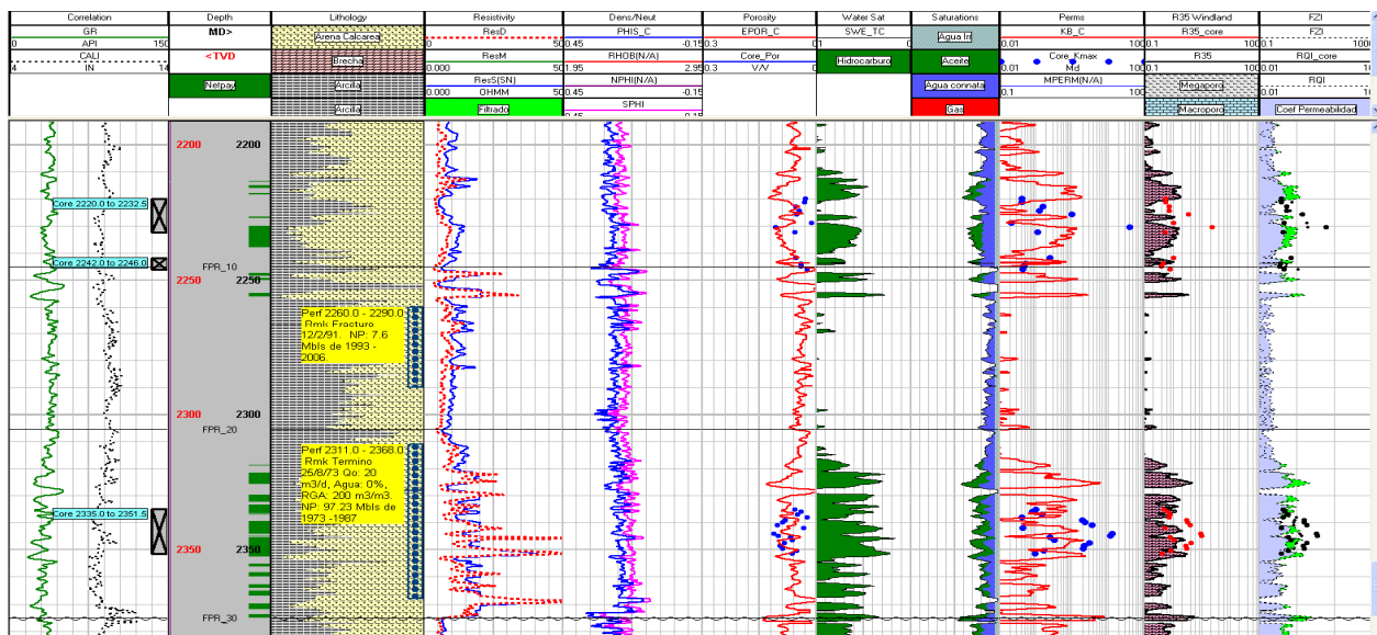
Figura 3.5 Pozo PA 202 (Con Datos de Núcleo)
