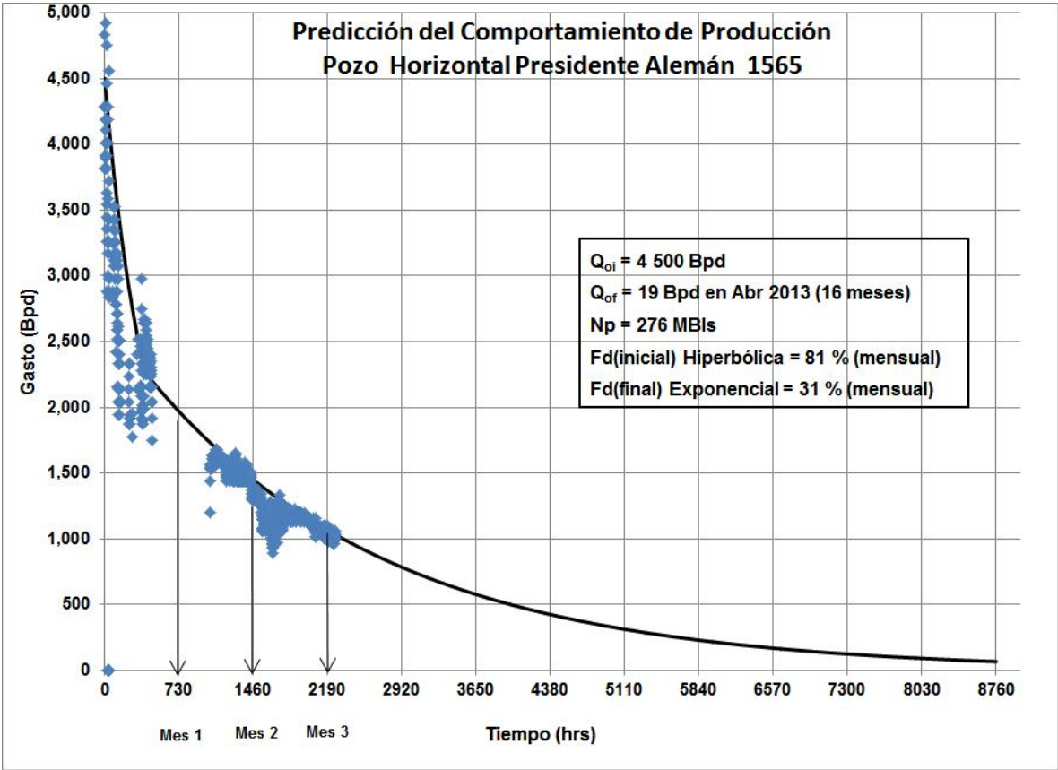
Figura 6.13 Comportamiento de producción PA-1565
