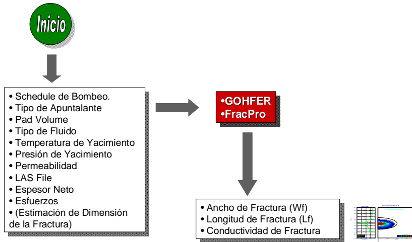
Figura 4.2 Flujo de Trabajo para Estimar Dimensión de la Fractura
