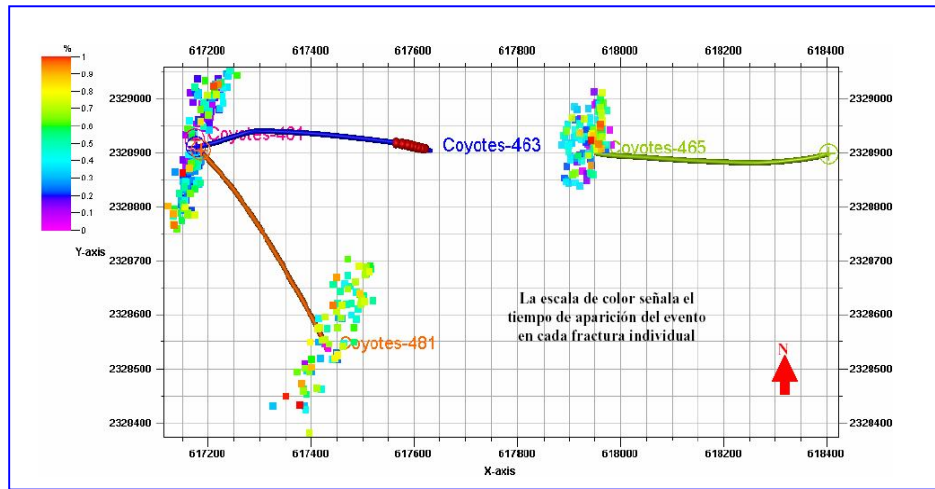
Figura 4.13 Microsísmica tomada en el campo Coyotes
