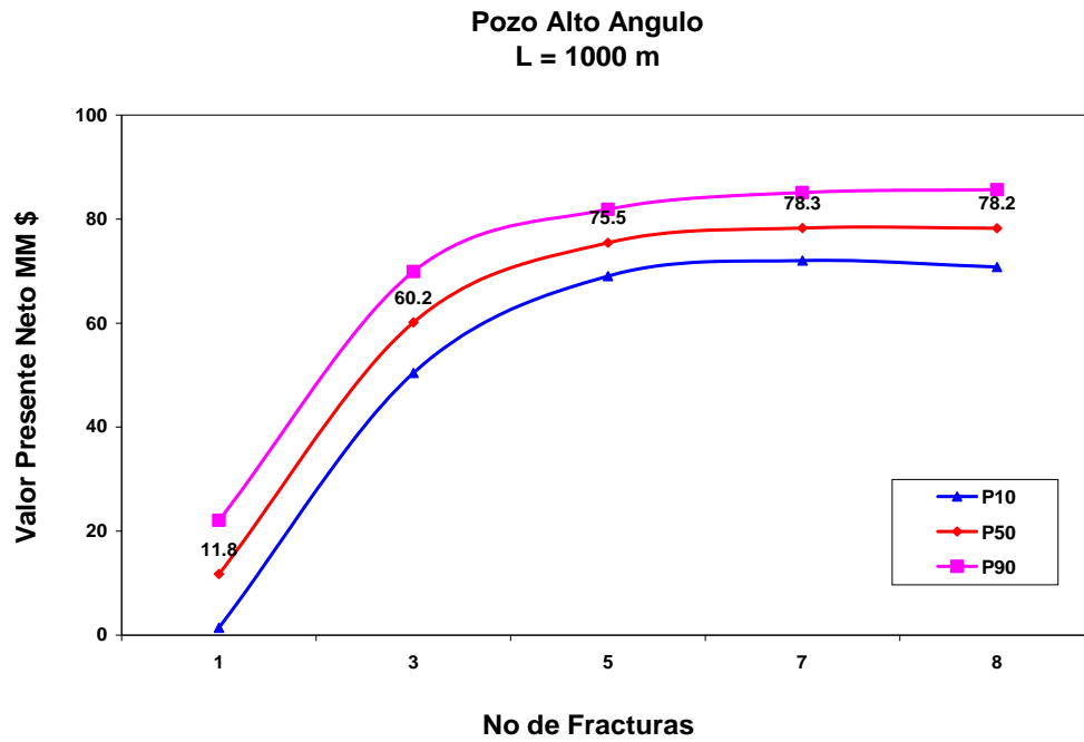
Figura 4.18 Valor presente neto vs número de fracturas
