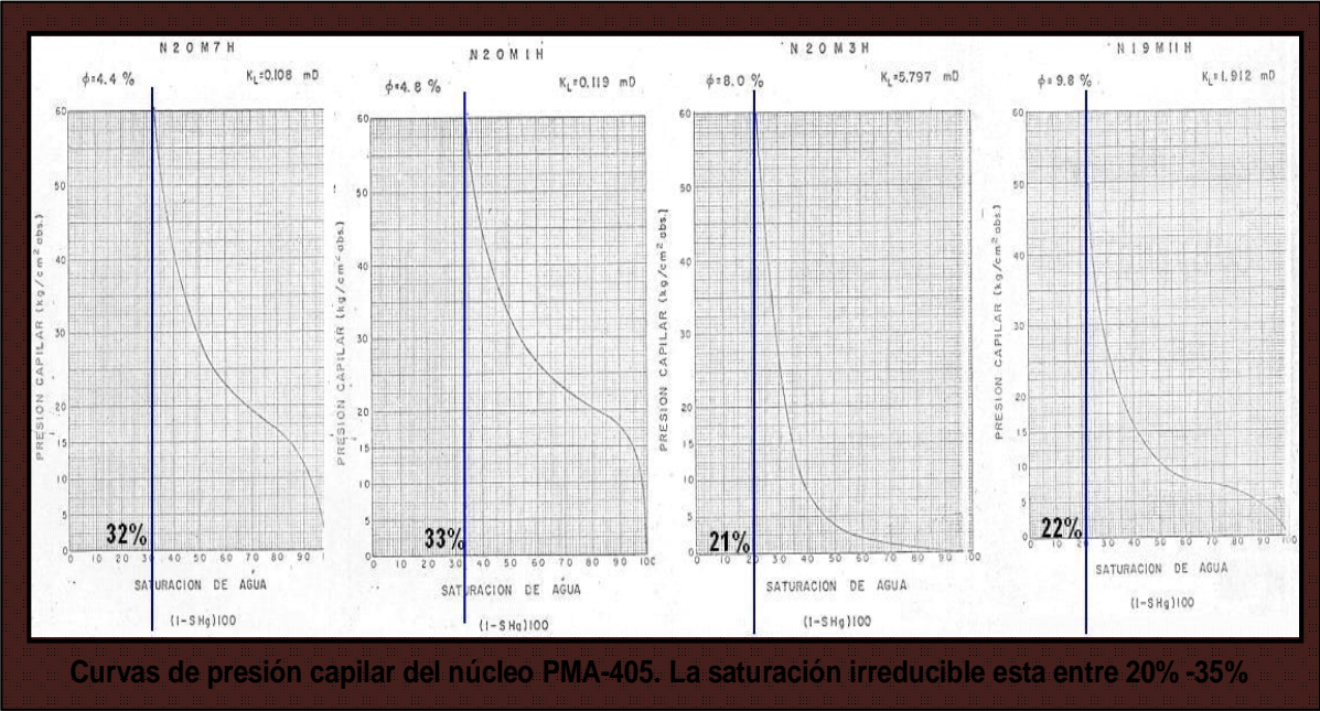
Figura 3.7 Curvas de presión capilar
