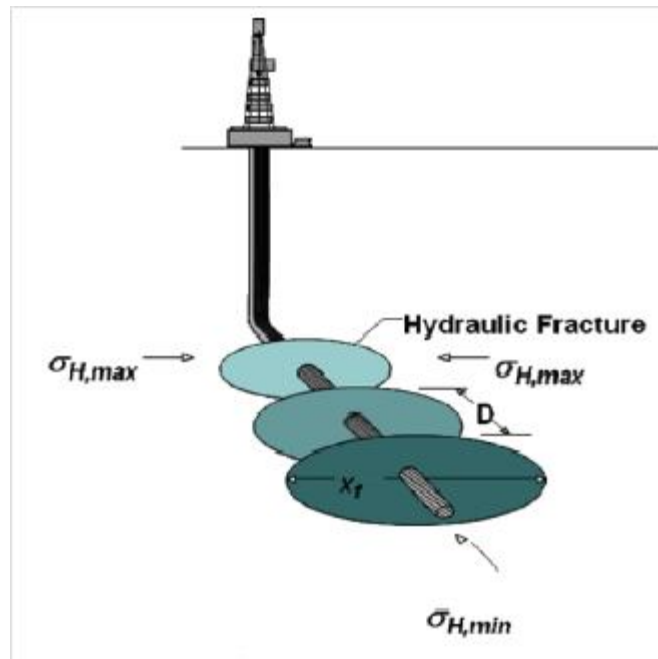
Figura 4.11 Pozo horizontal fracturado
