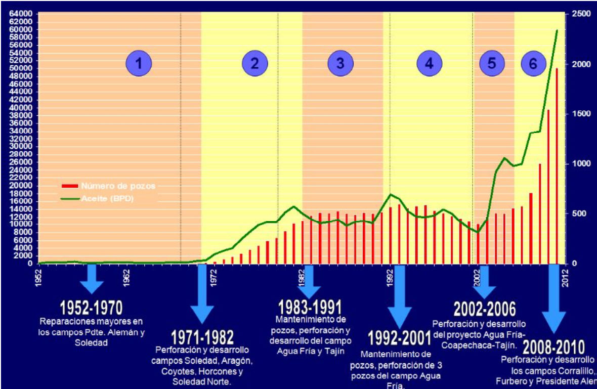
Figura 1.1 Comportamiento histórico de producción del Paleocanal Chicontepec.
