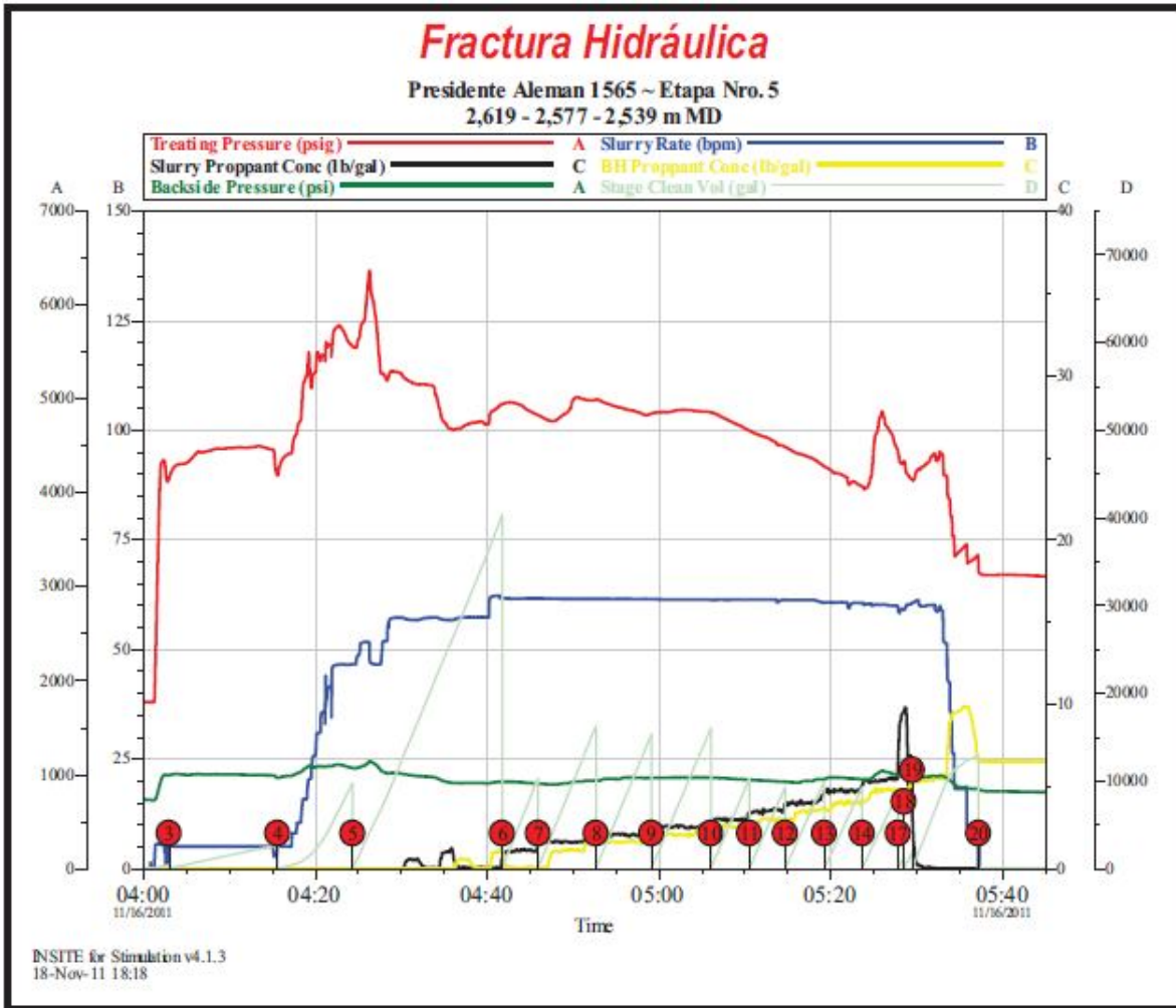
Figura 6.6 Comportamiento de presiones durante el bombeo de ácido y apuntalante de la etapa 5
