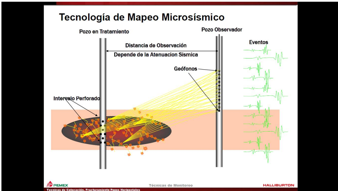
Figura 6.8 Tecnología de mapeo microsísmico
