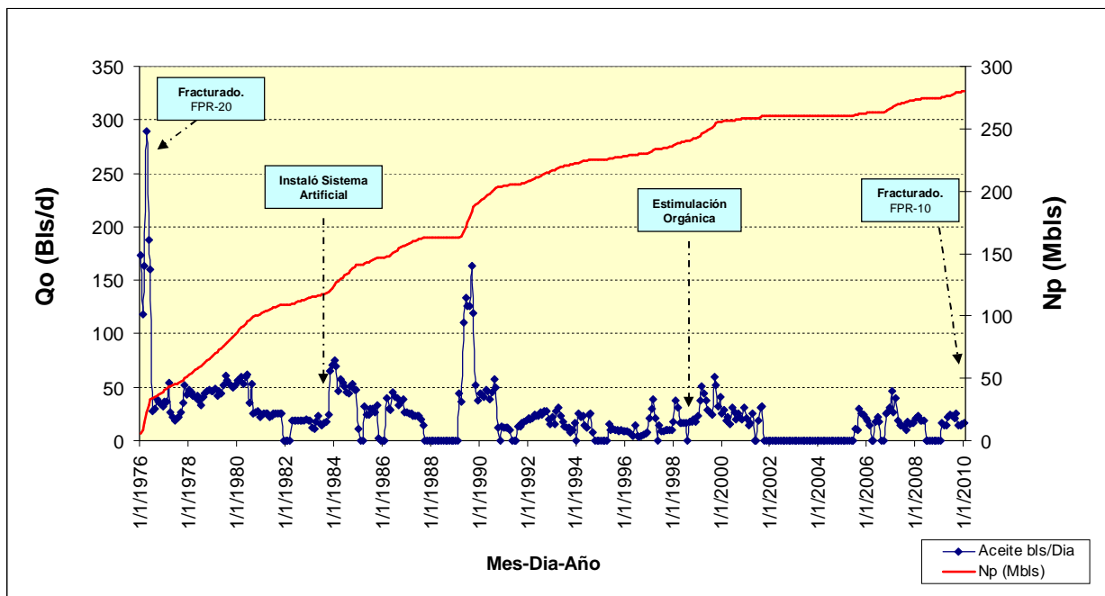
Figura 4.7 Histórico de Producción
