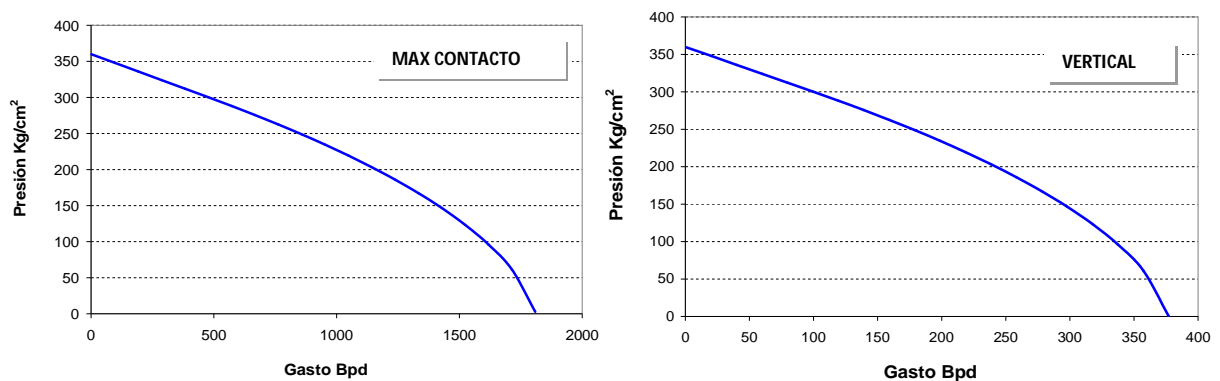
Figura 4.27 Curva de Afluencia Pozo Vertical vs Máximo Contacto, 5 Fracturas
