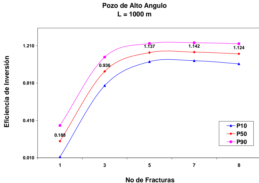
Figura 4.19 Eficiencia de inversión vs número de fracturas
