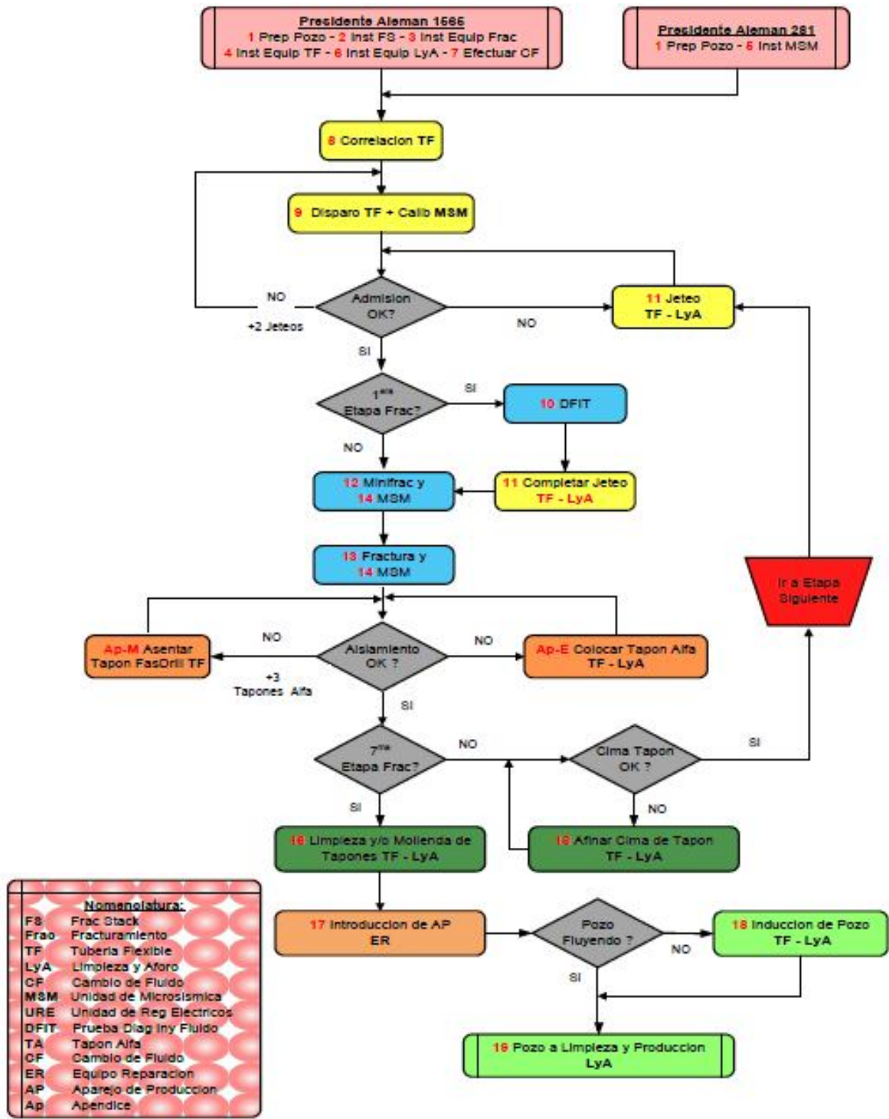
Figura 6.1 Flujo de trabajo para la ejecución de los trabajos de terminación.
