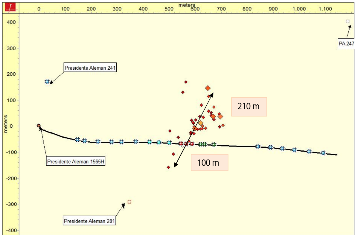
Figura 6.9 Vista de planta etapa 3
