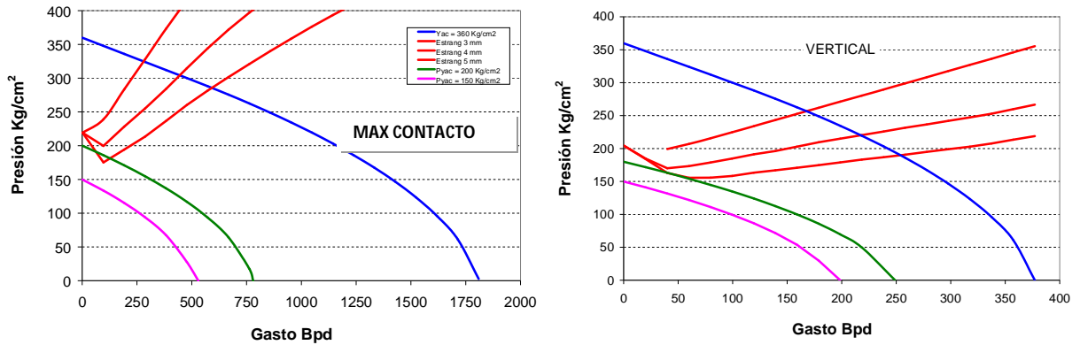
Figura 4.30 Sensibilidad a la Presión de Yacimiento
