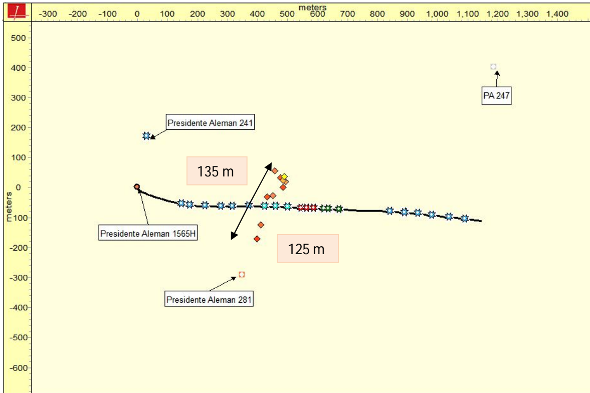
Figura 6.10 Vista de planta etapa 5
