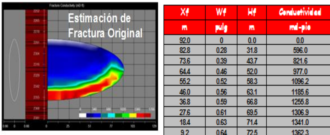
Figura 4.8 Estimación de Fractura Original
