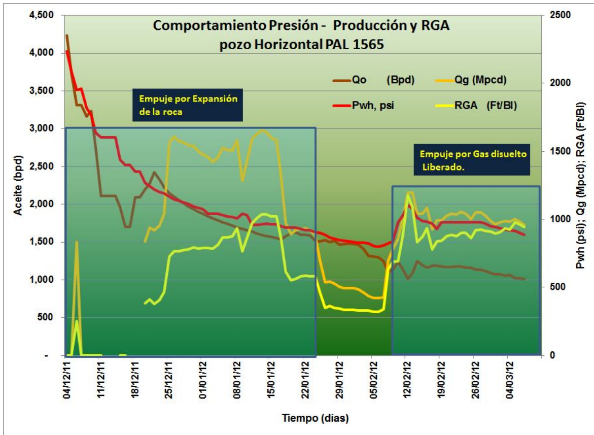
Figura 6.12 Comportamiento presión-producción PA-1565
