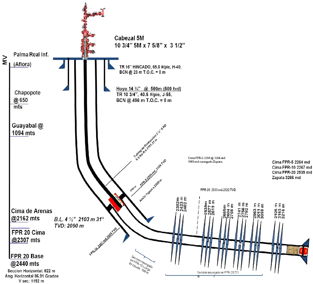
Figura 6.11 Estado mecánico final del pozo PA 1565
