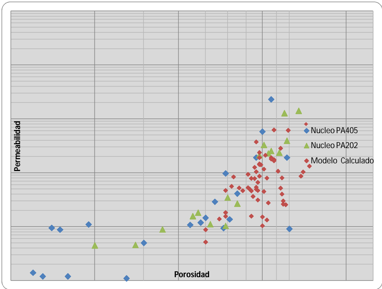
Figura 3.3 Relación de K vs \phi (Análisis de Núcleos contra Calculados en la Unidad FPR20)
