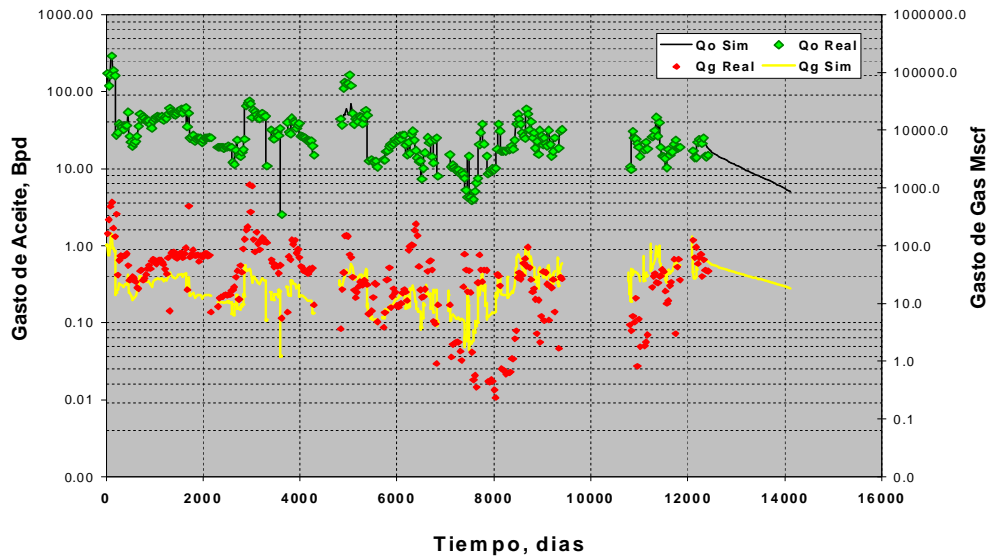
Figura 4.9 Histórico de producción simulado vs real
