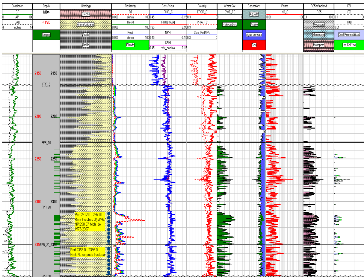
Figura 3.6 Evaluación Petrofísica PA 241
