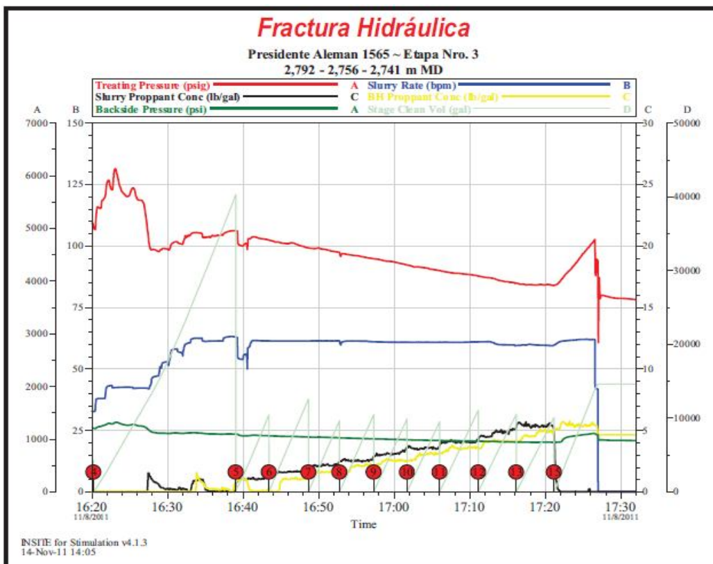
Figura 6.3 Comportamiento de presiones durante el bombeo de ácido y apuntalante de la etapa 3
