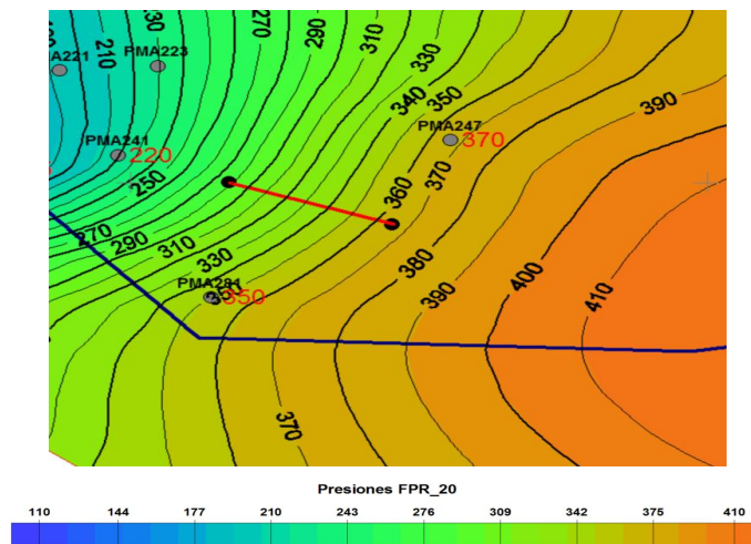
Figura 4.22 Mapa de Presiones. Unidad FPR-20
