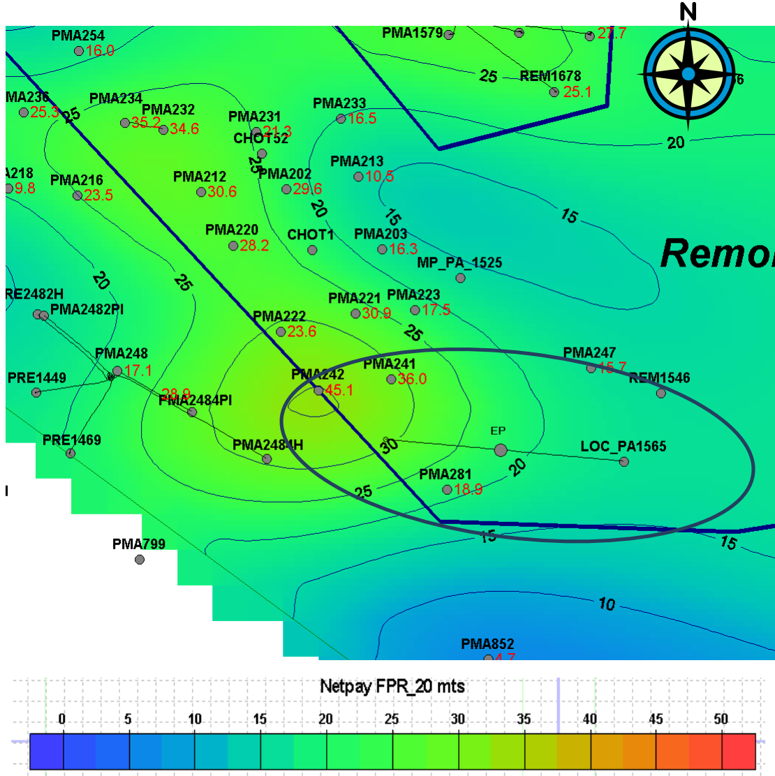
Figura 3.8 Mapa Espesor Neto FPR 20
