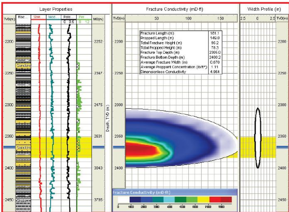
Figura 6.4 Geometría de la Fractura de la etapa 3.
