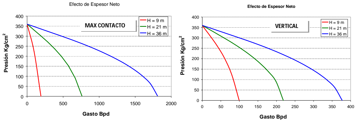
Figura 4.28 Sensibilidad al Espesor Neto Petrolífero
