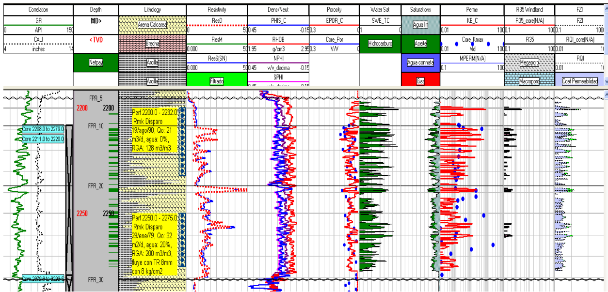
Figura 3.4 Pozo PA 405 (Con Datos de Núcleo)
