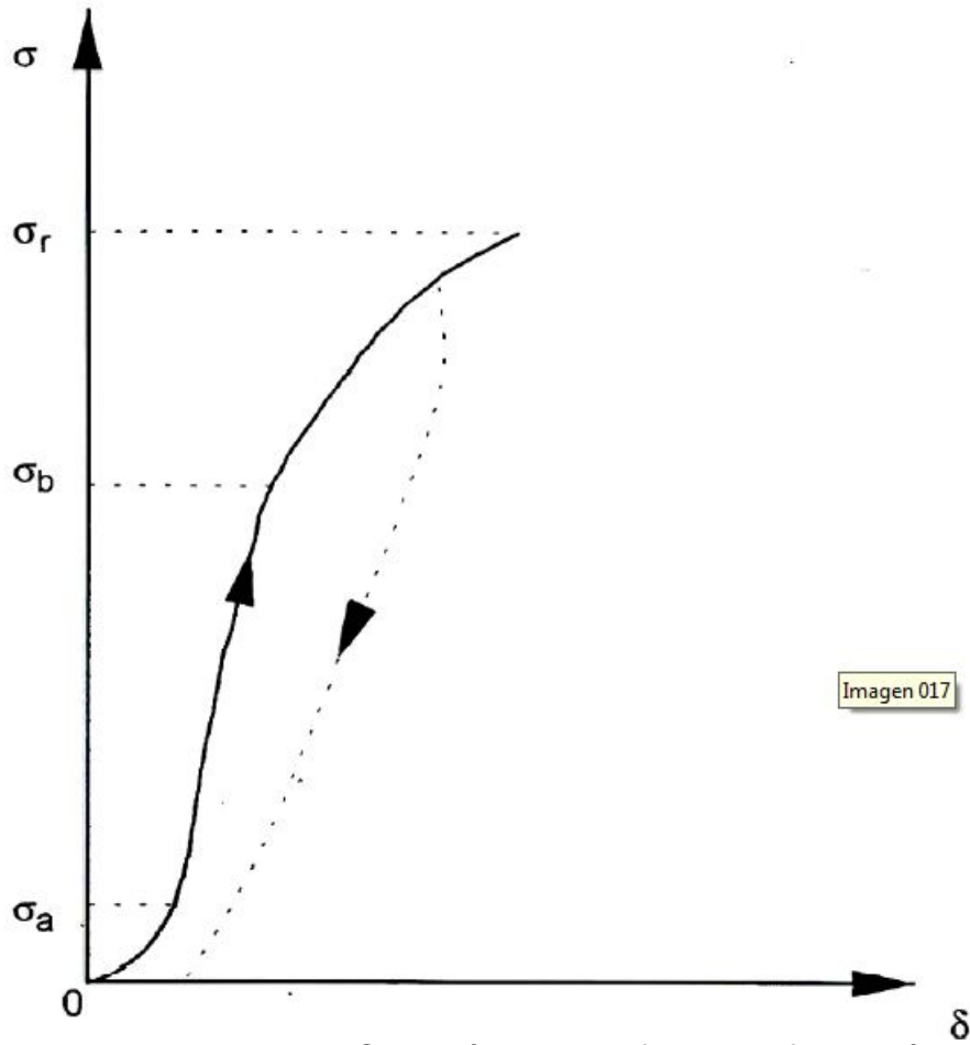
Figura 5.2. Curva típica de esfuerzo-deformación.
