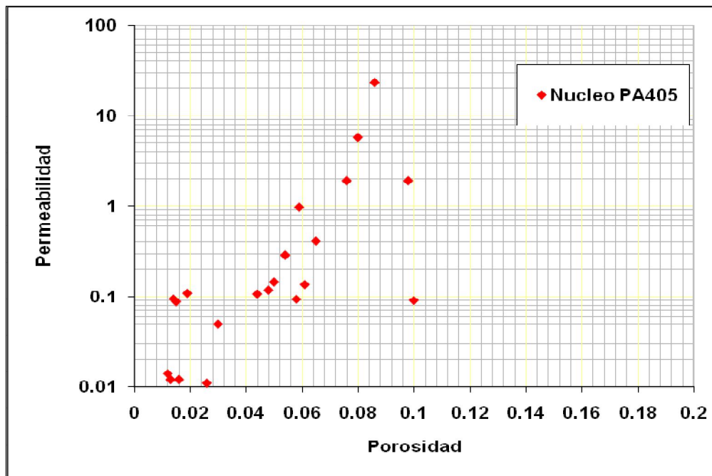
Figura 3.1 Relación de K vs \phi (Análisis de Núcleo PA 405 - Unidad FPR 20)
