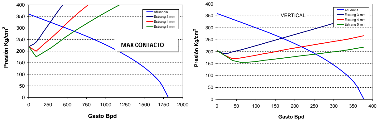
Figura 4.29 Sensibilidades al Diámetro de Estrangulador
