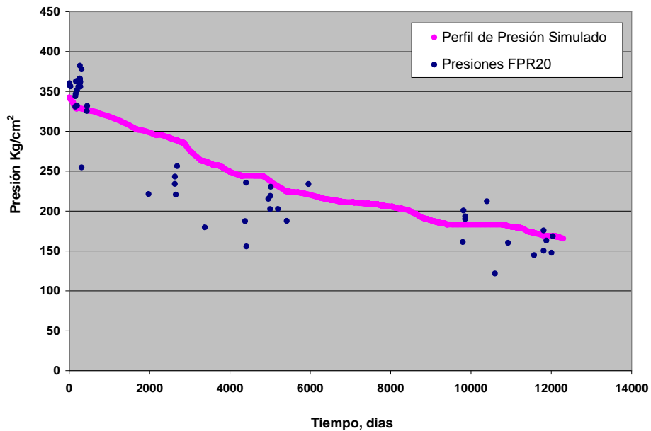
Figura 4.10 Perfil de Presiones Simulado vs Real
