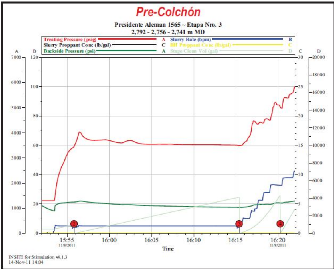
Figura 6.2 Comportamiento de presiones durante el Pre-colchón de la etapa no. 3
