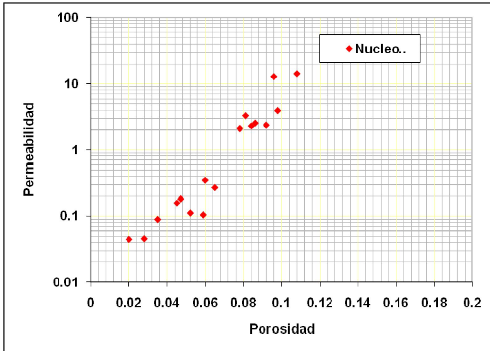
Figura 3.2 Relación de K vs \phi (Análisis de Núcleos PA 202 - Unidad FPR 20)
