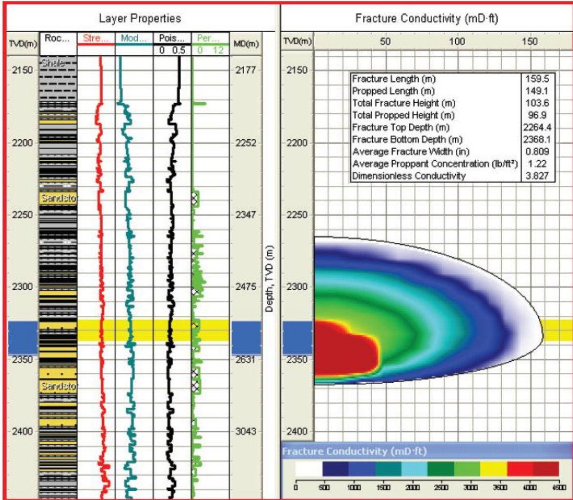
Figura 6.7 Geometría de la Fractura de la etapa 5.
