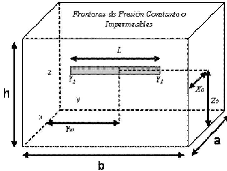
Figura 4.26 Modelo de Afluencia para Pozo Horizontal.
