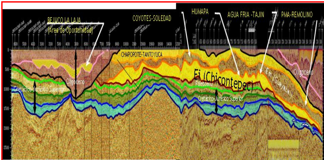
Figura 2.1 Sección Longitudinal NW – SE
