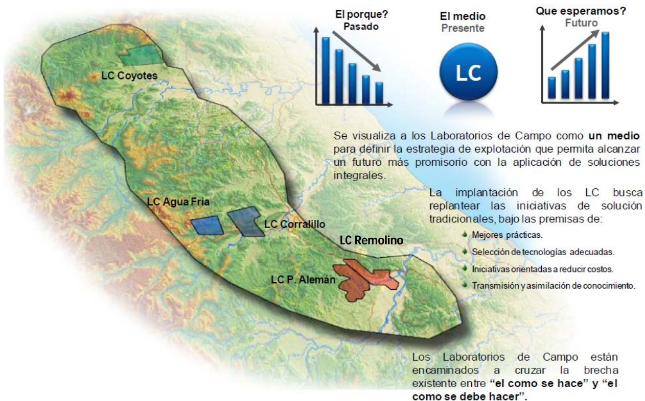
Figura 1.2 Ubicación de los Laboratorios de Campo en el Paleocanal.
