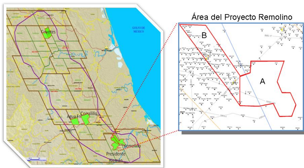
Figura 1.3 Plano de Ubicación del Proyecto Remolino.
