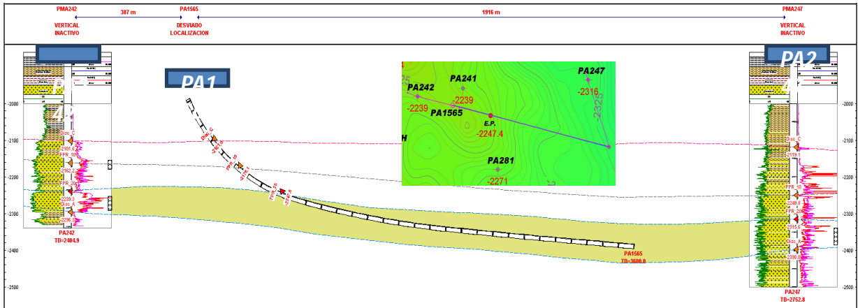
Figura 2.2 Sección Estructural sobre la trayectoria de la localización
