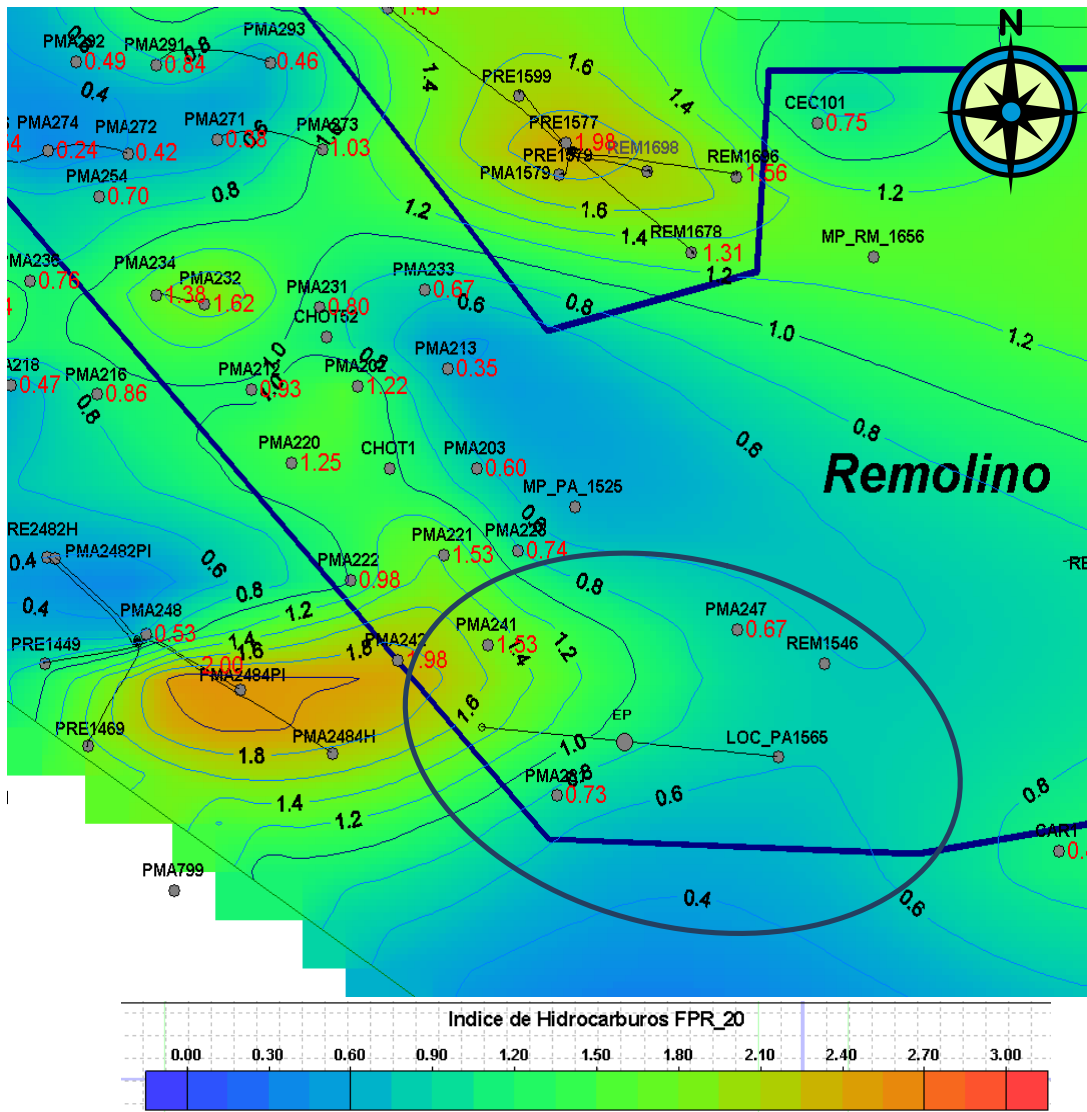
Figura 3.12 Mapa de Índice de Hidrocarburos FPR 20
