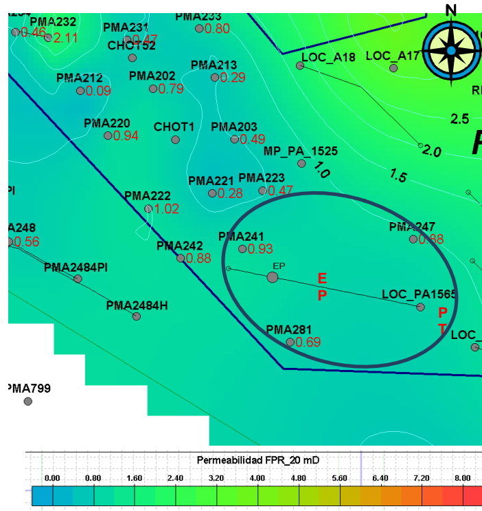
Figura 4.24 Mapa de Permeabilidad. Unidad FPR-20
