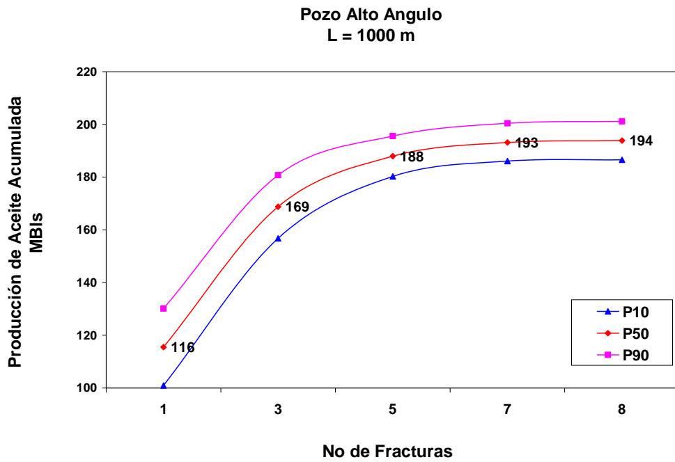
Figura 4.17 Producción de aceite acumulada vs número de fracturas
