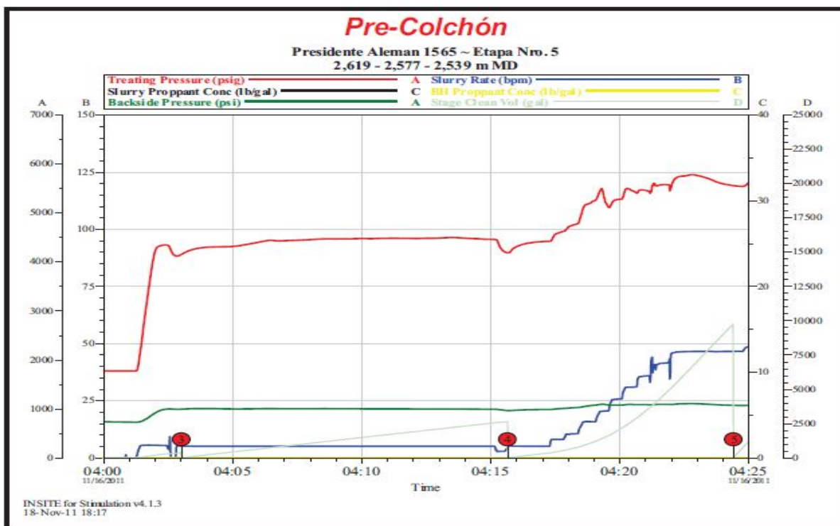
Figura 6.5 Comportamiento de presiones durante el Pre-colchón de la etapa no. 5
