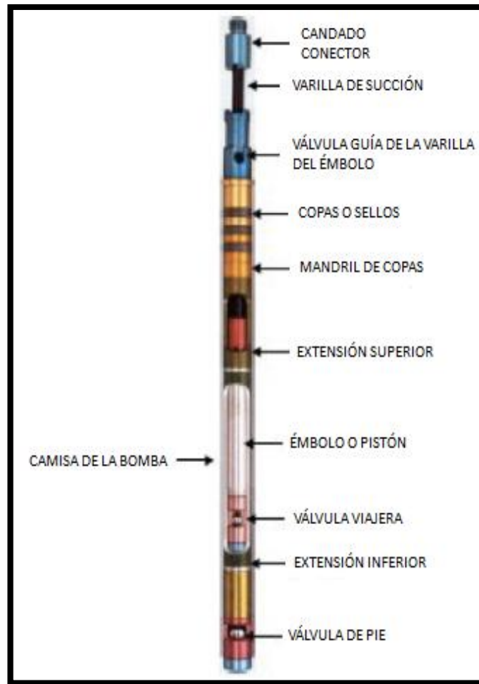
Figura 1.7 Componentes de una bomba subsuperficial de BM.
