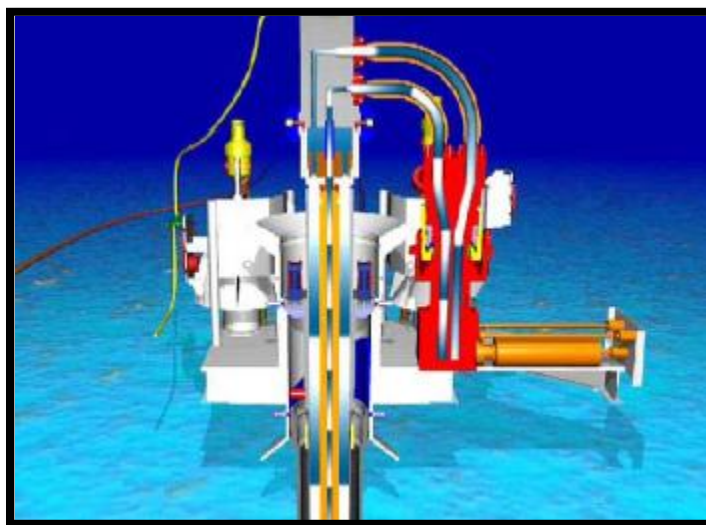
Figura 3.8 Módulo de bombeo. (otc 17398)
