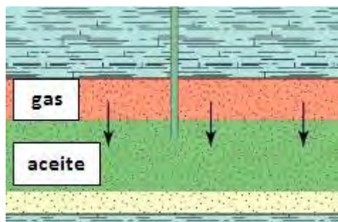
Fig. 3.5 Expansión del casquete de gas.
