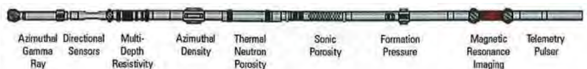
Fig. 19. Sarta de registros LWD/MWD cuádruple combo e imagen de resonancia
