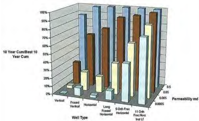
Fig. 22. Comparación de la producción de gas: permeabilidad contra tipos de pozo y de terminación.
