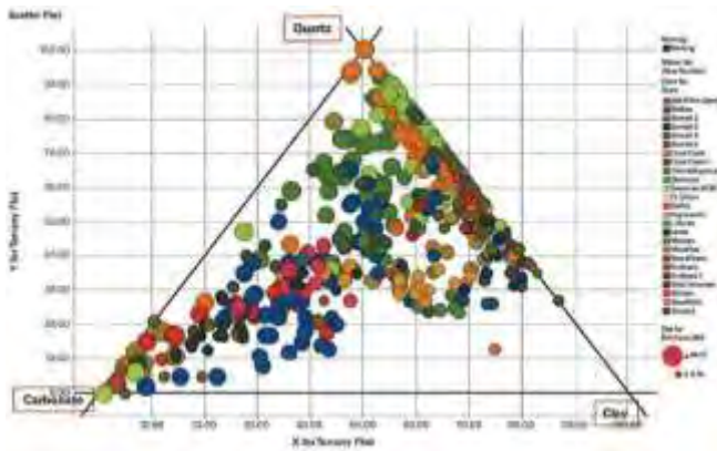
Fig. 5. Gráfica que ilustra la variación en la mineralogía de la lutita para un número de yacimientos productores. Mientras incrementa la reflectancia, la fragilidad decrece; mientras la fracción de cuarzo incrementa, la fragilidad incrementa; y mientras la fracción de carbonatos incrementa, la fragilidad es moderada (Rickman et al. 2008 SPE 115258).
