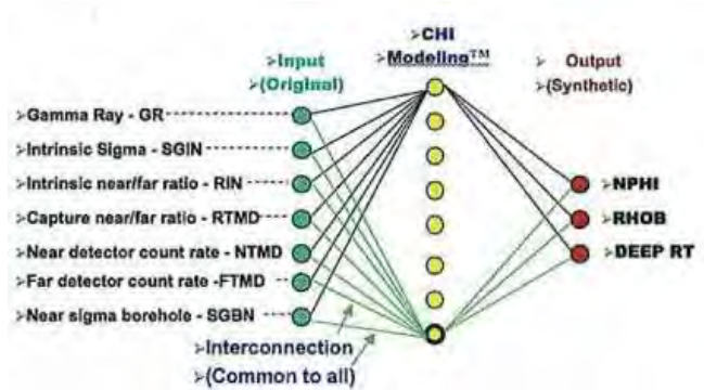
Fig. 20. Generación sintética de resultados del triple combo por medio de la herramienta de neutrón pulsado y modelado Chi
