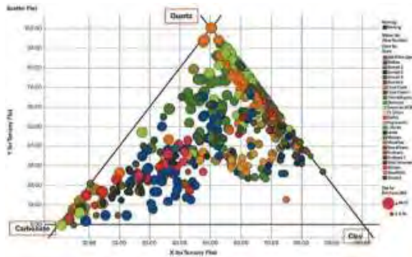
Fig. 10. Grafica que ilustra la variación en la mineralogía de la lutita para un número de yacimientos productores (Rickman et al. 2008 SPE 115258).
