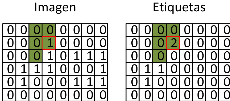
Figura 3.11 12 Recorrido de imagen binarizada y generación de la matriz de etiquetas.
