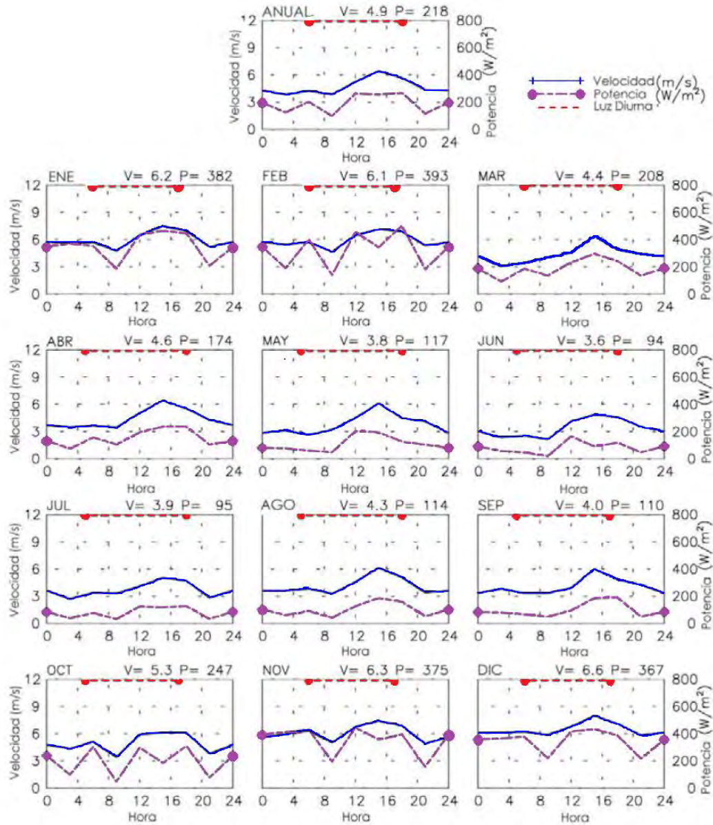
Figura 5.2 Gráficas de disponibilidad del recurso eólico en Salina Cruz
