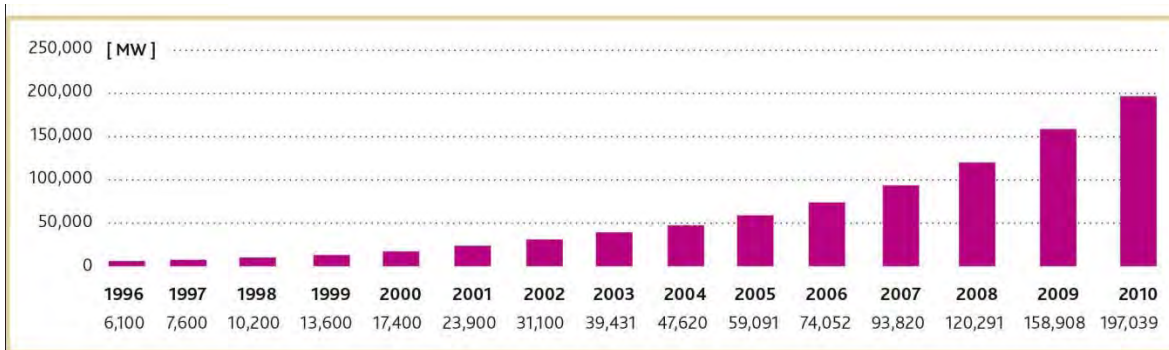
Figura 1.2 Evolución de la capacidad instalada en energía eólica en el Mundo.
