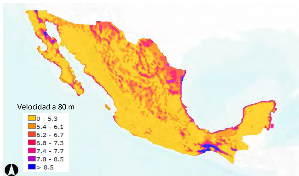
Figura 1.4 Recurso eólico en México, velocidades del viento a 80 m
