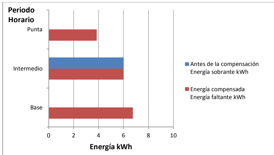
Figura 4.2 Compensaciones en periodos horarios diferentes, tarifas Marzo 2011
