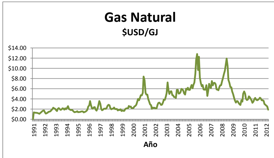
Figura 3.2 Histórico del precio del Gas Natural 1991-2012, $USD/GJ
