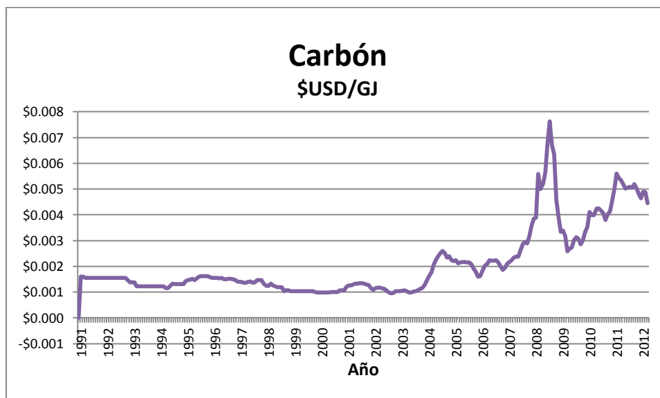
Figura 3.3 Histórico del precio del Carbón 1991-2012, $USD/GJ
