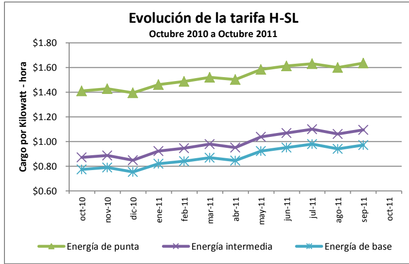
Figura 5.1 Evolución de la tarifa H-SL (Alta Tensión) de Oct. 2010 a Oct. 2011
