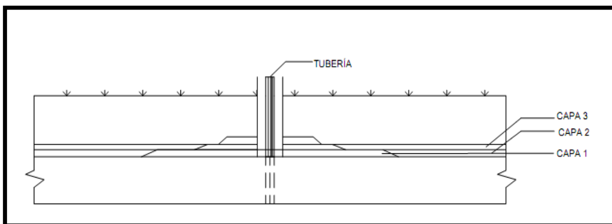
Fig. 4.7 Tubería
