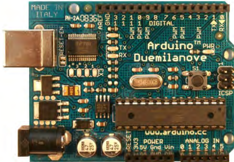
Figura 7. Arduino Duemilanove [12]
