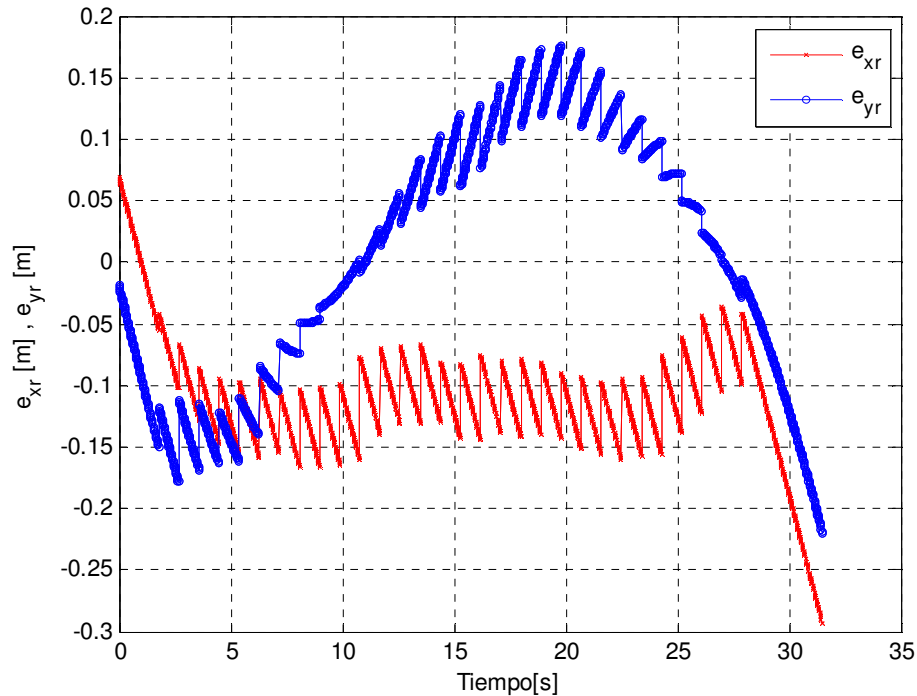
Figura 37. Error de seguimiento del punto de referencia del Robot Móvil.
