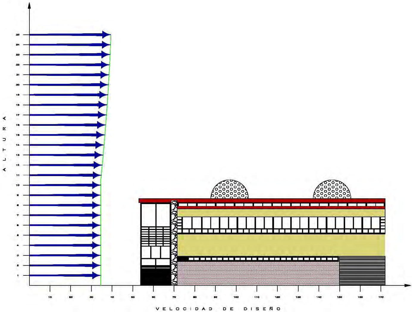
FIG. 3.8 DISTRIBUCION DE LA VELOCIDAD DE DISEÑO DEL VIENTO CON RESPECTO A LA ALTURA
