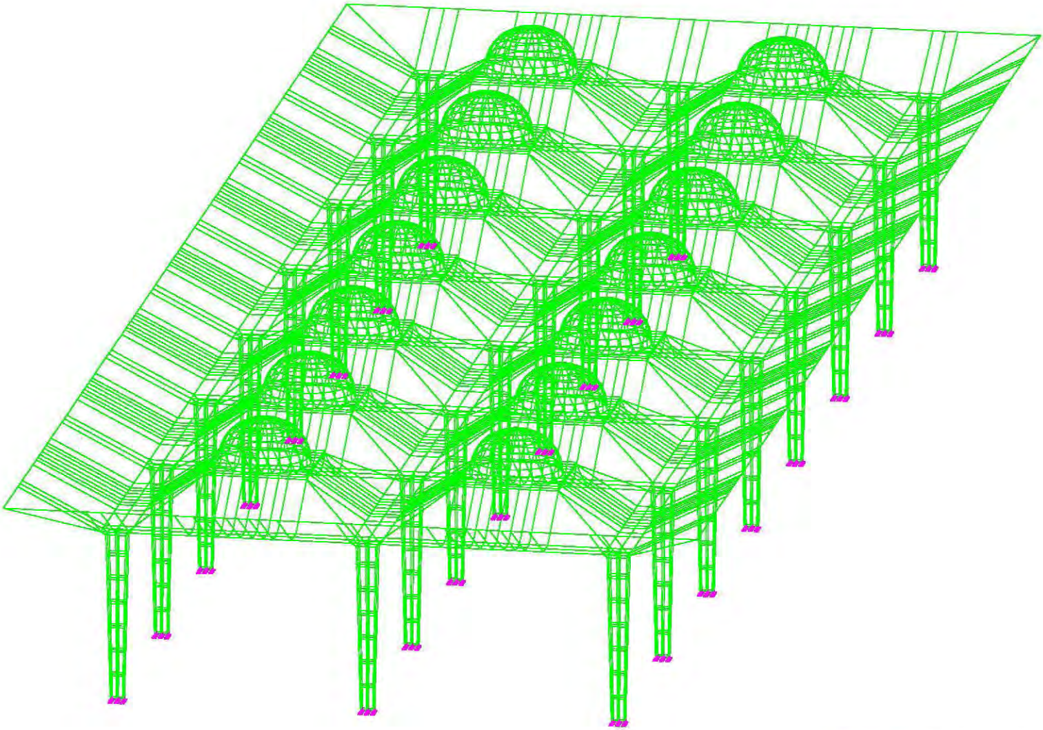
FIG. 3.2 ISOMÉTRICO 2
