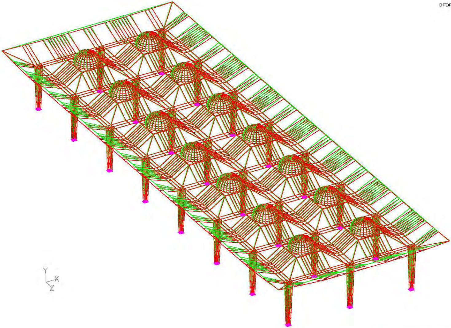
FIG. 4.1 ISOMÉTRICO 5 DESPLAZAMIENTOS DE COMBINACION DE CARGA 16
