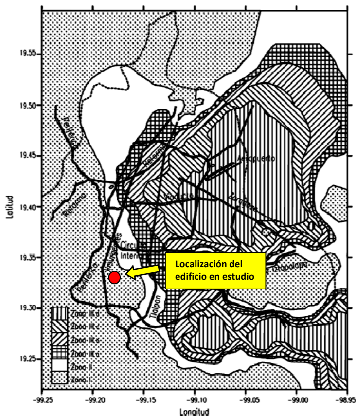
IMAGEN 2.5 ZONIFICACIÓN GEOTÉCNICA DE LA CIUDAD DE MÉXICO
