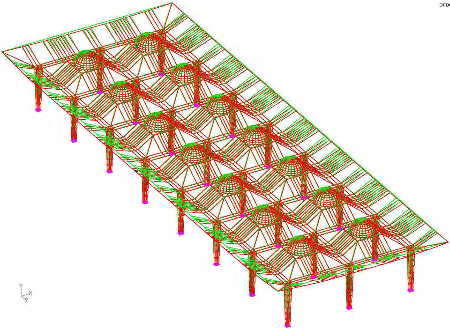
FIG. 4.5 ISOMÉRICO 9 DESPLAZAMIENTOS DE CARGA No. 20
