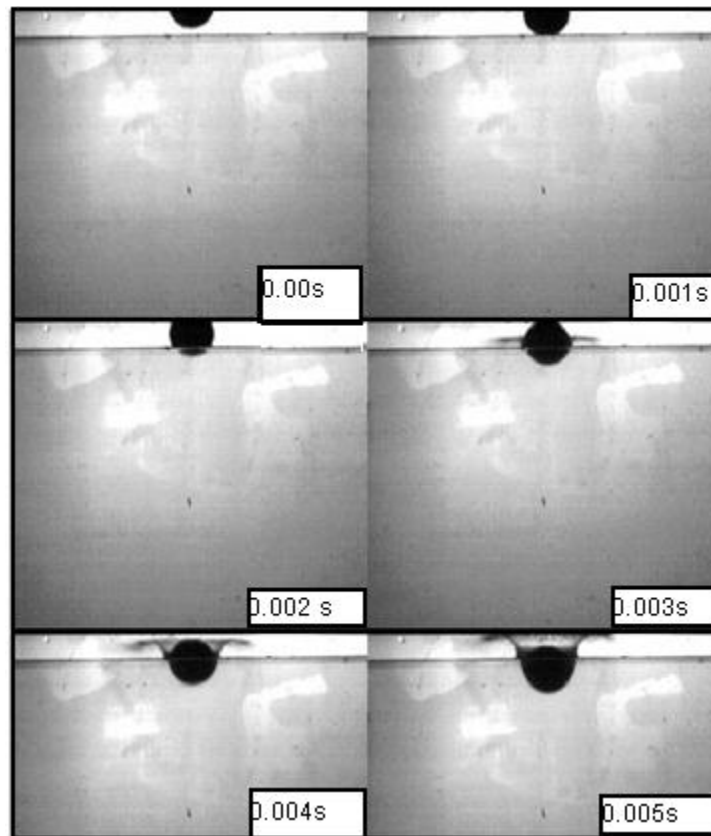
Figura 5. Contacto de la esfera con el agua desde el tiempo 0 al tiempo al 0.005 s. La esfera se impacta con una velocidad de 3.5 m/s
