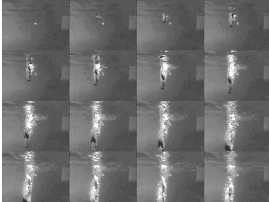
Figura 4. Entrada de un clavadista vista por medio de una pared de cristal para visualizar los efectos de los impactos de un cuerpo humano con el agua. Fotos tomadas después de la caída de la figura 3.
