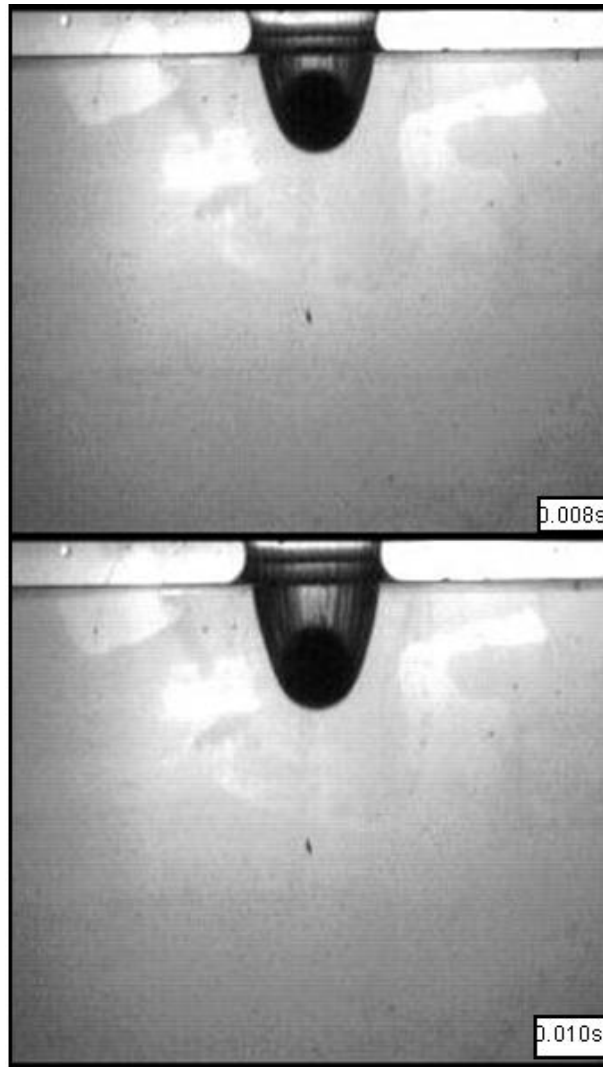
Figura 6 Formación de la cavidad por el impacto de una esfera de aluminio a 3.5 m/s para tiempos de 0.008 s a 0.010 s.
