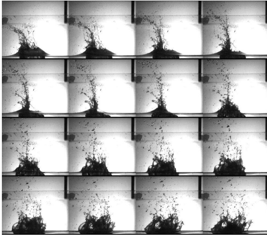
Figura 28. Pln zamamiento después de que cae el modelo a escala al agua.
