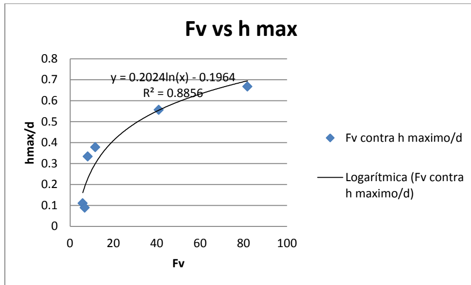
Figura 21. Variación del comportamiento del ancho de la cavidad con diferentes velocidades
