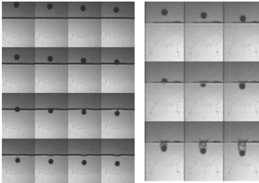
Figura 22. Secuencia fotográfica de la caída de un balón de plástico en agua para un cierre gentil
