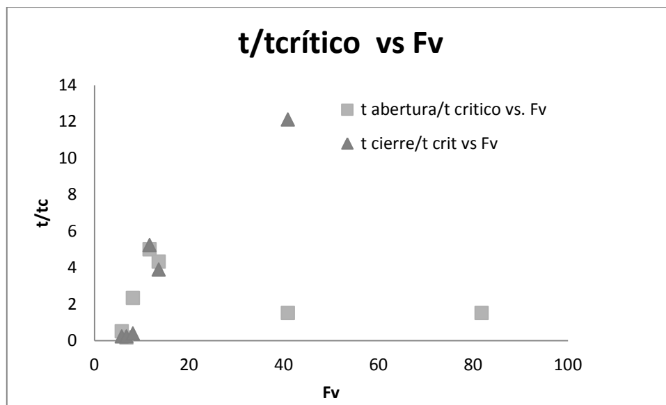
Figura 20. Comportamiento del tiempo de abertura y tiempo de cierre respecto a la velocidad
