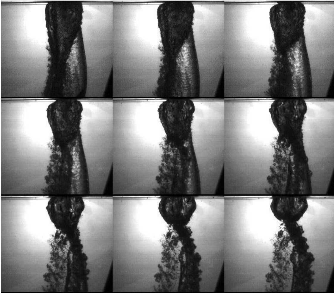
Figura 27 Cierre de la cavidad para el clavadista hecho a escala.
