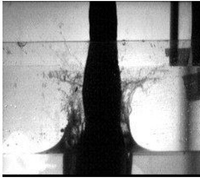
Figura 29. Fotografía del impacto del modelo para el primer caso.
