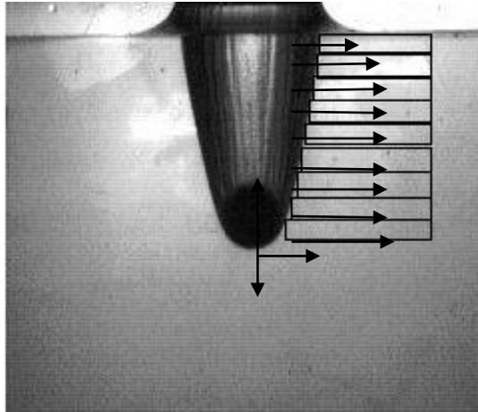
Figura 14 .Corte en el plano XY para la representación placas de agua durante la formación de la cavidad.
