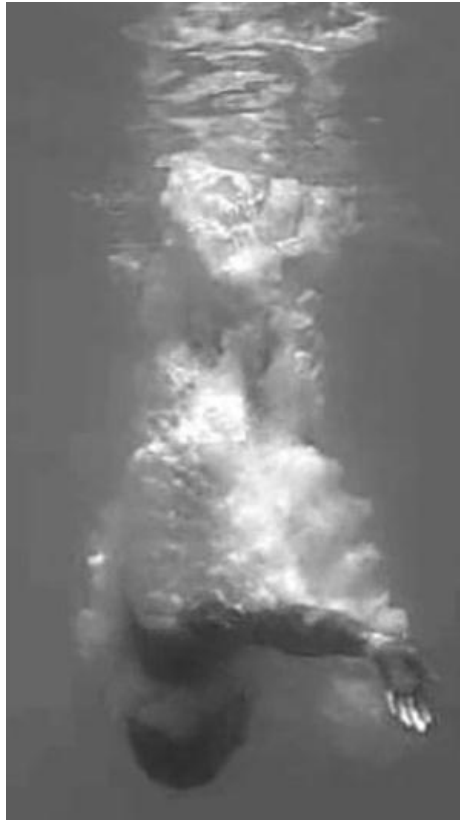
Figura 1. Imagen de la entrada al agua en un clavado típico (toma bajo la superficie)
