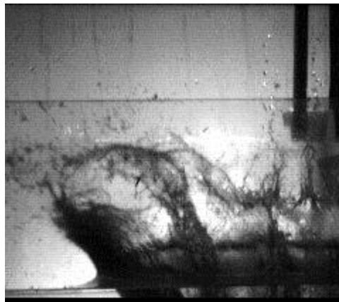
Figura 31. Formación de la cavidad para un modelo para el tercer caso
