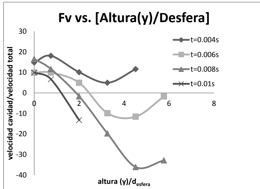
Figura 16. Comportamiento de la velocidad de la abertura de la cavidad respecto de t=0.004 s a t=0.01 s
