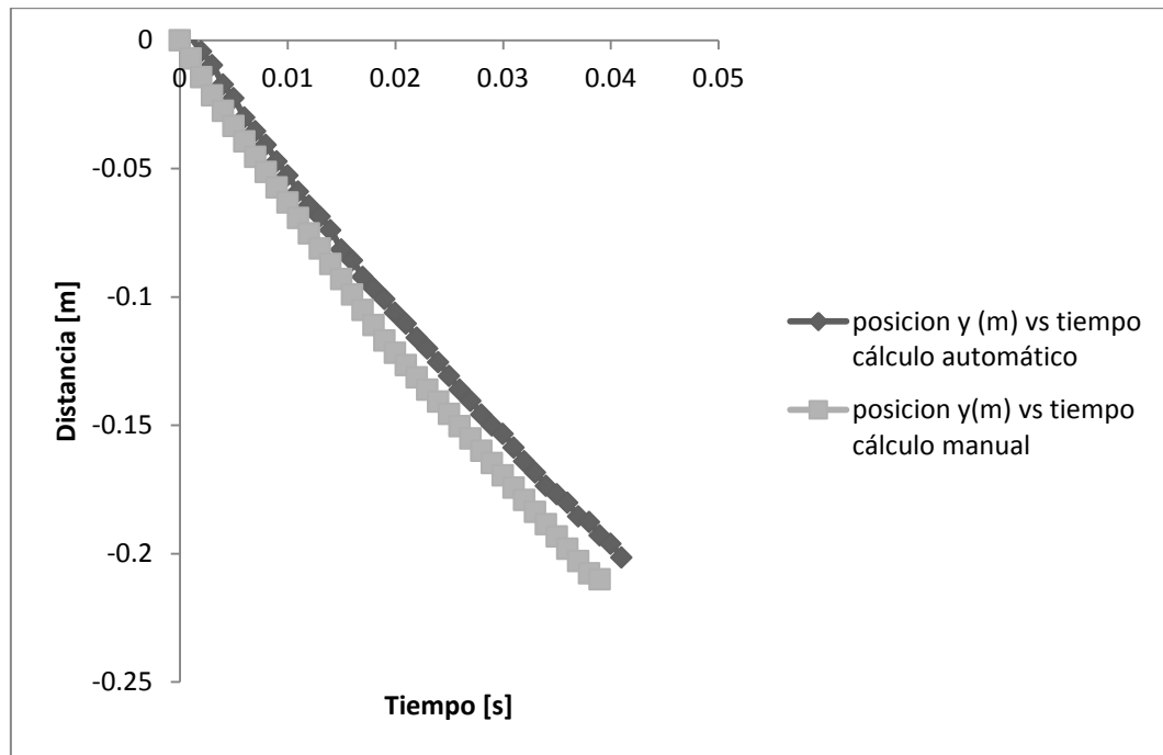
Figura 12. Comportamiento de la posición de la esfera respecto al tiempo
