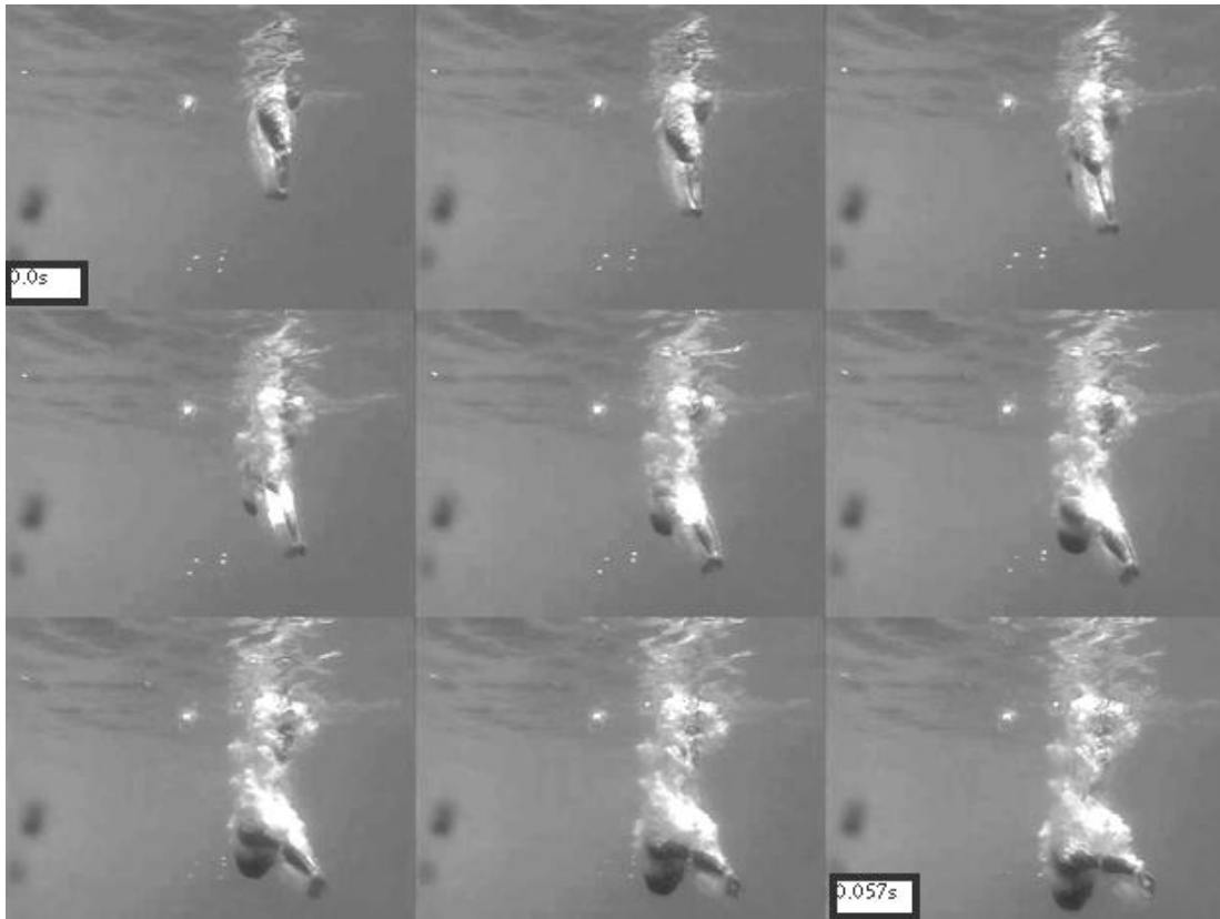
Figura 33 Movimiento de brazos después del contacto con el agua
