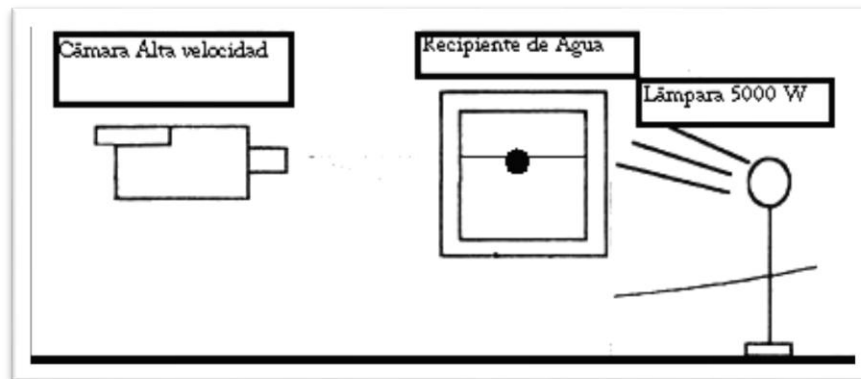
Diagrama 1. Muestra la colocación del material para la grabación de esferas y modelos a escala.
