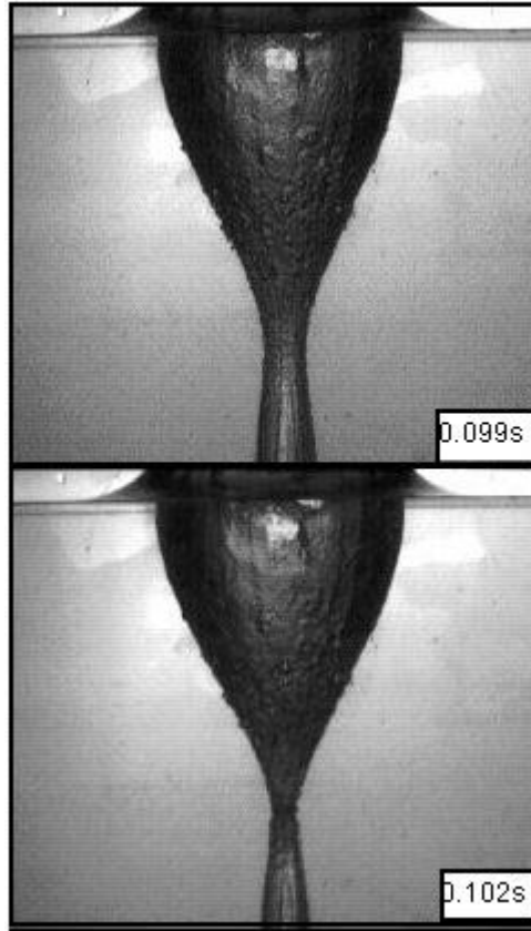
Figura 8. División de la cavidad en una cavidad grande y una burbuja de menor tamaño del segundo 0.099 al segundo 0.102.
