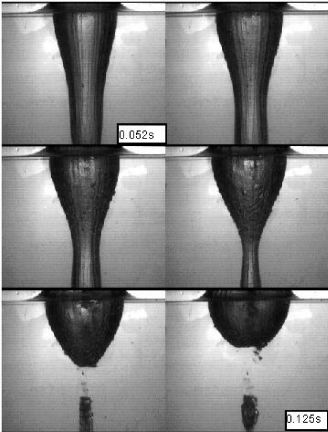
Figura 9. División completa de la burbuja de la cavidad y comienzo del cierre de la cavidad del segundo 0.052 al segundo 0.125.
