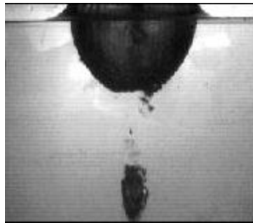
Figura 2. Imagen tomada después del colapso de la cavidad. Se observa el salpicado en la superficie y una burbuja remanente
