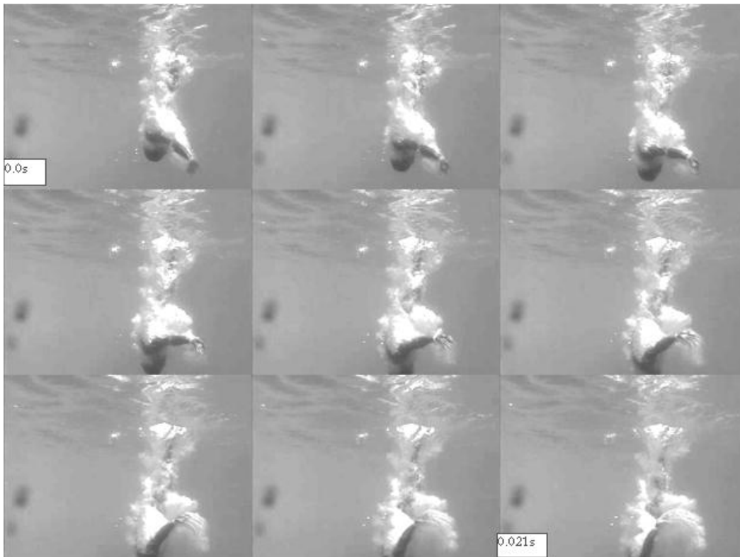
Figura 34 Técnica con movimiento lateral de brazos
