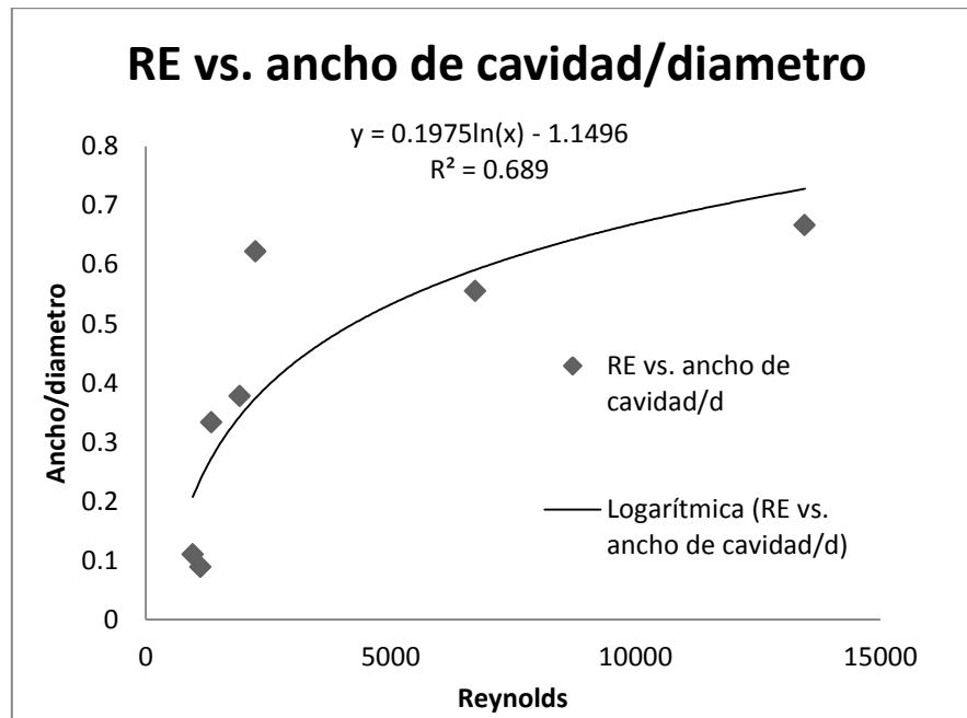
Figura 24. Gráfica de ancho/diámetro respecto al Número de Reynolds.
