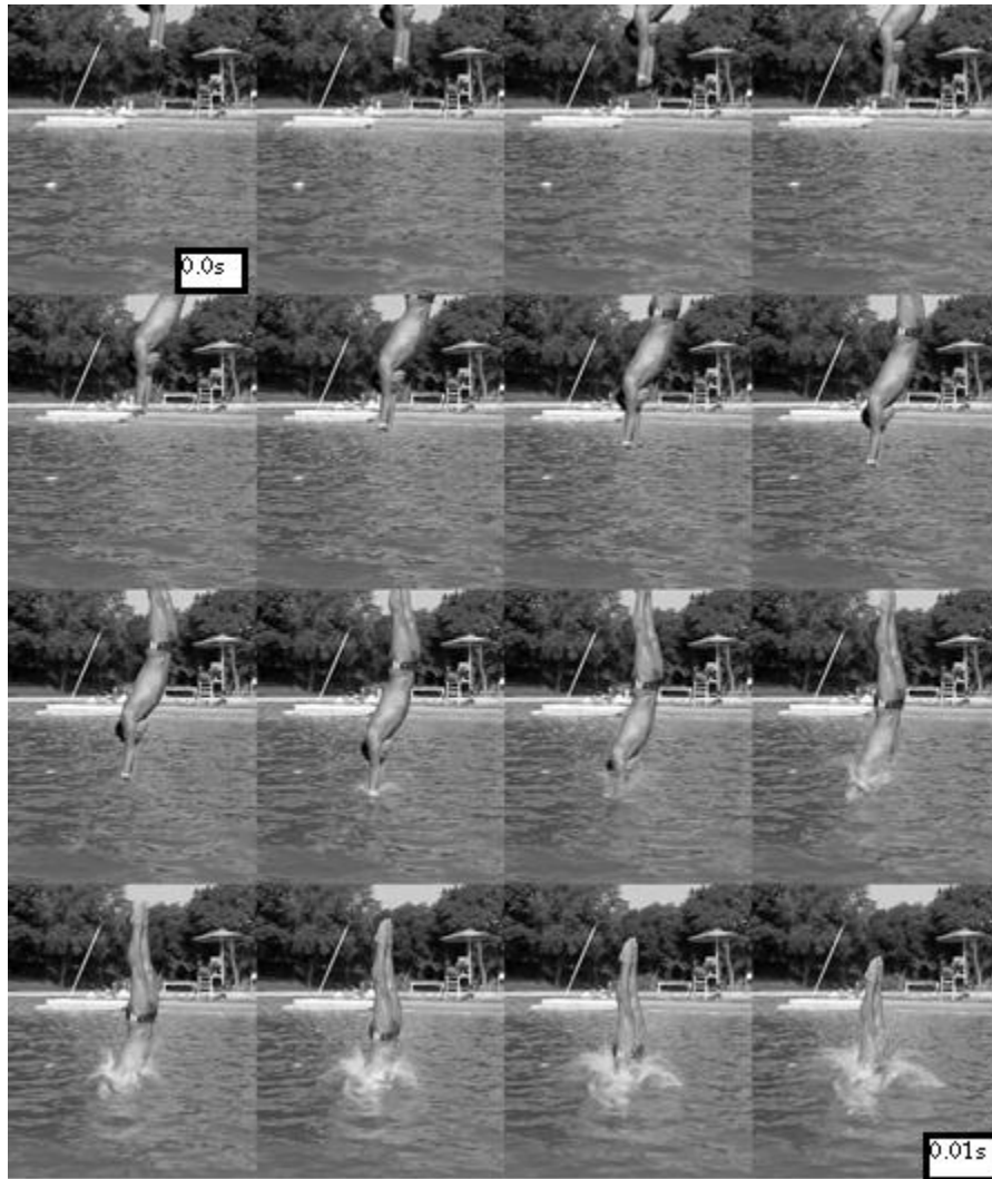
Figura 3 .Imágenes tomadas a partir de la entrada de un clavadista al agua.
