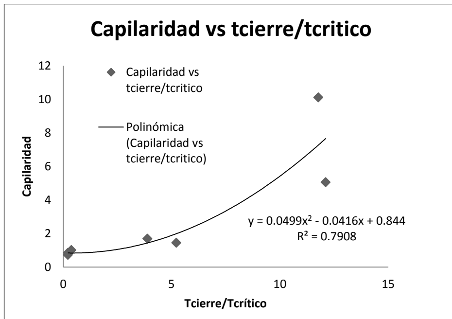
Figura 23. Gráfica de la capilaridad respecto al tiempo adimensional.
