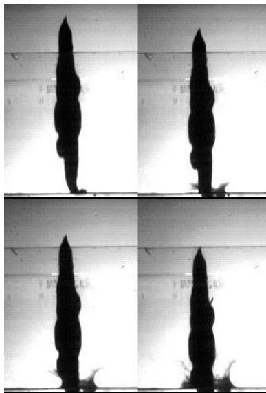
Figura 25. Primeras fases del choque de un clavadista a escala hecho de plastilina y cobre.
