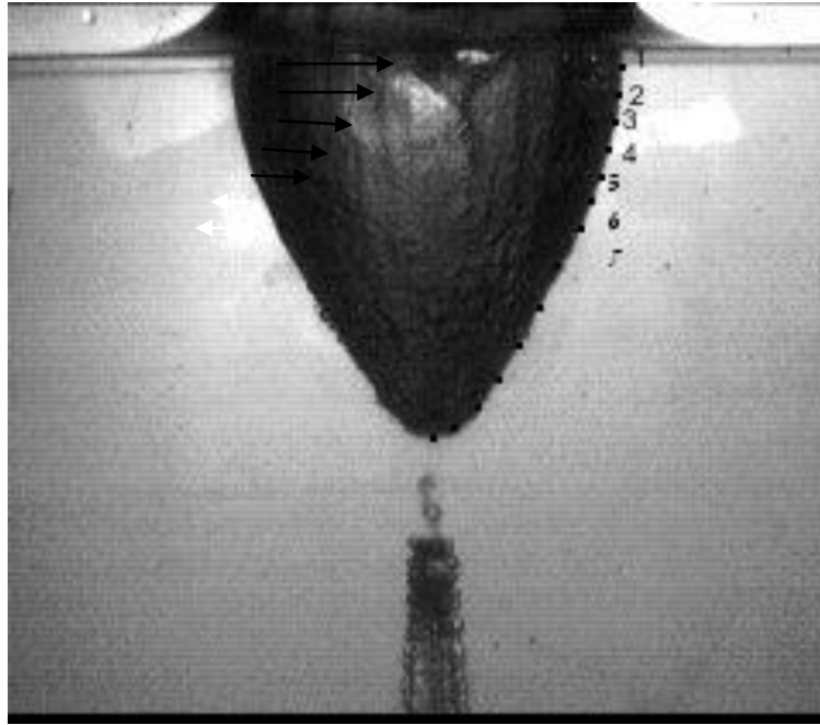
Figura 17. Comportamiento de las velocidades después de la separación de los principales cuerpos de aire.
