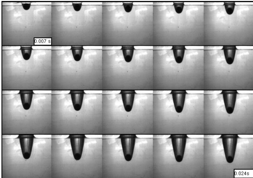
Figura 7 Alargamiento de la cavidad con el desplazamiento de la esfera en el líquido.
