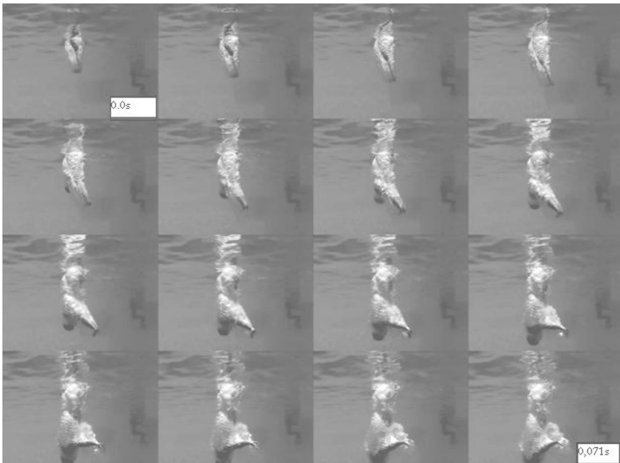
Figura 35. Movimiento frontal de brazos para la formación de la cavidad para un clavadista
