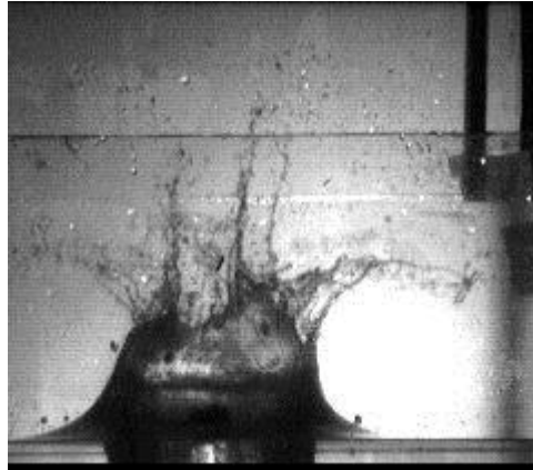
Figura 30. Fotografía del impacto del modelo escala para el segundo caso
