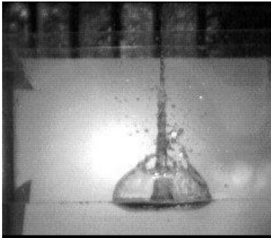
Figura 19 Cambio de ancho en “x” del pinzamiento con el cambio de altura “y”.
