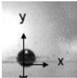
Figura 11. Ejes tomados para el análisis de la esfera
