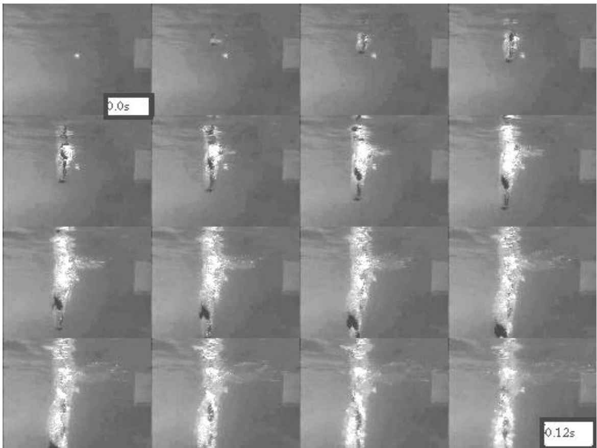
Figura 32 Entrada de clavadista al agua sin movimiento de brazos
