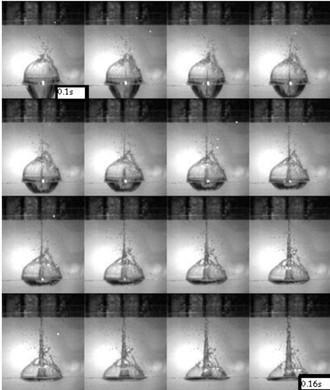
Figura 10. Secuencia fotográfica de comportamiento del impulso arriba de la superficie de agua
