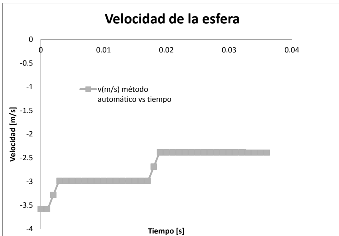
Figura 13 Comportamiento la Velocidad V_c de la esfera respecto al tiempo.
